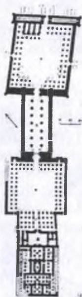
4-rasm. Luksordagi Amon Ra ibodatxonasi. Dastlabki qurilma — birinchi hovlining shimoliy burchagidagi uch xonali ibodatxona umumiy kompozitsion o'qning siniqligiga sabab bo'lgan (6-ad., 21-b.).
