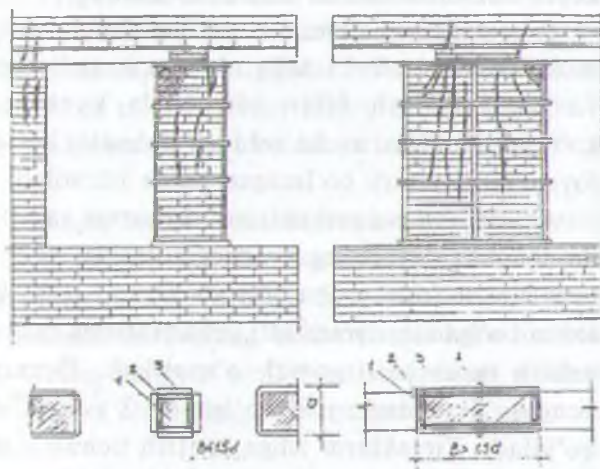
9.4-rasm. Oraliqni po'lat halqa bilan kuchaytirish 1 - to'rtburchakli stolb; 2 - po'lat burchak- lar; 3 - plankalar; 4 - ko'ndalang bog' lovchi.
