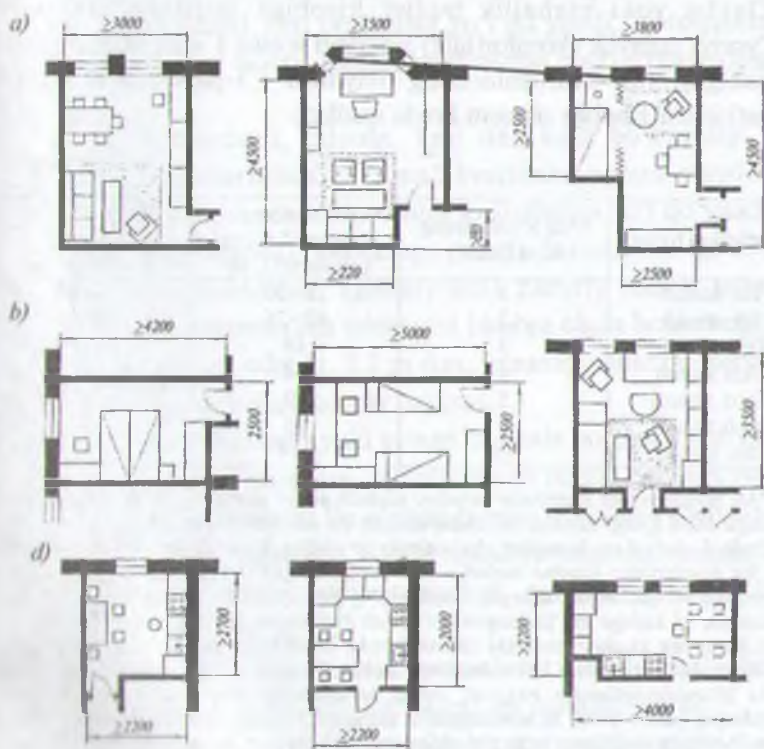
1.19-rasm. Kvartiraning rejayiy elementlari:
