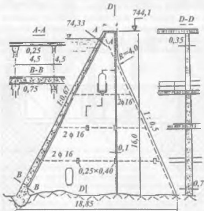
3.13- rasm. Yassi bosim plitalari va issiqlikni saqlash izolatsiyasiga ega bo'lgan yupqa devorli to'g'on:
