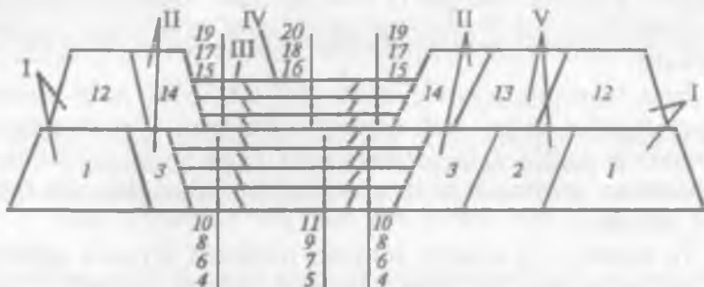
1.9- rasm. O'zakli tosh-tuproq to'g'onni qurish sxemasi: I—20— navbat bilan to'kiladigan gruntlar, I — to'kma tosh, II—III— sizgichning birinchi va ikkinchi qatlamlari, IV— o'zak, V— shag'al.
