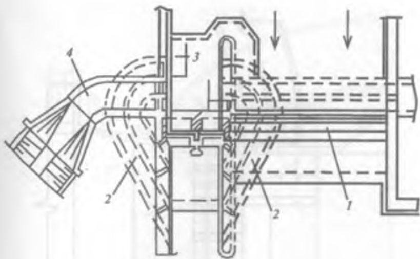
4.2- rasm. Oqindilarni ushlab qoluvchi galereyalari bo'lgan yon tomondan ikki tarafga suv olinadigan gidrotexnika inshootlari bo'g'ini: 1—suv tashlagich; 2—oqindilarni ushlab qoluvchi galereyalar; 3—yo'lak; 4—kanal.
