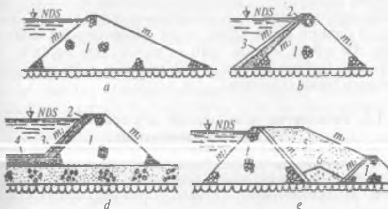
1.7- rasm. Portlatib uloqtirish yo'li bilan quriladigan to'g'onlarning turlari: a—bir jinsli; b—to'sqichli; d—to'sqich va ponurli; e—portlatib yuviladigan; 1—portlatish yo'li bilan hosil qilingan qoyatoshlar uyumi; 2—to'sqich; 3—gruntning himoya qatlami; 4—ponur; 5—yuvish yo'li bilan yotqiziladigan kam suv o'tkazuvchi bog'lanishli grunt; 6—teskari filtr.
