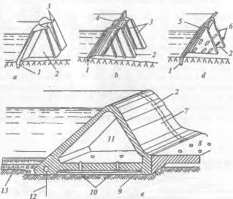
3.10- rasm. Kontroforsli to'g'onlarning sxemalari:
