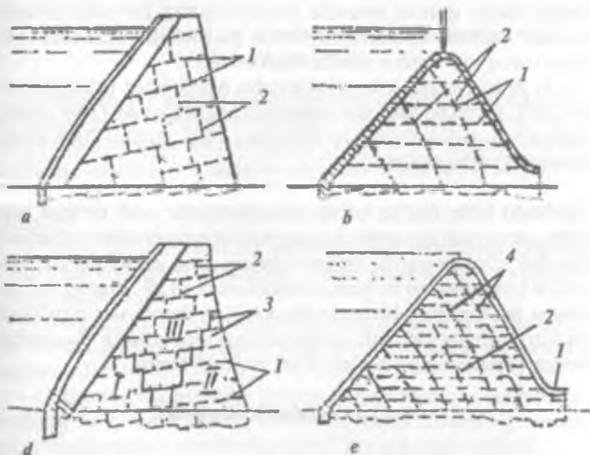
3.19- rasm. Kontroforslardagi choklarning sxemalari:
