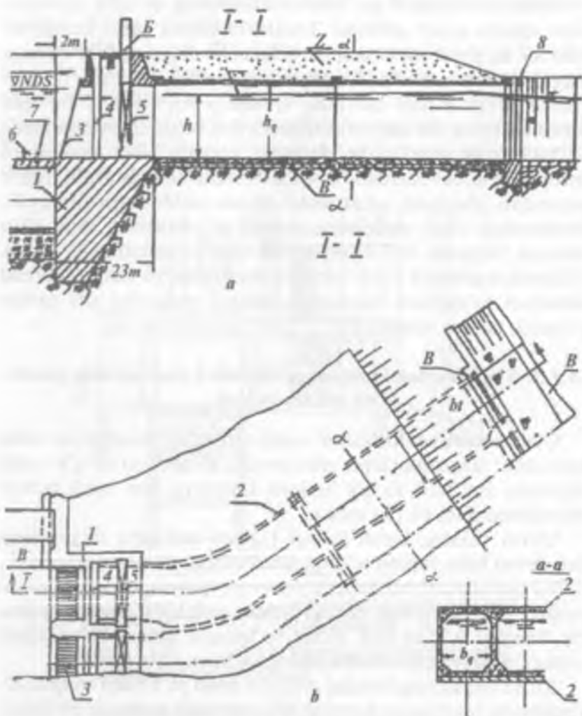
4.13- rasm. Yopiq turdagi yonboshdan suv olish inshootining konstruksiyasi: 1—kirish kallagi; 2—quvur; 3—panjara; 4—ta'mirlash qulfaklarining teshiklari; 5—asosiy qulfaklar; 6—suv tashlama to'g'onning ravoqlari; 7—A.V. Troiskiy tokchasi; 8—chiqish kallagi. I—I, II—II, — bo'ylama va ko'dalang kesimlar.
