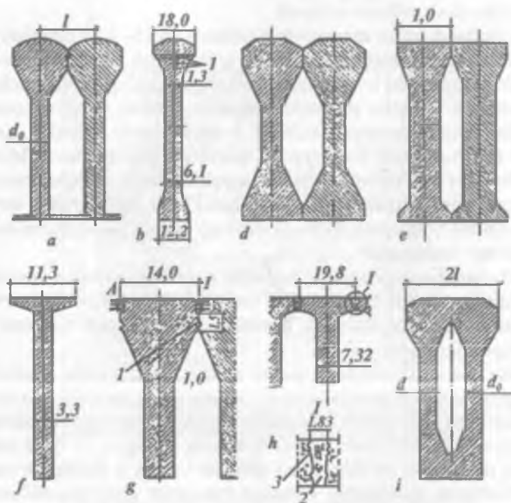
3.15- rasm. Har xil kallakli massiv kontroforsli to'g'onlar kontroforslari gorizontāl kesimlarining sxemalari:
