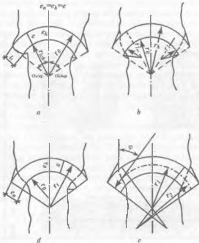
3.6- rasm. Ark halqalari sxemasi:
