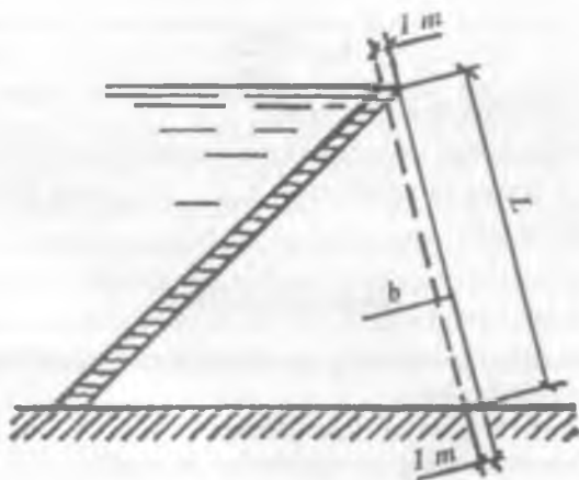
3.20- rasm. Hisoblash sxemasi.
