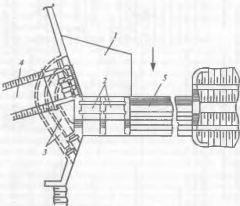
4.1- rasm. Yon tomondan bir tarafga suv olinudigan gidrotexnika inshootlari bo'g'ini:
