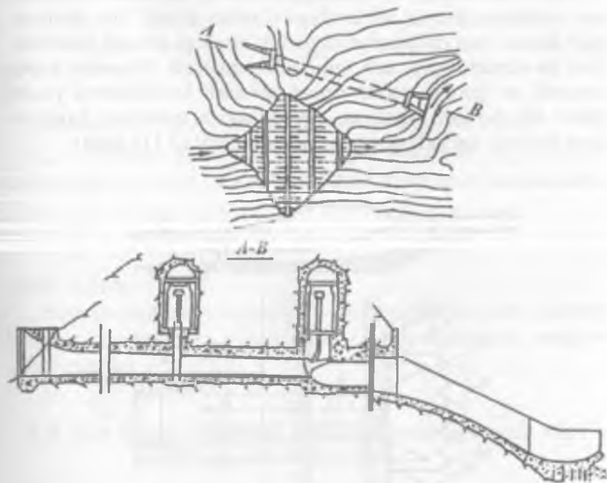
2.10- rasm. Tunnelli suv tashlagich: A— B bo'ylama kesim.
