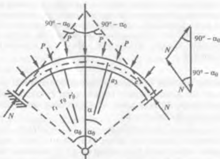
3.8- rasm. To'g'onni bir-biridan alohida ishlaydigan arklar sistemasi sifatida hisoblash sxemasi.
