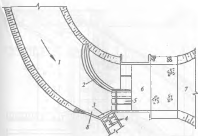
4.6- rasm. Oqimning ko'ndalang sirkulatsiyasidan foydalaniladigan hamda egri chiziqli avtomatik suv tashlagichli gidrotexnika inshootlari bo'g'in:
