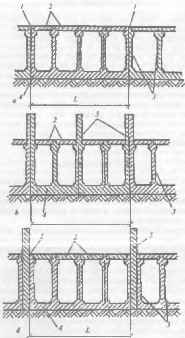
3.18- rasm. Yassi bosim yopmasi va poydevor plitasiga (to'g'onning bo'ylama o'qi bo'ylab vertikal qirgimlarga) ega kontroforli to'g'onlarning temperatura-ga qarab kiritiruvchi choklarini joylashtirish sxemalari:
