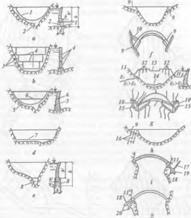
3.2- rasm. Arksimon to'g'onlarning sxemalari:
