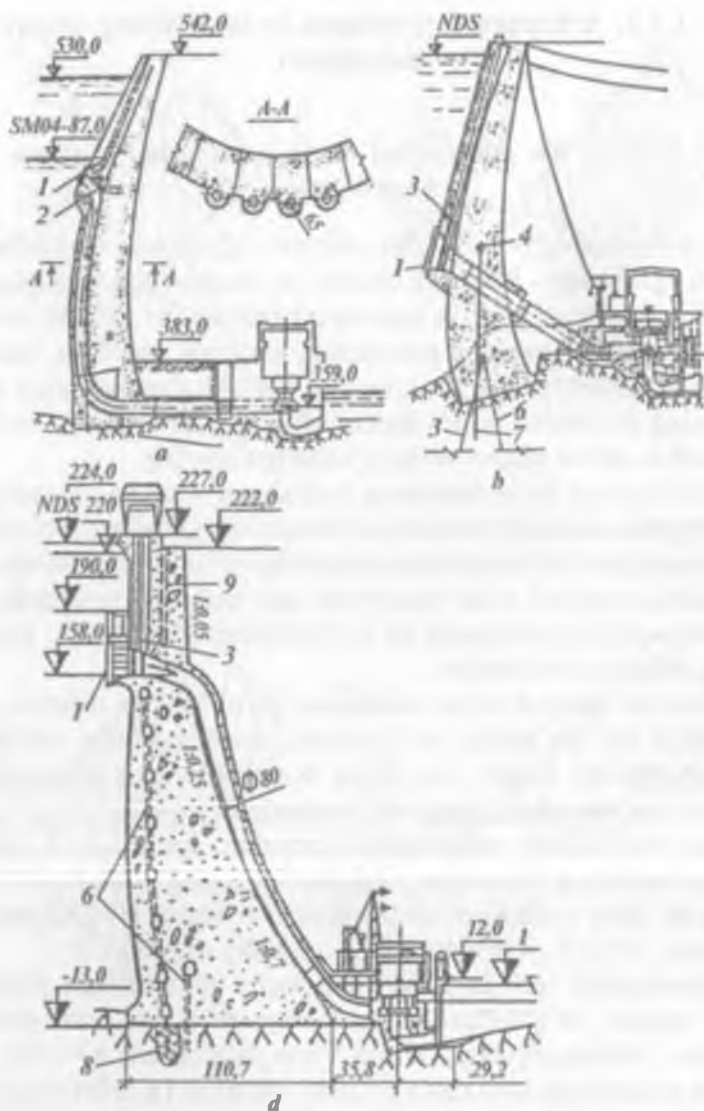
3.4-rasm. Hidroelektrostansiyalarning arksimon to'g'onlaridagi suv qabul qilgichlarning kesimlari:
