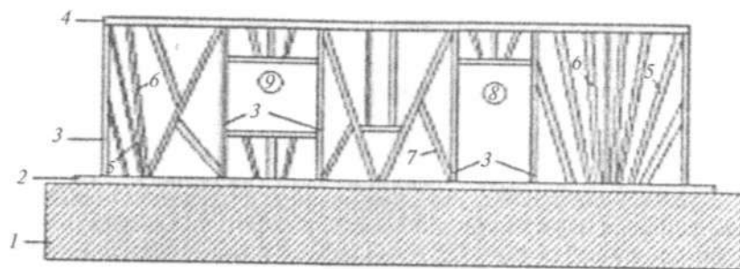
7.5- rasm. Eshik va deraza joyi qoldirilgan devor sinchlari: 1 – poydevor; 2 – tagsinch; 3 – ustunlar; 4 – sarrov; 5 – xovonlar; 6 – sinchlilar; 7 – qashak; 8 – eshik o'rni; 9 – deraza o'rni.
