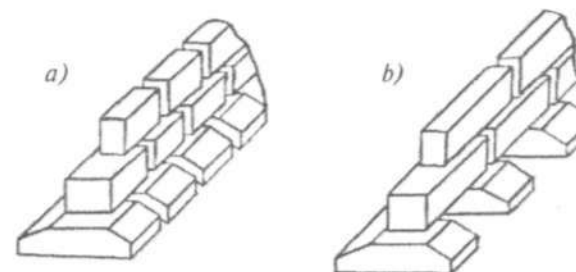
4.6- rasm. Yig'ma poydevorlar: a) zich joylashgan; b) siyrak joylashgan.
