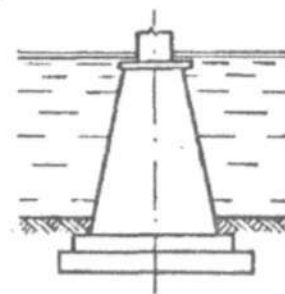
4.1- rasm. Ko'priklar ustuni poydevori.
