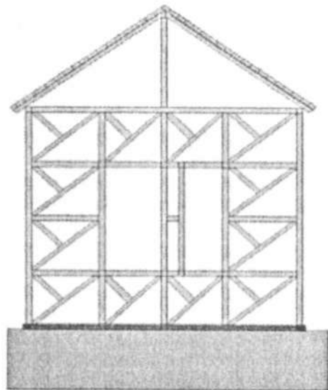
10.4- rasm. Sinchli konstruksiyaning umumiy ko'rinishi.
