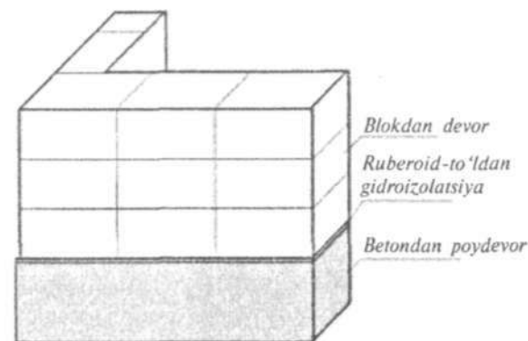
7.2- rasm. Blokli devor konstruksiyasi.
