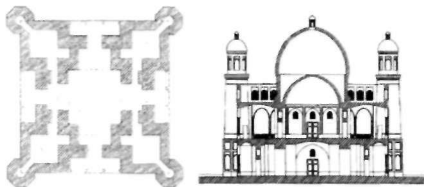
75-rasm. Bog'i Maydondagi «Chilstun» nomli ikki qavatli hashamatli saroy binosini qayta tiklash loyihasi (T.Mamatmusayev bo'yicha).
