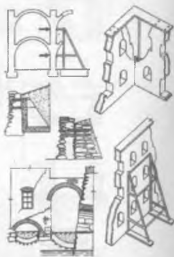
3.7.11-rasm. Nuragan konstruksiyalarni mustahkamlash.
