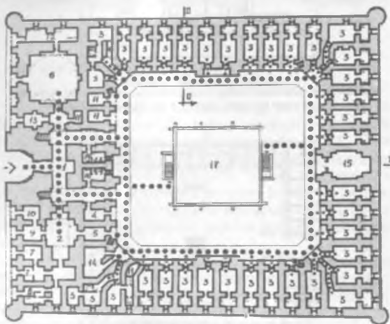
4.2.4-rasm. Mehmonxonaga moslashtirilgan Muhammad Aminxon madrasasi tarhi.
