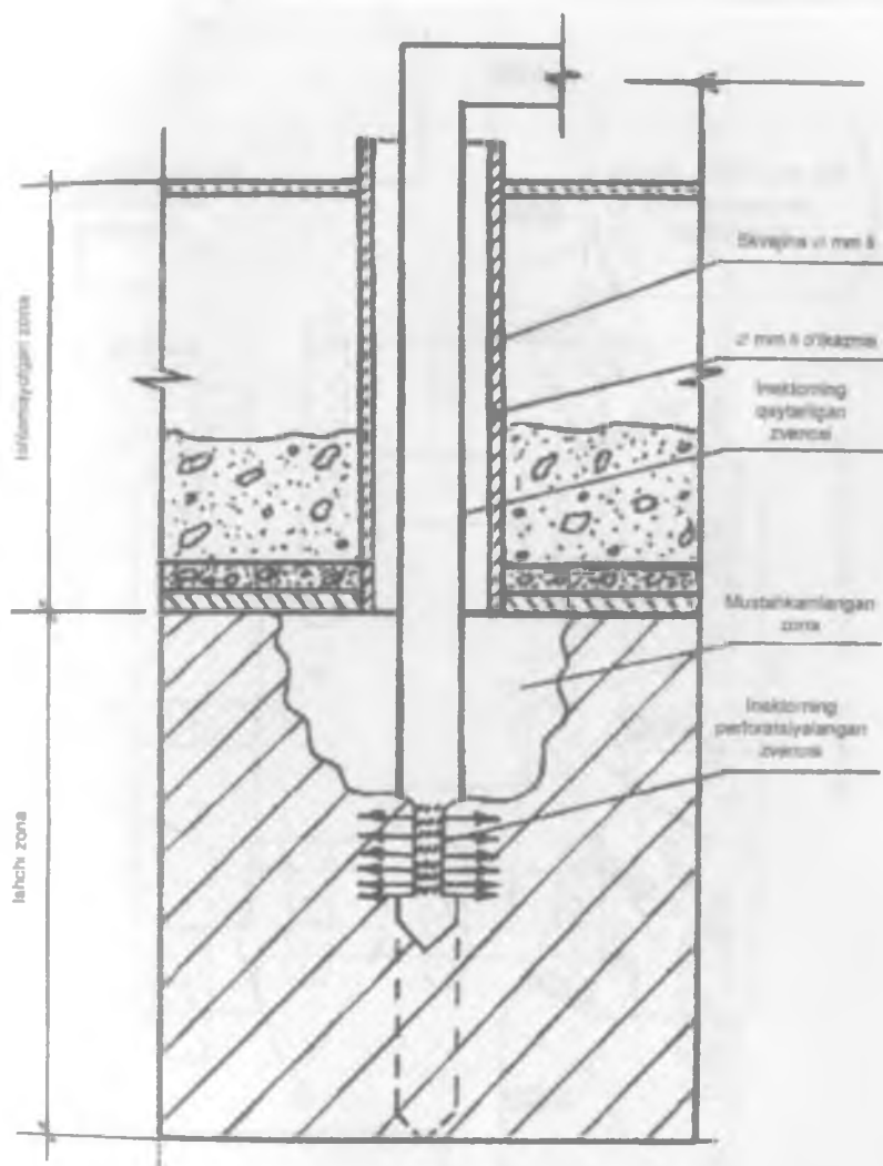
1-rasm. Skvajina konstruksiyasi.
