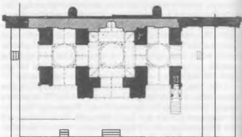
1.3.1-rasm. Buxoro namozgohi tarhi. XII asr (shtrixlangan qismi), XVI asr (qora rangdagi qismi). Yodgorlikning ko'p qatlamligiga yorqin misol.
