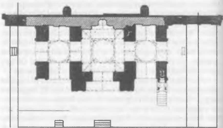
1.3.1-rasm. Buxoro namozgohi tarhi. XII asr (shtrixlangan qismi), XVI asr (qora rangdagi qismi). Yodgorlikning ko'p qatlamliligiga yorqin misol.
