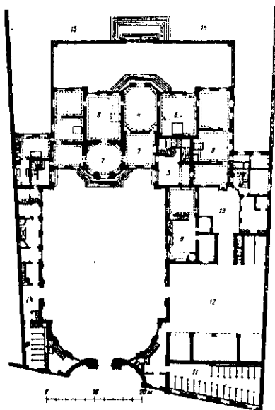
Parijdagi de Matinon mehmoxonasi. 1720 y. boshlangan. Arx. J. Kurtonn. Plan: 1-paradli hovli; 2-vestibul; 3- paradli zina; 4-7-paradli zallar; 8- yotoqxona; 9-oshxona; 10-11-otxona; 12-14-xizmat hovlilari; 15-bog'.
