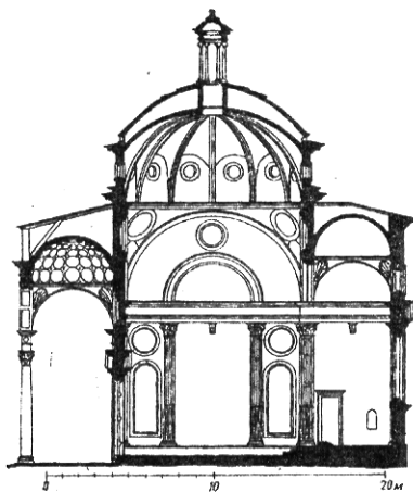
Florensiyadagi Kapella Passi. 1430-1443 y. Arx. Brunellesko. Qirqim.
