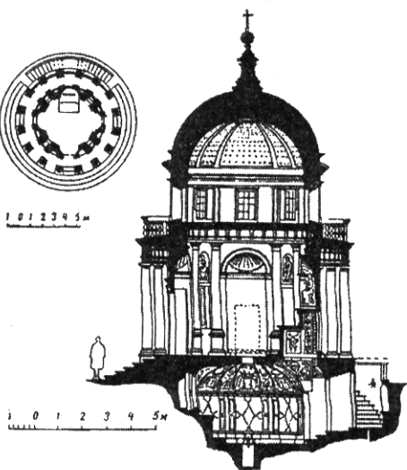
Rimdagi Tempetto, 1502 y. Arx. D.Bramante. Qirqim va plan.
