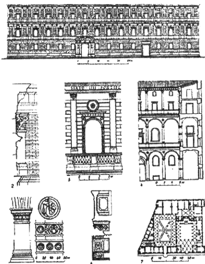
Rimdagi Palazzo Kanchelleriya, 1486 y. 1. Fasad. 2. Karniz profili va order fragmenti. 3. Ikkinchi qavat derezasi. 4. Hovli bo'yicha qirgim fragmenti. 5. Kapitel va ichki hovli arkad bazasi, dekorativ detallar. 6. Qirgimi va balkon sofiti. 7. Birinchi qavat plani.
