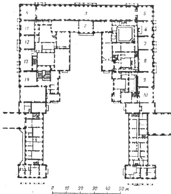
Versaldagi saroy XVII-XVIII asr Arx. L. Levo, J.A. Mansar va b. Ikkinchi qavatning markaziy qism plani. 1-Marmar hovli; 2-Lyudovik XIV ning xonasi; 3-Oynali galareya; 4- «Tinchlik» zali; 5- «Urush» zali; 6-«Apollon» zali; 7-«Merkuriy» zali; 8-«Mars» zali; 9-«Diana» zali; 10-«Venera» zali; 11-14-Qirol xonalari.
