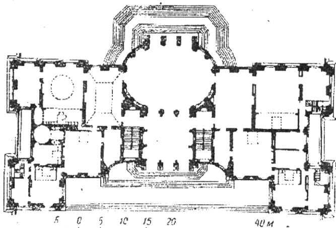
Vo le Vikont shahardan tashqaridagi saroy. Plan.
