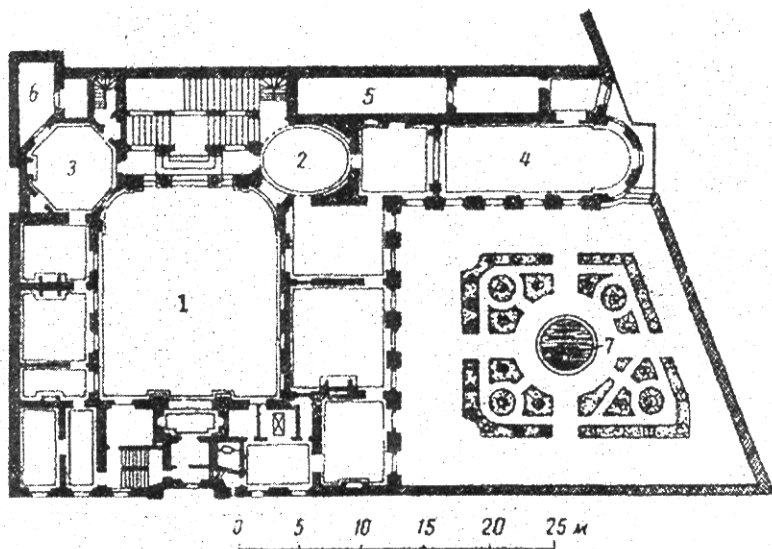
Parijdagi Lamber mehmonxonasi. Ikkinchi qavat plani: 1. paradli hovli; 2, 3 — vestibul; 4-kutubxona; 5, 6 — hovlilar; 7 — bog'
