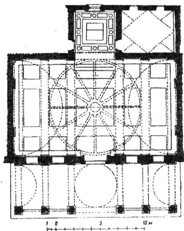
Florensiyadagi Kapella Passi. 1430-1443 y. Arx. Brunellesko. Plan
