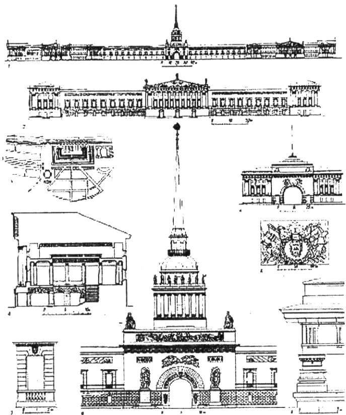
Peterburgdagi Admiralteystvo 1806-1823 y. Arx. A.D.3axarov. 1. Admiralteys maydoni tomonidagi fasad. 2. Qishki saroy tomonidagi fasad. 3. Bosh plan. 4. Heva tomonidagi pavilon fasadi. 5. Vestibyl qirqimi. 6. Olti ustunli portik Barelef. 7. Ikkinchi etaj d r zasi. 8. Asosiy minora fasadi. 9. Fasad orderi.
