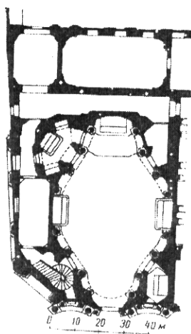
Rim, To'rt favvoradagi San-Karlo cherkovi, 1638 y. boshlangan, fasad 1667 y. arx. Borromini. Plan.
