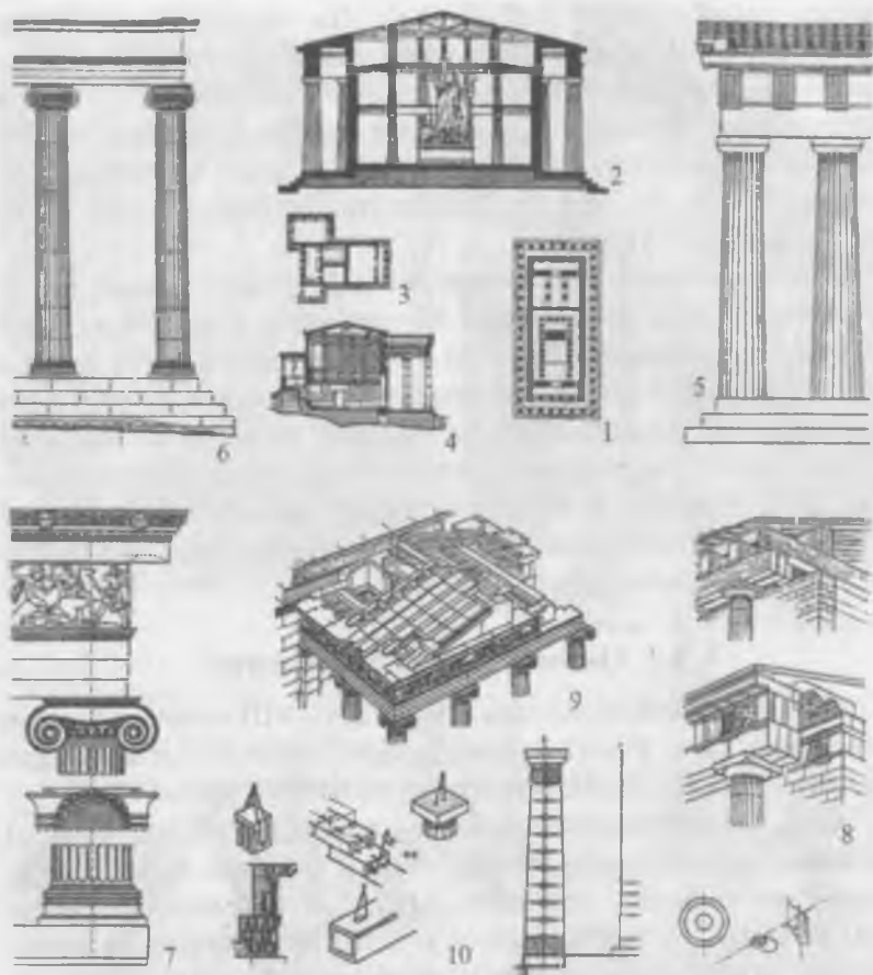
3.6 - rasm. Qadimgi Yunon arxitekturasida konstruksiya va orderlar (tartib). 1,2 – Parfenon (qizlar uchun xona) ning rejasi va ko'ndalang qirqimi (eramizdan oldingi 447–438 - yillar); 3, 4 – Erehteyonning rejasi va ko'ndalang qirqimi (eramizdan oldingi 421 – 406 - yillar); 5 – Parfenonning dorik orderi; 6 – Erehteyonning ionik orderi; 7 – Niki Apteros ibodatxonasining ionik orderi detallari (eramizdan oldingi 449 – 421- yillar); 8 – dorik order va uning yog'och prototipi; 9 – Erehteyonning tom konstruksiyasi; 10 – devor, ustunlarini terish va bloklarini bir - biriga birlashtirish
