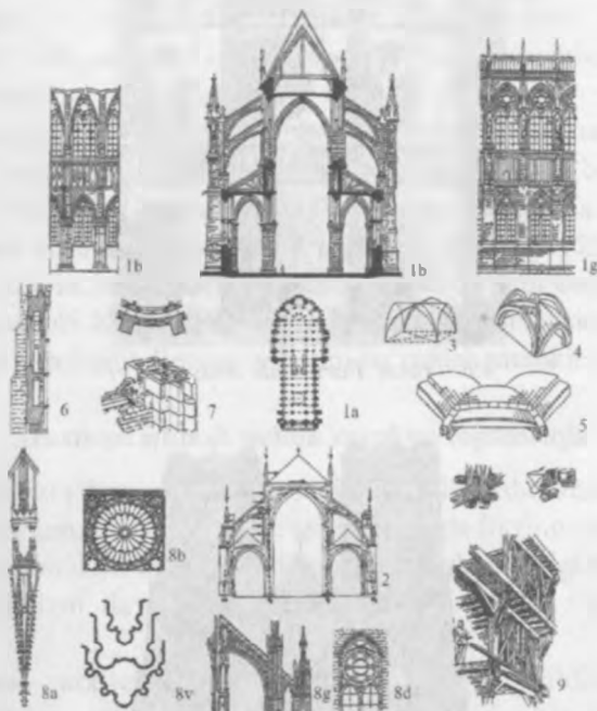
4.5-rasm. Gotika arxitekturasida konstruksiyalar va shakllarining plastik ishlanishi. 1 – Reymsdagi sobor (XIII asr): a – reja; b – ko'ndalang qirqim; v – asosiy nefning bo'linishi va dekori; g – yon tomon fasadining fragmenti; 2 – tirkagich va shamol bosimining tarqalish sxemasi; 3 – strelka shaklidagi xojsimon gumbaz; 4 – gumbazning nervyuralari; 5 – yog'och konstruksiyalardan gumbazning ko'tarilishi; 6 – ibodatxonaning tashqi devori bo'yicha qirqimi; 7 – g'isht terimi ichining to'ldirilishi; 8 – gotika detallari: a – fial; b – deraza - atirgul; v – nervyur profili, g – ikki proletli arkbutan; d – yon tomon fasadining derazasi; 9 – o'rta asr uyining yog'och faxverk konstruksiyasi
