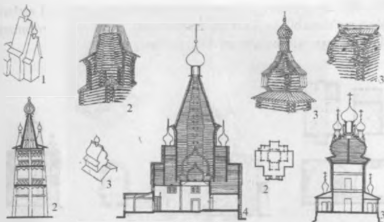
5.14-rasm Qadimgi rus arxitekturasida yog'ochdan tayyorlangan diniy inshootlarning konstruktiv shakllari. 1-ikki qiyali oddiy cherkov binosi; 2-cherkov va qo'ng'iroq inshootlari; 3-yopma konstruksiyasi bochka va kubsimon bo'lgan cherkov inshootlari; 4-cherkov binosi qirgimi
