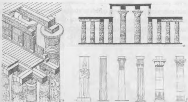
3.1 - rasm Qadimgi Misrda ustun - to'sin konstruktiv tizimi.
