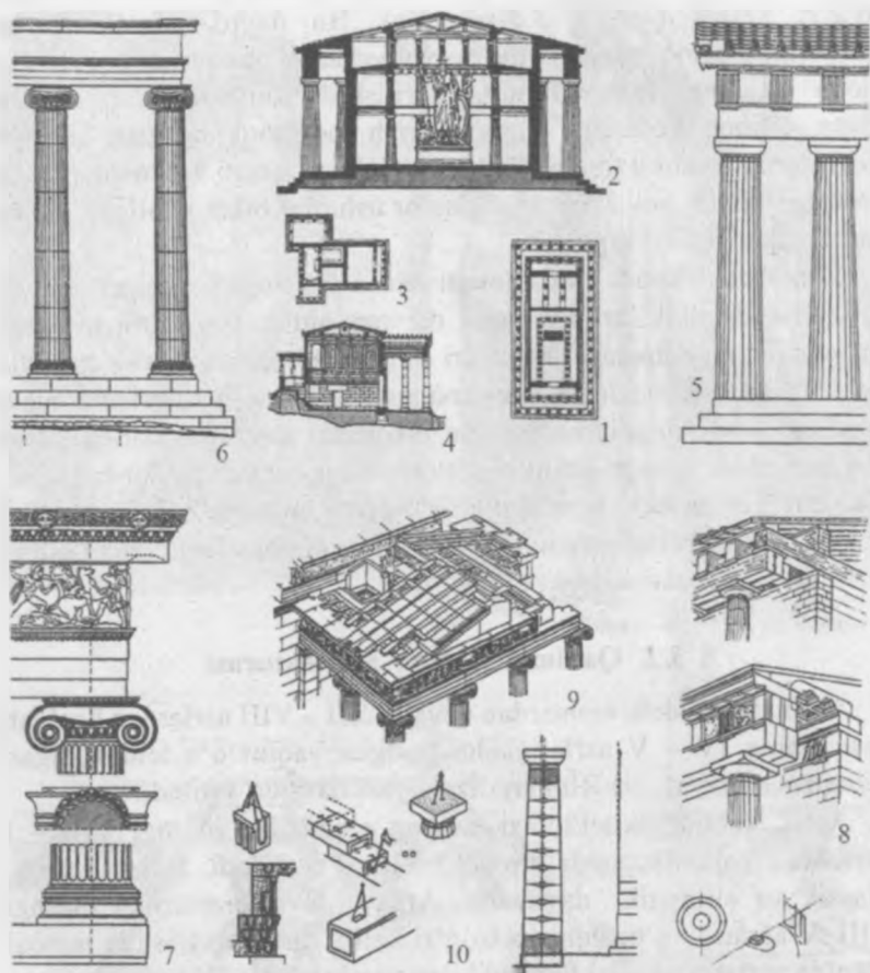
3.6 - rasm. Qadimgi Yunon arxitekturasida konstruksiya va orderlar (tartib). 1,2- Parfenon (qizlar uchun xona) ning rejasi va ko'ndalang qirqimi (eramizdan oldingi 447-438 - yillar); 3, 4 - Erehteyonning rejasi va ko'ndalang qirqimi (eramizdan oldingi 421 - 406 - yillar); 5 - Parfenonning dorik orderi; 6 - Erehteyonning ionik orderi; 7 - Niki Apteros ibodatxonasining ionik orderi detallari (eramizdan oldingi 449 - 421- yillar); 8 - dorik order va uning yog'och prototipi; 9 - Erehteyonning tom konstruksiyasi; 10 - devor, ustunlarini terish va bloklarini bir - biriga biriktirish
