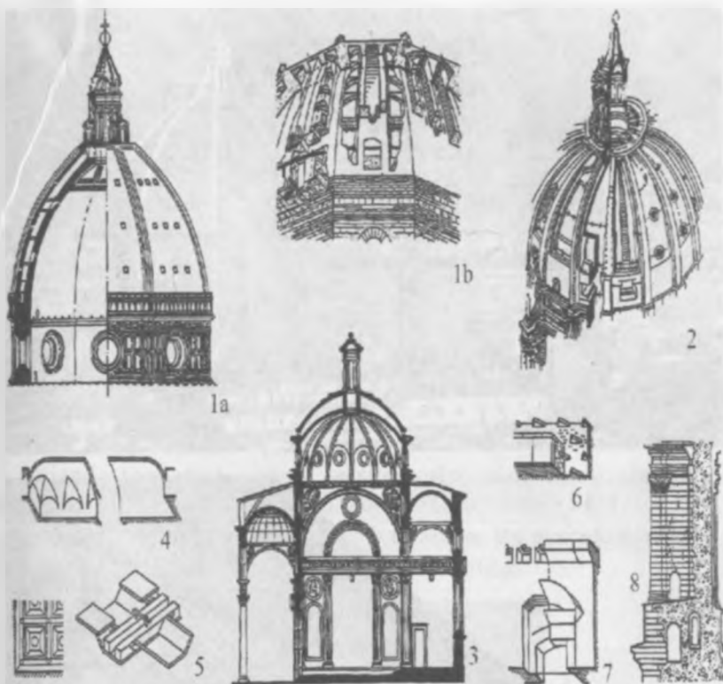
5.1-rasm. Uygʻonish davri arxitekturasining konstruksiyalari va qurilish usullari. 1 –Florensiyadagi sobor gumbazl (Fore sobori, 1420–1471 -yillar), a – qirim va fasad; b – gumbaz konstruksiyasi; 2 – Rimdagi avliyo Pyotr soborining gumbazi (XVI asr ikkinchi yarmi); 3 – Florensiyadagi Paststi kapellusi, qirgʻini; 4 – gumbazlar; 5 – osma shift detallari; 6, 7 – devorlarni pardozi usullari; 8 – devor boʻshliqlarini beton bilan toʻldirish (avliyo Pyotr sobori)
