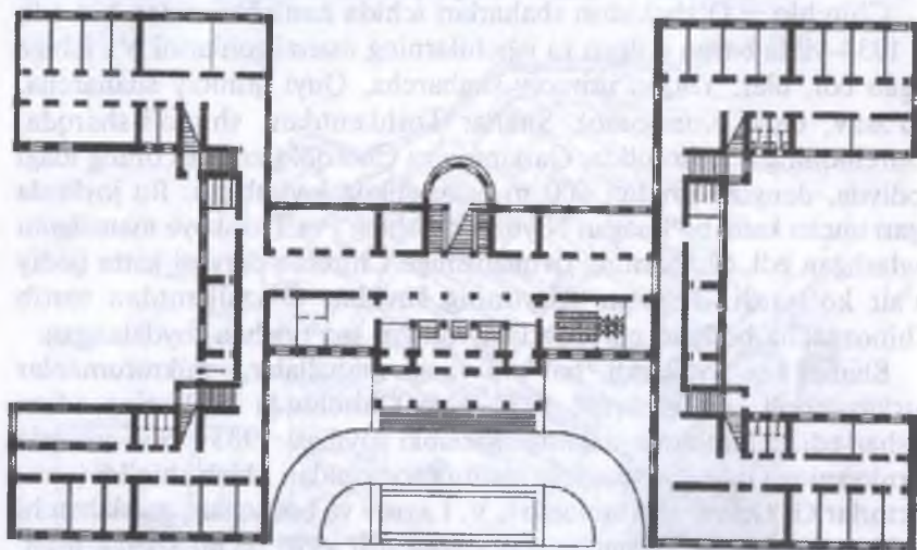
Toshkent. To'qimachilik kombinatiga qarashli poliklinika, 1936-y., arxitektor K. Babiyeveskiy. Umumiy ko'rinishi va birinchi qavat tarhi.
