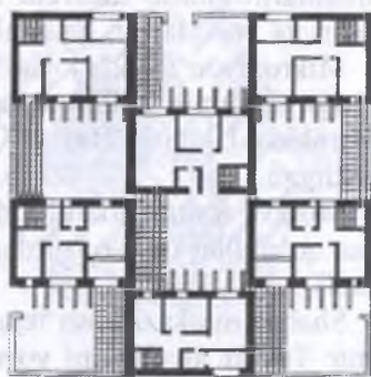
Markaz-5 mikrorayonda ikki qavatli blokli turar-joylar, 1967-y. Arxitektorlar B. Rubanenko, M. Vladimirova. Umumiy ko'rinishi va tarhi.
