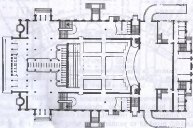
Temiryo'Ichilar Madaniyat saroyi, 1939-y, arxitektor A.Pavlov. Umumiy ko'rinishi va birinchi qavat tarxi.
