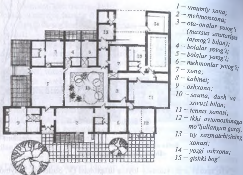
Yuqori qulaylik toifadagi turar-joylar loyihasi (katta oilalar uchun) «Doktor Mahkamov» firmasi.
