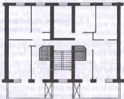
Turar-joylar uchun 1-310-I seriyalik tipik loyiha, 1964-y.
