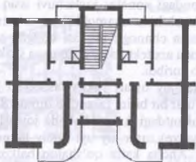
Toshkent. Mustaqillik (sobiq Pushkin) shoh ko'chasidagi turar-joy. 1924-y, arxitektorlar K. Babiyeviskiy, A. Petelin.
