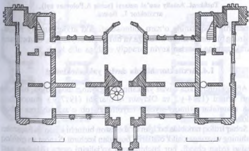
Toshkent. O'zbekiston Tashqi ishlar vazirligi Qabulxonasi (buyuk knyaz Nikolay Konstantinovichning sobiq saroyi), arxitektor L. Benua.
