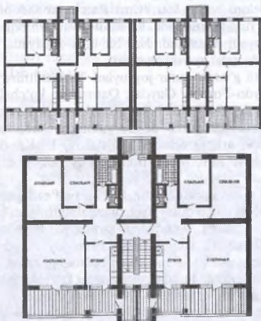
Toshkent. Qunayev ko'chasidagi yanada yaxshilangan rejali tutar-joy majmui. «Toshgiprogor» instituti.
