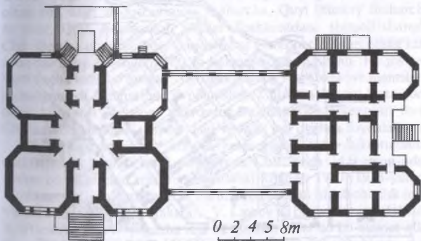
Qo'qon. Rus-Osiyo banki, 1910-y arxitektori I. Markevich. Umumiy ko'rinishi va tarhi (M. Yusupova kitobidan).
