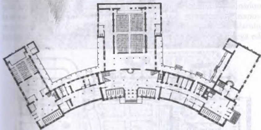
Toshkent. To'qimachilik kombinatining madaniyat saroyi, 1940-y., arxitektorlar A. Karnauxov, A. Galkin. Umumiy ko'rinishi va birinchi qavat tarhi.
