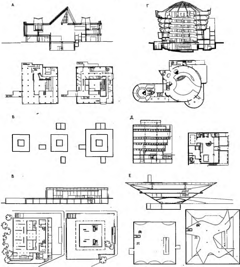
Рис. 16.3. Композиционные приемы решения музейных зданий
