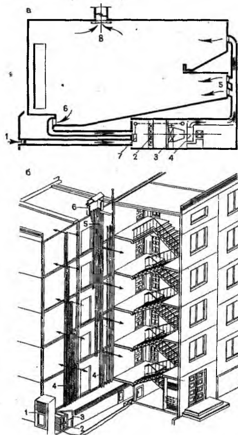
Рис. 6.2. Система воздушного отопления
