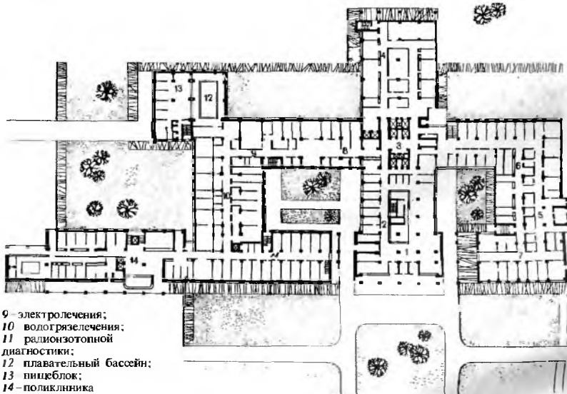
Рис. 30.2. Многопрофильная городская больница на 600 коек. Типовой проект. Архитекторы К. Матюхи и Е. Ефремова. Широкий палатный корпус решен по двухкоридорной системе. На этаже 60 коек (две секции по 30 коек). Лечебно-диагностический блок расположен в стиловатой части. Общий вид, генеральный план, план 1-го этажа
