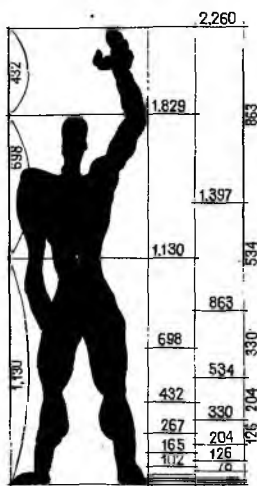
Рис. 1.15. Модульор Ле Корбюзье
