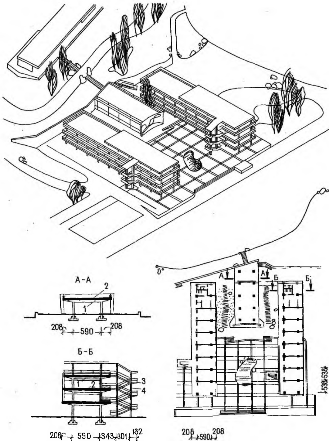
Рис. 3.3. Пионерский лагерь «Морской». Площадки Дружбы, Спальные корпуса и Лепинская комната между ними выполнены из четырех унифицированных
