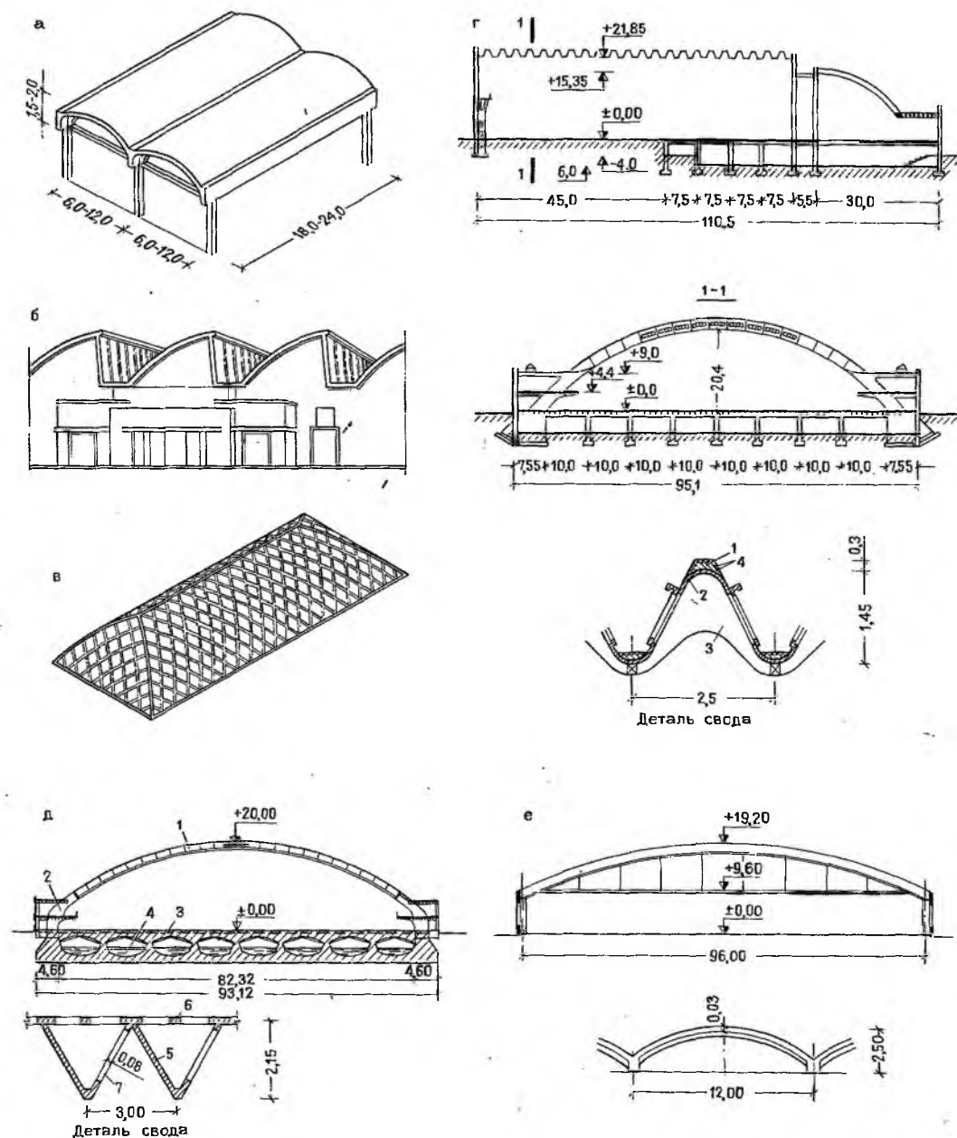
Рис. 4.9. Своды-оболочки а-в- цилиндрические оболочки. Волнистые своды: г- свод главного павильона выставочного центра
