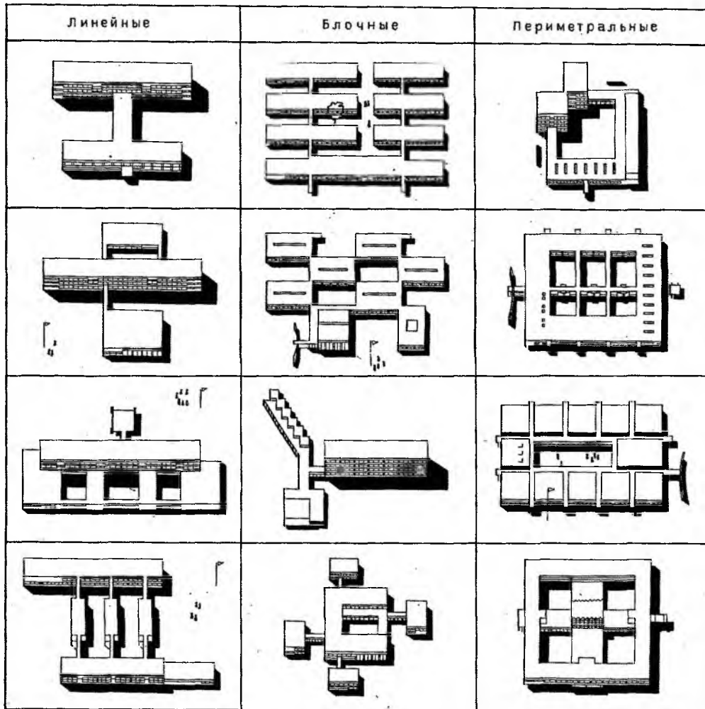
Рис. 9.6. Примеры композиционных схем школьных зданий
