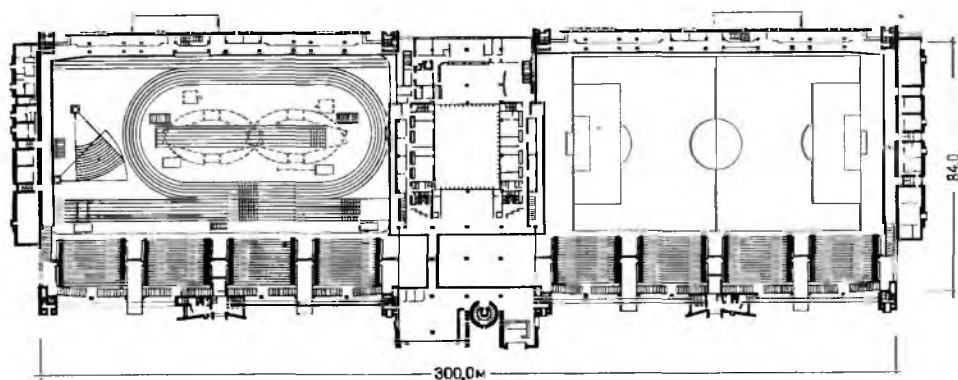
Рис. 20.3. Легкоатлетический и футбольный манеж ЦСКА Архит. Ю. Кривуценко
