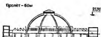
Пролет - 60м железобетонный многоугольный купол
