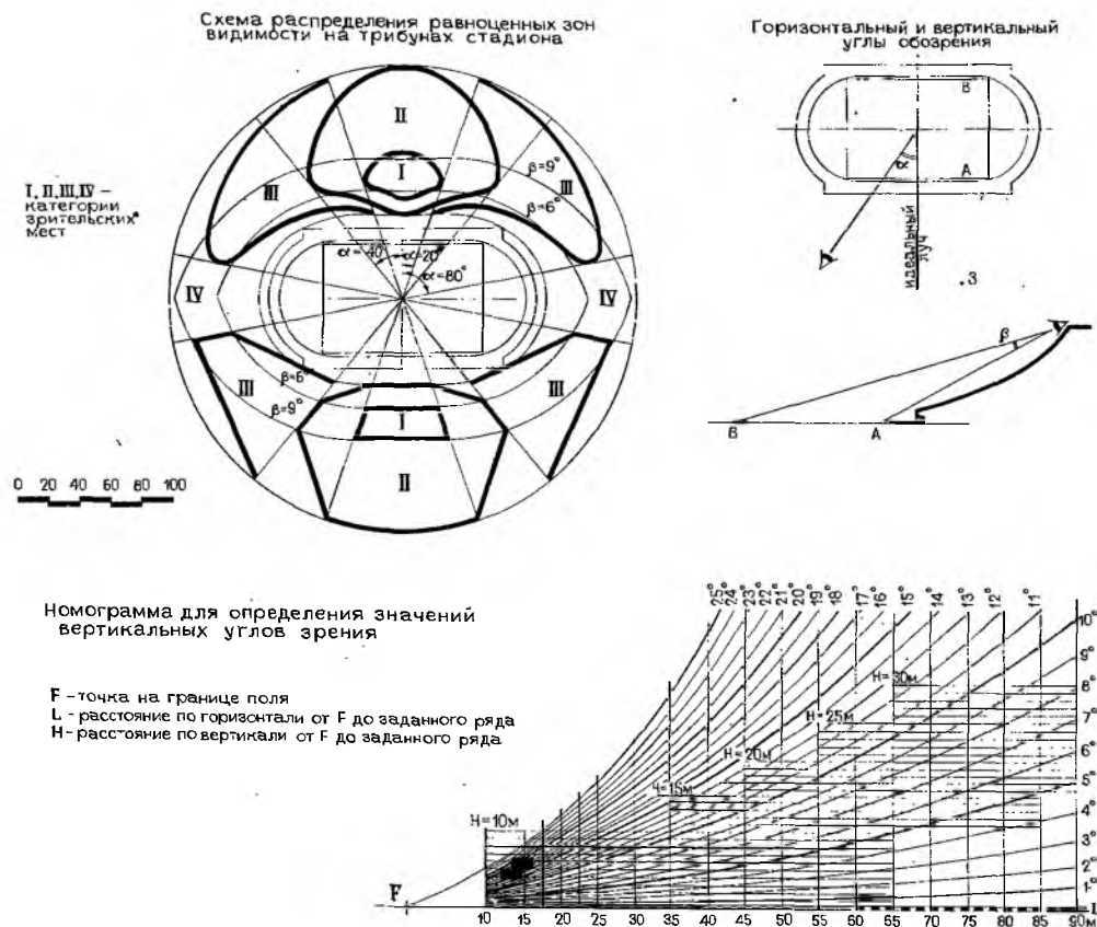
Рис. 19.4. Условия видимости арены
