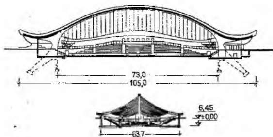
Нью-Хавен, США. Крытая спортивная арена с трибунами на 2900 мест
