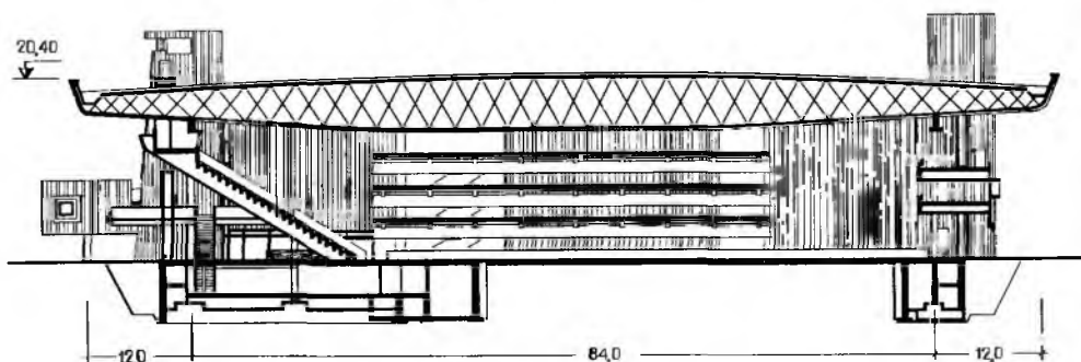
Рис. 20.4. Легкоатлетический и футбольный манеж ЦСКА План. Разрез
