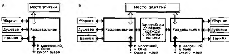
Рис. 21.1. Структурные схемы связи раздевальных с другими помещениями
