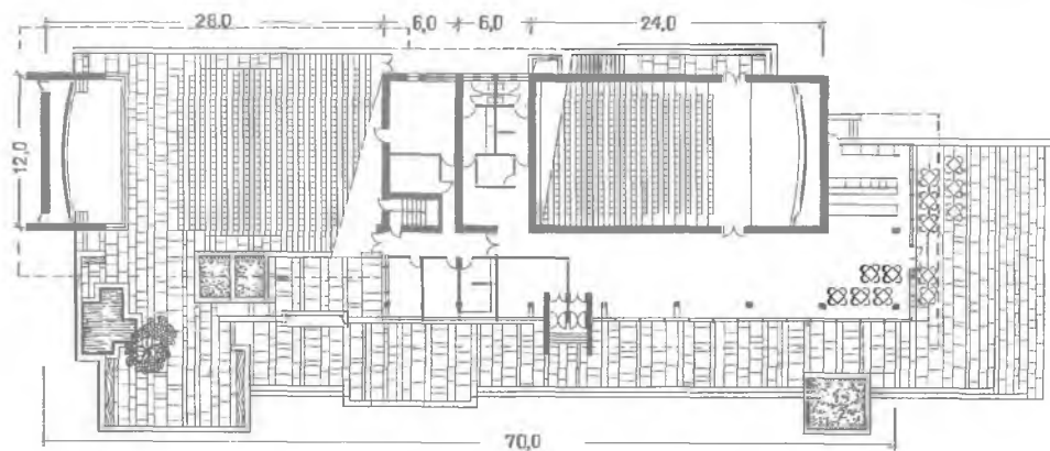
Рис. 12.4. Кинотеатр с залом на 300 мест с крытой киноплощадкой на 500 мест, план. Архитекторы М. Бубнов, В. Назарев, И. Семейкин, Э. Тер-Степанов
