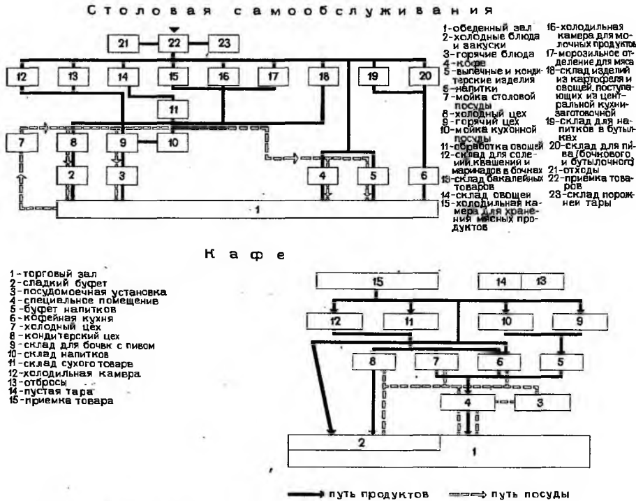
Схема пищеблока по бесцеховой системе
