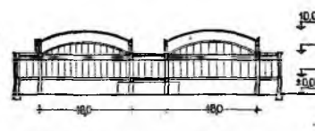
Гладкий железобетонный купол-оболочка
