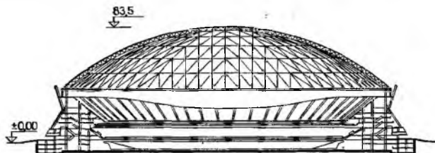
Новый Орлеан, США. Крытый стадион с трибунами на 72000 человек
