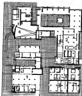
Торговый центр на 10-12 тыс. человек в квартале 24 по Гражданскому проспекту, г. Ленинград
