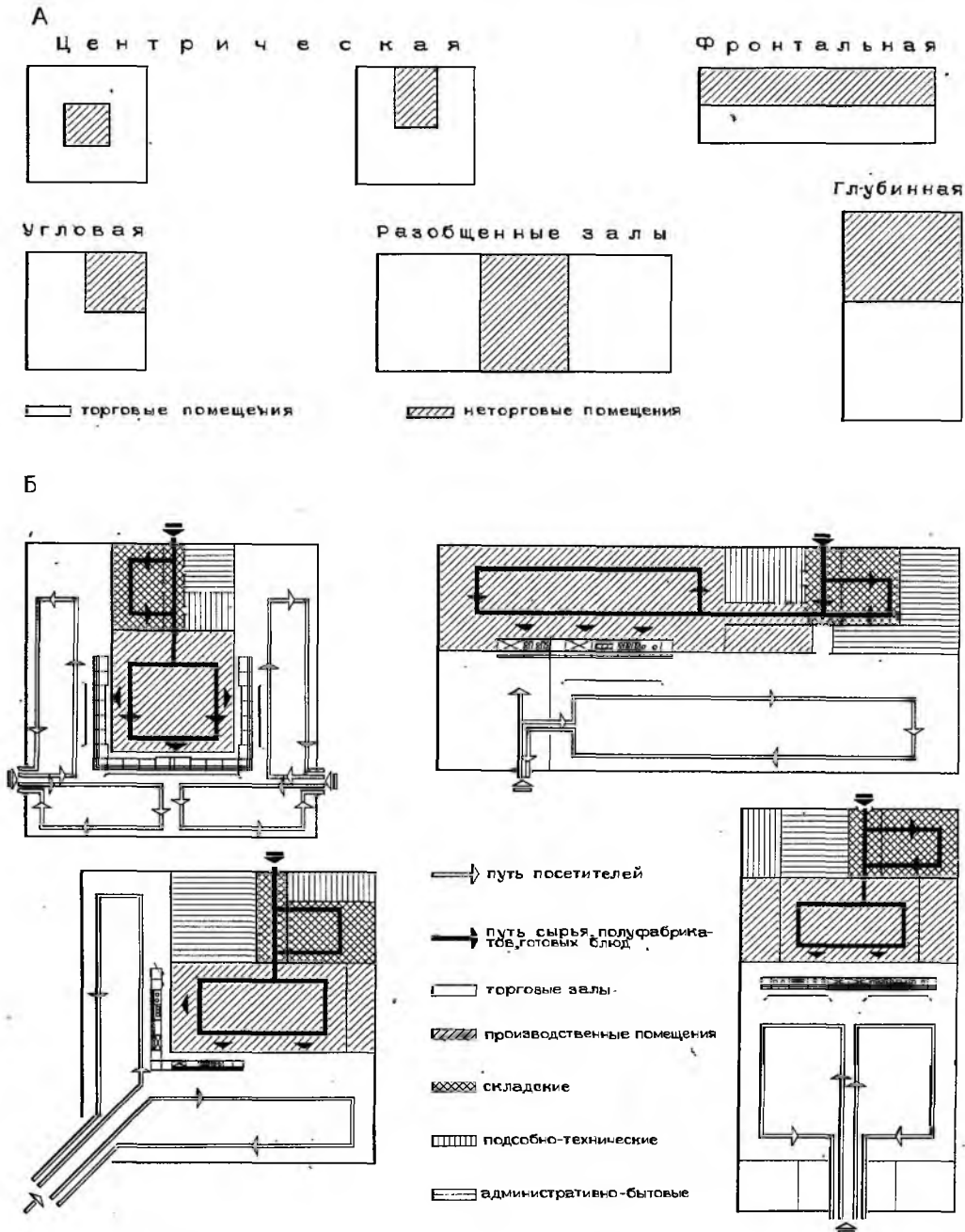
Рис. 23.13. Композиционные (А) и технологические (Б) схемы предприятий общественного питания
