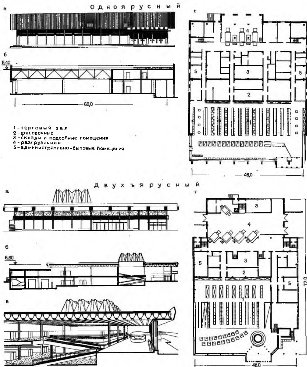
Рис. 23.1. Универсамы а-фасады; б-разрезы; в-перспектива интерьера; г-планы на уровне земли
