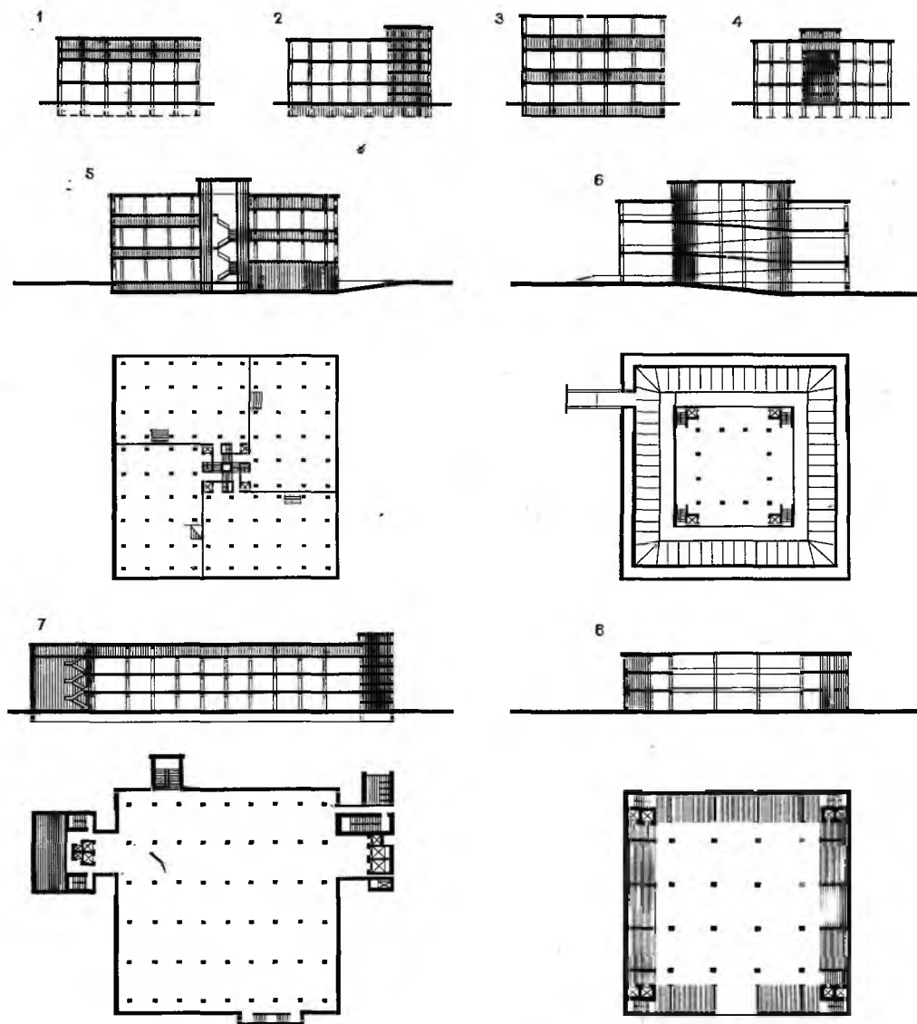
Рис. 23.3. Схемы объемно-планировочных решений универмагов 1—неторговые помещения располагаются над торговыми и в подвале; 2—неторговые и торговые помещения располагаются
