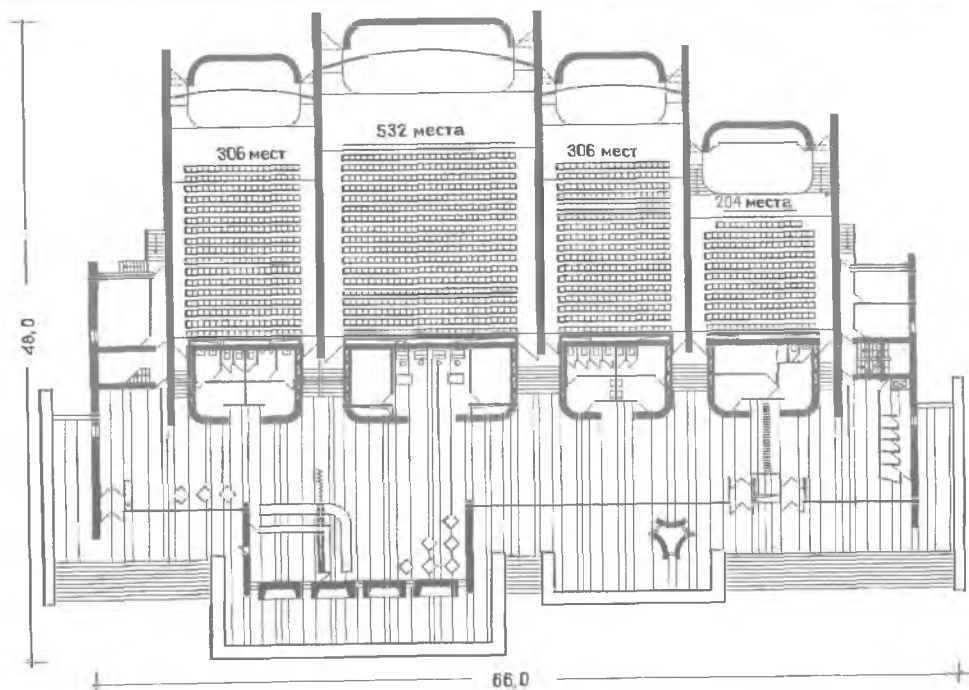
Рис. 12.2. Многозальный кинотеатр на 500; 300; 300 и 200 мест. Типовой проект. Архитекторы М. Бубнов,
