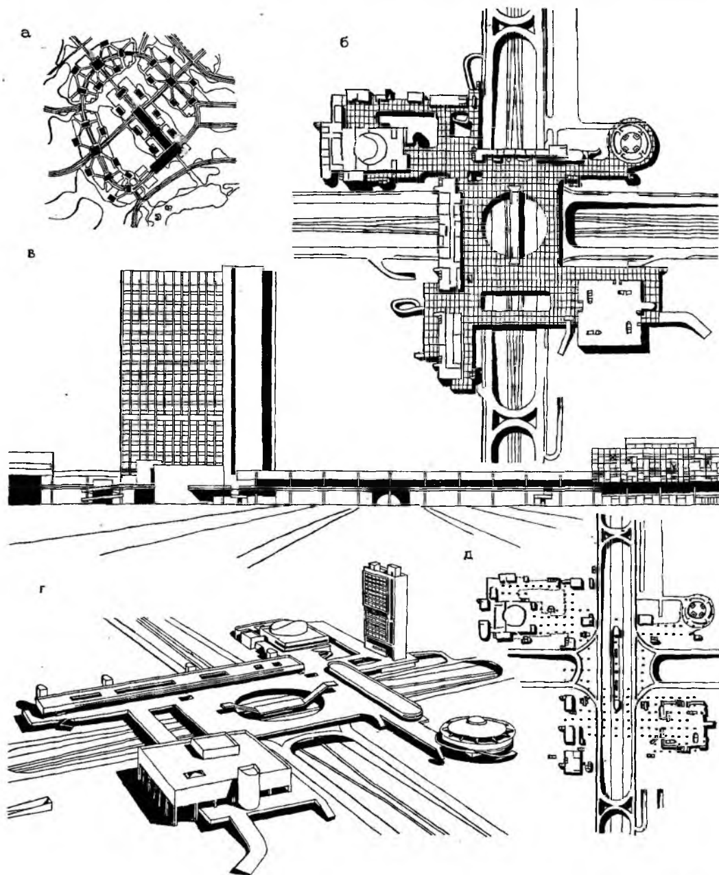
Рис. 24.5. Общественно-торговый центр в Челябинске (проект). Архитекторы А. Урбах, И. Зеедин. Общий вид
