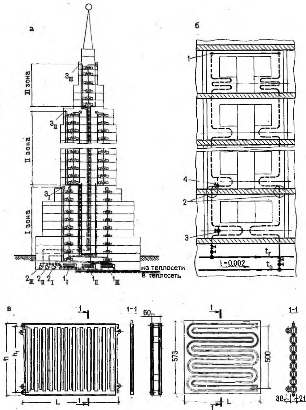
Рис. 6.1. Система водяного отопления
