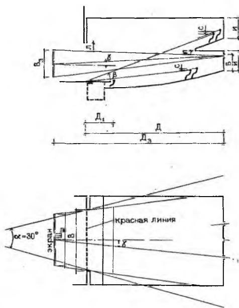
Рис. 14.3. Параметры зрительного зала
