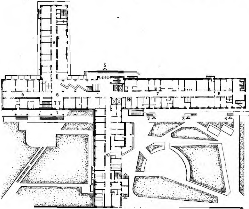
Рис. 30.4. Многопрофильная сельская районная больница на 300 коек. Архитекторы Э. Литвак, И. Каменская. Типовой проект. Т-образное решение палатных секций (60 коек на этаже) с торцовым примыканием поэтажно расположенного лечебно-диагностического блока
