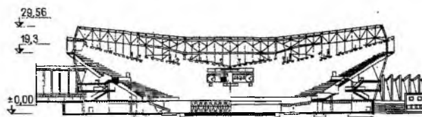
Вена. Большой спортивный зал с постоянными местами на 12 000 человек
