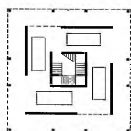
Стоянки под жилыми номерами (одно-, двусторонние и центрические)
