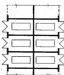
Стоянки под жилыми номерами (одно-, двусторонние и центрические)
