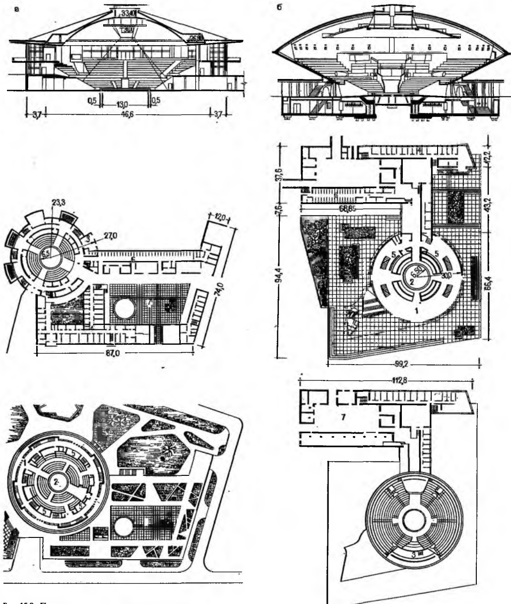
Рис. 15.2. Примеры архитектурных решений зданий цирков
