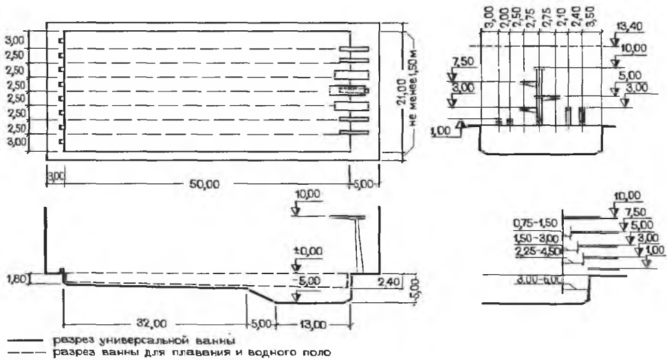
Рис. 20.21. План и продольный профиль универсальной ванны и прыжкового устройства
