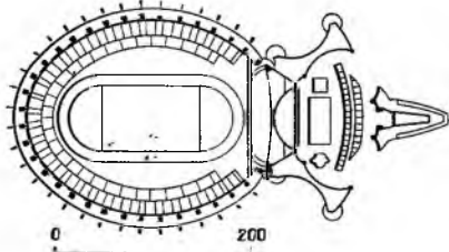
Рис. 19.15. Объемно-планировочные композиции трибун
