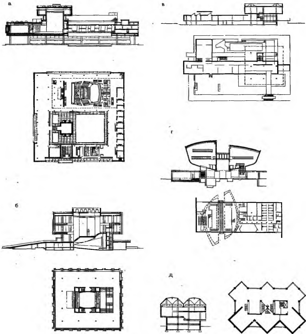
Рис. 16.4. Композиционные приемы решения музейных зданий
