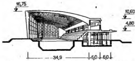
Минск. Комплекс открытых и закрытых плавательных бассейнов. В закрытом бассейне ванны 21 \times 50 , 20 \times 20 и 10 \times 20 м
