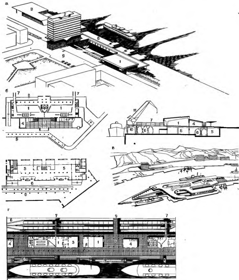
Рис. 29.5. Речные и морские вокзалы
