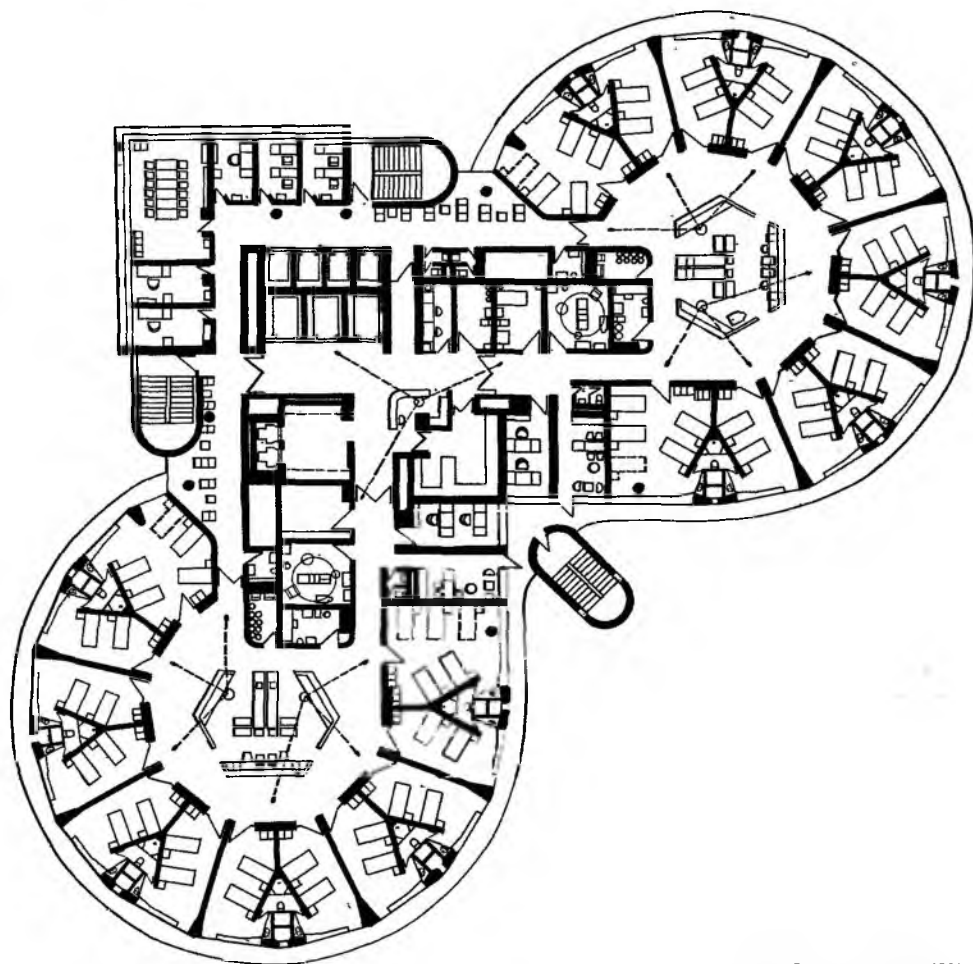
Рис. 30.5. Больница на 1800 коек в Мюнстере (ФРГ). Архитектор Шахнер. Пример компактного решения стационара с круглыми в плане палатными секциями. План типового этажа
