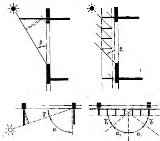
Рис. 5.10. Расчетные схемы защитных углов \beta и \gamma для выбора солнцезащитных устройств
