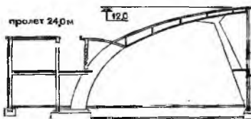
несущая конструкция - железобетонный консольный свод
