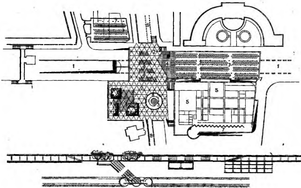
Рис. 27.2. Тоннельный переход развитого типа и вход в метро в составе многофункционального общественно-транспортного комплекса. Проектное
