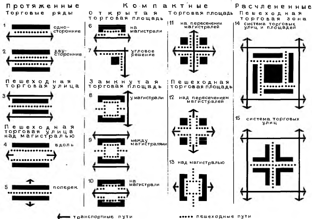
Рис. 24.7. Основные схемы планировочной организации торговых центров
