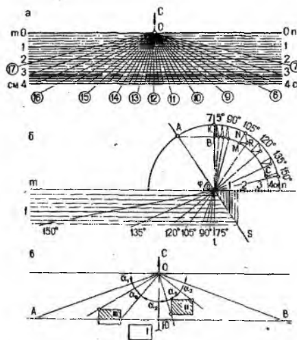
Рис. 5.9. График для определения условий инсоляции зданий и территорий и методы его построения и использования при проектировании
