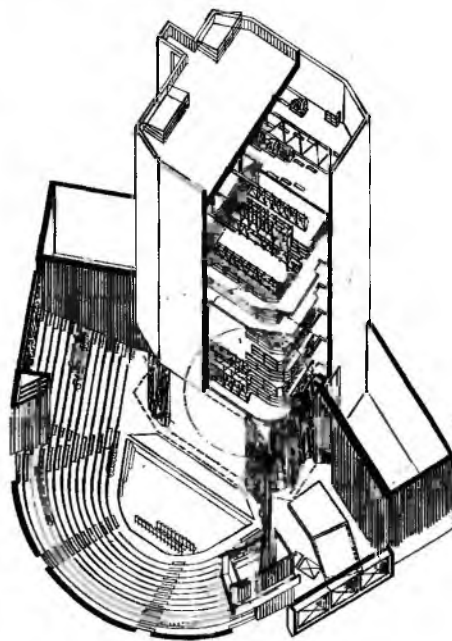
Рис. 13.7. Театр в Туле. Архитекторы С. Галаджева, В. Красильников, А. Попов, С. Шульхтер. АксонOMETрический разрез, план
