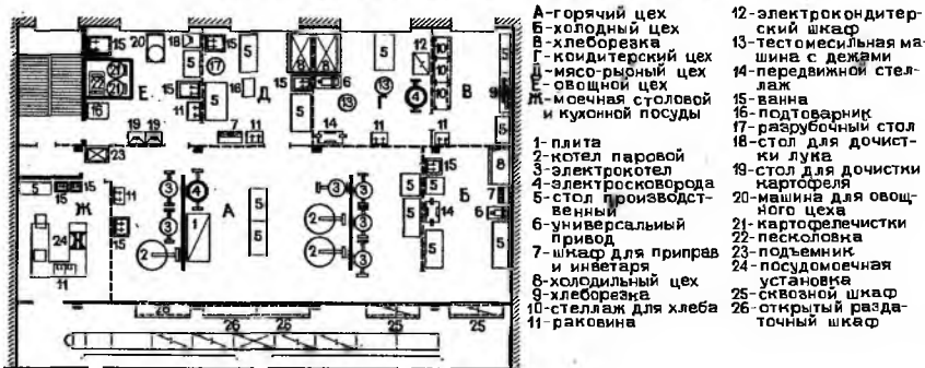
Схема пищеблока по бесцеховой системе
