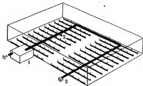
Рис. 6.7. Схемы организации пылеудаления из зданий 1 – камера; 2 – канал; 3 – пылесосная установка
