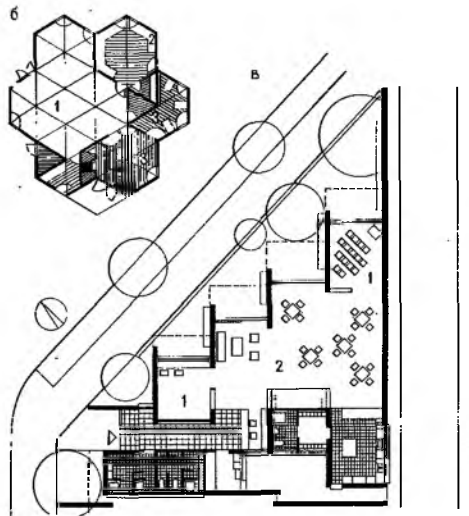
Рис. 14.2. Клубы для различных возрастных групп а - Дом молодежи в Благоевграде, Болгария. Архитекторы Я. Петров, Ив. Батраков; б - клуб молодежи в Валь-д'Оаз,
