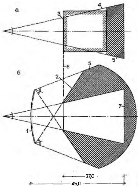
Рис. 14.4. Зоны размещения дополнительных зрительских мест
