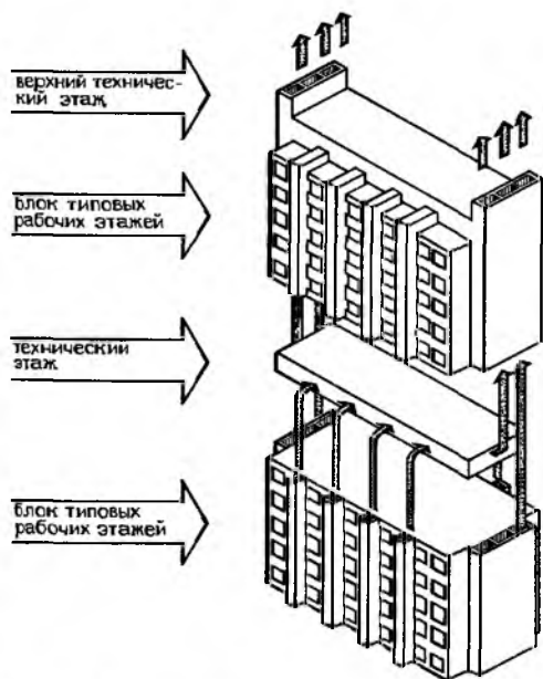
Рис. 11.10. Принципиальная схема инженерно-технологического обеспечения лабораторного корпуса
