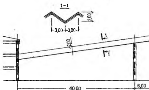
Рис. 4.7. Покрытие здания тренировочного катка Центрального стадиона имени В. И. Ленина в Москве
