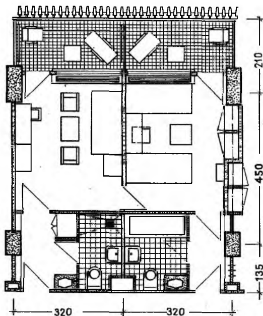
Рис. 31.12. Варианты планировки номеров в курортной гостинице «Ялта» в Крыму
