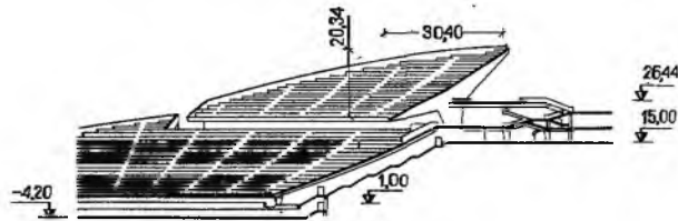
Стадион "Раздан". Ереван. 80 000 мест
