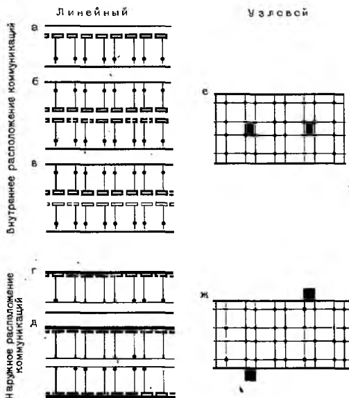
Рис. 11.7. Основные типы лабораторных зданий.
