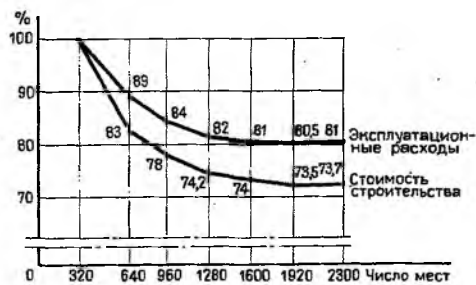
Рис. 7.1. Зависимость стоимости строительства (из расчета на одного ученика) от вместимости школьных зданий и эксплуатационных расходов
