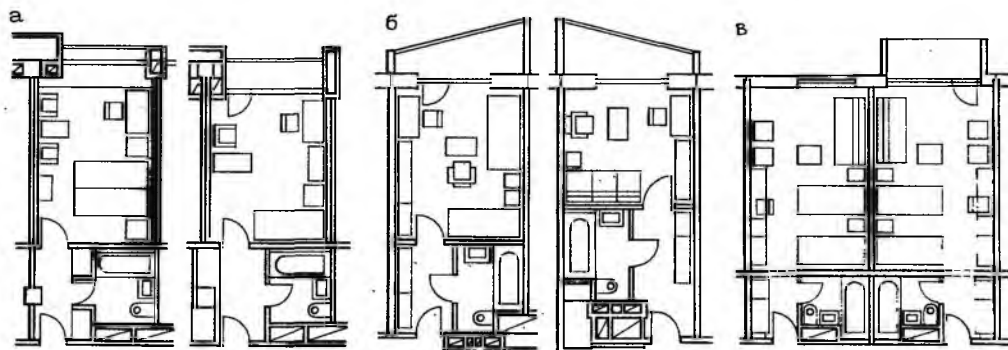
Рис. 26.6. Варианты планировки номеров
