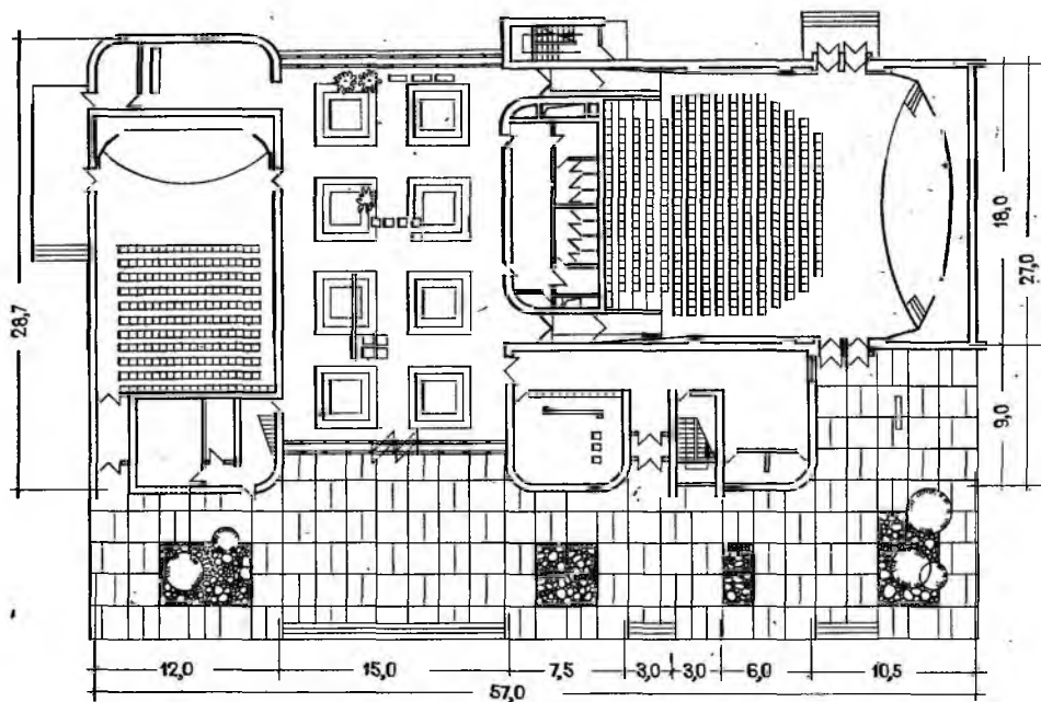
Рис. 12.7. Детский кинотеатр с залами на 400 и 200 мест. План. Архитекторы Г. Павлова, Ю. Федотов
