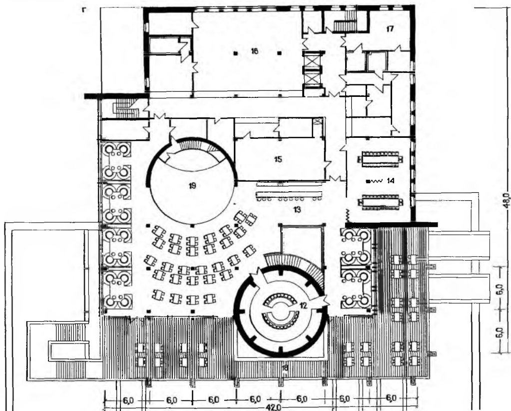
Рис. 23.16. Ресторан «Дом Башкирской кухни» в Уфе. Архитекторы З. Арзамасова, Т. Петрова. Общий вид (с.м. с. 385) а-фасад; б-разрез; в-план 1-го этажа; 2-план 2-го
