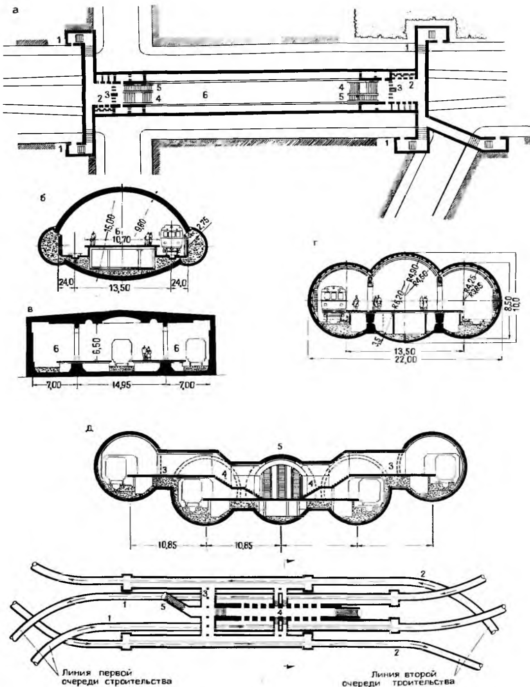
Рис. 27.4 Планировочные схемы и габариты станций и пересадочных узлов метрополитена
