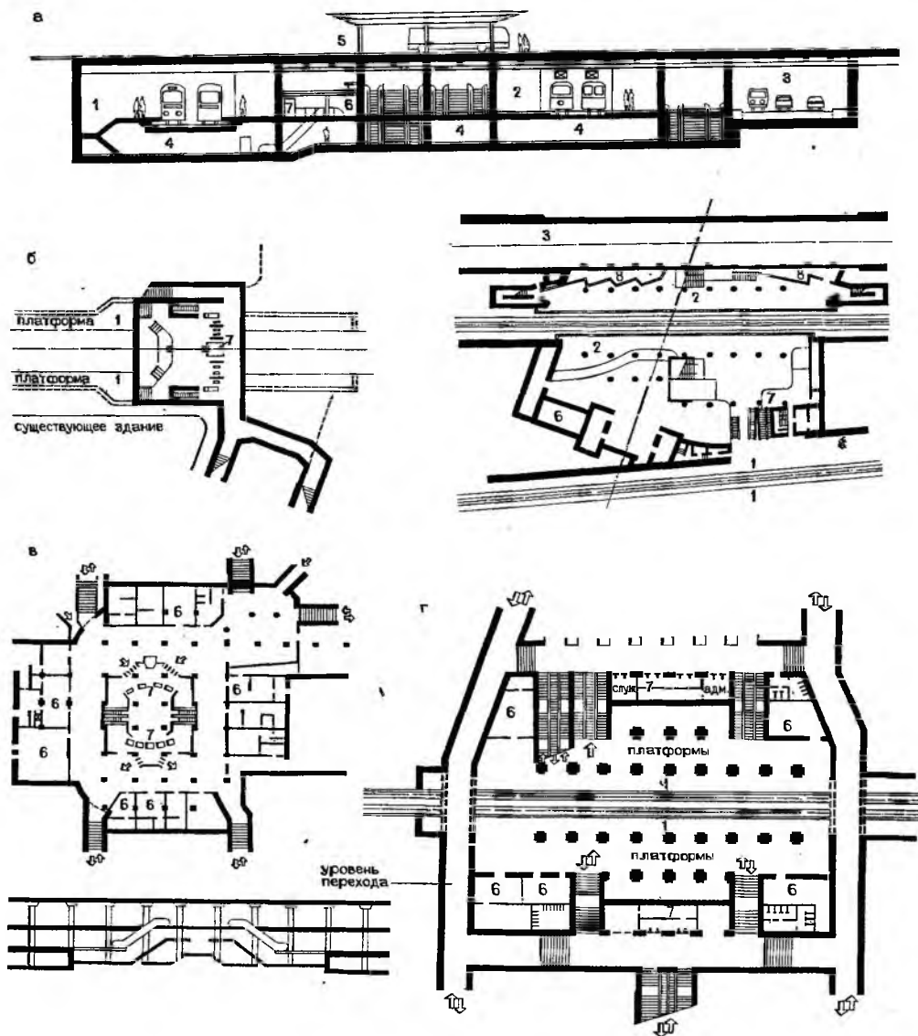
Рис. 27.5. Подземные вестибюли метрополитенов (зарубежная практика) а – пересадочная объединенная станция «трамвай-автobус-метрополитен» на площади Зюдтиролерплац в Вене (Австрия). Разрез и план: 1 – станция метро, 2 – подземная станция трамвая, 3 – автотранспортный тоннель, 4 – подземные переходы, 5 – остановки уличного
