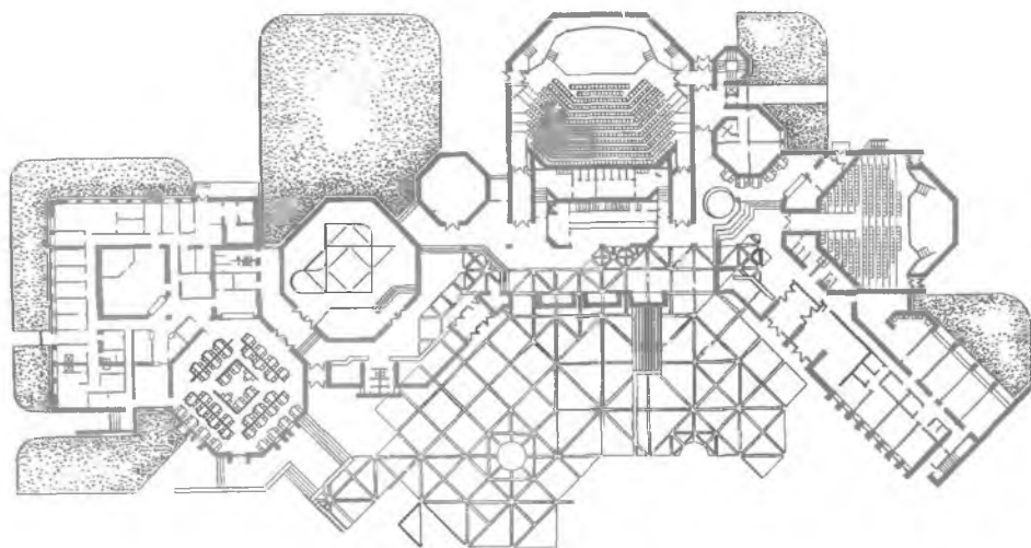
Рис. 12.3. Кинотеатр с залами на 500 и 200 мест, кафе на 150 мест и танцевально-выставочным
