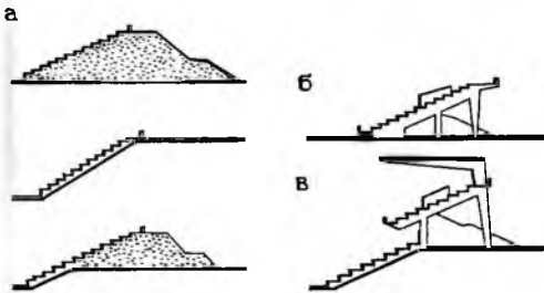
Рис. 19.9. Типы конструкций трибун а — на грунтовом основании: насыпные, на естественном
