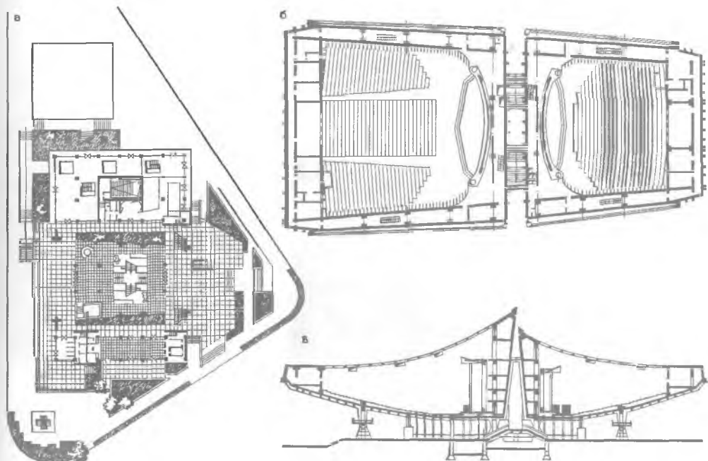
Рис. 12.10. Кинотеатр «Россия» в Ереване. Генплан, план, разрез
