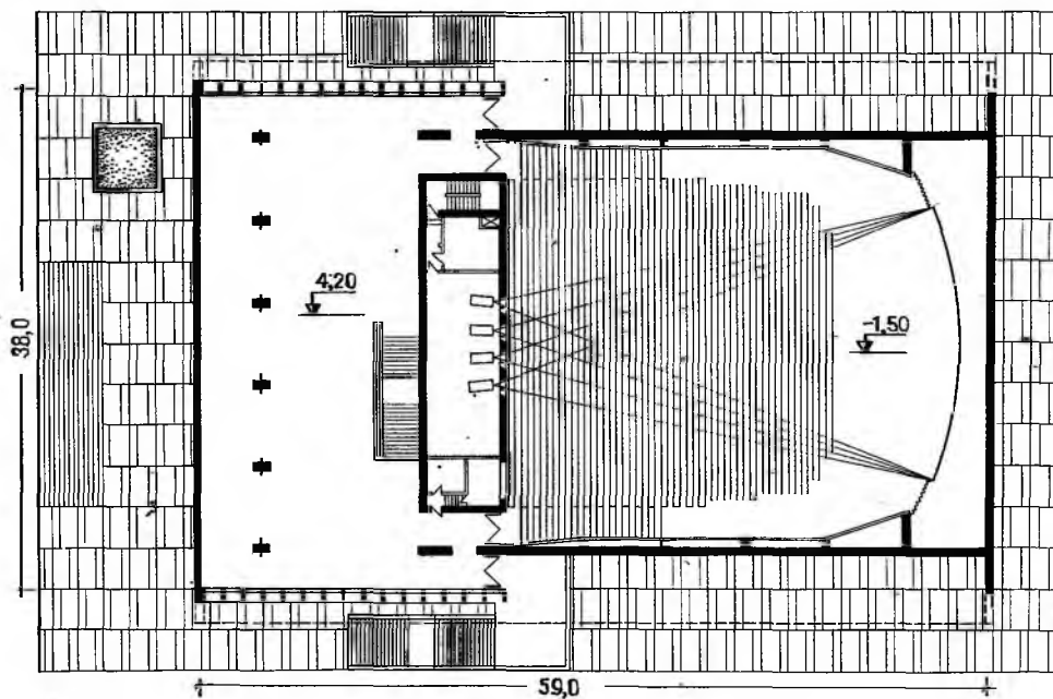
Рис. 12.6. Широкоформатный кинотеатр «Сатурн» в г. Тольятти. План 2-го этажа
