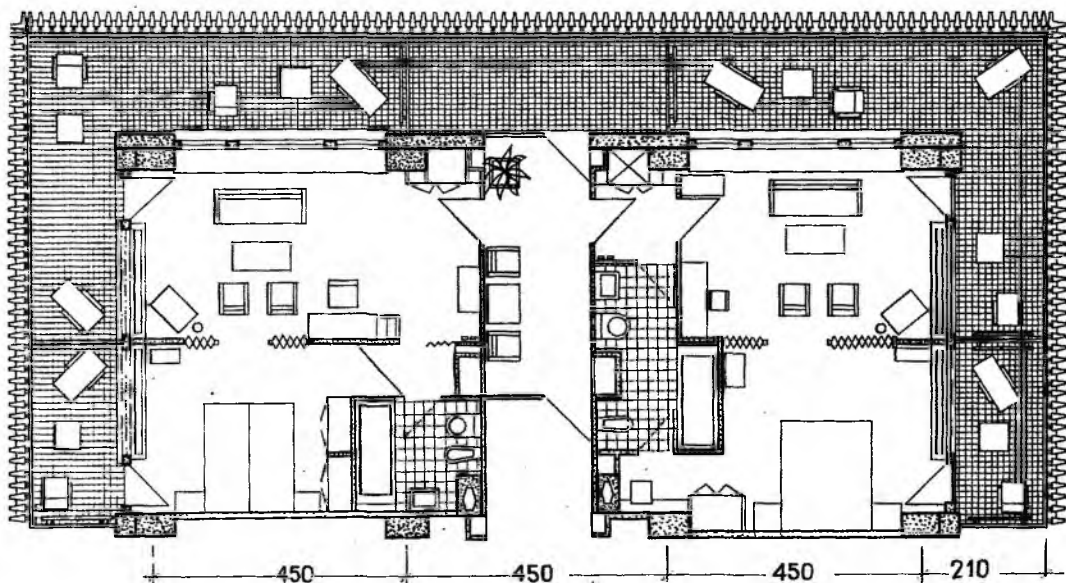
Рис. 31.13. Варианты планировки номеров в курортной гостинице «Ялта»
