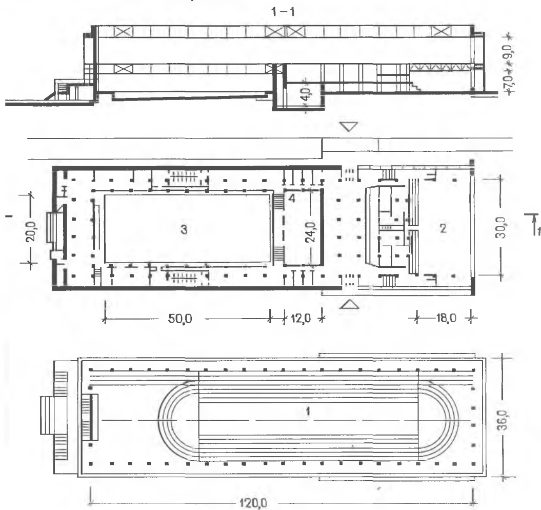
Рис. 20.1. Дворец тяжелой атлетики ЦСКА в Москве. Архит. Ю. Кривушенко
