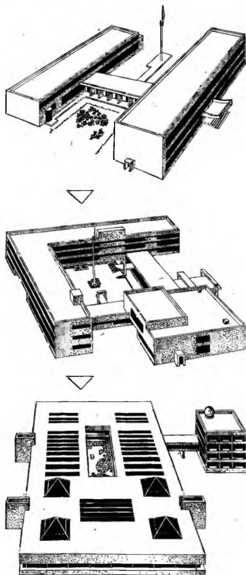
Рис. 9.7. Динамика развития объемно-планировочной структуры школьного здания (на 30 классов)
