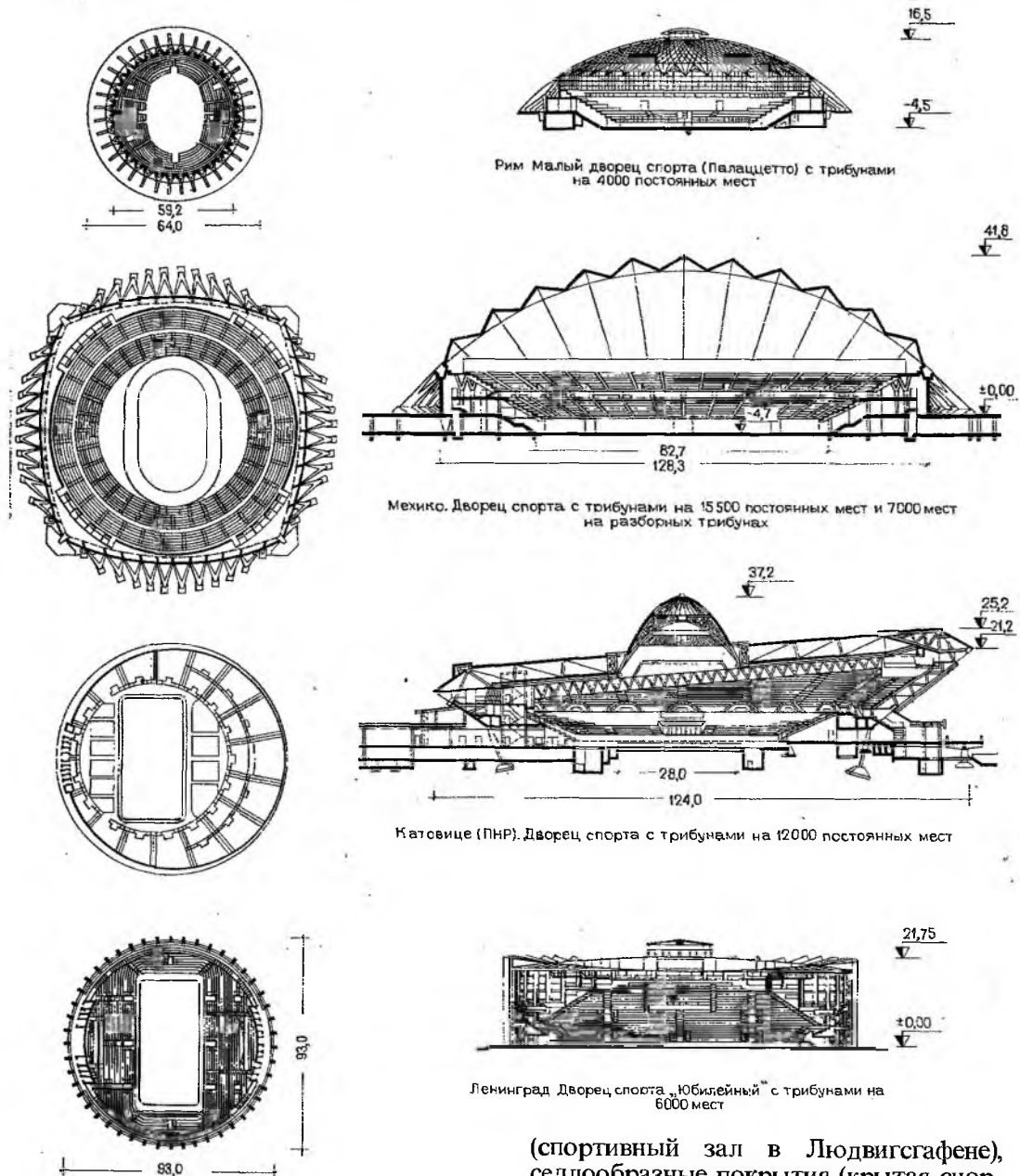
Рис. 20.9. Приемы композиции зрелищно-спортивных универсальных залов
