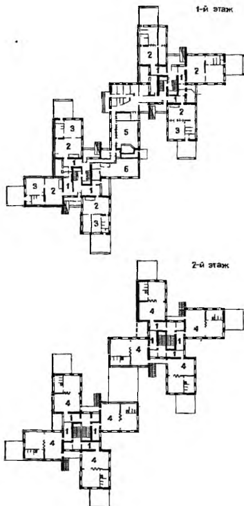
Рис. 8.4. Ясли-сад на 320 мест в г. Тольятти. Планы этажей
