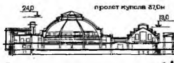
пролет купола 27,0м Покрытие квадратного зала - многоугольный железобетонный купол, прямоугольного - арочный свод
