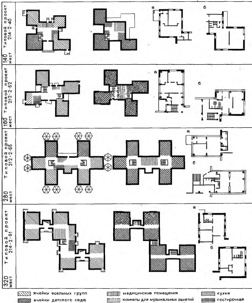
Рис. 8.3. Композиционные схемы зданий и решение групповых ячеек детских дошкольных учреждений а - ячейки ясельных групп; б - ячейки детского сада
