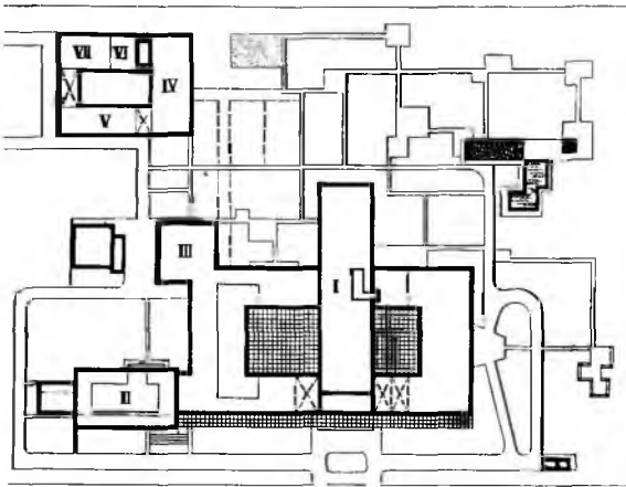
Рис. 30.2. Многопрофильная городская больница на 600 коек. Типовой проект. Архитекторы К. Матюхи и Е. Ефремова. Широкий палатный корпус решен по двухкоридорной системе. На этаже 60 коек (две секции по 30 коек). Лечебно-диагностический блок расположен в стиловатой части. Общий вид, генеральный план, план 1-го этажа
