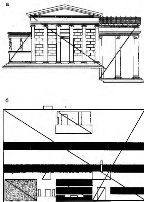
Рис. 1.11. Пропорции сооружений, построенных на подобии геометрических фигур
