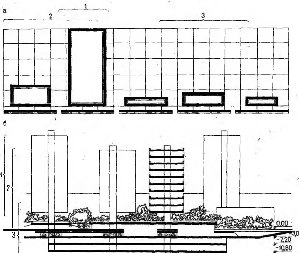
Рис. 11.3. Основные приемы функционального зонирования НИИ а - схема глубинного зонирования; б - схема
