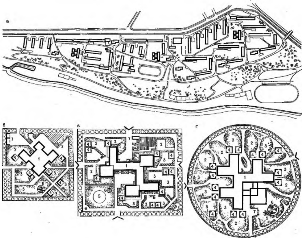
Рис. 8.1. Размещение в жилой застройке и планировка участков детских дошкольных учреждений а - микрорайон в Вильнюсе; б - планировка участка яслей-сада на 140 мест; в - планировка участка яслей-сада на 280 мест; г - планировка участка
