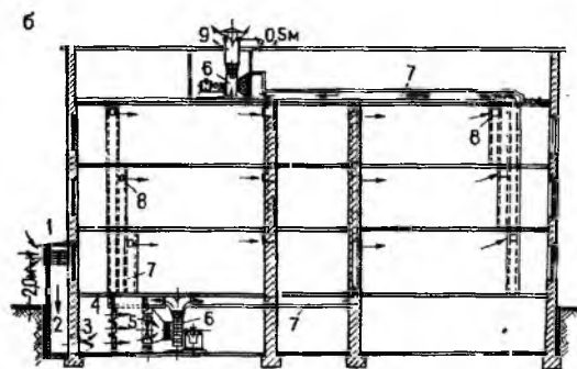
Рис. 6.4. Система вентиляции а — схема устройства вентиляции в многоэтажном здании с вертикальным сборным каналом (1), с горизонтальным сборным каналом (2); б — приточно-вытяжная вентиляция общественного
