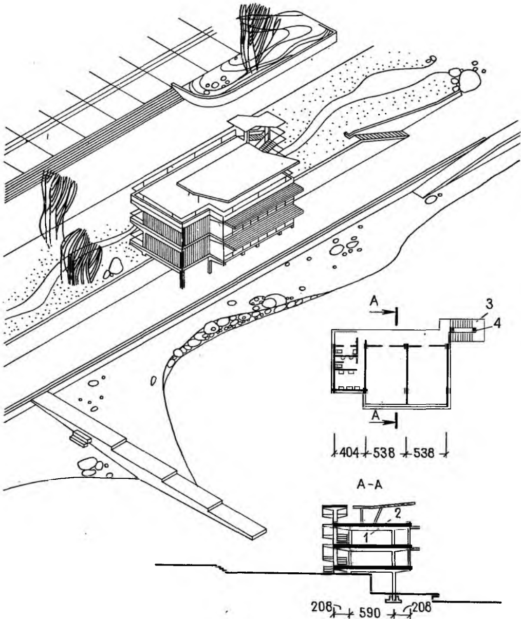
Рис. 3.2. Пионерский лагерь «Морской» Спальный корпус на один отряд выполнен из четырех унифицированных стандартных железобетонных
