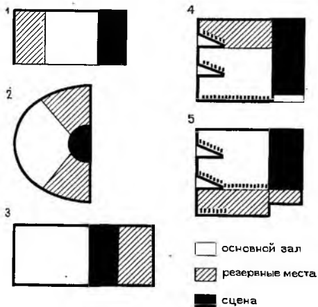
Рис. 14.5. Схемы трансформации клубного зала. Подключение резервного зала: 1 — за задней стеной (план); 2 — за боковой стеной (план); 3 — со стороны сцены (план); 4 — сверху движущийся подвесной потолок, разрез; 5 — снизу движущийся партер (разрез)
