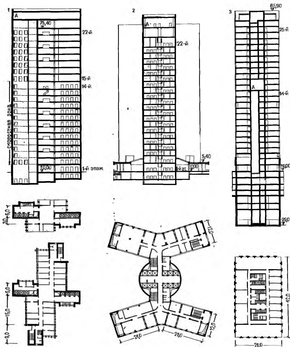
Рис. 25.10. Организация вертикального транспорта в зданиях повышенной этажности
