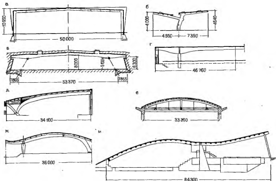
Рис. 4.4. Рамные конструкции больших пролетов а - выставочный павильон
