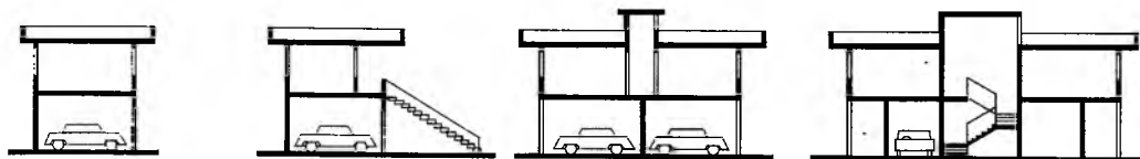
Стоянки автомобилей рядом с жилыми номерами (одно- и двусторонние)
