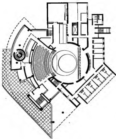
Рис. 13.11. Театр в Аркалыке, КазССР. Архитекторы Ю. Катаев, А. Лукьянов, Ю. Соколов, И. Раевская. План, разрез
