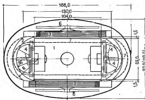
Рис. 18.1. Спортивное ядро Олимпийского стадиона
