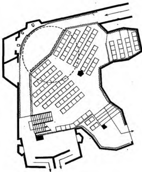
Рис. 13.9. Камерные театры. Италия. Планы этажей
