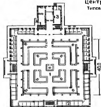
1-торговый зал, 2-палатка; 3-контрольная станция
