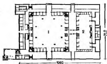
1-купольный зал для смешанной торговли; 2-зал для рыбной торговли
