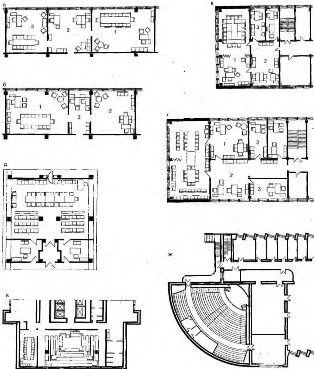
Рис. 25.4. Планировка помещений а и б — блок помещений руководства учреждением;
