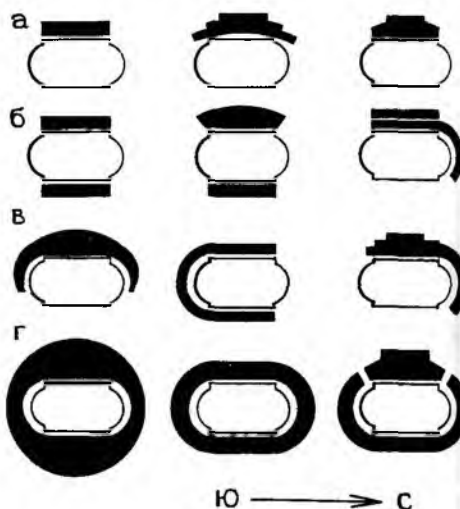
Рис. 19.6. Приемы расположения трибун стадиона
