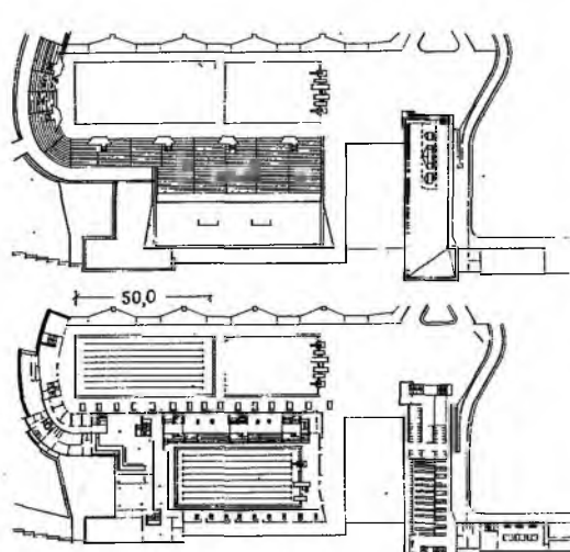
Прага. Плавательный бассейн „Не Подоле“
