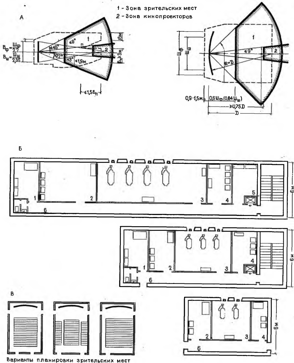
Рис. 12.12. Планировочные элементы кинотеатров А - схемы нормативного расположения зрительских
