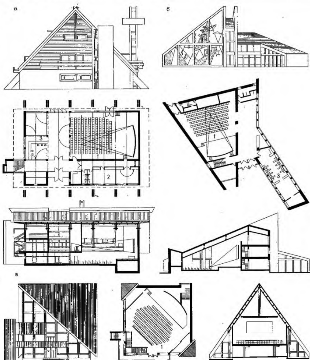
Рис. 14.1. Сельские клубы а – конкурсный проект сельского клуба с залом на 200 мест. Архитекторы Д. Радыгин, А. Баталов,
