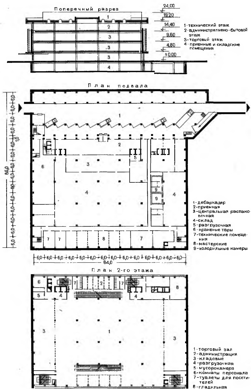
Рис. 23.4. Объемно-планировочная модель универсама с торговой площадью 10 тыс. м 2
