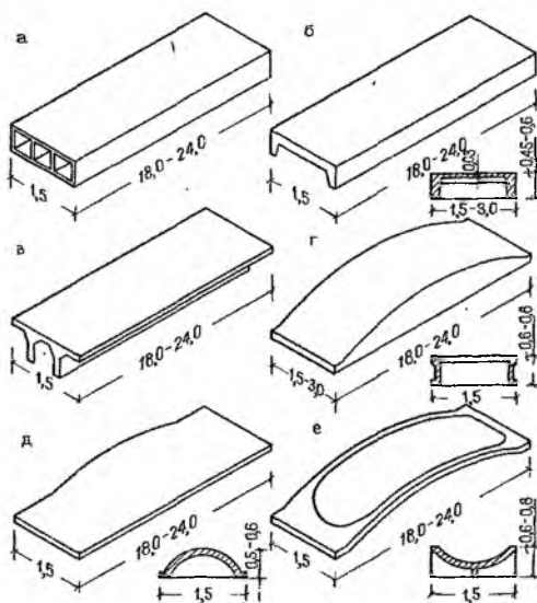
Рис. 4.3. Длиномерные железобетонные сборные настилы покрытий а - пустотный «слатник»;
