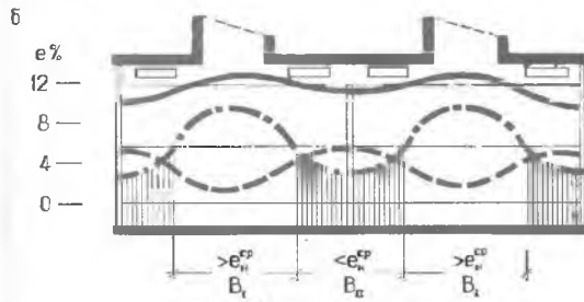
Рис. 5.3. Схемы совмещенного освещения интерьеров а – при боковом естественном
