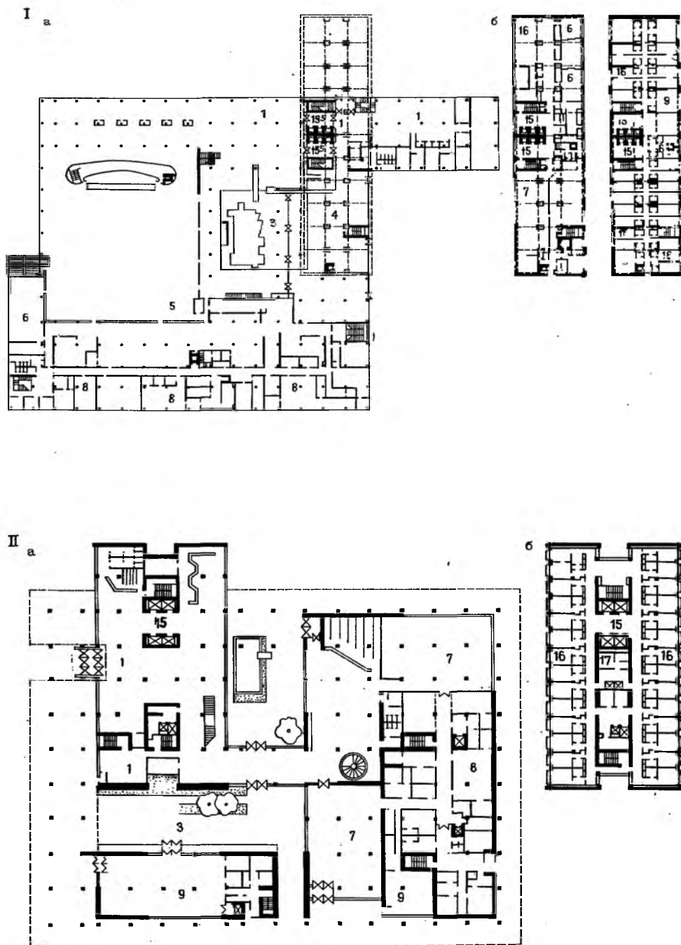
Рис. 26.9. Композиционные решения гостиниц I гостиница «Орлеан» на 1860 мест в Москве; II – гостиница на 935 мест в г. Тольятти; III – гостиница
