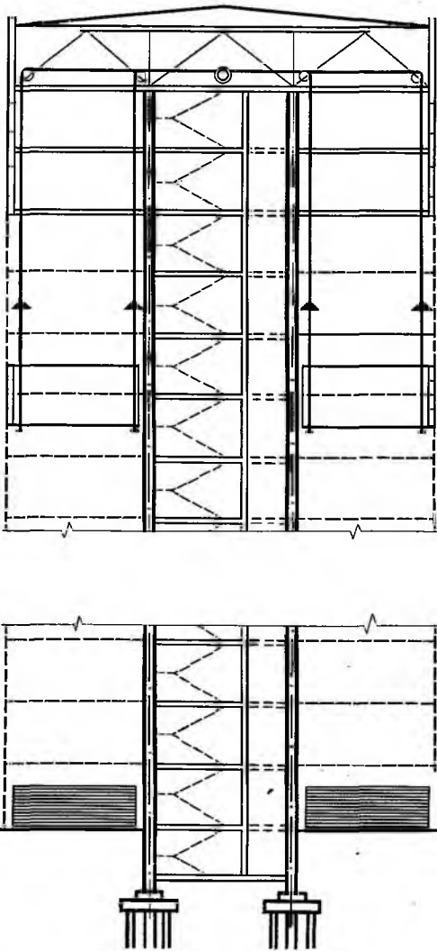
Рис. 4.2. Каркас высотного здания с несущим ядром жесткости
