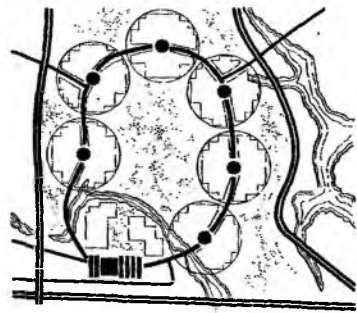
Отрадное (проект, г.Москва)
