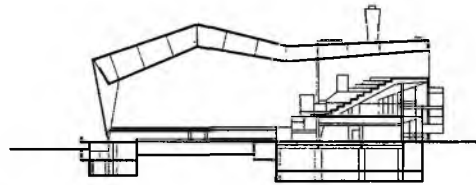
Токио. Крытый плавательный бассейн Центрального стадиона на 4000 мест с ваннами для плавания и прыжков в воду
