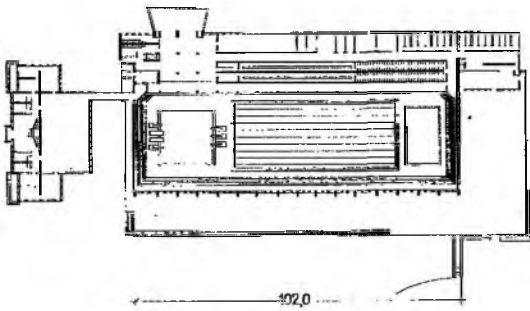
Минск. Комплекс открытых и закрытых плавательных бассейнов. В закрытом бассейне ванны 21 \times 50 , 20 \times 20 и 10 \times 20 м
