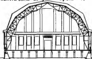
Покрытие - металлические трехшарнирные арки
