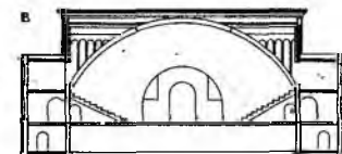
Покрытие - туфожелезобетонные короткие оболочки, защемленные арками
