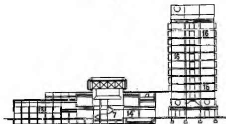
Рис. 26.10. Композиционные решения гостиниц
