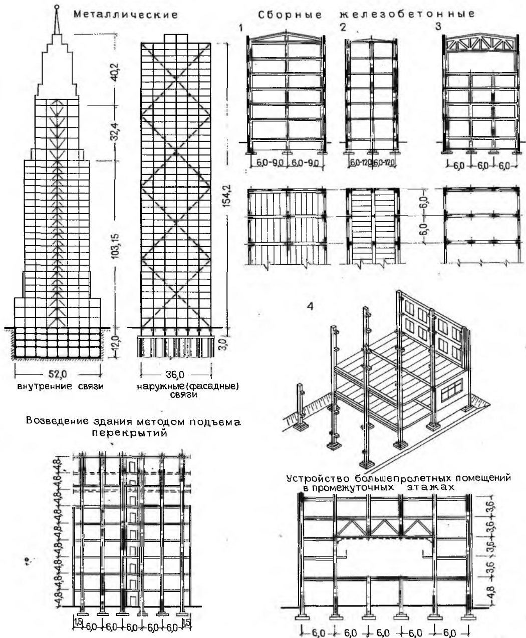
Рис. 4.1. Каркасы многоэтажных гражданских зданий
