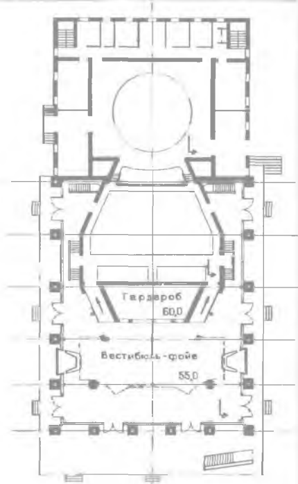
Рис. 13.10. Театр в Махачкале, ДзгАССР. Архитекторы Г. Мовчан, С. Галаджеева, В. Красильников. Общий вид, план
