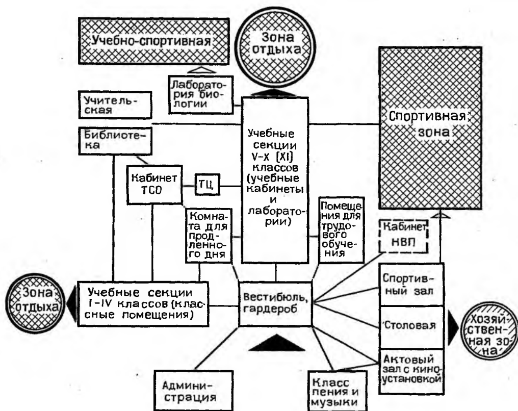
Рис. 9.3. Структура и взаимосвязь помещений школьных зданий
