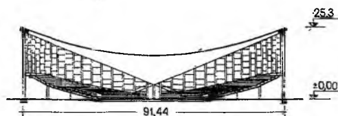
Рэлей, США. Крытая спортивная арена с трибунами на 5500 мест
