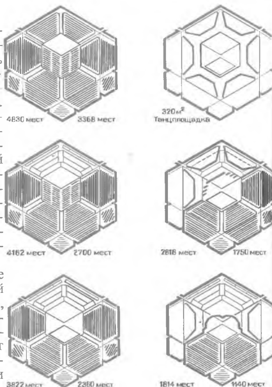
Рис. 13.2. Дворец Республики в Берлине, ГДР. Общий вид, планы этажей, разрез, схемы
