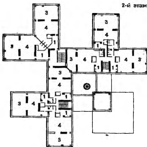
Рис. 8.4. Ясли-сад на 320 мест в г. Тольятти. Планы этажей
