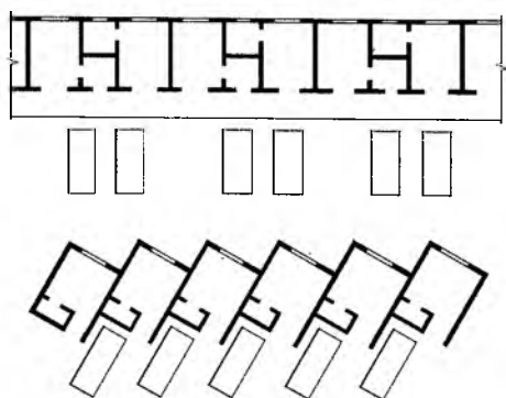
Стоянки автомобилей перед жилыми номерами (одно- и двусторонние)
