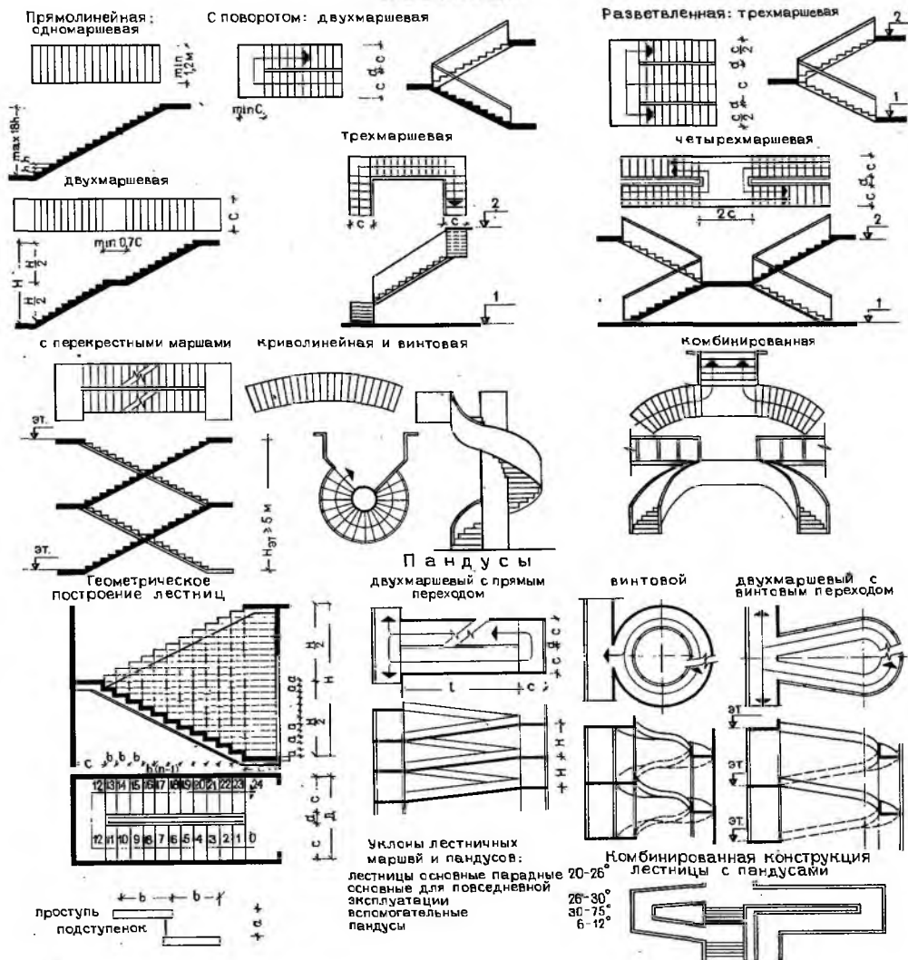
Рис. 2.5. Принципиальные схемы лестниц и пандусов
