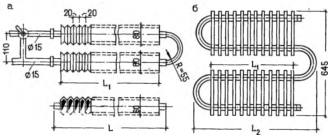
Рис. 6.3. Конвекторы а — плитусные КП без кожуха; б — «аккорд» двухрядный
