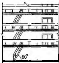
Рис. 2.4. Планировочные решения входных узлов
