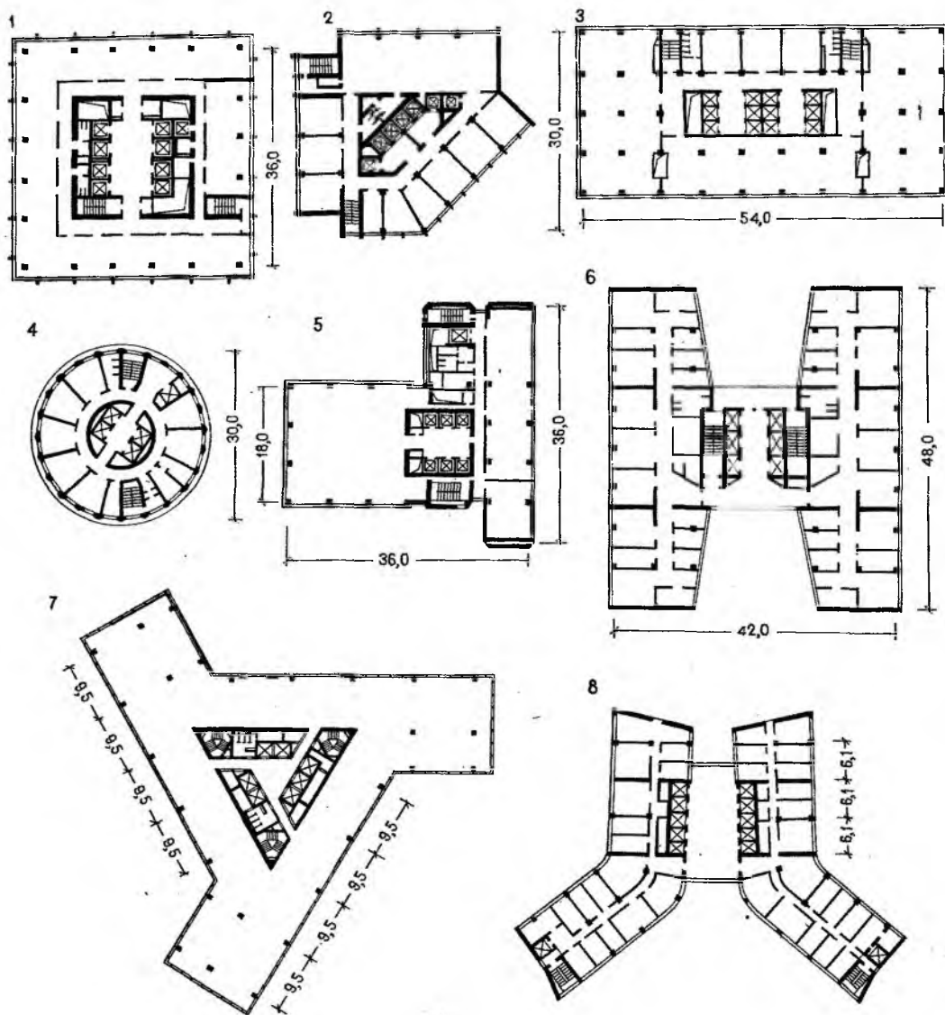
Рис. 25.8. Типичные системы планировки зданий повышенной этажности. Компактная планировка: 1- здание заводоуправления в г. Тольятти (проект); 2- административное здание в Кисево; 3- Дом проектных организаций на просп. Вернадского в Москве; 4- здание
