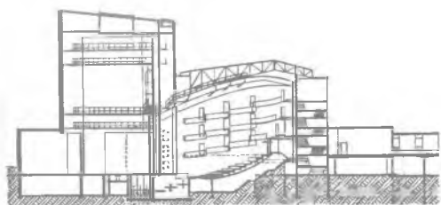
Рис. 13.8. Театр в Мюнстере. ФРГ. Архит. Рунгау. Интерьер зала, план, разрез
