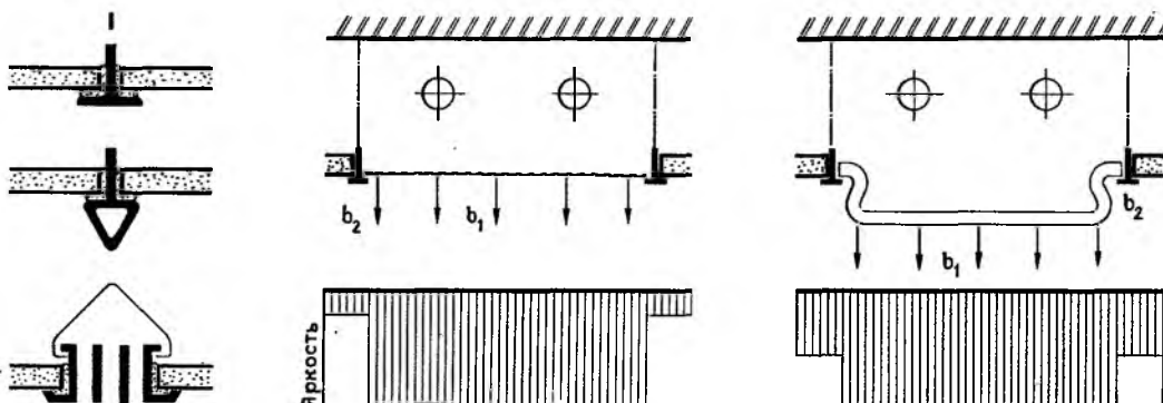
Рис. 5.7. Детали потолка, создающие различные яркостные контрасты между светящейся поверхностью и переплетом
