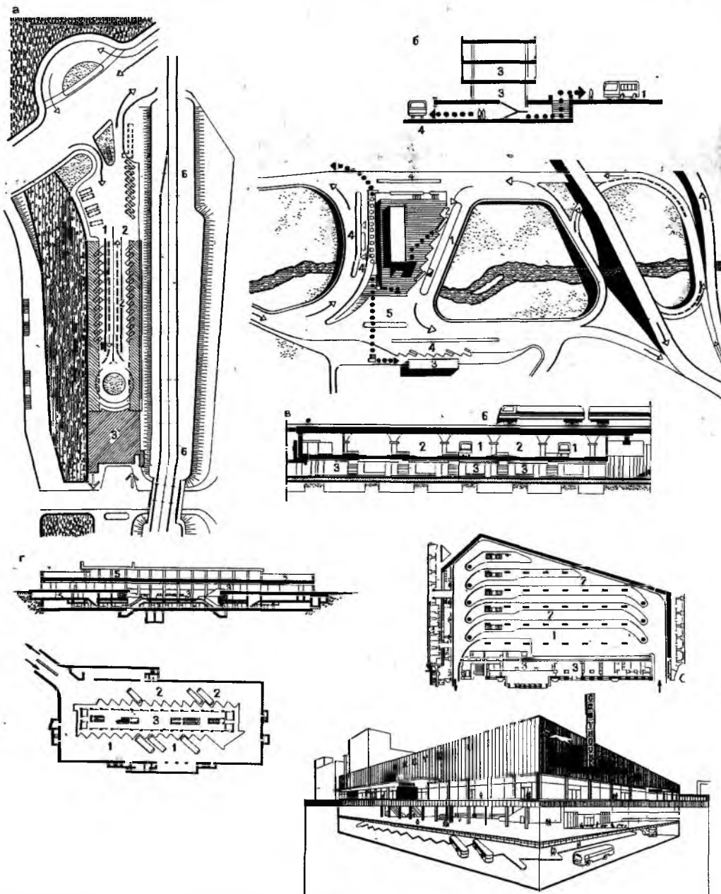
Рис. 29.6. Автобусные вокзалы а - автобусный вокзал в Риге, генеральный план; б - автобусный вокзал в Ялте, генеральный план и поперечный разрез;
