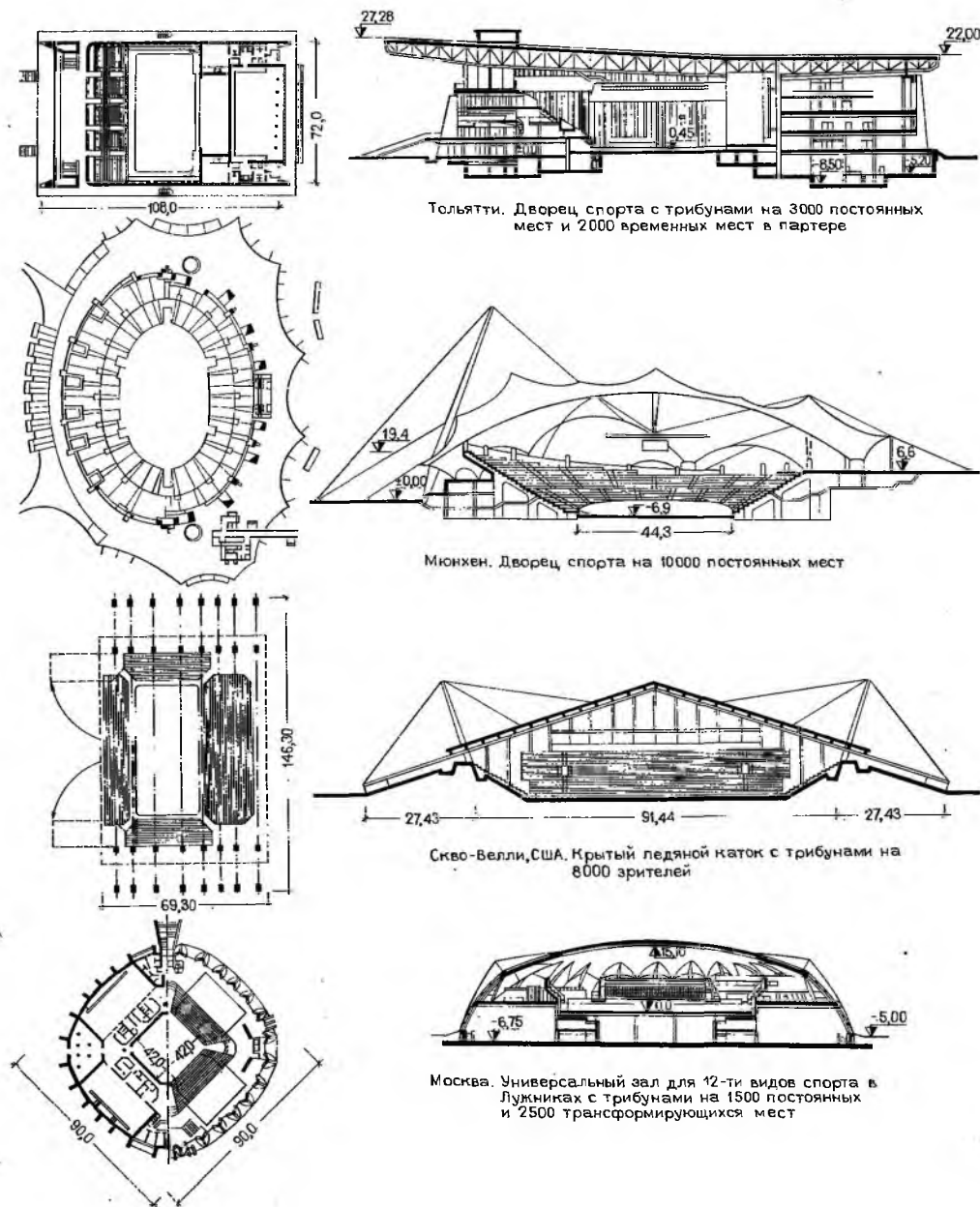
Рис. 20.10. Прямые композиции зрелищно-спортивных универсальных залов
