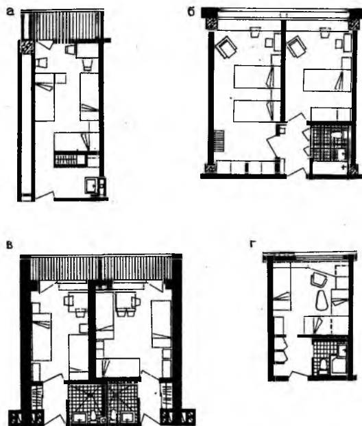
Рис. 26.7. Варианты планировки номеров
