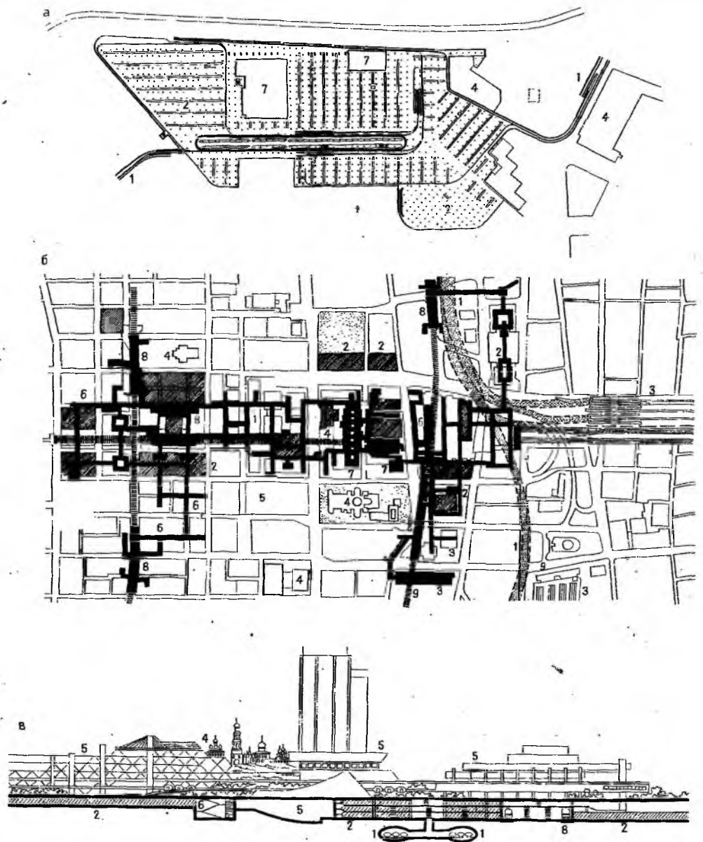
Рис. 28.5. Проекты многоуровневых подземных автостоянок и гаражей, распространяющихся на значительные территории крупнейших городов а — проект реконструкции Центральной площади района Каипи в Хельсинки
