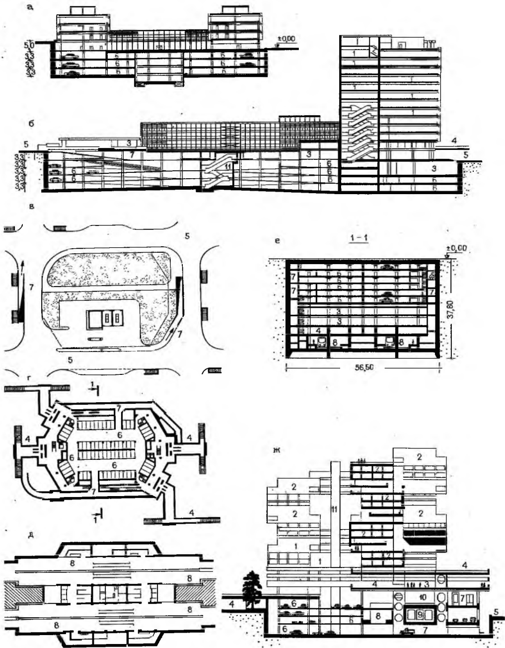
Рис. 28.4. Многофункциональные общественно-транспортные комплексы с многоуровневой организацией хранения транспортных средств а, б — административный комплекс в Лос-Анджелесе (США) со встроенными подземными автостоянками
