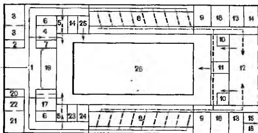
Рис. 20.20. Схема планировки бассейна
