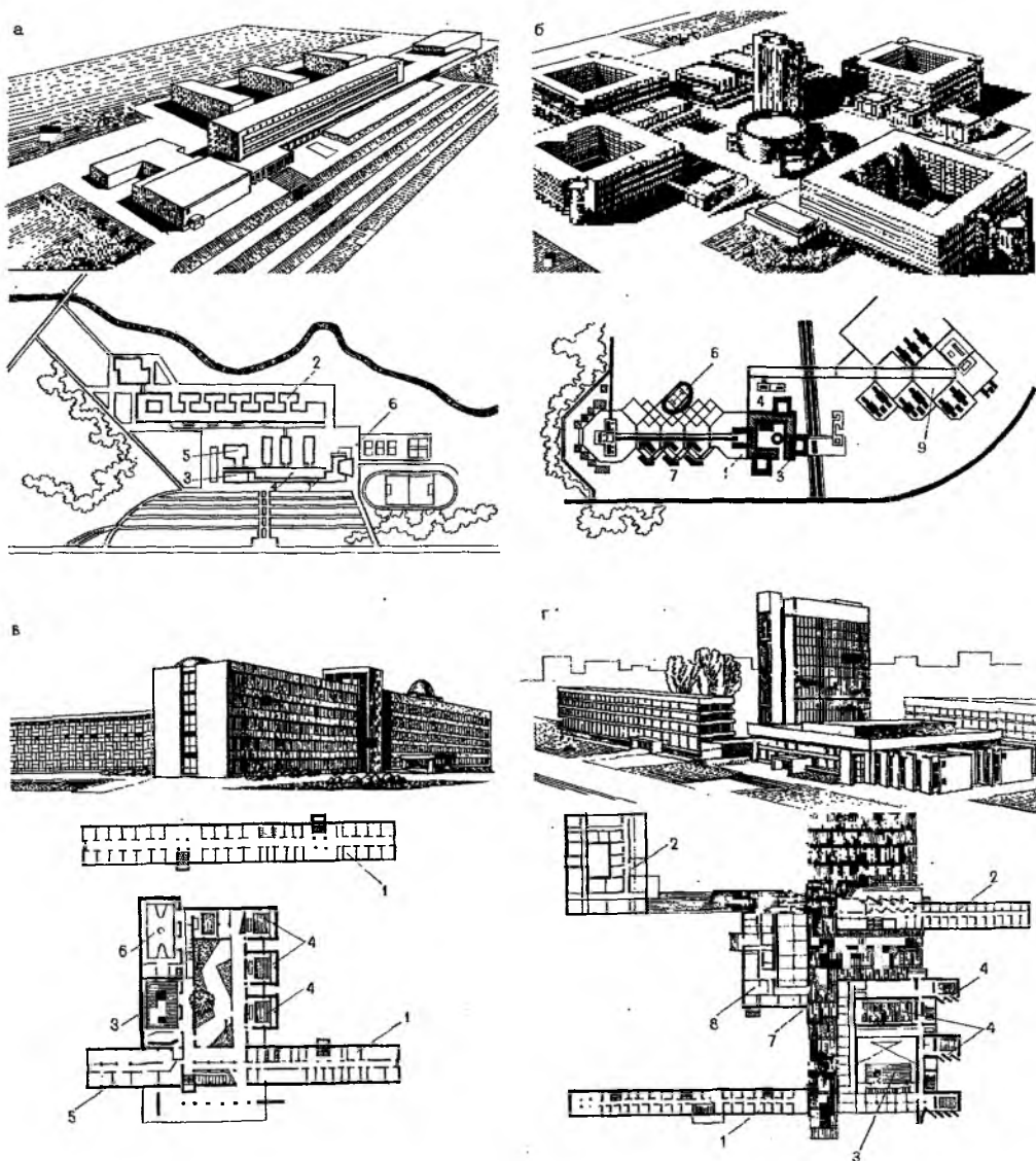
Рис. 10.3. Высшие учебные заведения с контингентами студентов средней величины (2-5 тыс. студентов)
