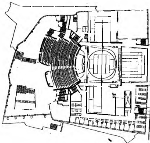
Рис. 13.3. Театр в Эссене, ФРГ. Архит. А. Аапо. Разрез, планы этажей
