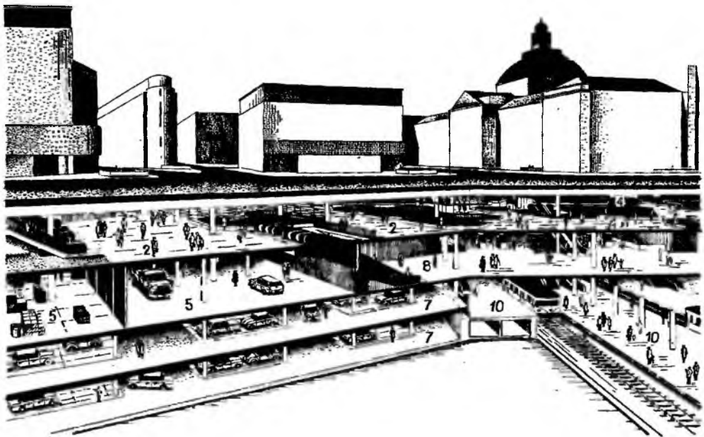
Рис. 27.3. Система подземных пешеходных переходов, объединенная с подземным торговым центром, подземной железнодорожной
