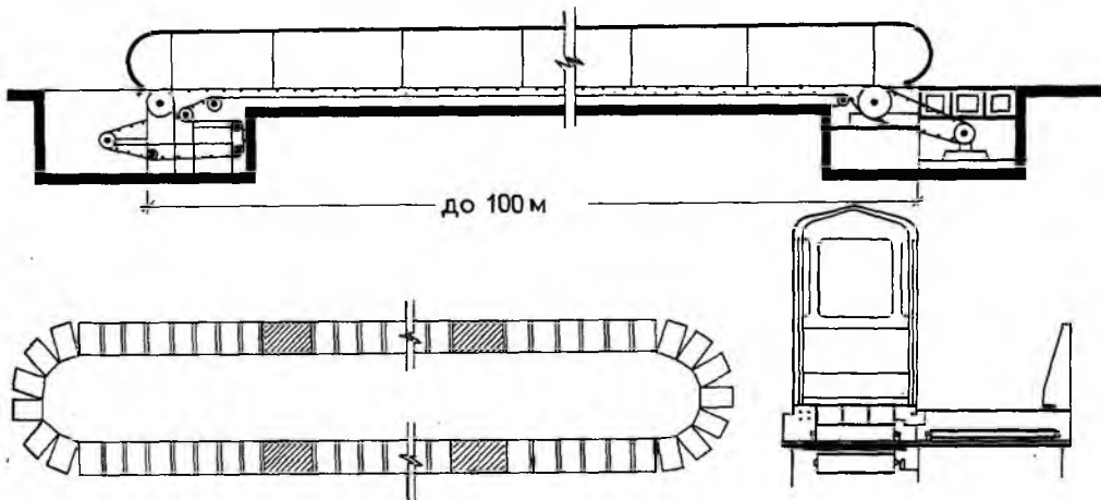
Рис. 28. Движущийся тротуар и карьерейер
