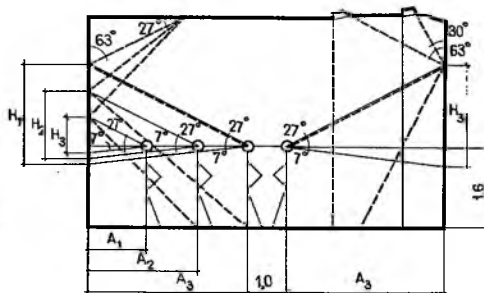
Рис. 16.7. Теоретические условия освещения при верхнем свете (по Г. Реттмузу)
