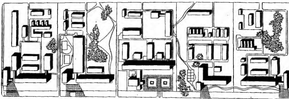
Рис. 11.2. Схема генерального плана комплекса НИИ научного центра в г. Пушкине. Планировочная структура комплекса основана на
