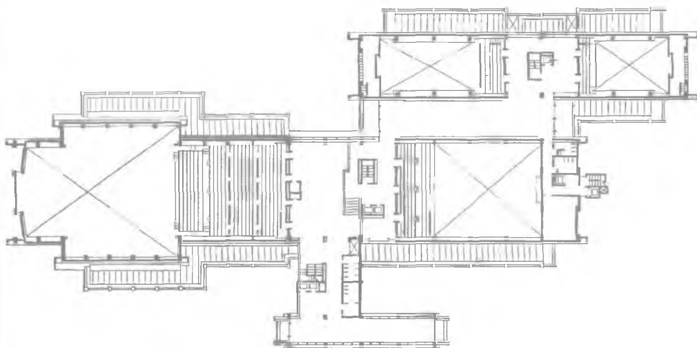
Рис. 13.15. Международный центр в Киото. Япония. Общий вид, план этажа
