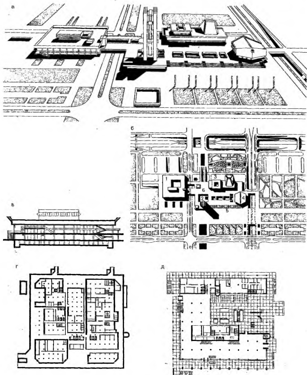
Рис. 24.8. Общественно-торговый центр в г. Тольятти. Архитекторы Б. Рубанико, А. Образцов
