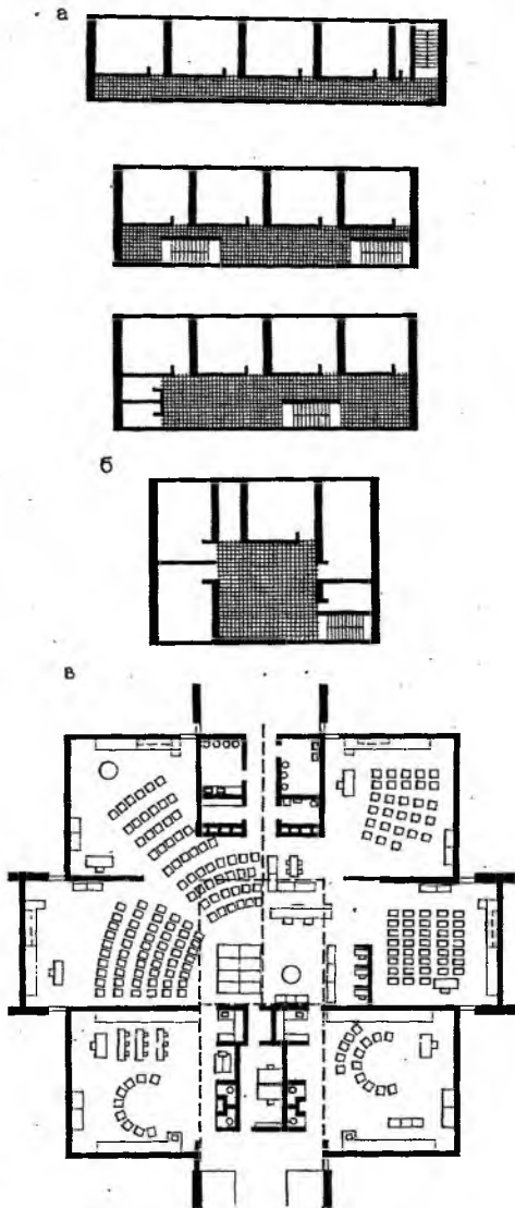
Рис. 9.5. Динамика преобразования учебной секции школьного здания а - линейная учебная секция;
