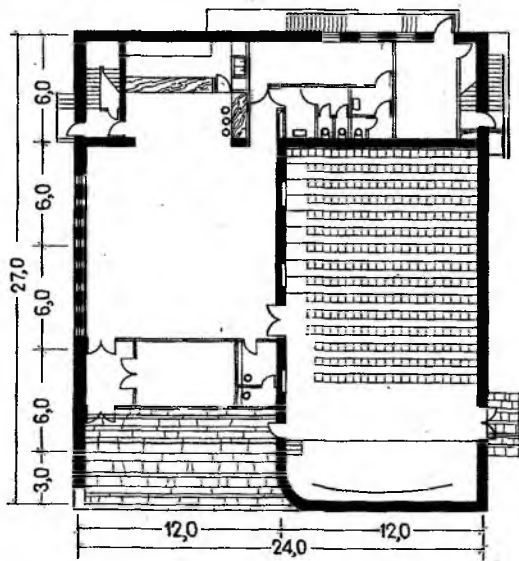
Рис. 12.1. Кинотеатр на 300 мест. Типовой проект. Архитекторы М. Бубнов, В. Лазарев. План
