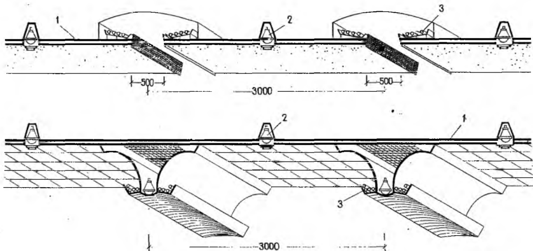
Рис. 5.7. Детали потолка, создающие различные яркостные контрасты между светящейся поверхностью и переплетом
