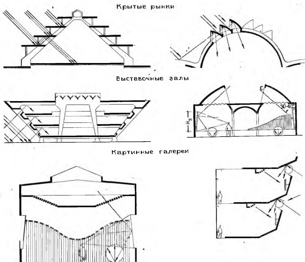
Рис. 5.6. Приемы естественного освещения зданий
