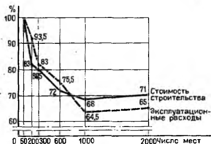
Рис. 7.3. Влияние вместимости больницы на стоимость строительства и эксплуатационные расходы (из расчета на 1 койку)
