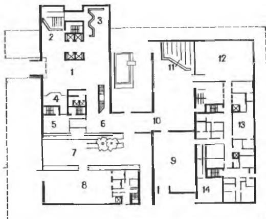
Рис. 26.5. План общественной части
