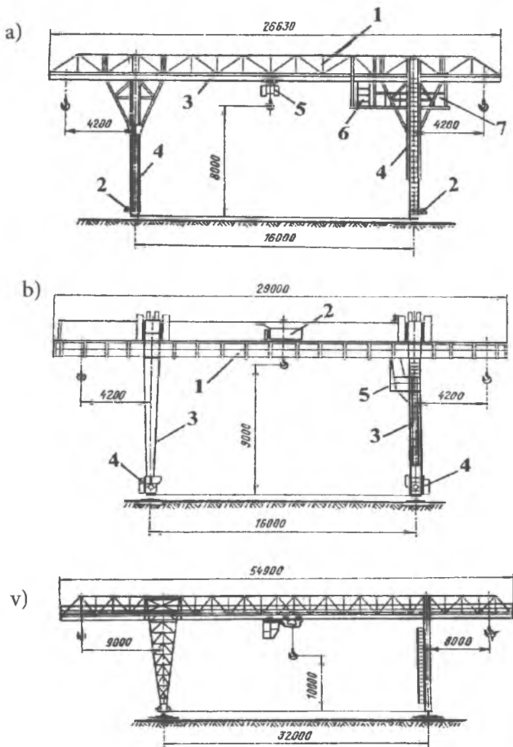
5.18-rasm. Ikki konsolli chorpayali kranlar.
