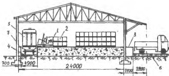
6.7-rasm. Ichkarisida temir yo‘li va tashqarisida avtoyo‘lak joylashgan yopiq ombor (1GS) ning ko‘ndalang chizmasi
