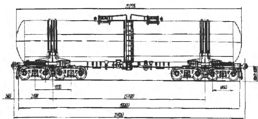
5.10-rasm. Sakkiz o'qli universal sistema
