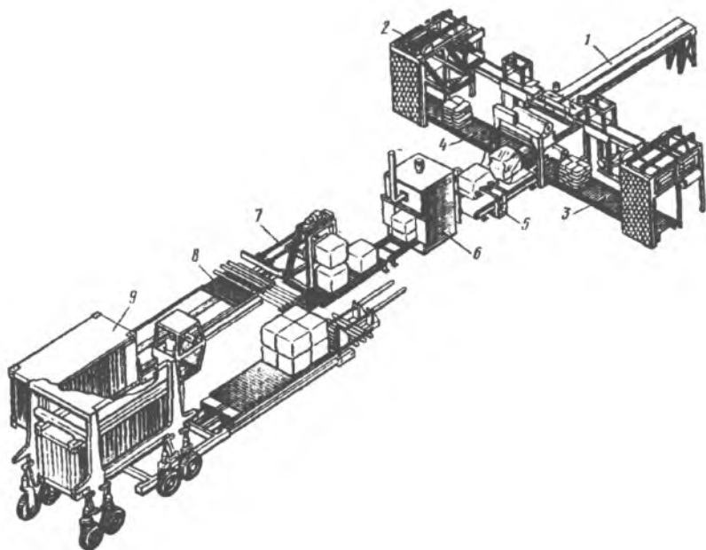
5.6-rasm. Avtomatik qoliplovchi liniya chizmasi.
