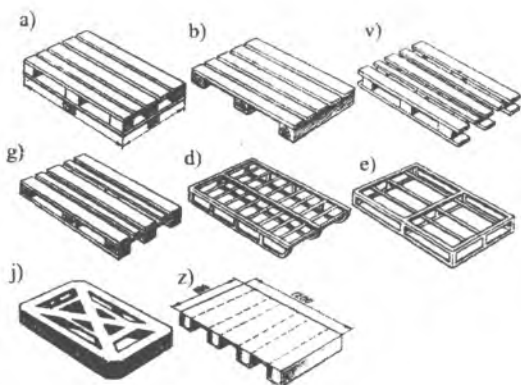
5.1-rasm. Yassi tagliklar.
