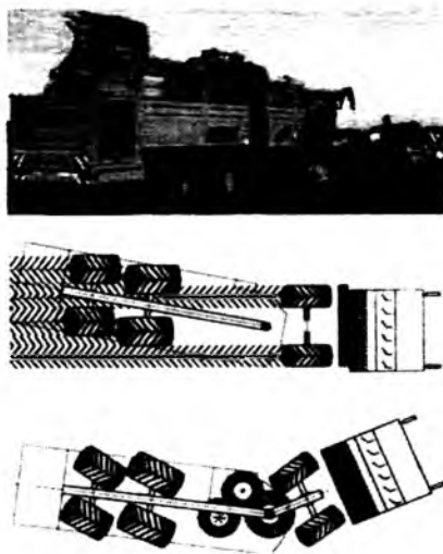
1.14-rasm. Kompyuterlashtirilgan rul boshqarmasi ega Ropa firmasining gidrostatik uzatkichli o'ziyurar mashinasi.
