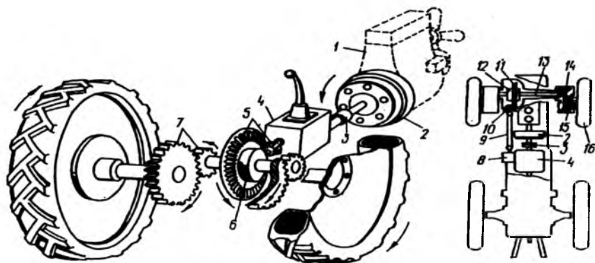
1.8-rasm. G'ildirakli traktorlar kuch uzatmasining sxemasi:
