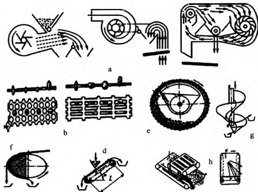
2.36-rasm. Mahsulotlarni tozalash va saralash usullari:
