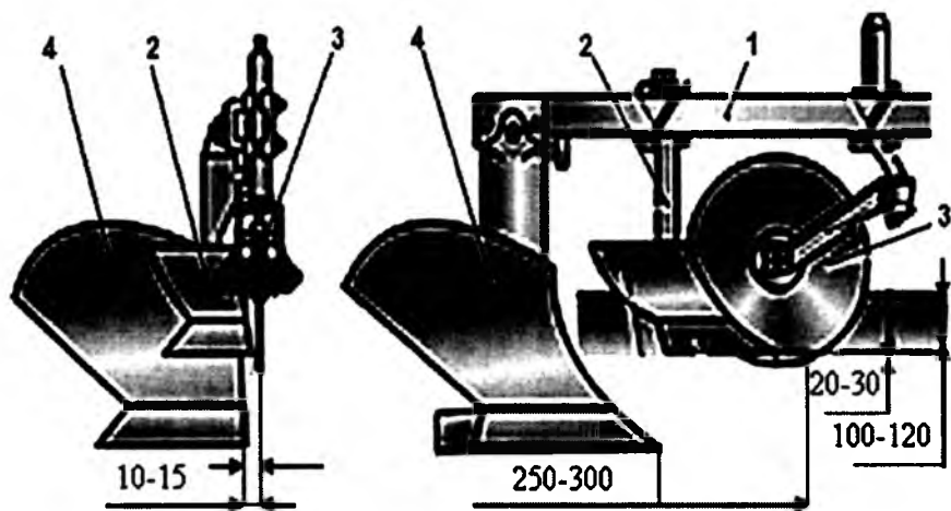
2.3-rasm. Plugning asosiy qismlari va ularni rostlash o'lchamlari: 1 – rama; 2 – chimqirqar; 3 – diskli pichoq; 4 – asosiy korpus.
