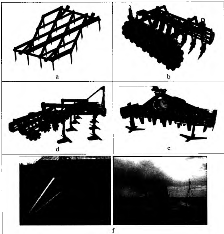
2.7-rasm. Tuproqqa sayoz ishlov berish mashinalari: a) tishli borona; b) diskli borona; d) chizel kultivator; e) tuproq frezasi; f) lazer boshqaruvli yer tekislagich.
