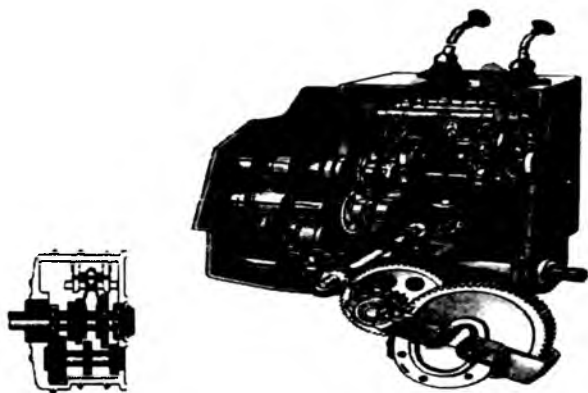
1.7-rasm. Traktor uzatmalar qutisi 1920-yillar (chapdagi rasm) va 2 guruppali uzatmalar qutisi Schonenber firmasi 8 ta oldinga va 8 orqaga tezligi bilan, dvigatel bilan uzatmalar qutisi sapfa validagi yoqilishlar 1950-yillar oxiri.
