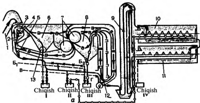
2.41-rasm: SM-4 don tozalash-saralash mashinasining tuzilishi va ish jarayoni: 1 – yuklovchi transporter; 2 – havo bilan tozalash qurilmasi; 3 – g‘alvirlar; 4 – ikki oqimli elevator; 5 – triyerlar.
