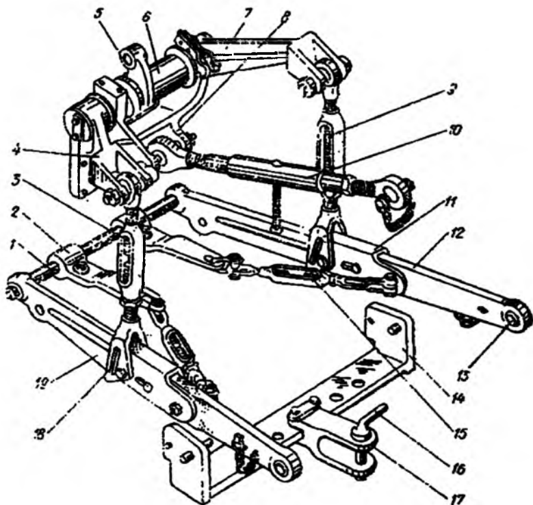
1.15-rasm. Traktorning o'rnatish mexanizmi:
