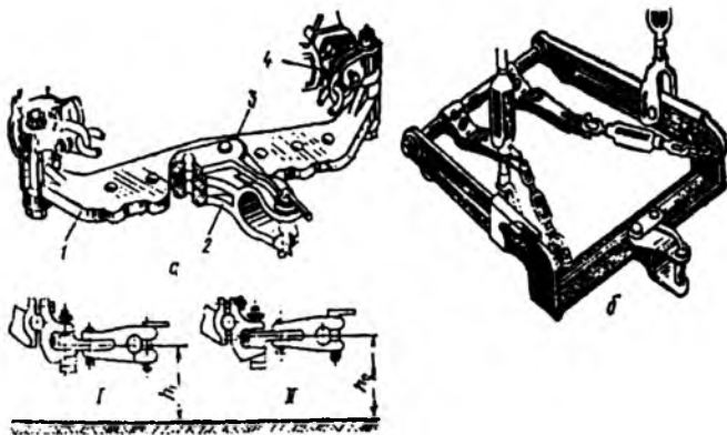
1.16-rasm. Traktorning tirqash moslamasi:
