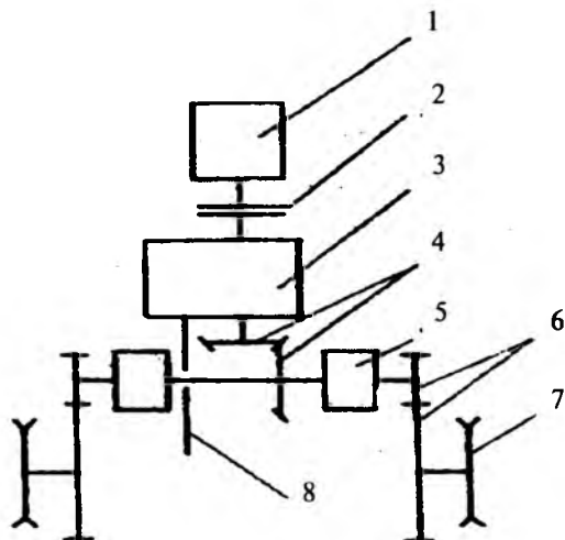
1.9-rasm. Avtomobilning kuch uzatish qismi: 1 — dvigatel; 2 — ilashish muftasi; 3 — uzatmalar qutisi; 4 — bosh uzatma; 5 — planetar mexanizm; 6 — oxirgi uzatma; 7 — yetaklovchi g'ildirak; 8 — quvvat olish vali.
