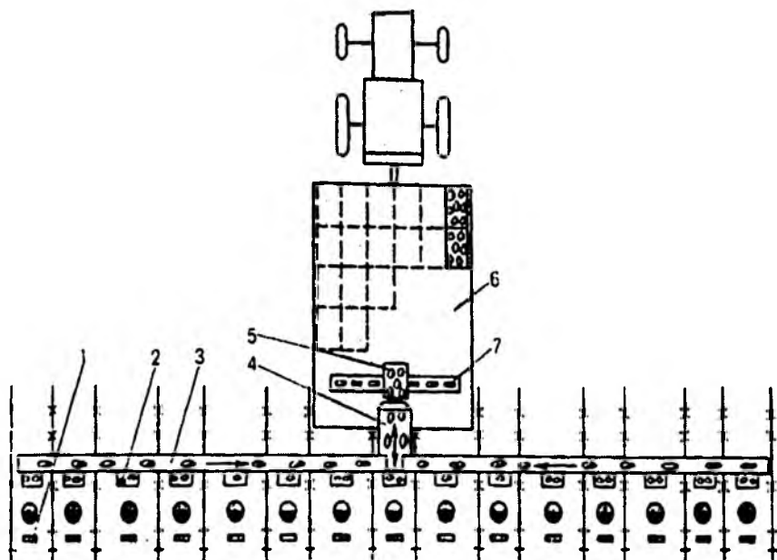
2.45-rasm. AUS-0,1 sabzavotlarni qo'lda terib olish agregati:
