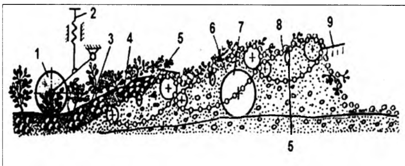
2.44-rasm. KST-1,4 kartoshka kovlagichning tuzilishi va ish jarayoni:
