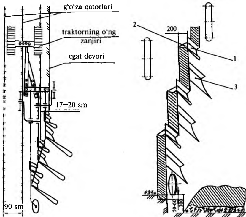
2.6-rasm. Ikki yarusli plugning texnologik jarayoni:
