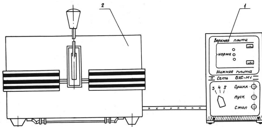
4 -rasm. VXS-M1 tezkor namlikni o'lchash uskunasi 1-boshqarish bloki, 2-quritish kamerasi
