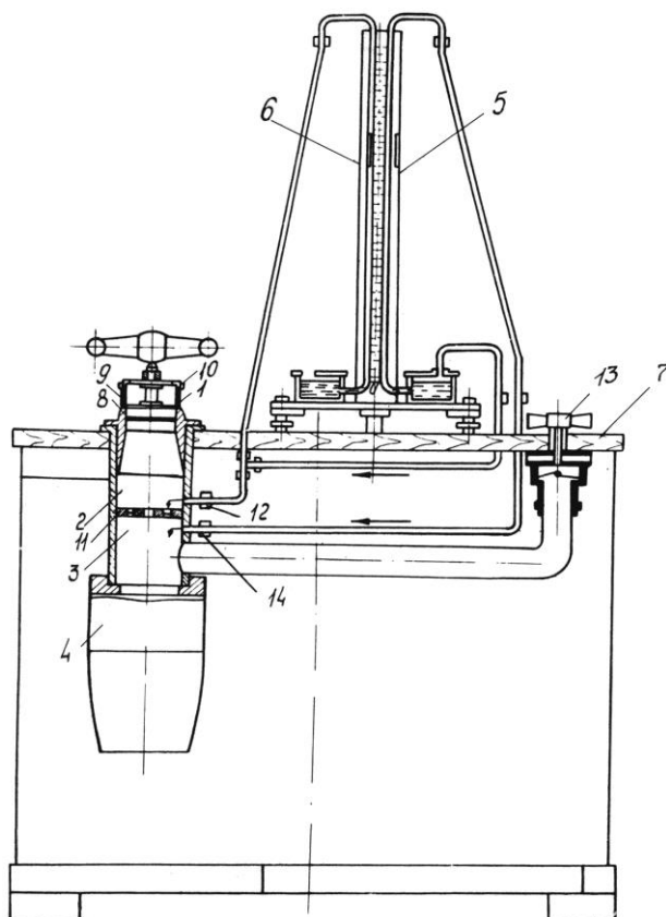
14-rasm. LPS-4 uskunasi chizmasi
