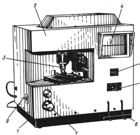
18- rasm. PSV-1 proyeksion tola sanagichining umumiy ko'rinishi
