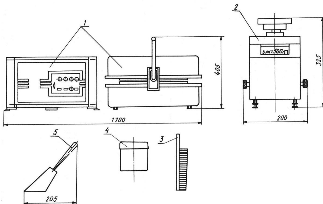
3-rasm. VXS tezkor namlikni o'lchash uskunas
