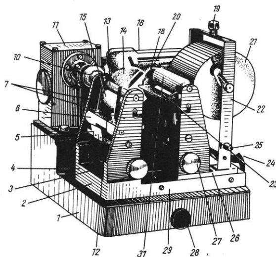
17–rasm. PPL- pilik tayyorlash uskunasi chizmasi
