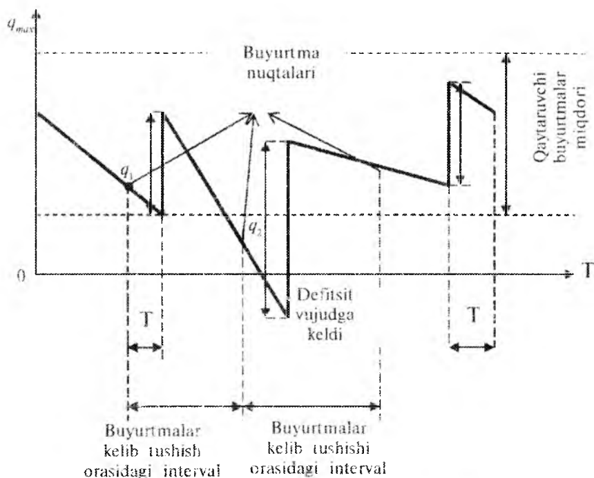
7.2-rasm. Buyurtma davriyligi belgilangan tizim.
