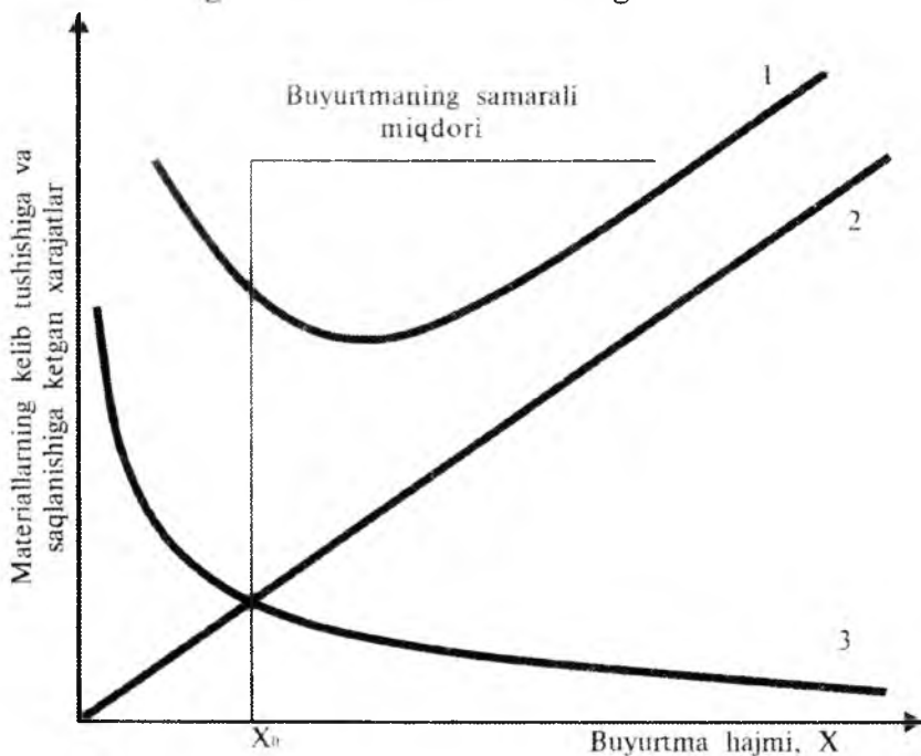
10.3-rasm. Buyurtmaning bajarilishiga va materiallarni saqlashga ketadigan xarajatlarning buyurtma hajmiga bog'liqligi.
