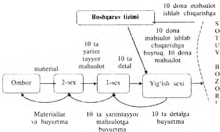
3.4-rasm. Moddiy oqimlarni boshqarishning tortib olish tizimi.
