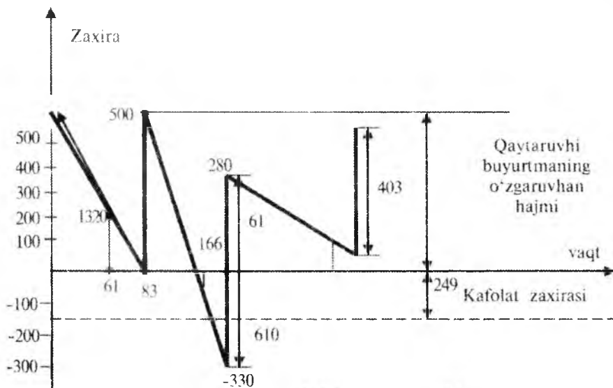
7.3-rasm. Buyurtma davriyligi belgilangan tizimda va materiallarning iste'mol qilinish intensivligi har xil bo'lganda joriy zaxiralar harakatining grafigi.
