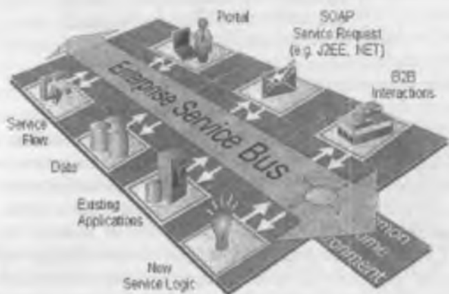
3.1.6. – rasm. SOA komponentlari konsepsiyasi va EBS tuzilishining strukturasi
