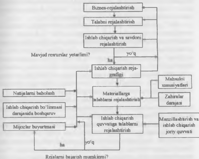
4.2.1-rasm. MRP II tizimining funktsional bloklari
