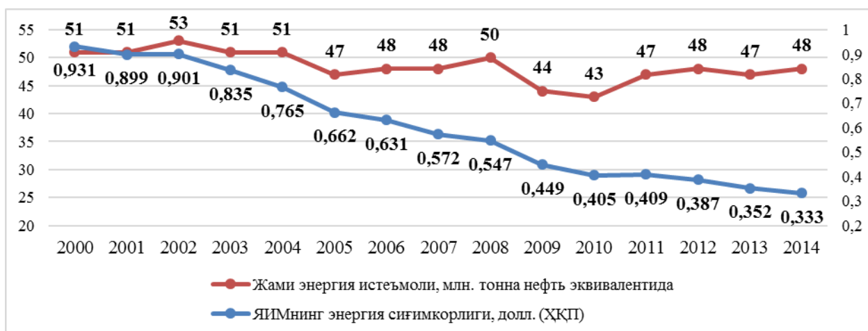
15.2-rasm. O‘zbekistonda jami energiya iste‘moli va yalpi ichki mahsulotning energiya sig‘imkorligi 59
