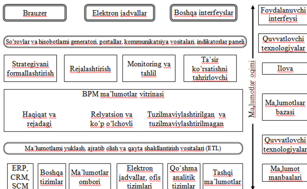
4.2.5.-rasm. BPM-tizim texnologik arxitekturasini
