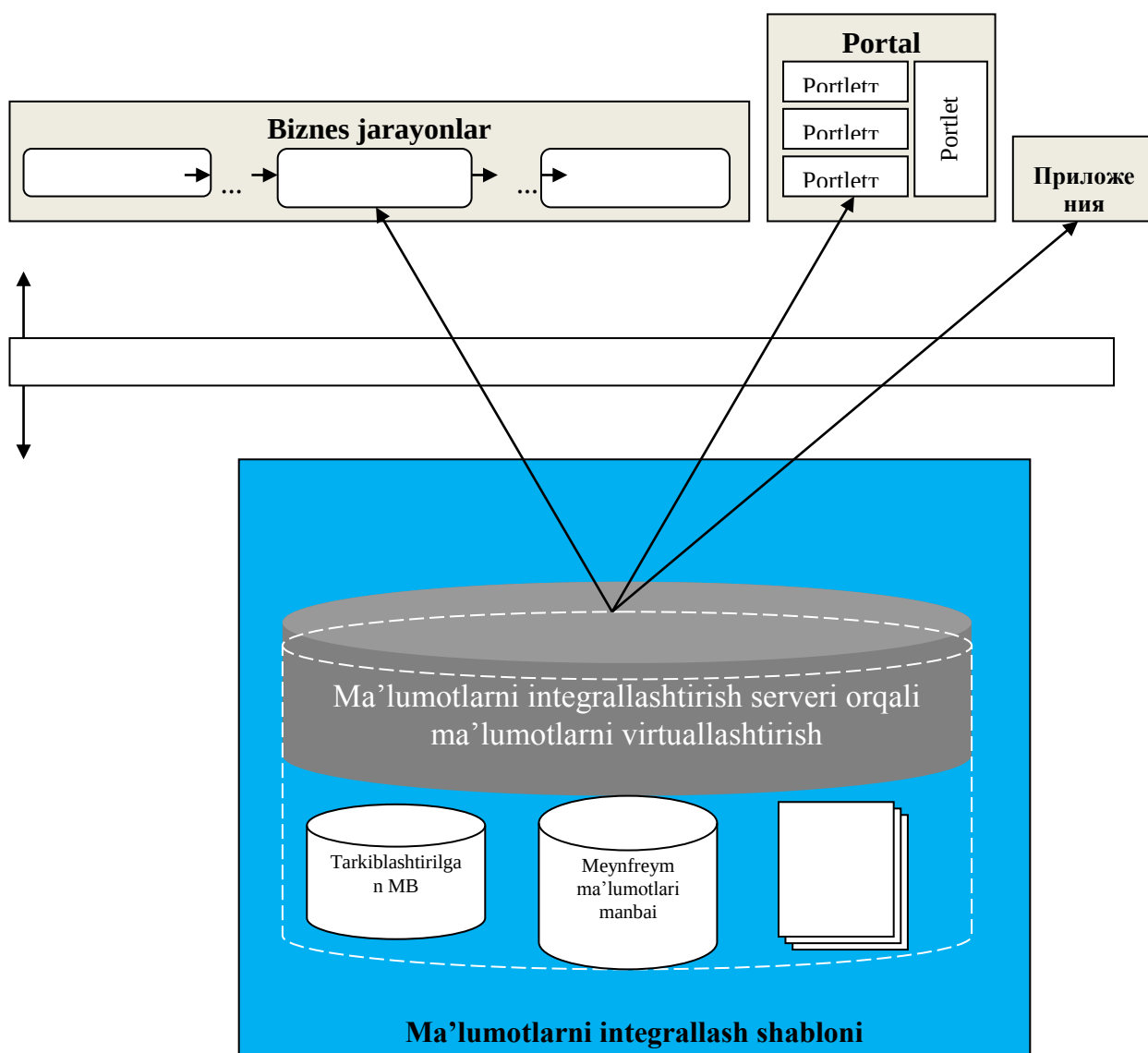
3.1.4. –rasm. Integrallashtirish ma'lumotlar sxemasi
