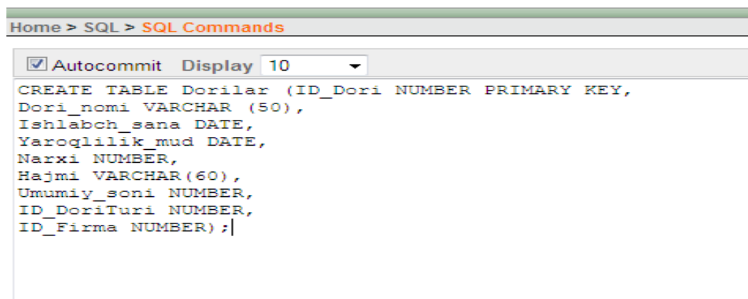
2.2.6-rasm. Dorilar jadvalini SQL tilida yaratish
