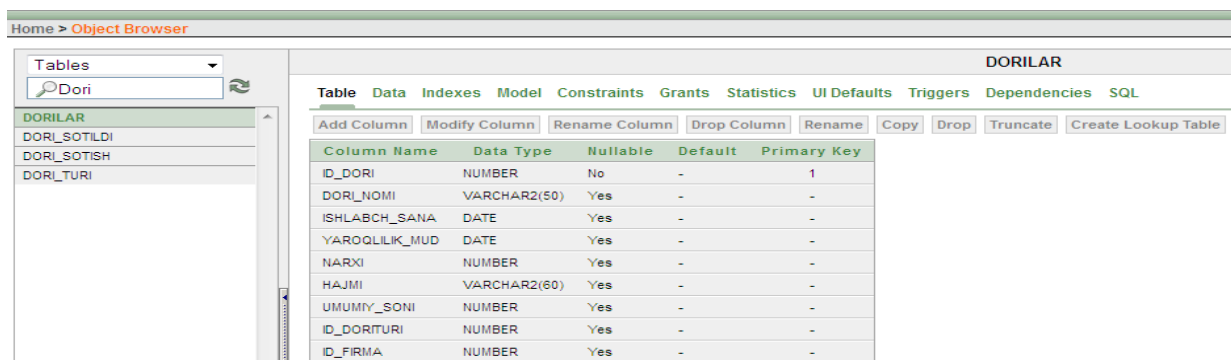
2.2.7-rasm. Dorilar jadvali oynasi
