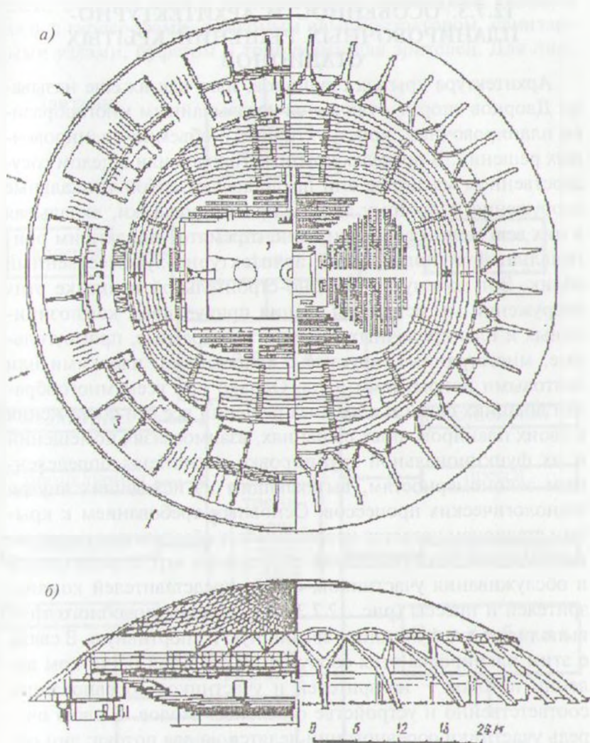
Рис. 12.7.2.1. Малый Дворец спорта в Риме с ареной 28х40 м и трибунами на 5 тыс. мест (арх. А. Вителоччи, инж. П. Перви): а — план (слева — на уровне пола, справа — на уровне верха наклонных опор); б — детали покрытия (пролет 59 м)
