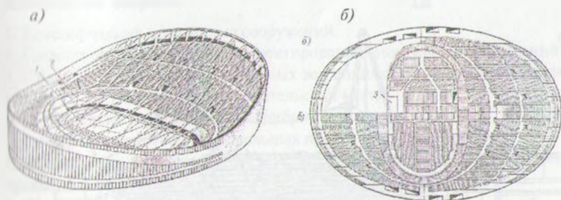
Рис. 12.7.4.2. Пример устройства покрытия стадиона, выполненного в вантовой конструкции из стальных тросов, работающих на растяжение (Дворец спорта в Париже с трибунами на 14 тыс. мест и с трансформируемой овальной ареной): а — общий вид, б — план (трансформация зала: под хоккей, велотрек, под концерты, бокс)
