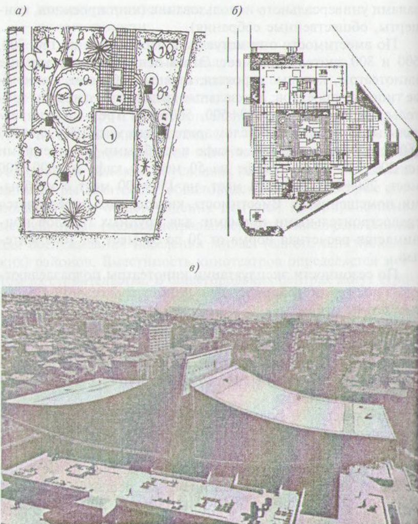
Рис. 14.1.3.1. Примеры организации территорий кинотеатров: а — принципиальная схема: 1 — здание кинотеатра, 2 — реклама, 3 — автостоянка, 4 — разгрузочная площадка перед кинотеатром, 5 — фонтаны и малые архитектурные формы, 6 — декоративные водосмы, 7 — хозяйственная зона, 8 — эвакуация; б — генеральный план кинотеатра «Россия» в Ереване и в — его общий вид
