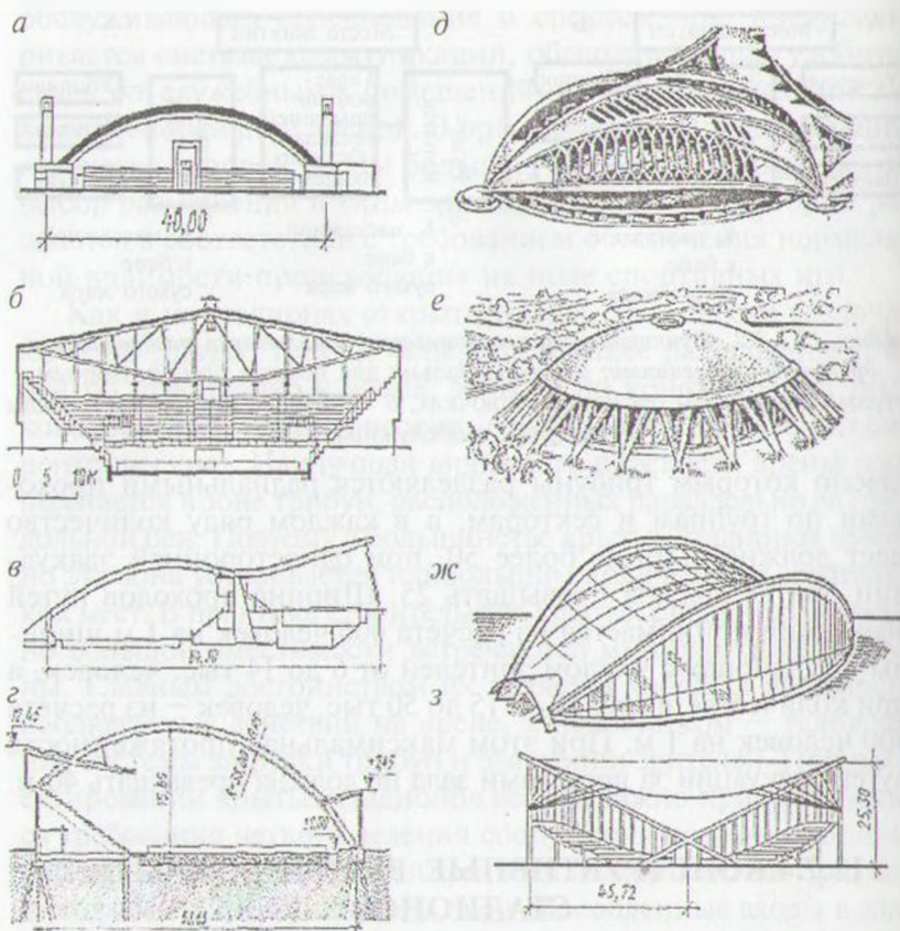
Рис. 12.7.4.1. Примеры конструктивных и архитектурных решений крытых спортивных комплексов: а — спортивный зал в Амерсфорде (Нидерланды), деревянные арки, б — зал с хоккейной ареной в г. Оуду (Финляндия), деревоклеянные конструкции, растяжка ферм из круглой стали, в — спортивный комплекс с хоккейной ареной и бассейном в г. Реймсе, деревоклеянная балка, г — крытый каток в Гренобле (Франция), деревоклеянные конструкции, д — спортивно-зрелищный зал в г. Нордфолде (США), сборно-монокрипный сферический купол, е — крытый велодром Олимпийского комплекса в Монреале (Канада), железобетонные конструкции, ж — крытый стадион с хоккейной ареной в Париже, преднапряженная сетка стальных тросов, з — релей-арена в США, перекрестная сетка тросов
