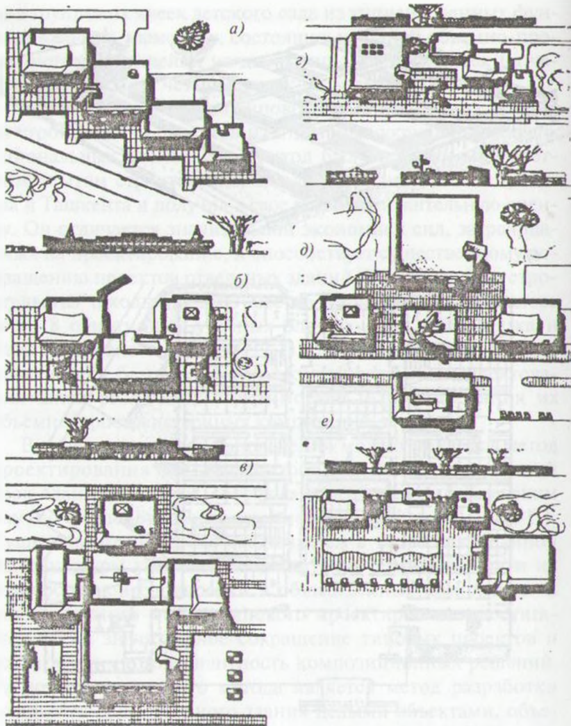
Рис. 7.2. Примеры формирования общественных комплексов системы «Босфор»: а — фронтальное решение с уступами, б — композиция с полукрытым хозяйственным двором, в — композиция с полукрытым хозяйственным двором, г — фронтальное решение с курдонером, д — свободная расстановка блоков, е — угловое решение
