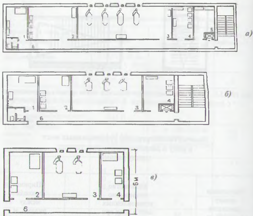
Рис. 14.1.5.7. Схемы планировок кинопроекторных в различных типах кинотеатрах: а — в широкоформатных, б — в обычных, вместимостью 300 мест, в — в кинотеатрах вместимостью до 300 мест; 1 — комната киномеханика, 2 — агрегатная, 3 — кинопроекторная, 4 — перемоточная, 5 — мастерская
