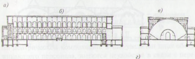
Рис. 15.6.2.3. Крытый рынок в Ереване — центрическая композиция (арх. А. Агабабян): а — общий вид, б — продольный разрез, в — поперечный разрез, г — план рынка
