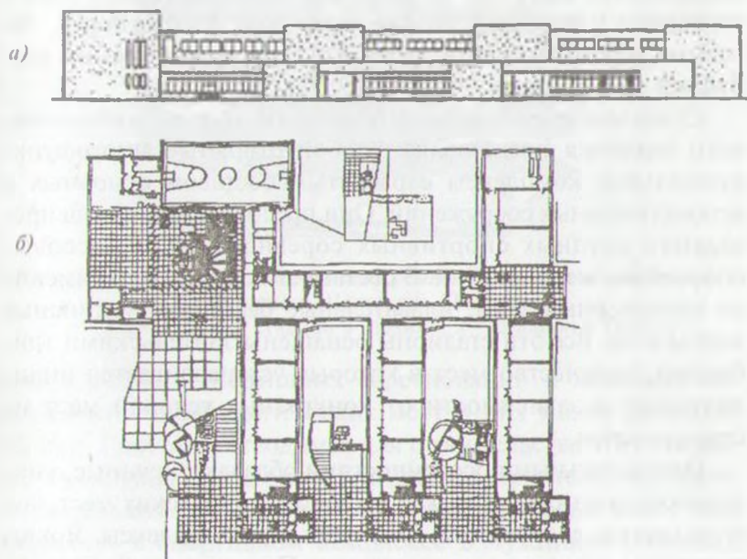
Рис. 12.2.2. Пример размещения гимнастического зала у входной группы школы в целях обслуживания взрослого населения во внеурочное время (типовая школа на 1176 учащихся): а — общий вид, б — план 1-го этажа
