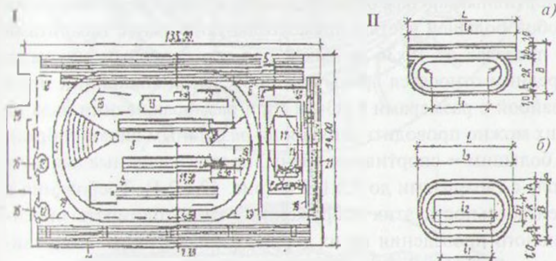
Рис. 12.7.1.4. Примеры организации залов манежей: 1 – план манежа: 1 – прыжки в длину, 2 – прыжки с шестом в длину, 3 – прыжки в длину, 4 – прыжки с шестом, 5 – замкнутая дорожка 200 м, 6 – прямая дорожка 150 м, 7, 8 – толкание ядра, 9 – участок дорожки с виражом, 10, 11 – места для прыжков в высоту, 12 – метание диска и молота, 13 – метание копья, 14, 15 – места для прыжков в длину и тройного, 16 – сетка, 17 – игровые площадки, 18 – футбольное поле, 19 – скамейки, 20 – помещение для гимнастики, 21 – трибуны; II – габаритные схемы основных залов манежей: а – прямая дорожка примыкает к круговой, б – прямая дорожка расположена в пределах внутреннего контура
