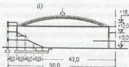
Рис. 5.6. Примеры арочных конструкций: 1: а — пространственная решетчатая арка из алюминиевых сплавов, б — арочные конструкции из стальных элементов; 2: а — арка, б — арка с затяжкой
