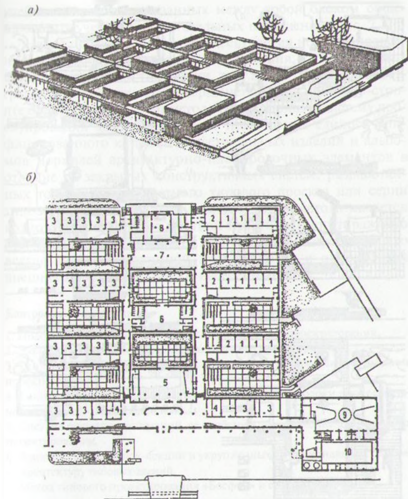
Рис. 7.1. Здание школы на 2600 учащихся в Ташкенте: а — общий вид, б — план 1 этажа: 1 — классы, 2 — комната продленного дня, 3 — кабинеты, лаборатории, мастерские; 4 — учительская, 5 — актовый зал, 6 — малый спортивный зал, 7 — столовая, 8 — кухня, 9 — большой спортивный зал, 10 — плавательный бассейн
