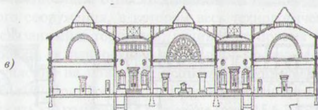
Рис. 15.6.2.4. Приморский рынок в Петербурге — блочная композиция (арх. Д. Хидекель, О. Голынкин): а — общий вид, б — план, в — разрез
