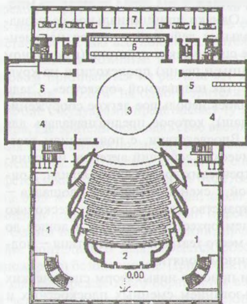
Рис. 14.2.5.1. Организация сценической и зрительской частей театра (на примере Хабаровского музыкально- драматического театра): 1 – фойе, 2 – зрительный зал, 3 – сцена, 4 – карман сцены, 5 – склад объемных и станковых декораций, 6 – аръерсцена, 7 – артистические комнаты
