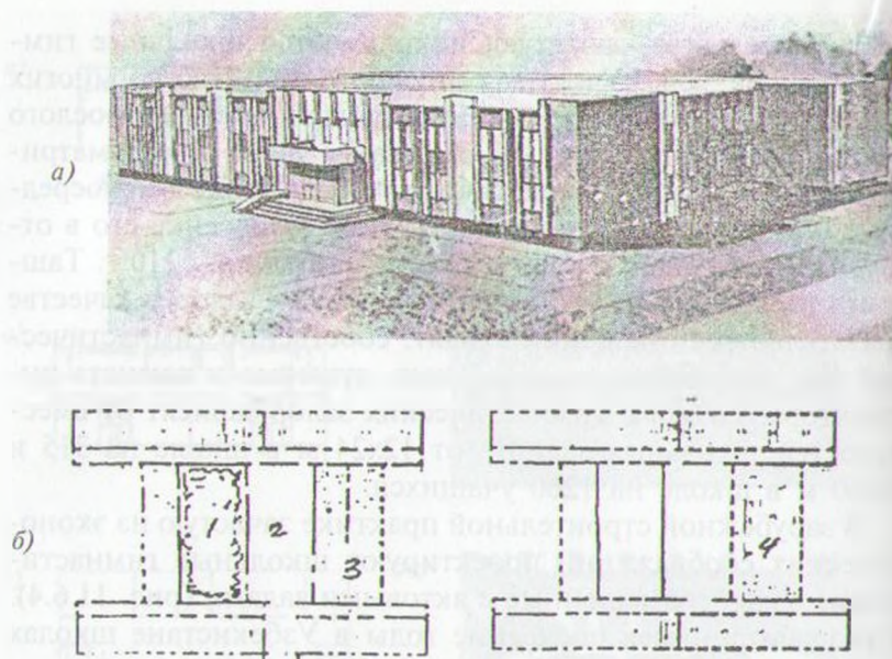
Рис.11.6.5. Прием компактного размещения гимнастического зала с актовым залом и столовой (отечественный опыт): а — общий вид; б — схема: 1 — внутреннее дворовое пространство, 2 — гимнастический зал, 3 — столовая, 4 — актовый зал
