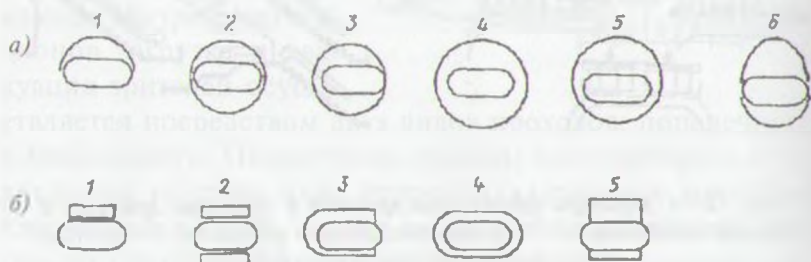
Рис. 12.5.1. Варианты композиционных решений расположения и форм трибун спортивных арен стадионов: а — криволинейные формы с расчетом на обеспечение оптимальных условий видимости, б — упрощенные формы: 1 — односторонние, 2 — двухсторонние (симметричные), 3 — трехсторонние, 4 — четырехсторонние (симметричные), 5 — четырехсторонние (несимметричные), 6 — двухсторонние (несимметричные)
