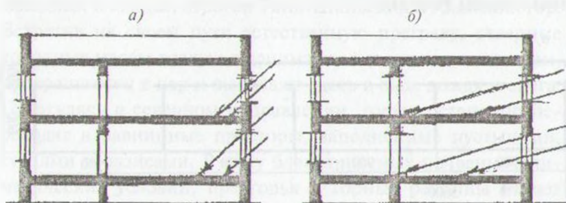
Рис. 3.4. Характер поступления солнечных лучей при ориентации классов по сторонам света: а — юго-зап., юг, юго-вос., б — зап., вос.
