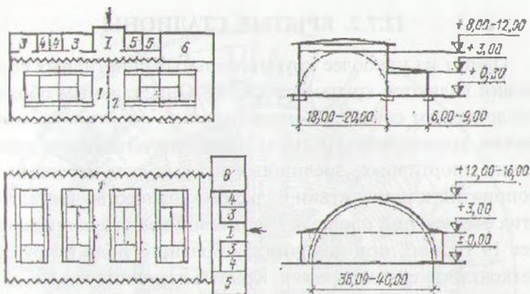
Рис. 12.7.1.3. Варианты объемно-планировочных решений крытых теннисных кортов: 1 — вестибюль, 2 — основной зал, разделительная сетка, 3 — раздевалные с душевыми, 4, 5 — помещения администрации (тренеров, врача)
