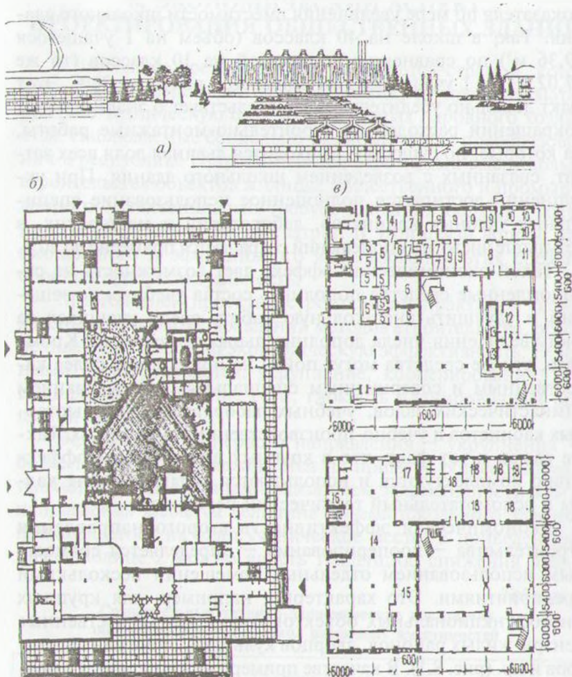
Рис. 8.1. Примеры кооперирования зданий общественного назначения. Планировочные решения общественных центров в поселке Липриндо (Байкало-Амурская магистраль): а — общий вид общественного центра поселка, б — план здания кооперированного общественного центра (автор М. Чернов), в — типовый проект общественного центра для строительства в микрорайоне на 9 тыс. жителей в Узбекистане (автор А. Быков). Планы 1-го и 2-го этажей.
