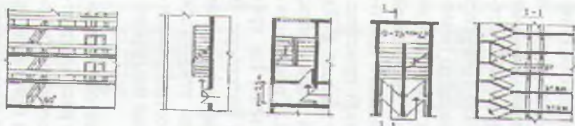
Рис. 9.1.8. Схемы вариантов незадымляемых эвакуационных лестниц
