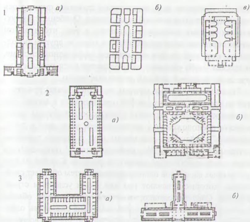
Рис. 15.6.2.6. Схемы планировок одно-, двух- и трехзальных крытых рынков: 1 — однозальные рынки: а — Полюстровский в Петербурге, б — в Ростовс-на-Дону, в — в Милане; 2 — двухзальные рынки: а — центральный рынок в Ереване, б — рынок в Полтаве; 3 — трехзальные рынки: а — центральный рынок в Кишиневе, б — центральный рынок в Казани
