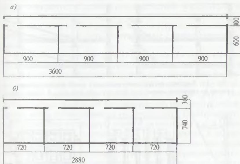
Рис. 3.3. Пример зависимости длины здания от глубины помещений (на примере учебных корпусов школ): а — учебный блок с продольными классами, б — учебный блок с квадратными классами
