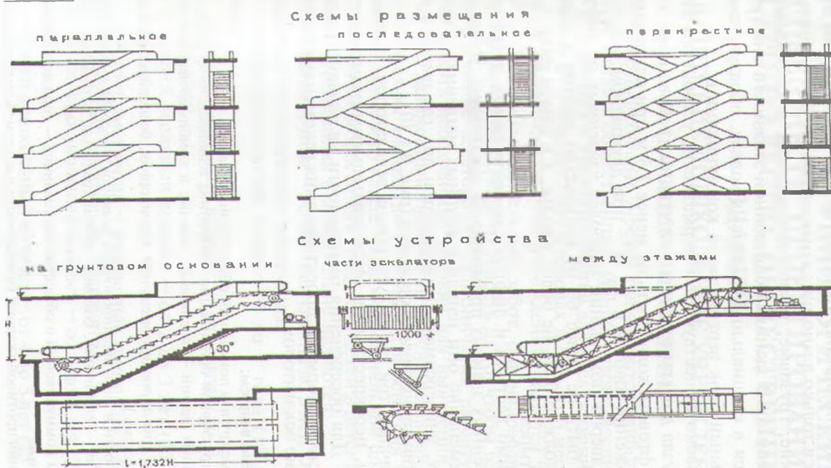
Рис. 9.1.10. Схемы устройств эскалаторов в общественных зданиях
