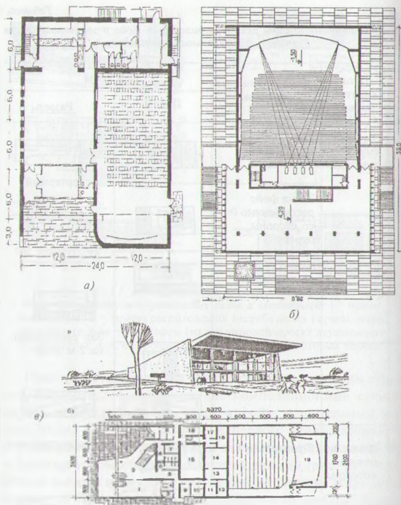
Рис. 14.1.4.2. Приемы планировочных решений однозальных кинотеатров: а — кинотеатр на 300 мест, фронтальное расположение фойе, б — кинотеатр на 500 мест, торiovое расположение фойе; в — кинотеатр на 800 мест в Зеленограде (Россия), фронтальное расположение двухуровневого вестибюля
