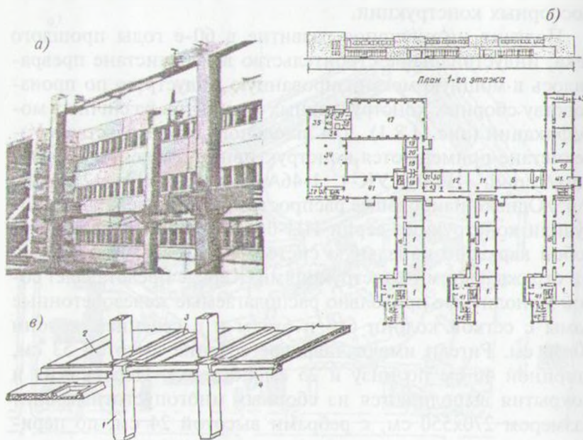
Рис. 11.8.1. Конструктивные системы типовых проектов школ Узбекистана: а — фрагмент конструктивной структуры железобетонного каркаса, б — план 1-го этажа типовой школы, строящейся на основе конструктивной системы ИИС-04, в — каркас серии ИИС-04. Общий вид: 1 — колонна, 2 — панель перекрытия, 3 — связевая панель, 4 — ригель
