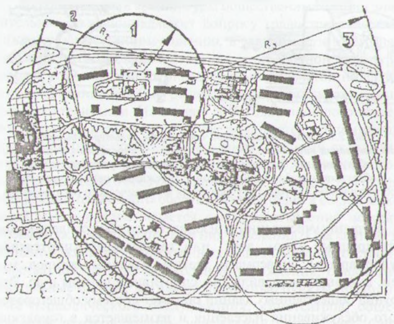
Рис. 2.2. Схема планировки жилого района: 1 — жилая группа с учреждениями первичного обслуживания. R — 150–200 м; 2 — микрорайон с учреждениями повседневного обслуживания. R_1 — 350–700 м; 3 — жилой район с учреждениями периодического обслуживания. R_2 — 1200–1400 м.
