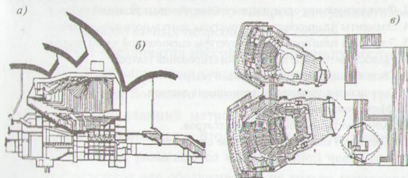
Рис. 14.2.6.4. Культурный центр в Сиднее (Австралия, арх. Г. Уотсон):
