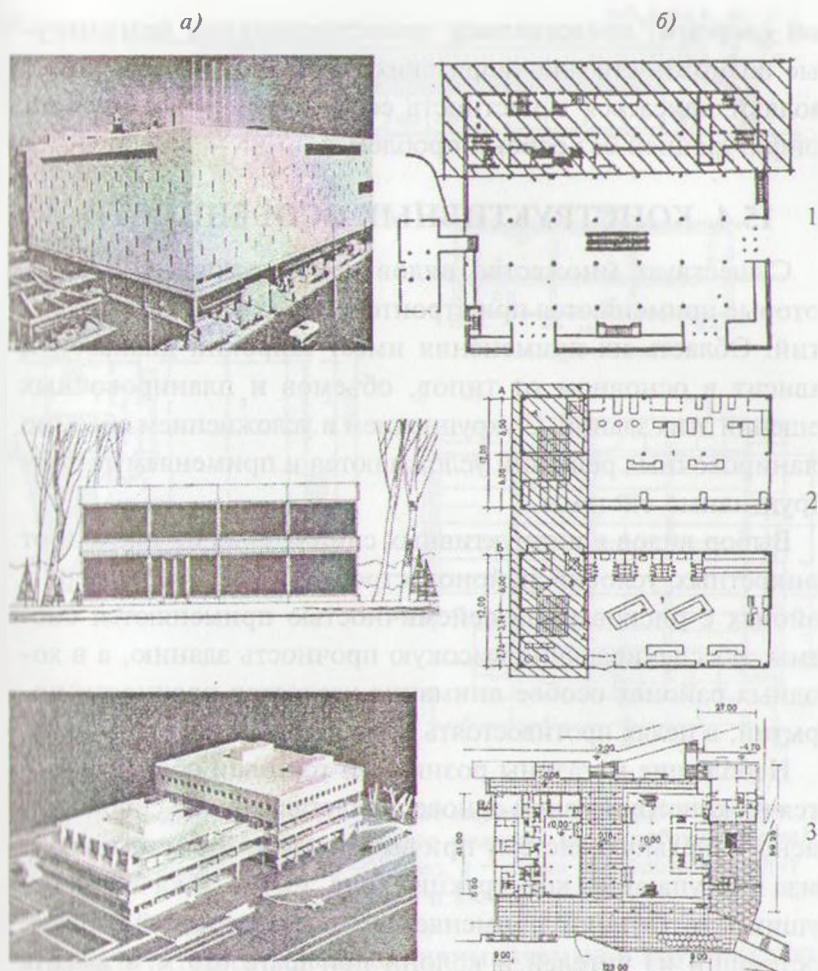
Рис. 15.3.12. Примеры центрических и блочных объемно-пространственных композиций: 1, 2 — центрическая композиция с размещением группы административно-хозяйственных помещений в объеме малого и крупного торгового здания, 3 — блочная композиция торгового комплекса: в четырехэтажном объеме — универмаг с администрацией, в трехэтажном объеме — гастроном, столовая и предприятие бытового обслуживания (заштриховано — помещения административно-технического назначения); а — общий вид, б — планы
