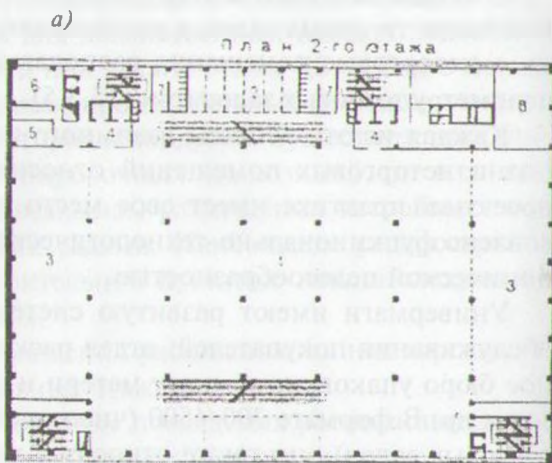
Рис. 15.3.6. Принципиальная схема планировочной модели универсама: а — план второго этажа, б — разрез, в — план подвала
