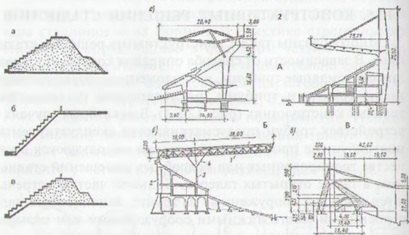
Рис. 12.6.1. Примеры конструктивных решений трибун стадионов:
