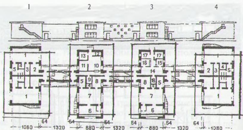
Рис. 4.4. Функциональное зонирование основных и вспомогательных помещений детского сада-яслей: 1, 4 — зоны ясельных групп; 2, 3 — зоны садовских групп и административно-вспомогательных помещений
