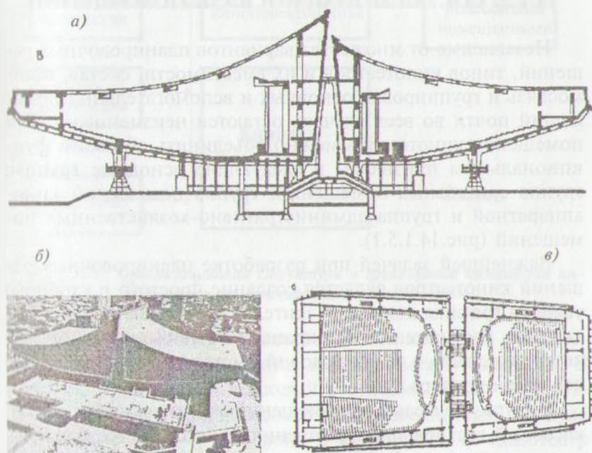
Рис. 14.1.4.4. Кинотеатр «Россия» в г. Ереван. Пример размещения киноаппаратного комплекса между двумя залами: а — разрез, б — общий вид, в — план
