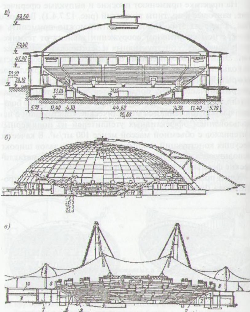
Рис. 12.7.4.3. Примеры большепролетных покрытий: а - Дворцы спорта в Тбилиси, купол - сборные железобетонные элементы, б - крытый стадион в Питсбурге (США), купол - монолитный железобетон (пролет свыше 100 м), в - крытый плавательный бассейн в Мюнхене (пролет свыше 100 м)
