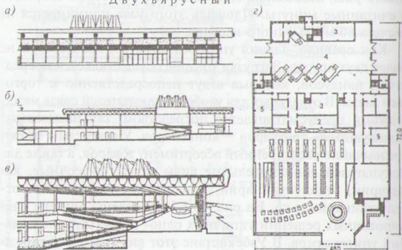
Рис. 15.3.7. Примеры типичных планировочных решений одно- и двухъярусных универсамов: а — общие виды, б — разрезы, в — перспектива, г — планы торговых залов с расположением дебаркадеров
