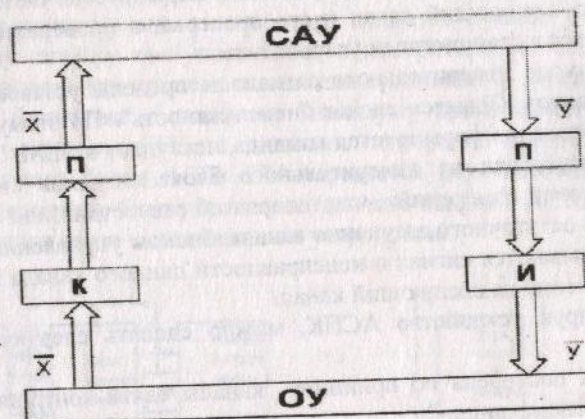
Рис. 4.2. Схема САУ.
