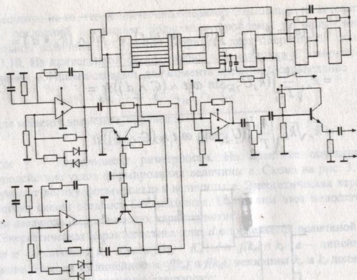
Рис. 3.11. Принципиальная схема передатчика СИОЗ.
