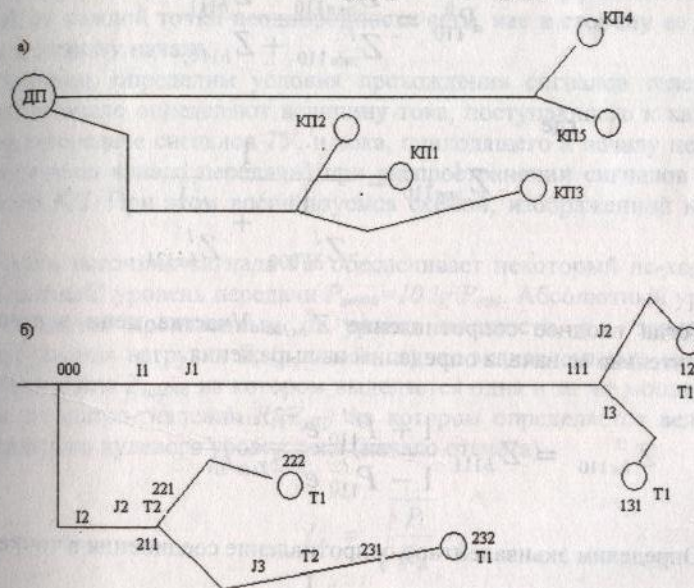
Рис.2.4. а)- схема организации сети ТМ, б)- приведенная схема сети ТМ для математической модели.
