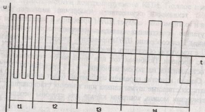
Рис. 2.2.2. Широтно-модулированные сигналы.
