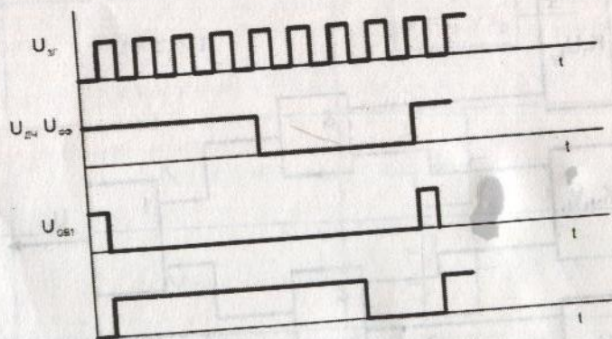
Рис. 3.4. Временные диаграммы работы узлов ГТИ.
