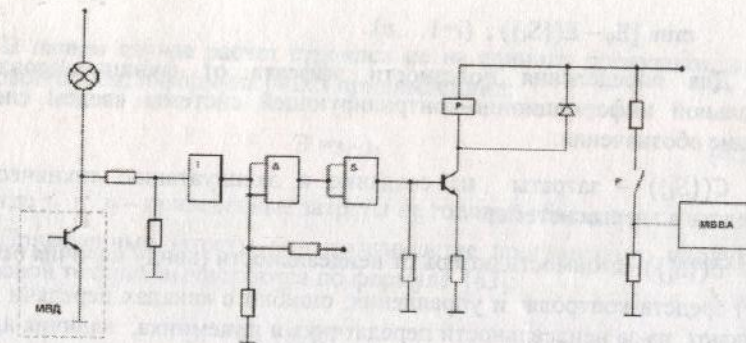
Рис. 4.12. Принципиальная схема блока индикации занятости канала.
