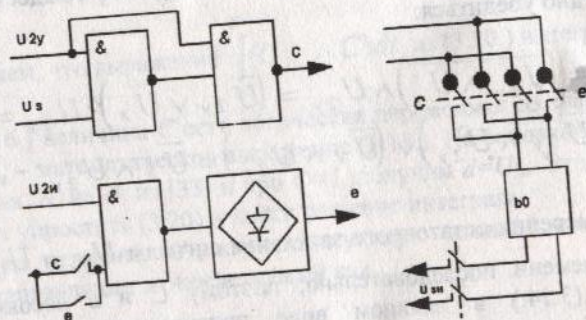
Рис. 3.9. Структурные схемы операторов, формирующих величину C(a) , величину e(б) и величину U_{2u}(в) .
