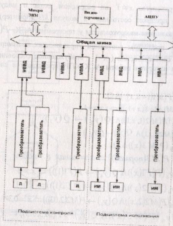
Рис. 7.4. Структурная схема АСУ.
