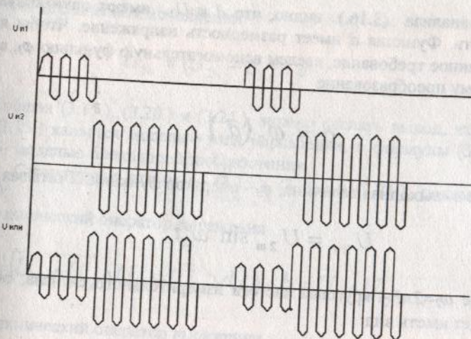
Рис. 3.8. Временные диаграммы работы передатчика.
