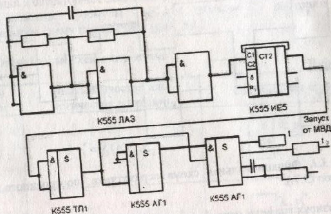
Рис. 3.3. Принципиальная схема блока ГТИ.
