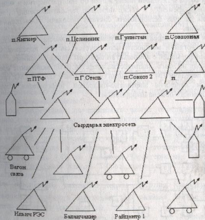
Рис. 1.5. Кустовая радиосеть Сырдарьинской электросети.
