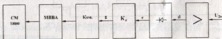
Рис. 4.8. Структурная схема приемной части АСК.
