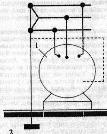
12-расм. Асбобни «ноль» рақамли сим орқали ерга улаш ҳимоя воситаси схемаси.
