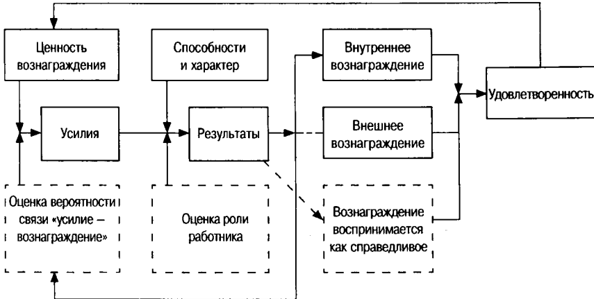
Рис. 8.3. Модель Портера—Лоулера
