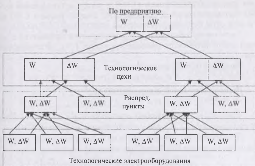
Рис. 2.2. Структурная схема формирования расчетных данных энергобаланса объекта энергосистемы.
