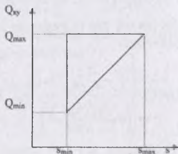
Рис. 3.9 Граничные значения регулируемых параметров СЭС.
