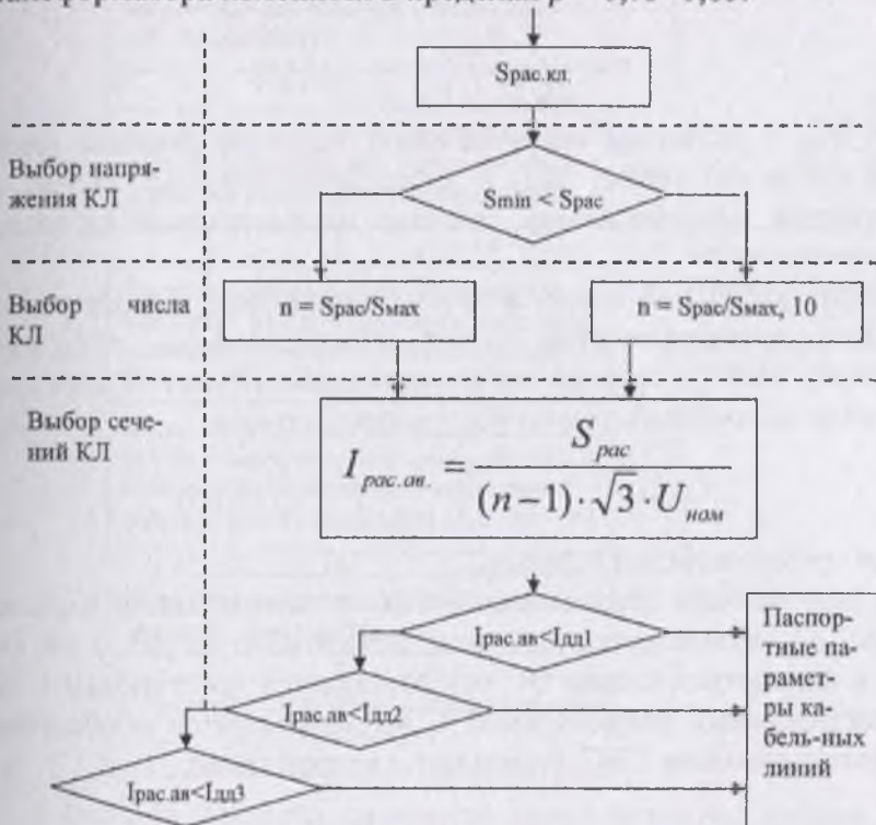
Рис. 4.15. Алгоритм выбора кабельных линий.
