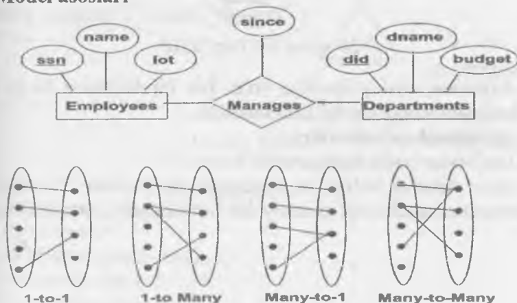
2.5-rasm ER modeli bazasidagi sxema
