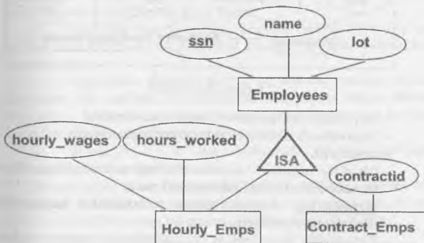
2.8-rasm ER to'plam
