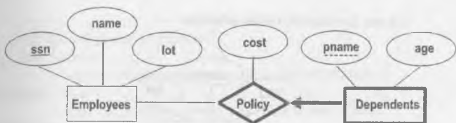
2.7-rasm ER obyekt
