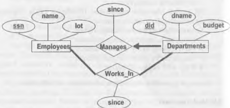
2.6-rasm ER bog'lanish
