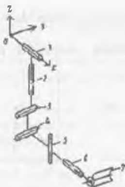
2.2 – rasm. Robot qo‘li mexanizmining sxemasi: 1,2,3-regional harakatlari; 4,5,6- orienterlash harakatlari; 7- ishchi organ;
