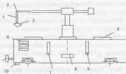
9.3-rasm. MP-12t robokarasida tashqi informatsiya datchiklarining joylashtirilishi:
