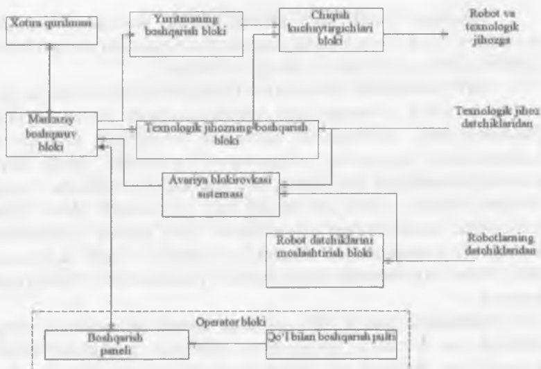
4.5- rasmi. Unifikatsiyalangan sikli boshqarish qurilmasi USM-663 ning struktura sxemasi.
