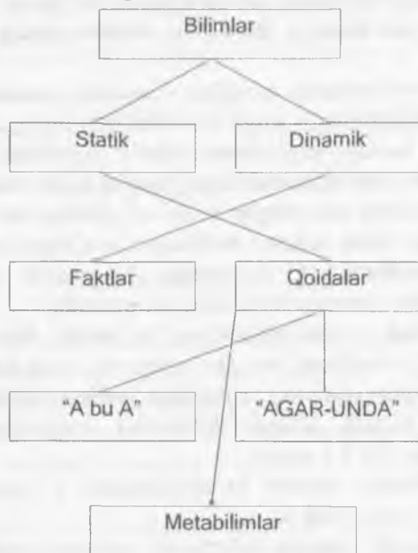
13.2-rasm. Intellektual tizimdagi bilimlarning sinflanishi.
