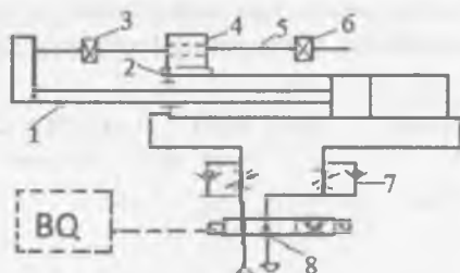
3.2 – rasm. Sanoat roboti pnevmoyuritmasining sxemasi:
