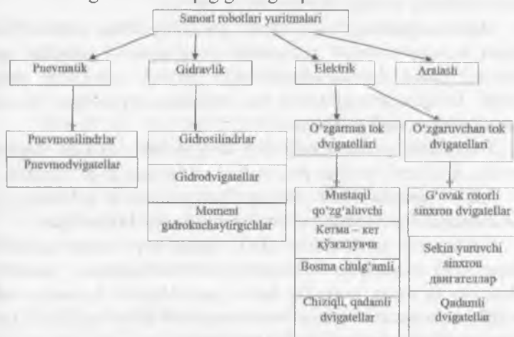
3.1 – rasm. Sanoat robotlari yuritmalarining sinflanishi.
