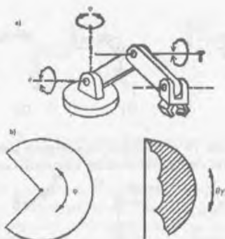
2.7 rasm. Burchak koordinatalar sistemasida ishlovchi robot va uning ishchi zonasi: a) robotning konstruktiv sxemasi, b) ishchi zonasi
