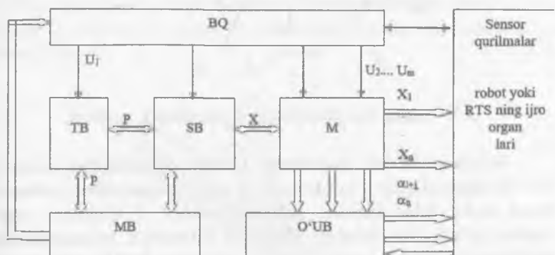
3.6 – rasm. Ko'pkoordinatali yuritmaning umumlashgan struktura sxemasi.
