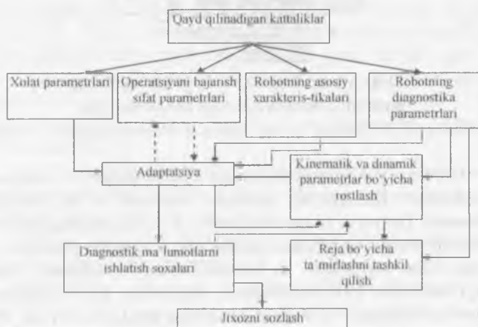
12.5. - rasm. Robotning nazorat qilinadigan asosiy parametrlarining strukturasi.
