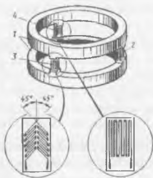
10.6- rasm. Kuch va moment datchigi:
