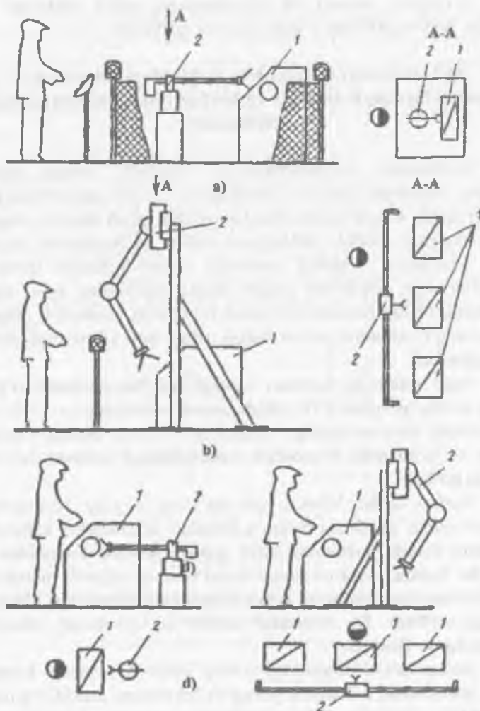
14.1- rasm. RTK ning rejalashtirilishi: 1- texnologik jihoz, 2- sanoat roboti.
