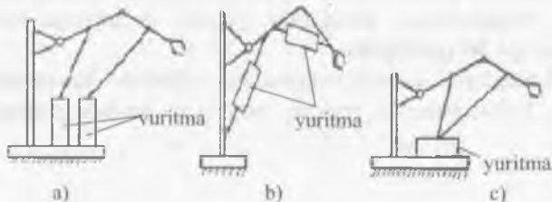
2.12 – rasm. Yuritma qurilmalarini joylashtirish usullari.
