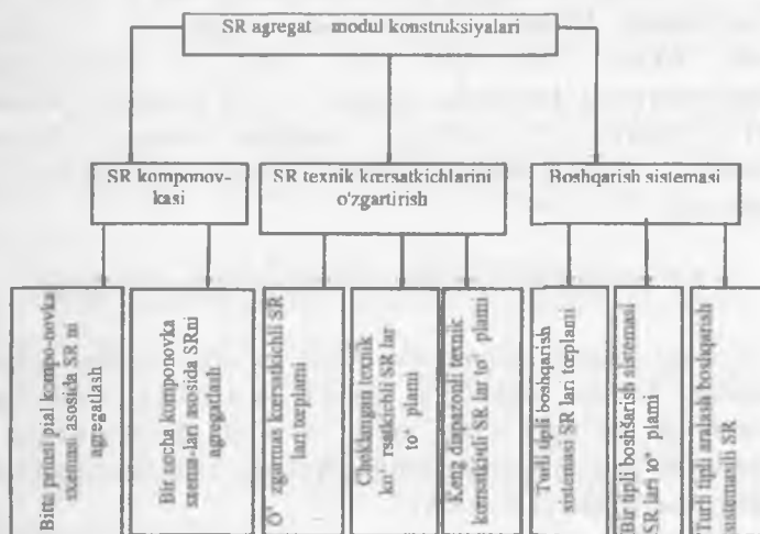
1.6 – rasm. Sanoat robotlarini agregat – modul qurishning struktura sxemasi.
