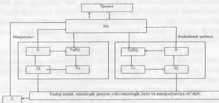
1.2 – rasm. Sanoat robotining struktura sxemasi:
