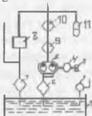
3.4 – rasm. Sanoat roboti gidrostansiyasining funksional sxemasi
