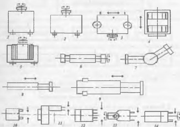
1.7 – rasm. Robot manipulyatorining unifikatsiyalangan modullari:
