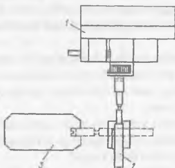
11.3- rasm Bir pozitsiyali robototexnik kompleks: 1-tokar dastgohi; 2-sanoat roboti; 3-gorizontaal magazin to'plagich.
