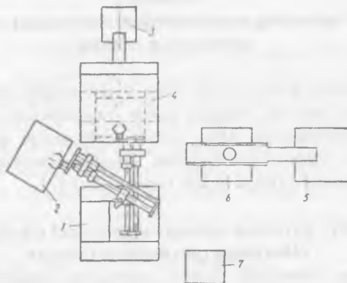
11.1- rasm. Pressga xizmat qiluvchi robot asosidagi robototexnik kompleks
