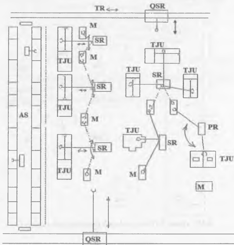
6.14 - rasm. Robotlashtirilgan texnologik kompleksning chiziqli aylanali joylashtirish sxemasi.
