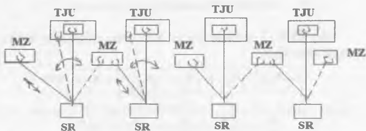
6.11 - rasm. RTK ning chiziqli joylashtirish sxemasi: MZ-xom mahsulotni donalab berib turuvchi magazin.
