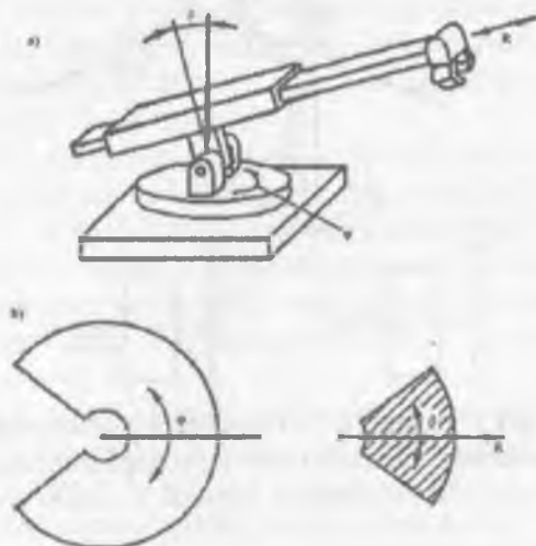
2.6 –rasm. Sferik koordinatalar sistemasidagi robot va uning ishchi zonasi: a) robotning konstruktiv sxemasi, b) ishchi zonasi
