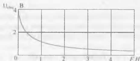
10.3- rasm. Elastomer taktill sensorning chiqish xarakteristikalari.
