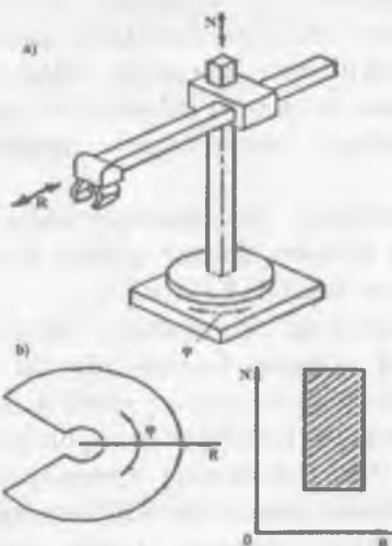
2.5 rasm. Silindrik koordinatalar sistemasida ishlovchi robot va uning ishchi zonasi: a) robotning konstruktiv sxemasi, b) ishchi zonasi
