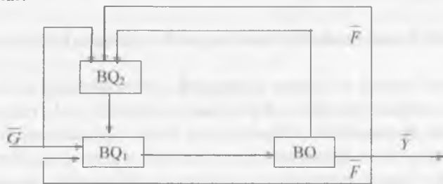
4.2-rasm. Sanoat robotini adaptiv boshqarishning funksional sxemasi.
