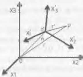
2.13-rasm. Manipulyator koordinat tizimi.
