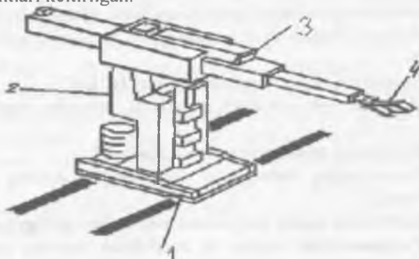
2.1 – rasm. Sanoat roboti konstruksiyasining asosiy elementlari:
