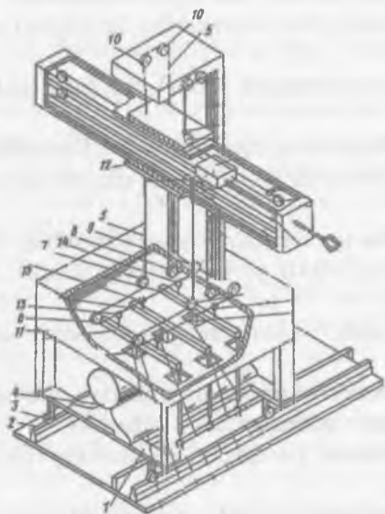
3.8- rasm. Ko'p koordinatali yuritmal sanoat robotining konstruktiv sxemasi:
