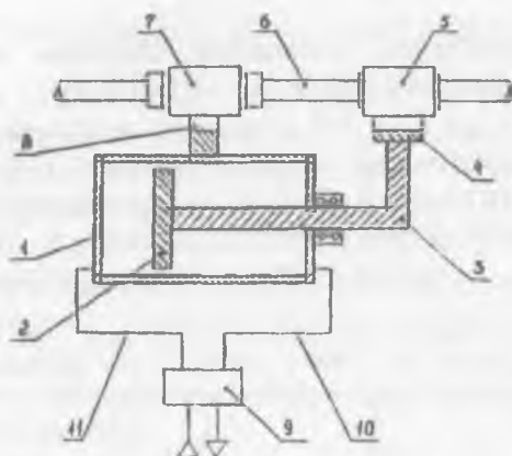
3.7 – rasm. Ko'pkoordinatali pnevmatik yuritma.
