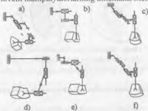
2.9– rasm. Silindrik koordinatalar sistemasidagi kinematik sxemalar:
