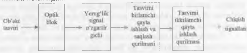
10.4- rasm. Texnik ko'rish tizimining struktura sxemasi.
