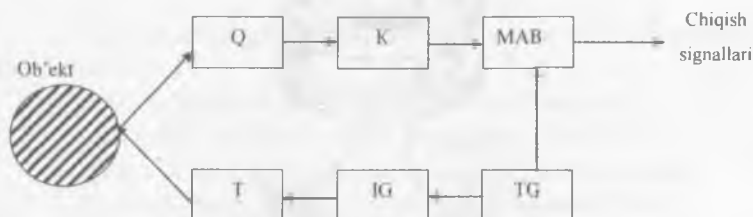
10.5- rasm. Lokatsion datchikning struktura sxemasi: Q- qabul qiluvchi qurilma; K- kuchaytirgich; MAB- masofani aniqlash blogi; T- to'lqin tarqatuvchi qurilma; IG- impuls generatori; TG- tayanch generatori.
