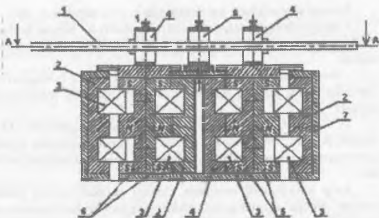
15.4-rasm. Bir-biriga bog'liq bo'lmagan uchta chiziqli ko'p koordinatali KMHMning konstruksiyasi:
