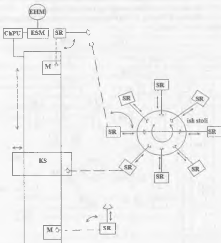
6.15 - rasm. RTKning aylanali joylashtirish sxemasi.
