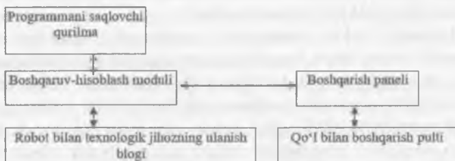
4.4- rasm. Siklli boshqarish tizimining umumiy tarkibi
