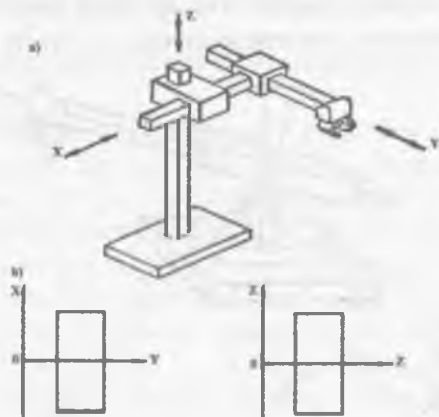
2.4 – rasm. To'g'ri burchak koordinatalar sistemasida ishlovchi robot va uning ishchi zonasi: a) robotning konstruktiv sxemasi, b) ishchi zonasi
