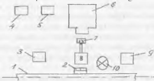
8.3- rasm. Sonli programmali boshqariladigan robototexnik bo'linmalarining struktura sxemasi:
