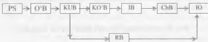
4.7 - rasm. Sanoat roboti kontur boshqarish qurilmasining struktura sxemasi:
