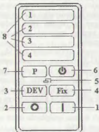
4.5-rasm. Protsessorning boshqaruv pulti.
