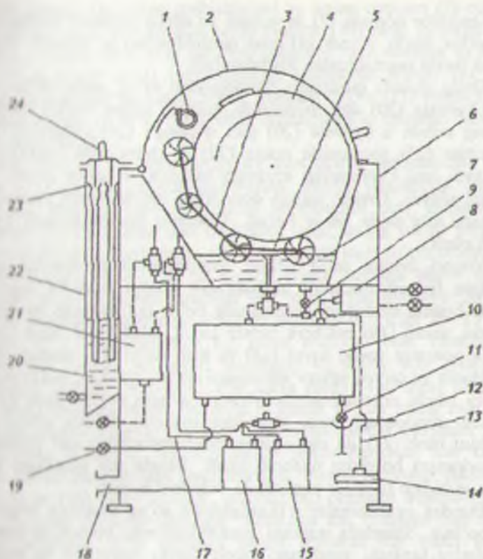
6.10-msm. Yuqori va fleksograf bosish usulidagi FBQga ishlov berish protsessorlar.
