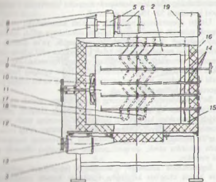
6.21-rasm. Fotopolimer qoliplarni quritish uskunasi- ning prinsipul sxemasi.
