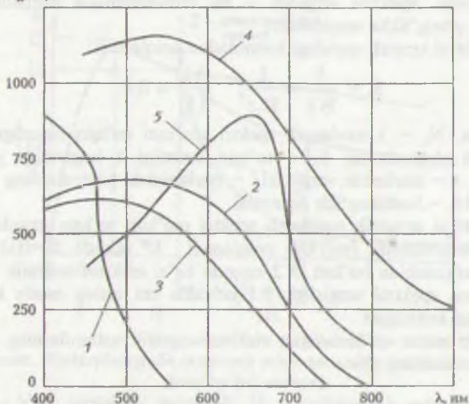
8.2-rasm. Ko'p marta qo'llanadigan EFQning spektral sezgirliigi: S_{\lambda} – fotosezgirlik; \lambda – to'liqin uzunligi; 1 – Se, 2 – Se-Te; 3 – \text{As}_2\text{Se}_3 ; 4 – ko'p komponentli tuzilmalar; 5 – amorf kremniy.
