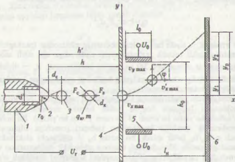
8.26-rasm. Uzlüksiz oqimli bosmada zaryadlangan tomchining siljishini hisoblash sxemasi:
