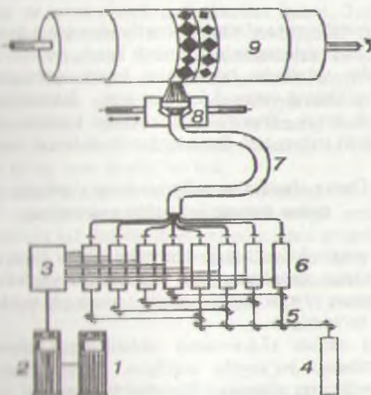
1.5-mm. Linotronic 830, 930 fotonabor avtomatlarning skanerlash qurilmasining sxemasi.
