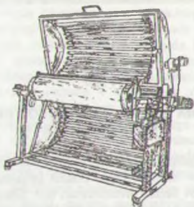
5.12-rasm. Ochiladigan nurlantiruvchi moslamali eksponirlovchi qurilma.
