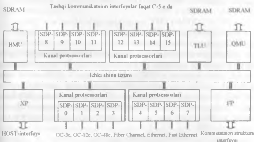
3.14-chizma. C-port turkumidagi tarmoq protsessorlarining umumlashtirilgan strukturasi
