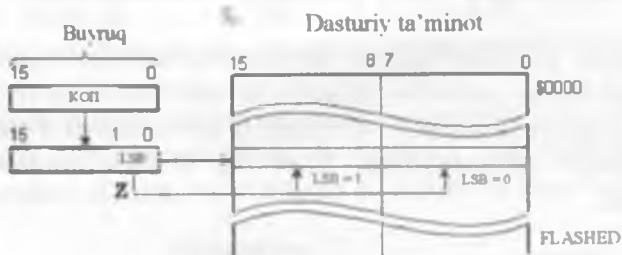
4.30-chizma. Konstantani adreslash
