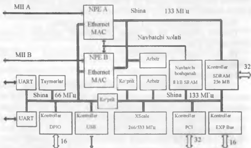
3.10-chizma. IXP420 protsessor arxitekturasini
