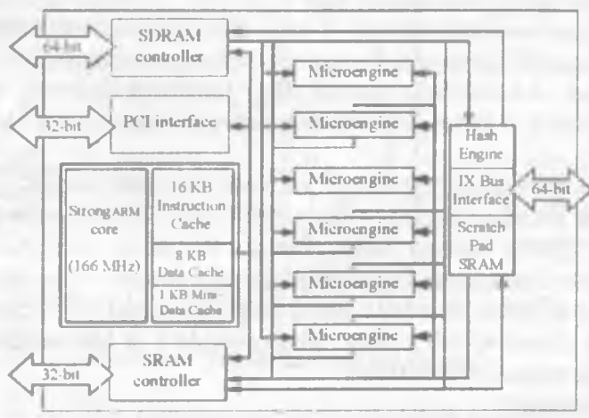
3.5-chizma. IXP1200 mikroprotssessor blok-sxemasi
