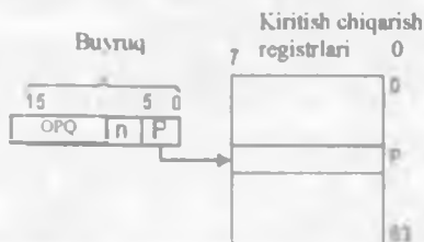
4.21-chizma. Kiritish-chiqarish registrini to'g'ridan-to'g'ri registrli adreslash
