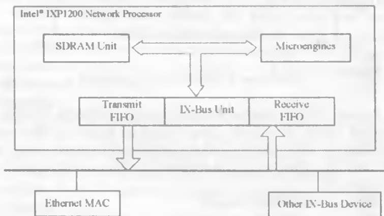
3.7-chizma. IX shinasi ma'lumotlar shinasi
