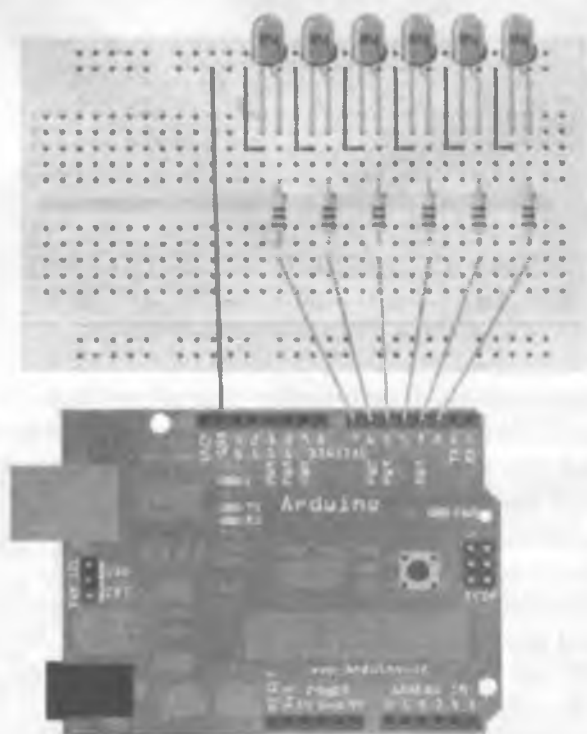
5.5-rasm. Arduino ga ulangan qurilmalarni boshqarish
