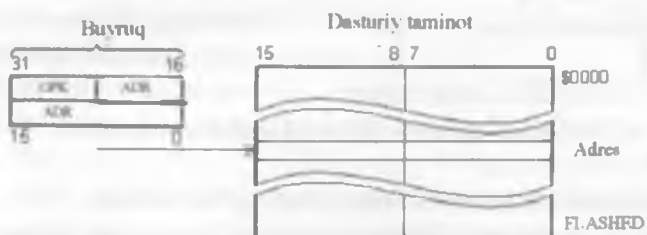
4.27-chizma. Dastur xotirasini bevosita adreslash
