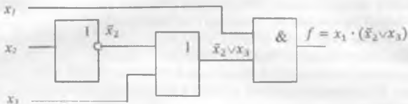
1.7-chizma. f = x_1 \cdot (x_2 \vee x_3) funksiyaning kombinatsion sxemasi
