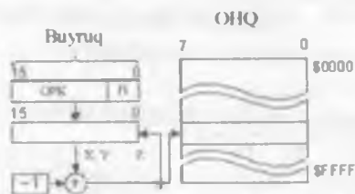
4.25-chizma. Ma'lumotlar operativ xotirasini qisman predekrementli adreslash
