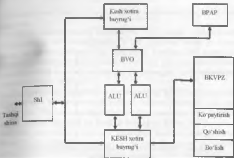
2.5-chizma. Pentium mikroprotssessorining umumlashgan struktura sxemasi
