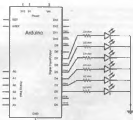
5.43-chizma. Arduino ga ulangan qurilmalarni boshqarish prinsipial sxemasi
