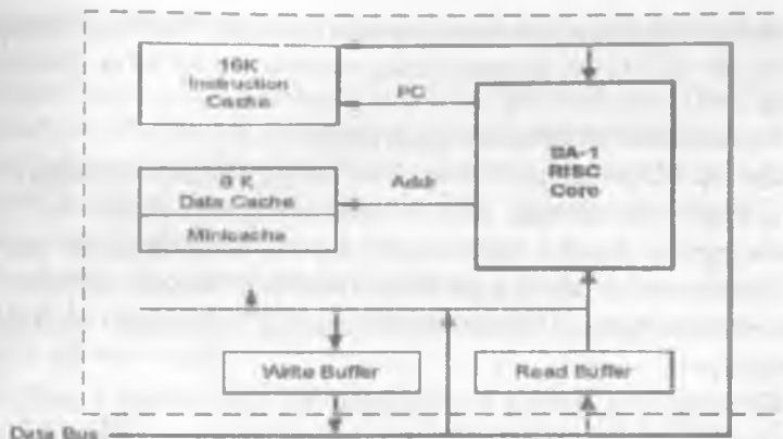
3.4-chizma. StrongARM mikroprotssessor blok-sxemasi
