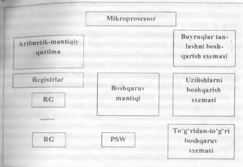
2.4-chizma. Oddiy MP ning tuzilishi
