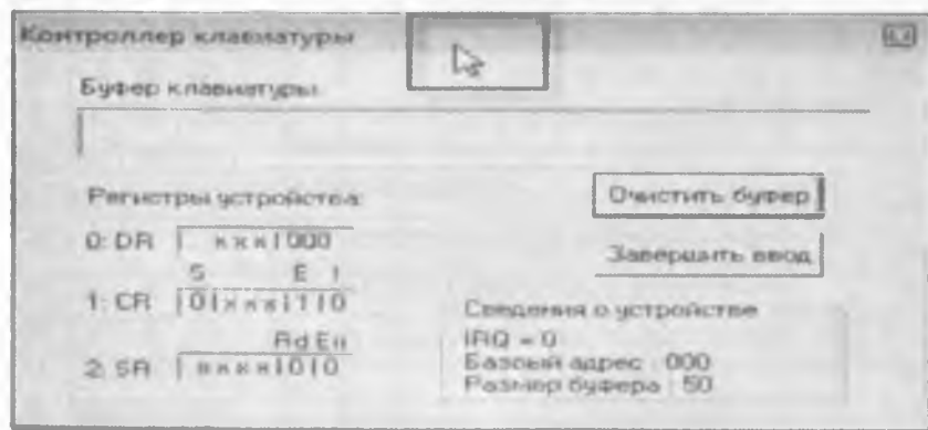
5.14-chizma. Klaviatura kontroller sharhlovchisi
