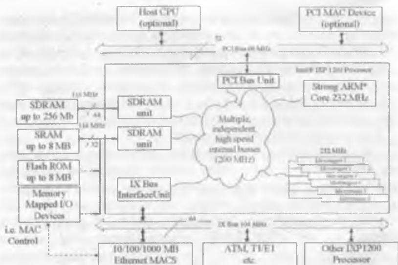
3.3-chizma. IXP1200 protsessori blok-sxemasi
