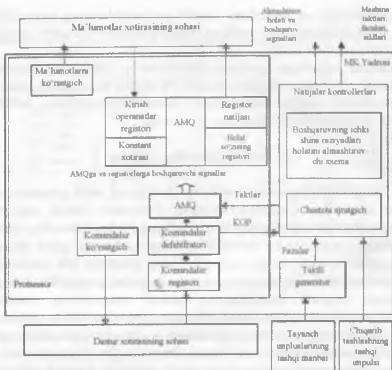
4.4-chizma. Mikrokontroller yadrosining tuzilmaaviy sxemasi
