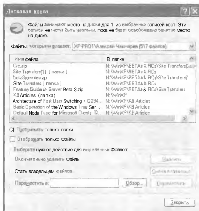
Рис. 3.6. В этом окне перечисляются все файлы (вместе с их точным местоположением), принадлежащие выбранному пользователю на указанном томе с включенным квотированием
