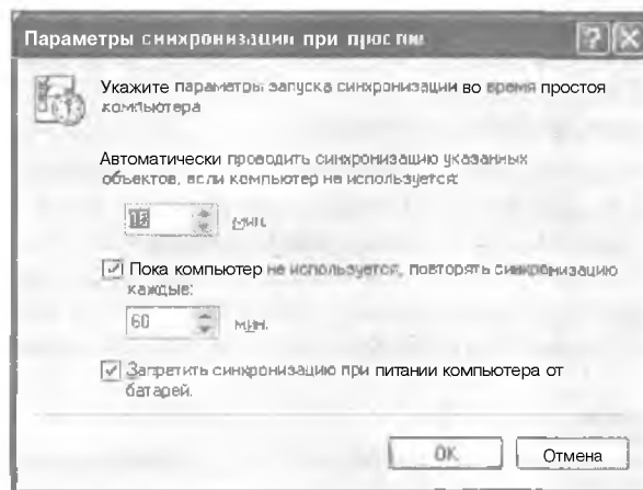
Рис. 9.32. Окно установки параметров синхронизации во время бездействия компьютера
