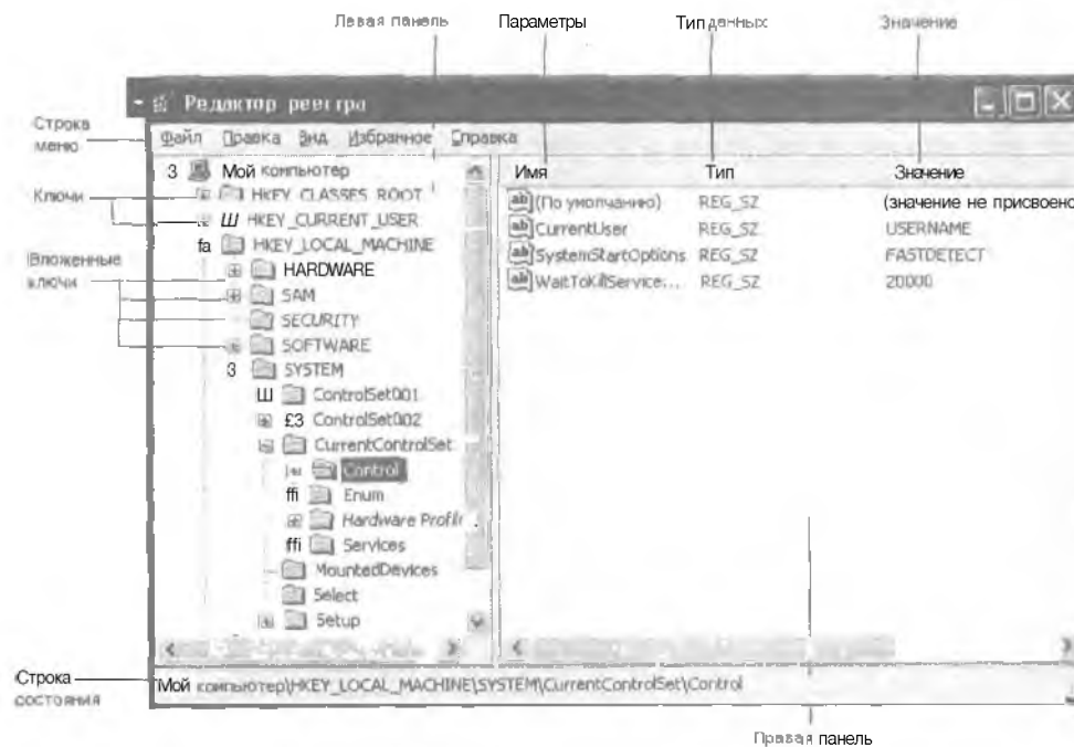
Рис. 16.3. Окно редактора реестра Regedit.exe с обозначением основных областей
