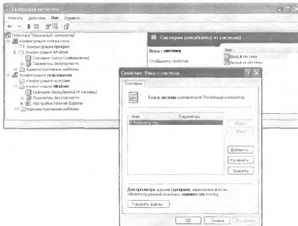
Рис. 10.12. Назначение пользователям сценария схода
