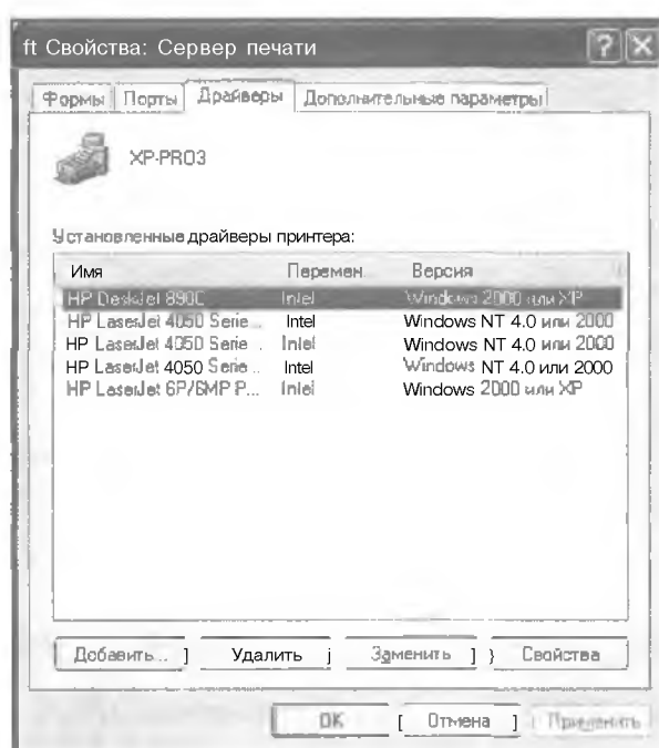
Рис. 7.9. Настройка драйверов принтера для различных платформ
