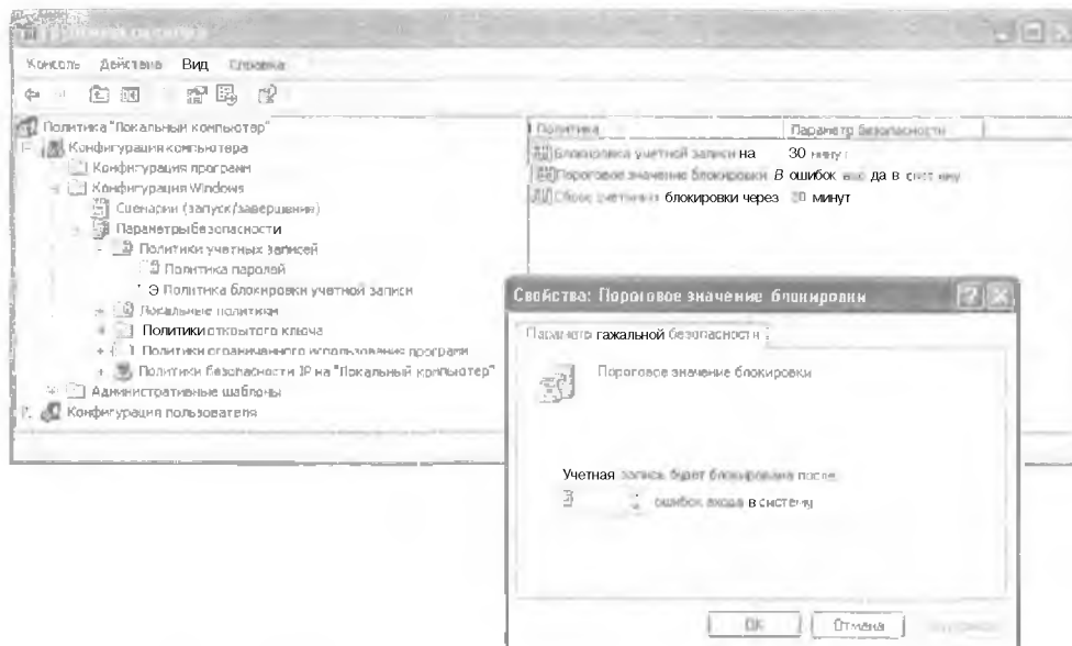
Рис. 10.11. Настройка политики блокировки учетных записей
