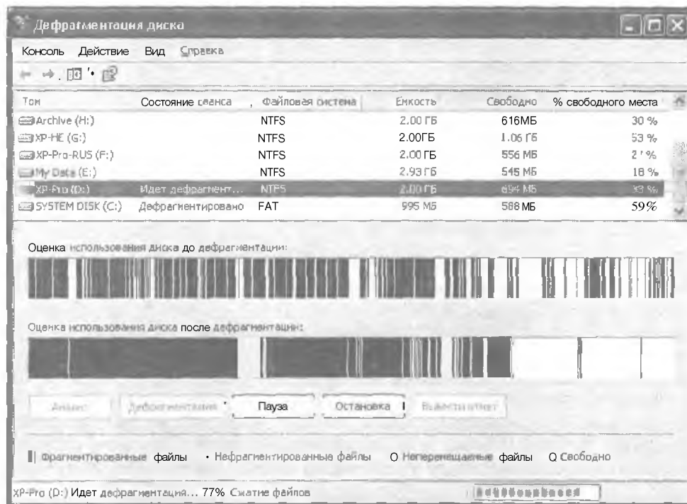
Рис. 3.8. Окно оснастки Дефрагментация диска
