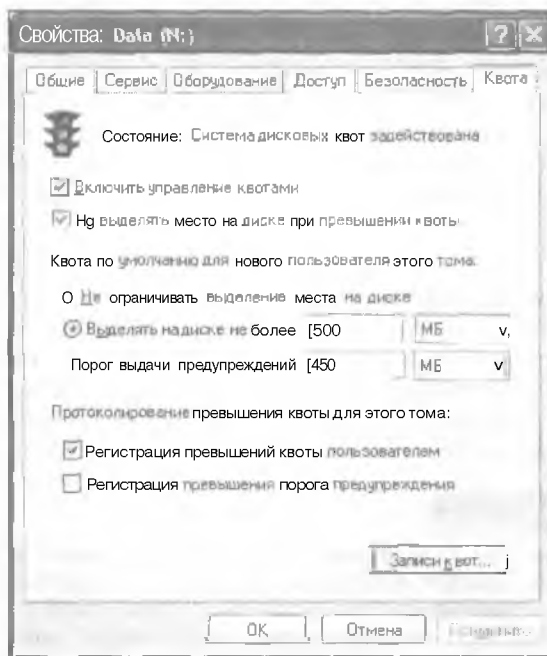
Рис. 3.1. Вкладка Квота окна свойств дискового тома
