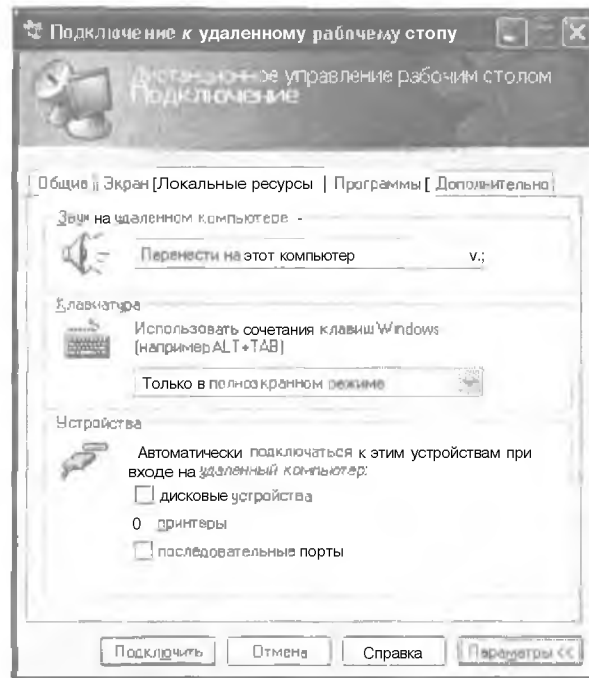
Рис. 9.11. Вкладка, управляющая переназначением локальных устройств
