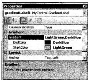
Рис. 8.5. Свойство GradientParameters состоит из двух полей
