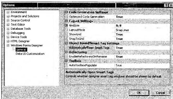
Рис. 7.3. Диалог параметров дизайнера
