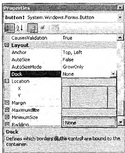
Рис. 2.15. Редактор привязки (свойство Dock)
