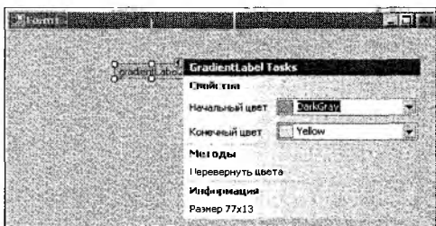
Рис. 6.6. Новый тег компонента GradientLabel (с группировкой)
