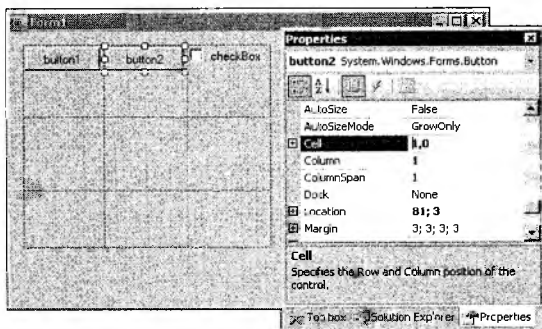
Рис. 12.1. Свойства Cell, Column, ColumnSpan, Row и RowSpan добавляются ко всем компонентам, расположенным на TableLayoutPanel
