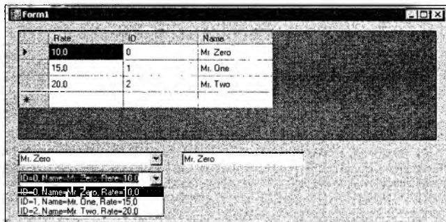
Рис. 13.4. Привязка данных: GridView , ComboBox и TextBox
