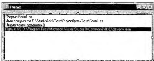
Рис. 7.5. Получение информации о проекте
