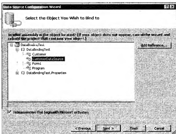
Рис. 13.9. Класс CustomerDataSource как источник данных
