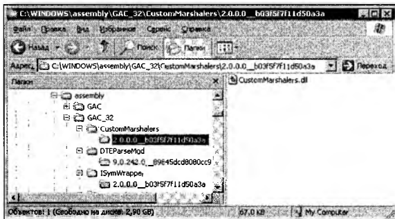
Рис. 14.2. Физическое расположение GAC
