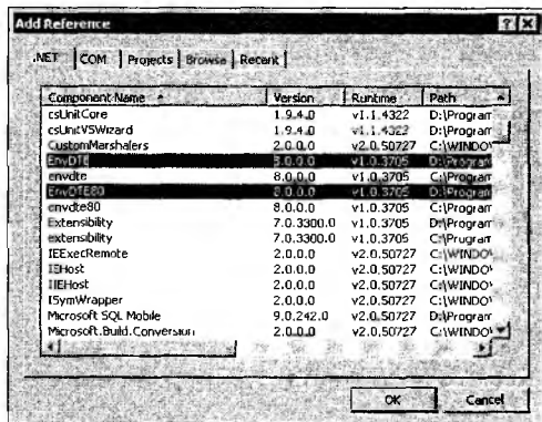
Рис. 7.6. Добавление ссылок на библиотеки EnvDTE и EnvDTE80
