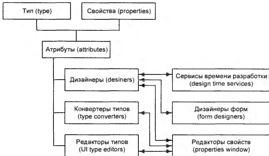
Рис. 4.1. Архитектура времени разработки
