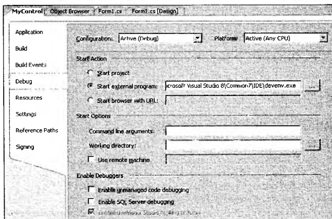
Рис. 4.5. Вкладка Debug в свойствах проекта
