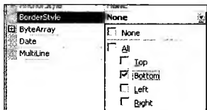
Рис. 9.5. Редактор BorderSidesEditor
