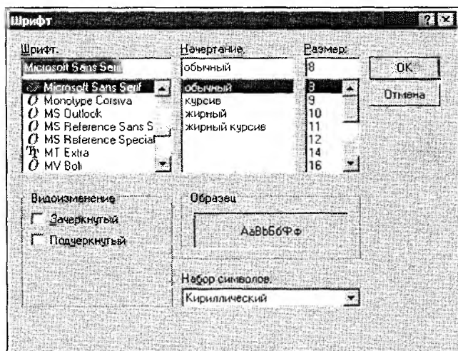
Рис. 2.13. Редактор шрифта
