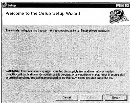
Рис. 14.17. Установка компонента
