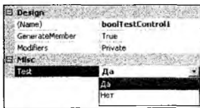
Рис. 8.2. Работа BooleanConverter
