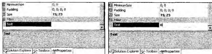
Рис. 12.3. Generic-свойство
