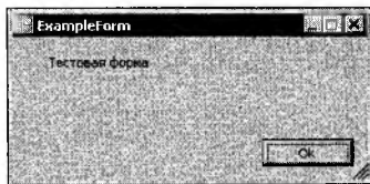
Рис. 7.11. Вывод формы
