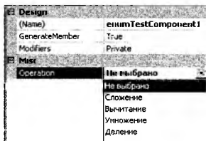
Рис. 8.3. Работа EnumConverter
