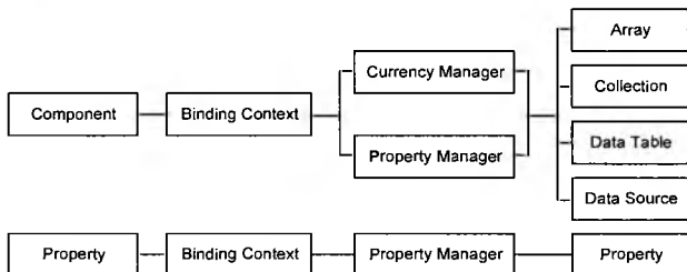
Рис. 13.2. Модель привязки данных
