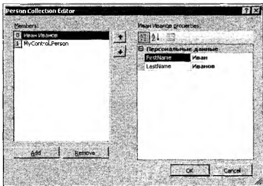
Рис. 9.14. Редактор коллекции объектов Person
