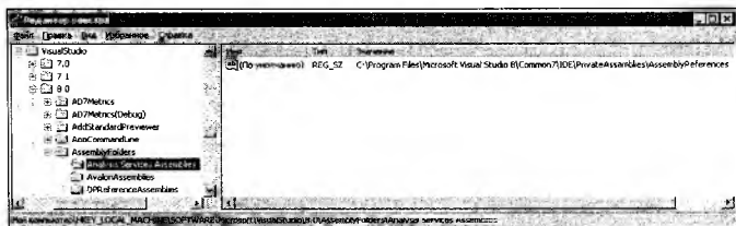
Рис. 14.1. Ключ AssemblyFolders описывает дополнительные каталоги для поиска сборок
