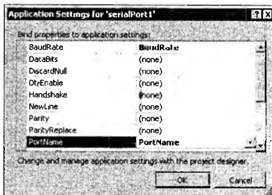
Рис. 10.7. Редактор свойства (PropertyBinding)
