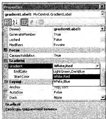
Рис. 8.6. Стандартный набор для свойства GradientParameters
