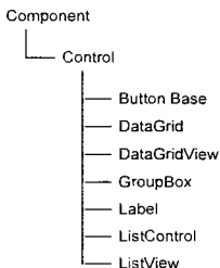
Рис. 4.4. Иерархия классов
