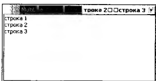
Рис. 9.3. Редактор MultilineStringEditor
