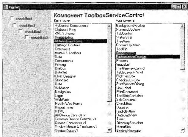
Рис. 7.8. Компонент ToolboxServiceControl
