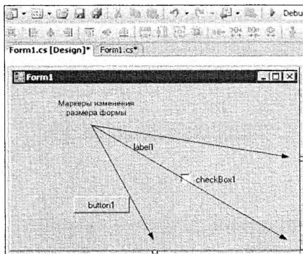
Рис. 2.2. Редактор формы
