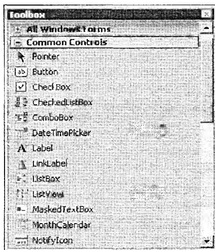
Рис. 2.7. Окно Toolbox
