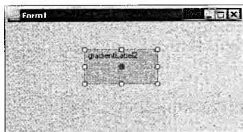
Рис. 6.11. Маркер Zoom
