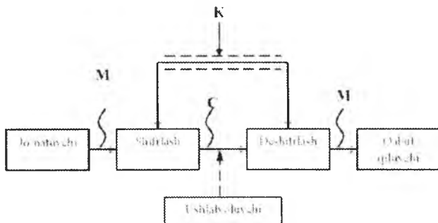
21.1-rasm. Umumlashma kriptotizim sxemasi
