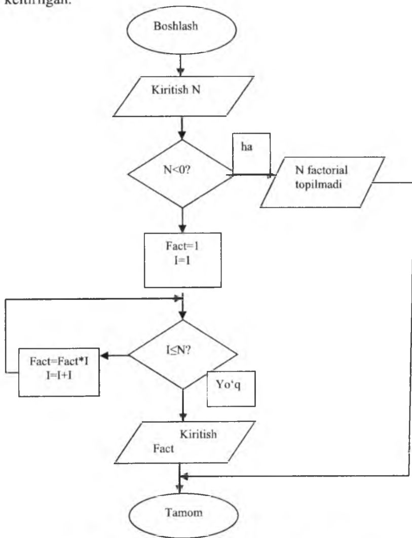
11.11-rasm. Sonlarni faktorialini aniqlash algoritmi 43 .
