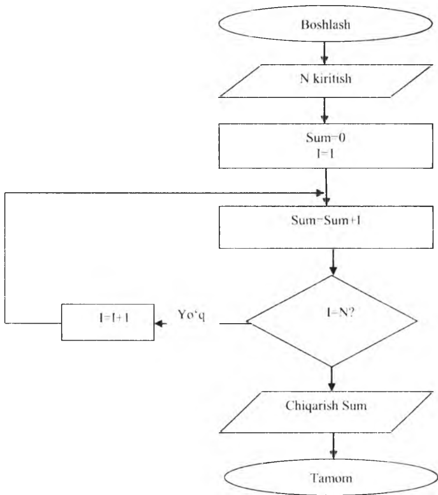
11.10-N sonlar yig'indisini topish algoritmi
