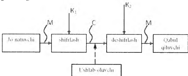
21.2-rasm. Ochiq kalitli asimmetrik kriptotizimning umumlashma sxemasi
