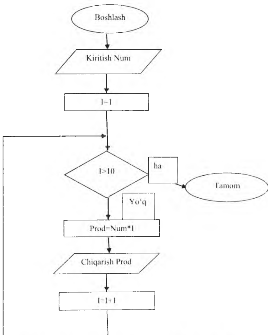
11.9-rasm. Sonlarni ko'paytirish jadvalini chiqarish algoritmi
