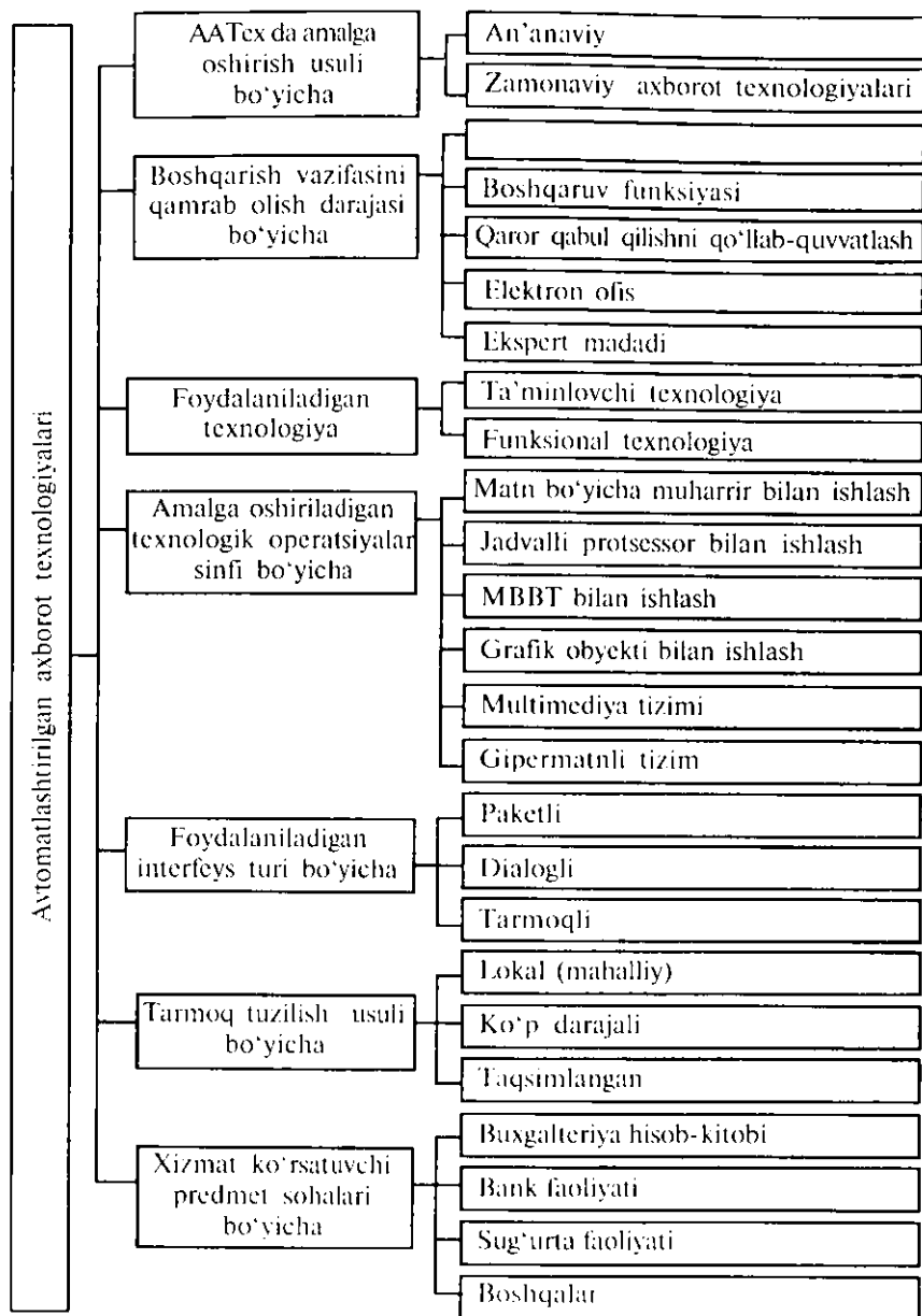
2.3-rasm. Avtomatlashtirilgan axborot texnologiyalari tasnifi.
