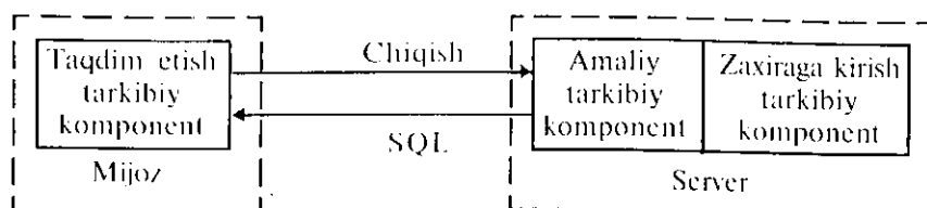
10.5-rasm. Ma'lumotlar bazasining serverli modeli.
