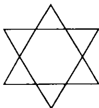
Oddiy fraktal „uchburchagi“
