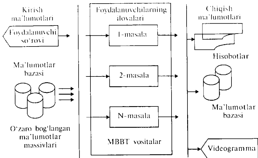
6.5-rasm. Foydalanuvchilar masalalarida ma'lumotlar to'plamini ishlab chiqish chizmasi.
