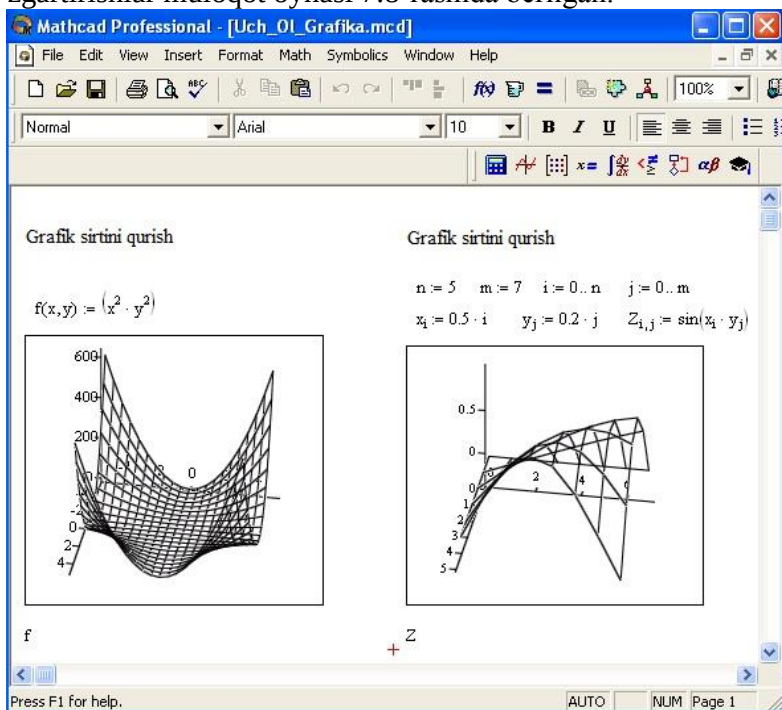
7.8-rasm. Ikki o'zgaruvchili funksiya grafagini qurish
