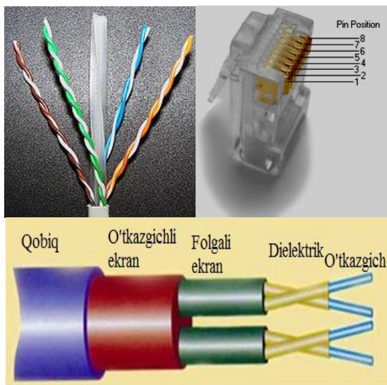
8.2-rasm. O'rama juft kabel
