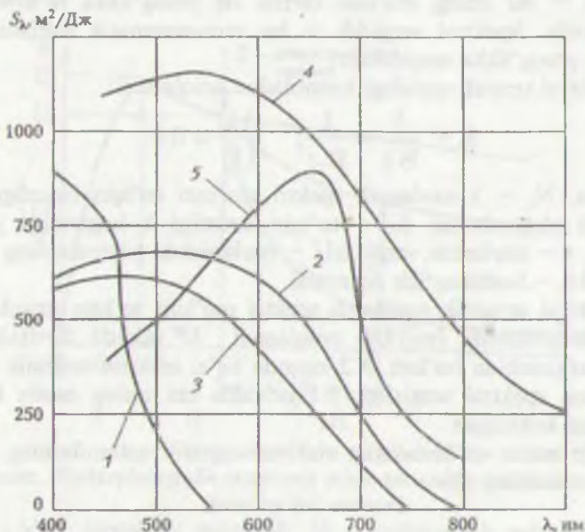
8.2-rasm. Ko'p marta qo'llanadigan EFQning spektral sezgirliqi: S_{\lambda} – fotosezgirlik; \lambda – to'liqin uzunligi; 1 – Se, 2 – Se-Te; 3 – \text{As}_2\text{Se}_3 ; 4 – ko'p komponentli tuzilmalar; 5 – amorf kremniy.
