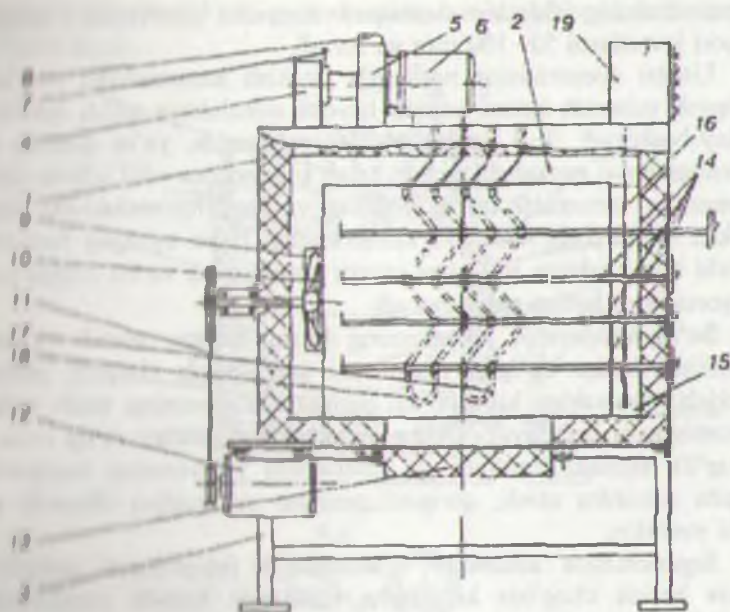
6.21-rasm. Fotopolimer qoliplarni quritish uskunasi- ning prinsipul sxemasi.
