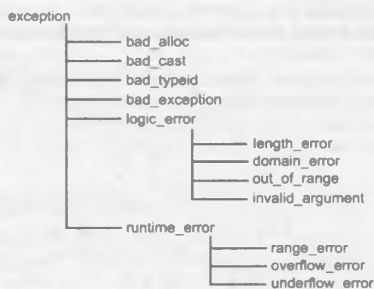
Рис. 16.1. Иерархия классов стандартных исключений
