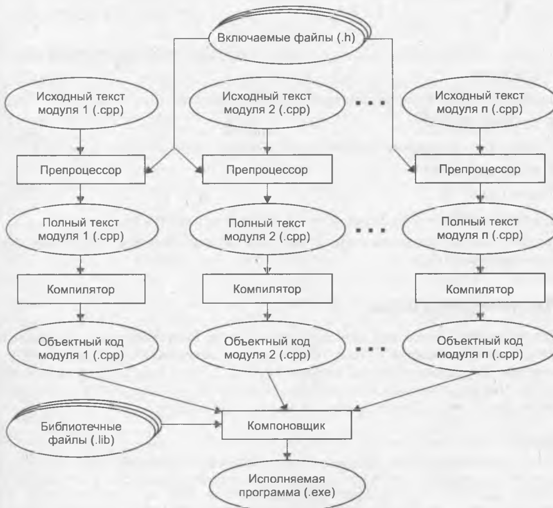
Рис. 1.2. Этапы создания исполняемой программы
