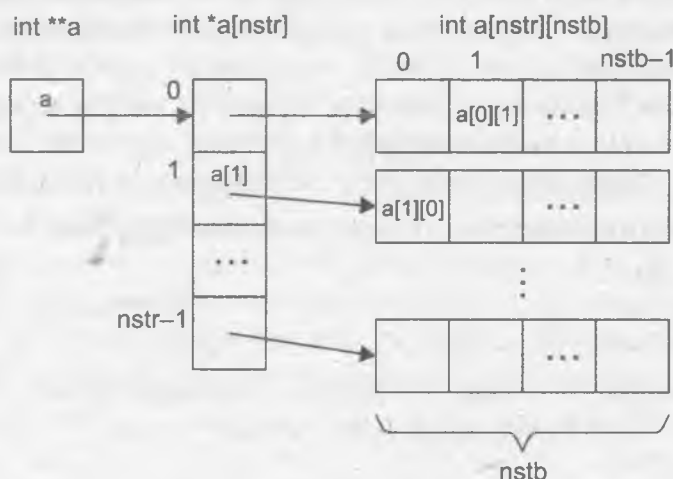
Рис. 1.10. Выделение памяти под двумерный массив
