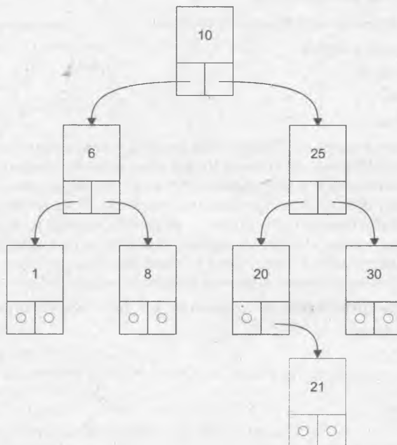
Рис. 3.3. Бинарное дерево
