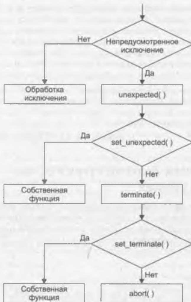
Рис. 7.1. Алгоритм обработки исключения
