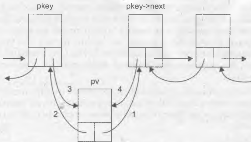
Рис. 3.2. Вставка элемента в список
