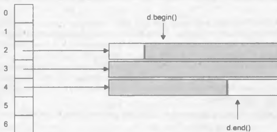
Рис. 12.1. Организация двусторонней очереди
