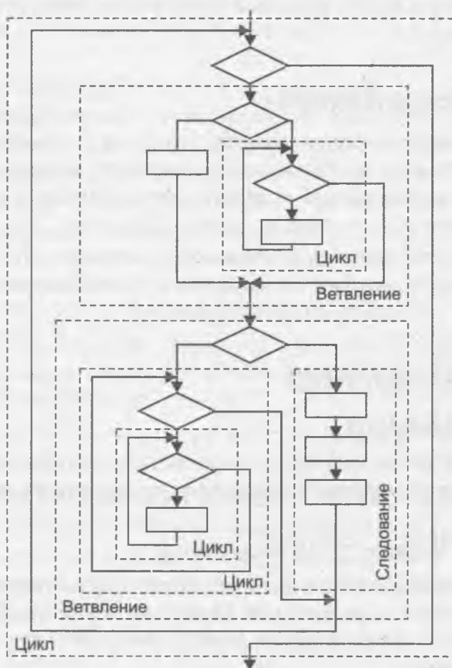
Рис. 1.4. Вложение базовых конструкций
