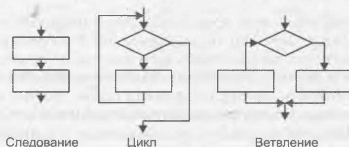
Рис. 1.3. Базовые конструкции структурного программирования
