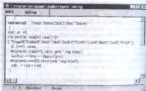
4.2-rasm. Kod Muharriri bajarilayotgan modul matnining Unit1.cpp faylida kiritilishi va tahrir qilinishini ta'minlaydi.
