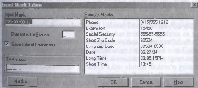
4.17-rasm. Telefon raqamlarini kiritish uchun niqobni yaratish.
