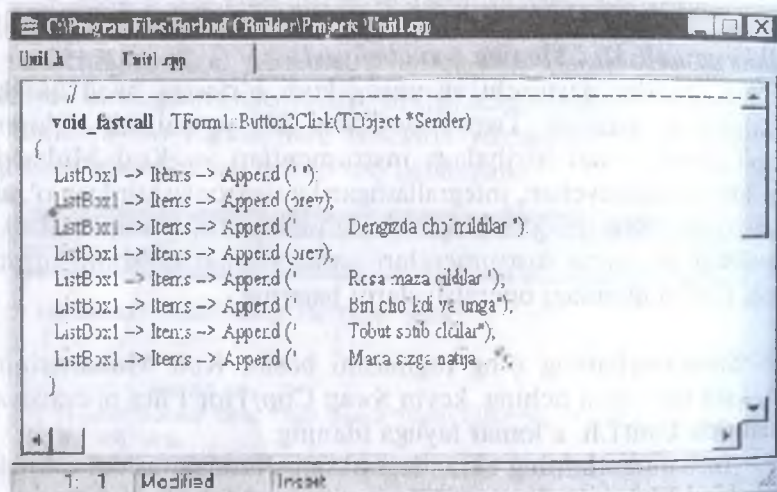
4.3-rasm. Unit1.cpp faylida voqcaning yangi qayta ishlatgichi.
