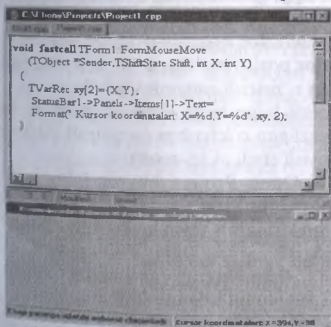
4.14-rasm. Axborotning holatlar satri paneliga chiqarilishi.
