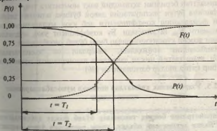
3.05- чизма. Ишончилилик коэффициенти P(t) ва рад этишлик эҳтимоли F(t) нинг буюмни эксплуатация қилиш вақтига боғлиқлиги
