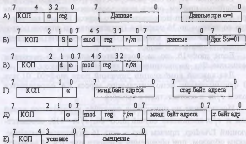
Рис. 5.8. Формат команд микропроцессора 8086.
