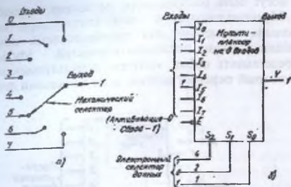
Рис.2.15. Механический коммутатор – аналог мультиплексора/ селектора данных (а) и мультиплексор на восемь входов (б).
