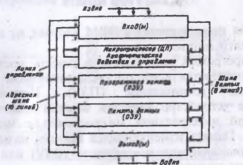
Рис. 1.6. Типовая структура микро-ЭВМ.
