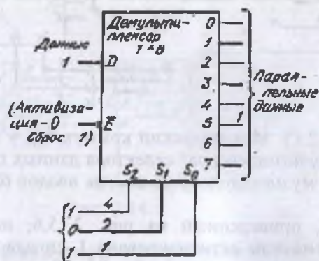
Рис. 2.16. Схема демультиплексора 1x8.
