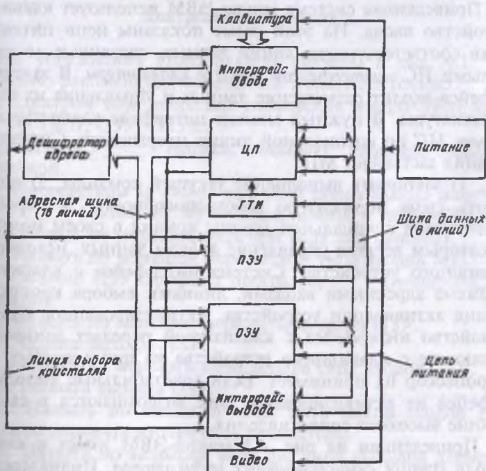
Рис. 4.1. Архитектура микро-ЭВМ.
