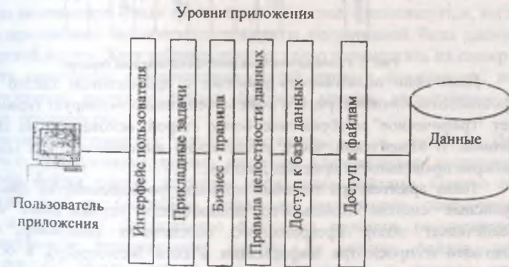
Рис. 4. Типичные уровни компьютерного приложения
