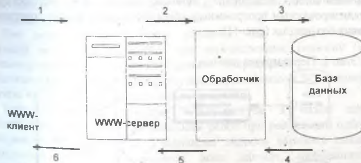
Рис. 10. Динамическое создание гипертекстовых документов на основе содержимого базы данных
