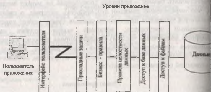
Рис. 5. Размещение большей части задач на сервере
