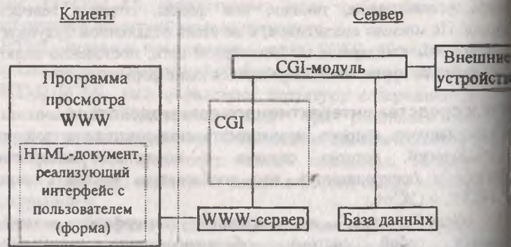
Рис. 3. Две части интерактивного интерфейса
