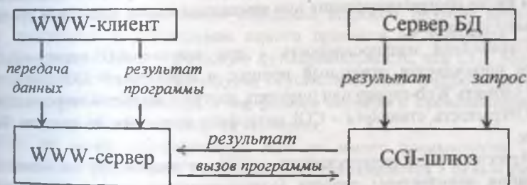
Рис.14. Схема взаимодействия CGI-шлюза
