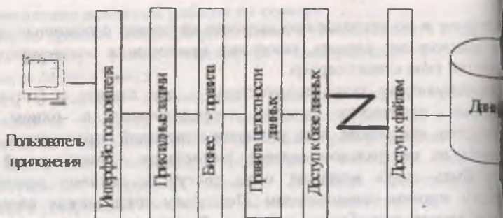
Рис. 6. Размещение большой части задач на стороне клиента
