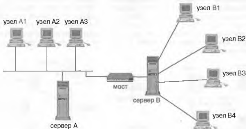
Рисунок 2.19. Две сети соединены через мост.
