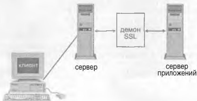
Рисунок 8.11. SSLD заменяет обычного клиента для безопасного сервера.
