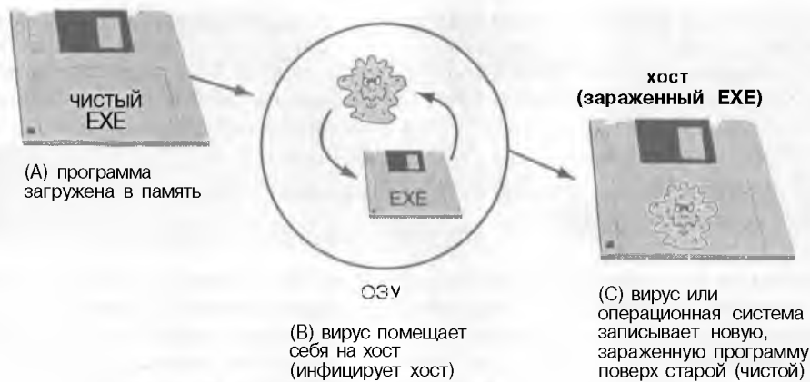
Рисунок 14.3. Вирус копирует себя внутрь расположенного в памяти файла.
