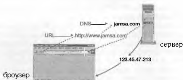
Рисунок 9.21. Имя DNS зависит от идентификатора URL, который, в свою очередь, зависит от выбранной пользователем гиперссылки.
