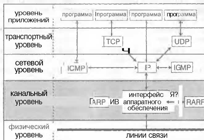
Рисунок 2.4. Реализация модели ISO/OSI в рамках TCP/IP.
