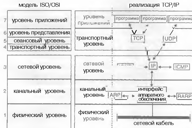
Рисунок 2.2. Модель ISO/OSI и стек протоколов.
