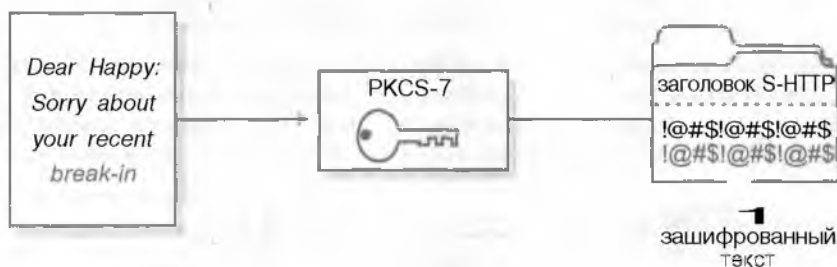
Рисунок 7.3. Сервер зашифровывает обычный текст и помещает его в пакет S-HTTP.
