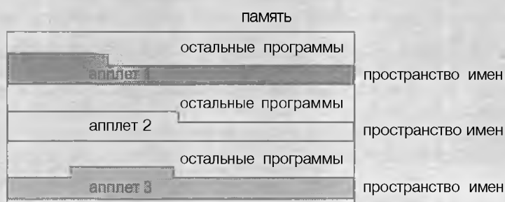
Рисунок 13.6. Виртуальная машина Java поддерживает несколько пространств имен.
