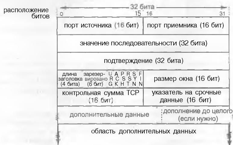
Рисунок 2.13. Структура заголовка сегмента (или сообщения) TCP.
