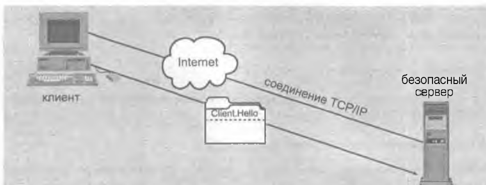
Рисунок S.3. Сообщение Client.Hello .
