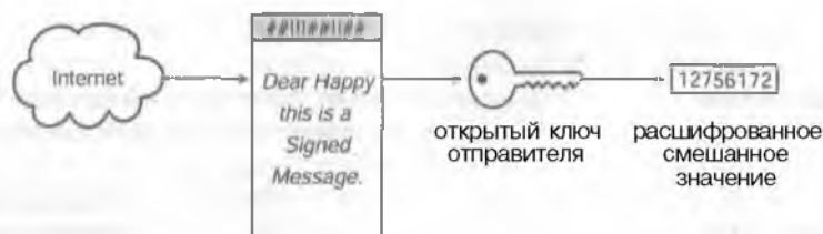
Рисунок 5.3. При помощи открытого ключа отправителя получатель может расшифровать значение цифровой подписи.
