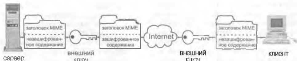
Рисунок 7.16. Обмен сообщениями при помощи внешних ключей.
