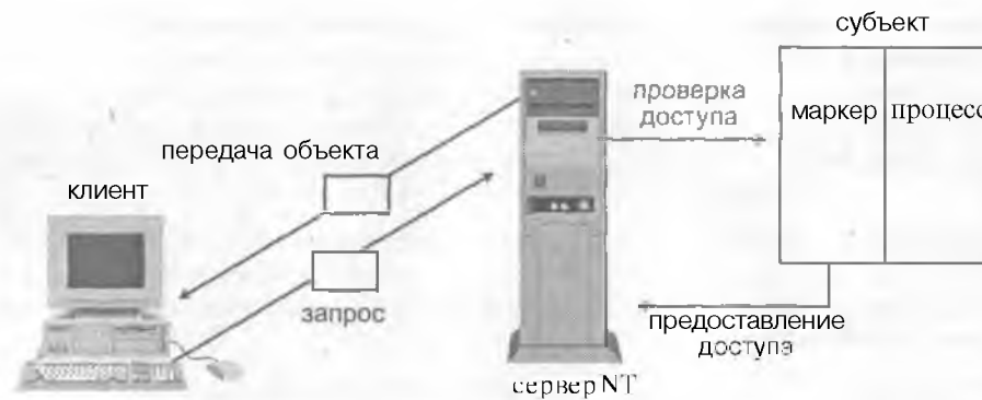
Рисунок 15.7. Операционная система проверяет маркер субъекта.
