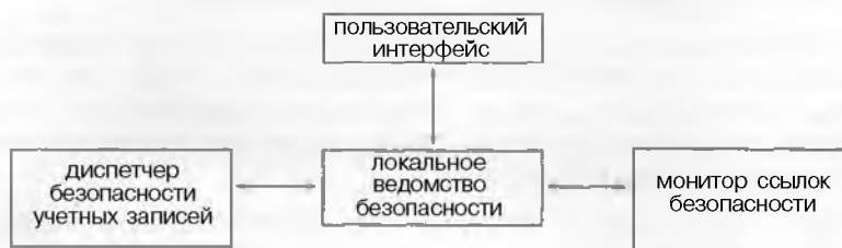
Рисунок 15.4. Взаимодействие четырех компонентов безопасности Windows NT.
