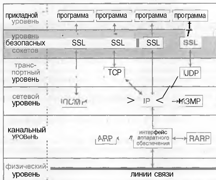
Рисунок 8.1. Уровни SSL расположены между существующими протоколами TCP/IP.
