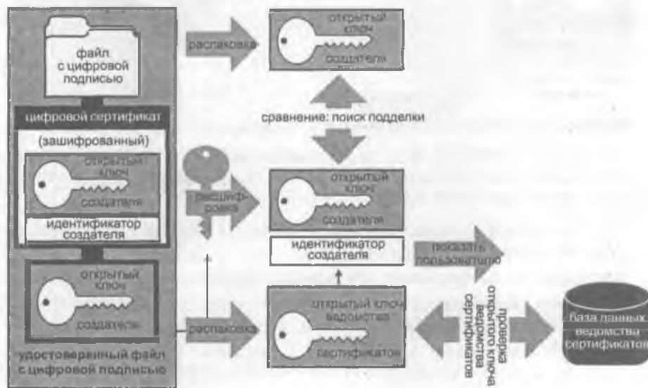
Рисунок 5.19. Проверка цифровой подписи и сертификата.
