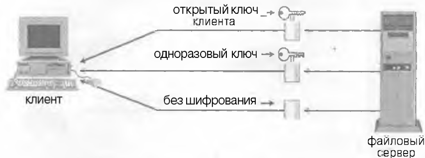
Рисунок 10.5. Файловый сервер может зашифровать пересылаемый файл или отправить его в виде обычного текста.
