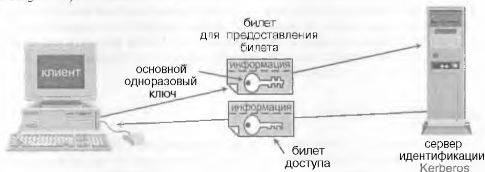
Рисунок 10.7. Клиент посылает билет для предоставления билета и получает билет доступа.
