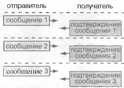
Рисунок 2.8. Передача данных с использованием простых подтверждений.
