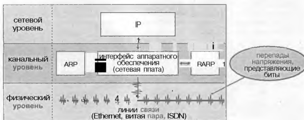
Рисунок 2.5. Канальный уровень осуществляет передачу данных между сетевым и физическим уровнями.
