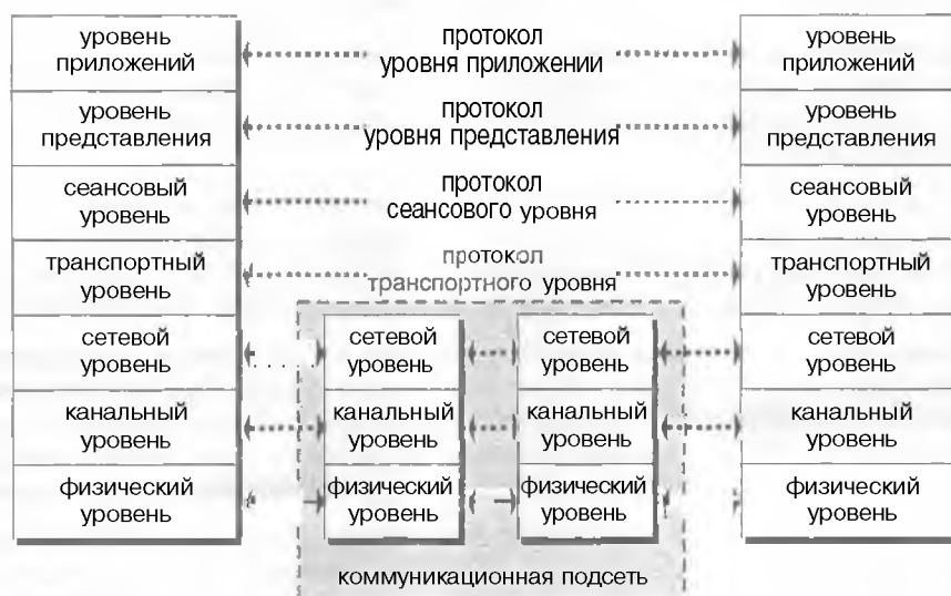
Рисунок 2.23. Коммуникационная подсистема сети.
