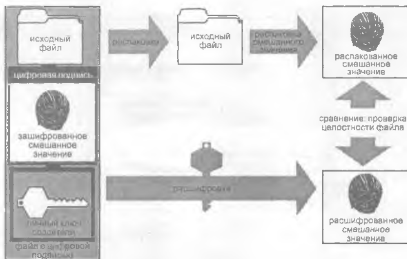
Рисунок 11.2. С помощью цифровой подписи можно идентифицировать создателя документа.
