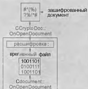
Рисунок 4.19. Переопределение функции OnOpenDocument .
