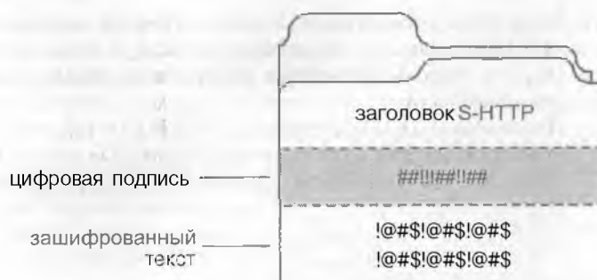
Рисунок 7.12. Зашифрованное сообщение с цифровой подписью.
