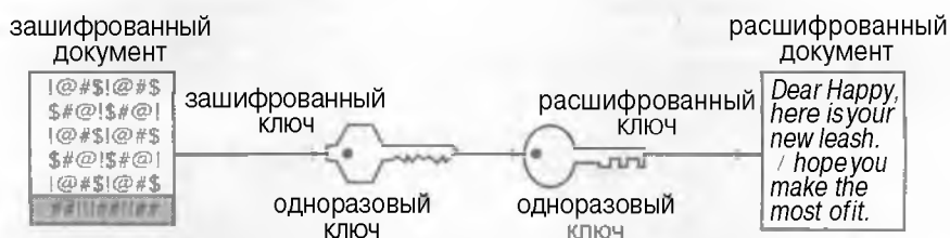
Рисунок 4.15. Для расшифровки полученного одноразового ключа получатель использует свой личный ключ.
