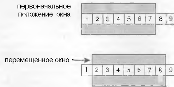
Рисунок 2.9. В протоколе TCP используется скользящее окно.
