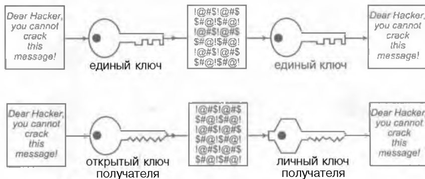
Рисунок 7.7. Сравнение систем с симметричным и асимметричным ключом.
