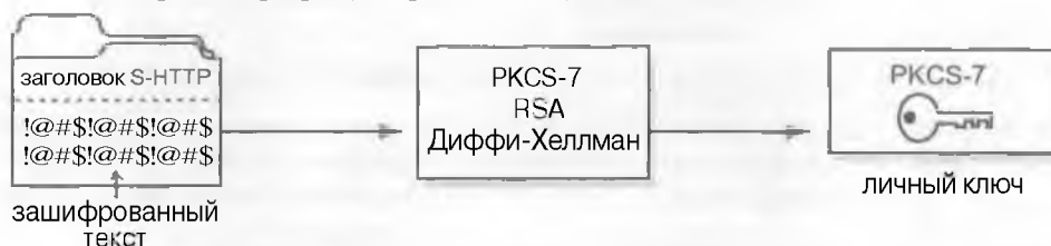
Рисунок 7.4. Клиент считывает заголовок сообщения и сравнивает его с известными стандартами шифрования.
