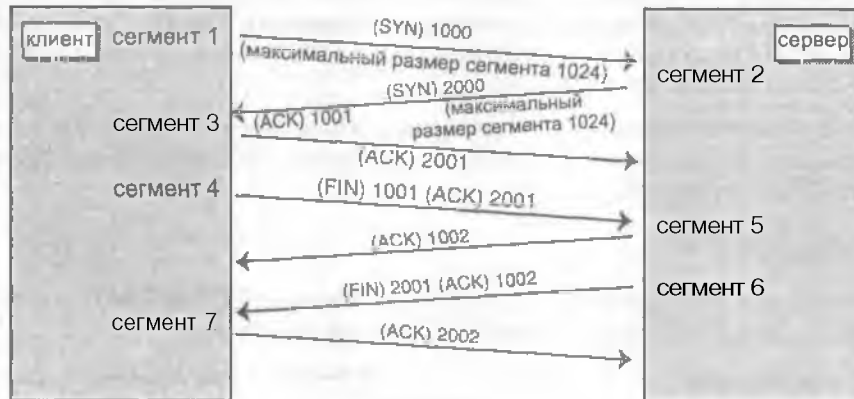
Рисунок 2.12. Идентификация данных и потоков с точки зрения клиента TCP-модуля.
