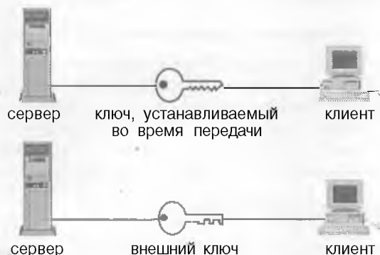
Рисунок 7.8. В S-HTTP используется два метода работы с ключами.
