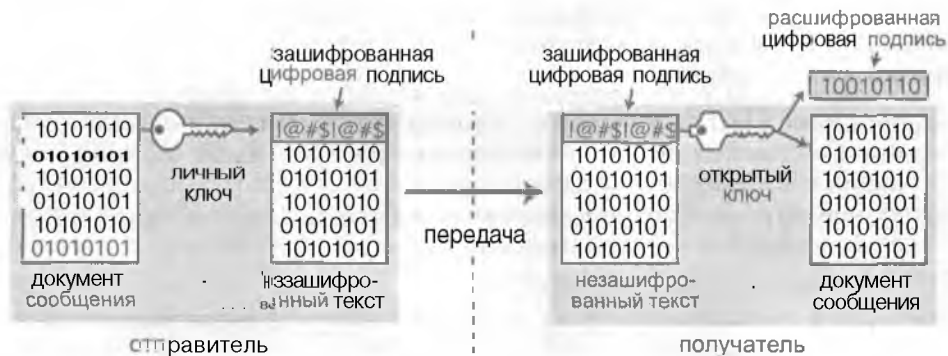
Рисунок 4.12. При помощи цифровых подписей можно идентифицировать автора документа.
