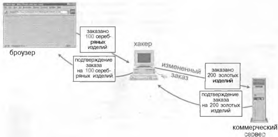
Рисунок 9.23. Хакер может изменить передаваемую информацию.
