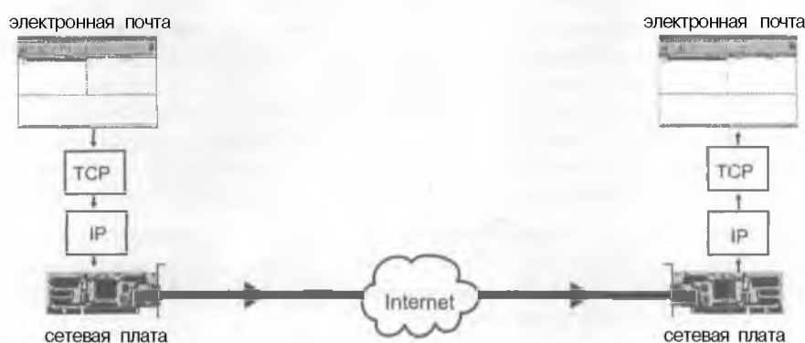
Рисунок 2.3. Этапы передачи файла электронной почты.
