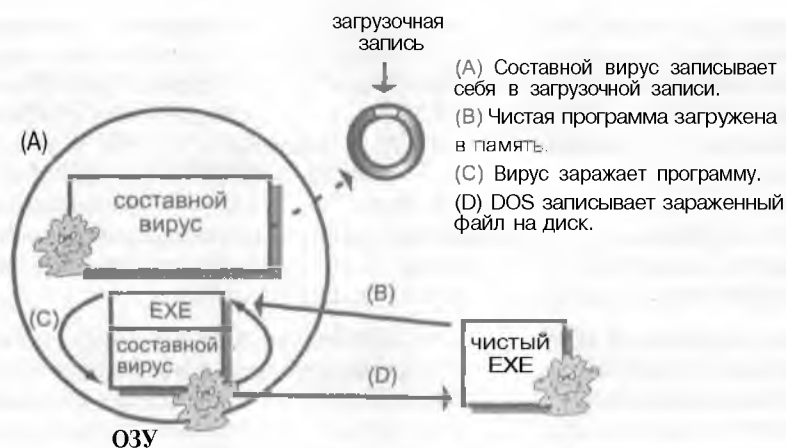
Рисунок 14.7. Действия составного вируса.
