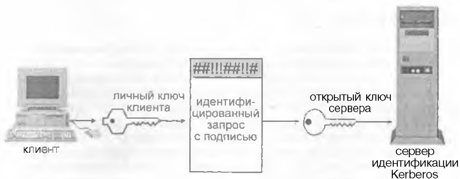
Рисунок 10.1. Клиент пересылает зашифрованное сообщение надежному серверу.
