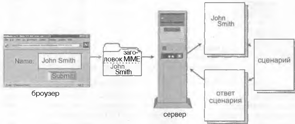
Рисунок 20.7. Процесс обработки данных сценарием.
