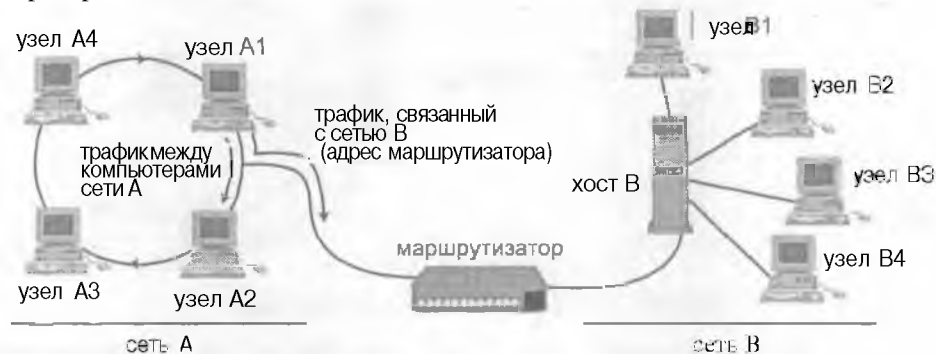
Рисунок 2.21. Маршрутизатор пропускает только те пакеты, которые содержат его адрес или адрес другой сети.
