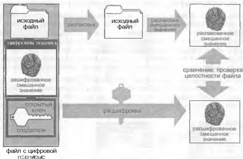
Рисунок 5.18. Проверка целостности файла при помощи цифровой подписи.
