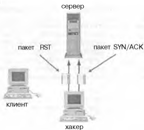
Рисунок 9.11. Хакер посылает два пакета серверу.
