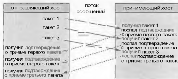
Рисунок 2.10. Передача данных и подтверждений с помощью скользящего окна.
