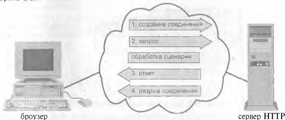
Рисунок 20.6. Изменение транзакции при использовании сценариев CGI.
