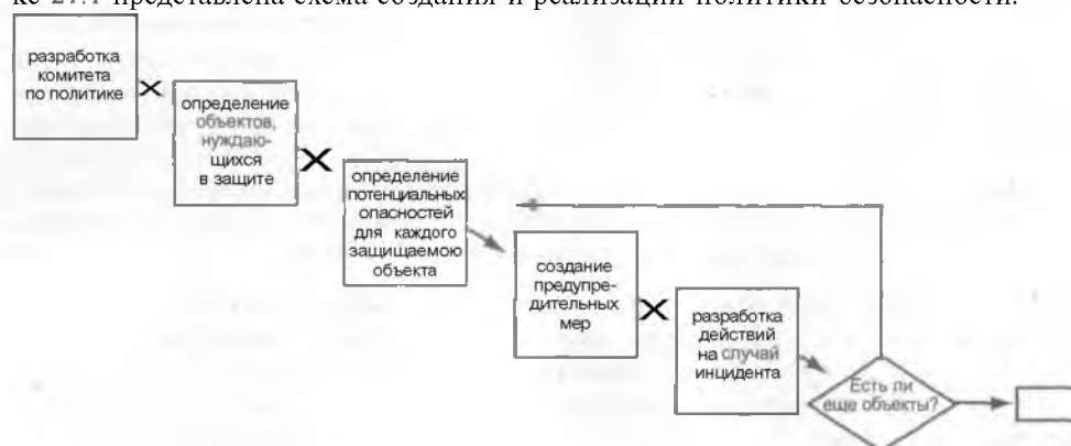
Рисунок 21.1. Процесс создания и реализации политики безопасности.
