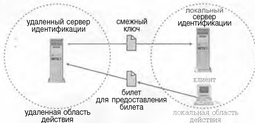
Рисунок 10.10. Сервер идентификации использует смежный ключ для проверки удаленного клиента,
