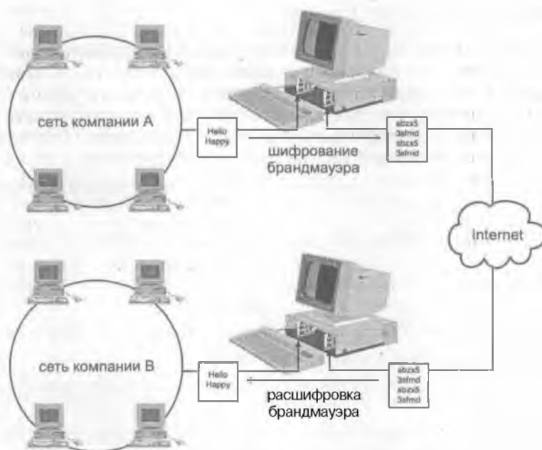
Рисунок 3.9. Использование функций шифрования некоторыми брандмауэрами.
