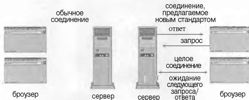
Рисунок 6.3. Сравнение обычного и нового стандартов.
