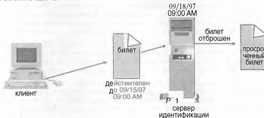
Рисунок 10.16. Сервер идентификации отбрасывает переигранные билеты с просроченным временем.
