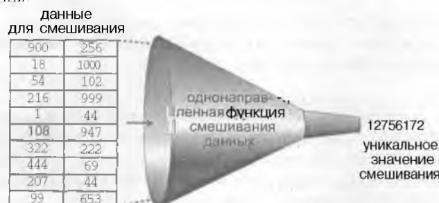
Рисунок 4.18. Преобразование сообщения в профиль сообщения.
