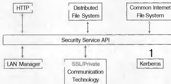
Рисунок 15.12. Модель интерфейса SSPI.
