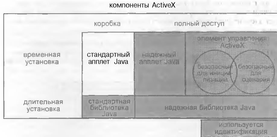
Рисунок 19.5. Схема безопасности элементов управления ActiveX.
