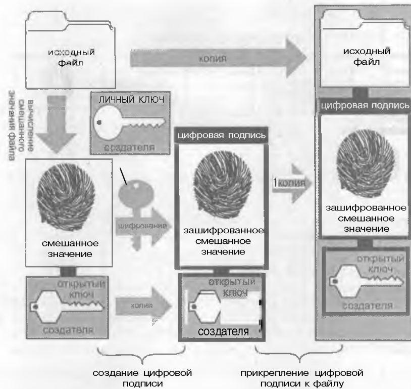
Рисунок 5.17. Создание и использование цифровых подписей в алгоритме с открытым ключом.
