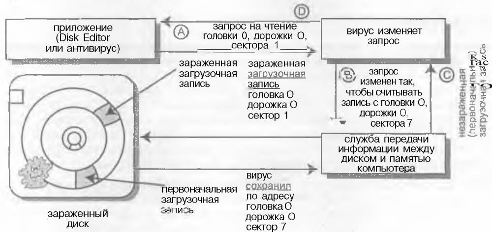
Рисунок 14.5. Стелс-вирус атакует загрузочную запись дискеты.
