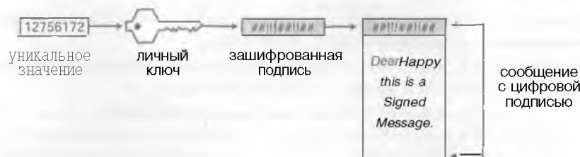
Рисунок 5.2. Создание цифровой подписи письма.
