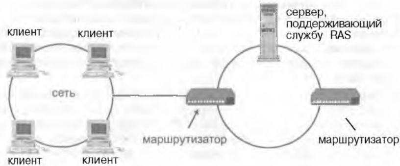
Рисунок 15.16. Брандмауэр экранирующей подсети и сервер RAS.
