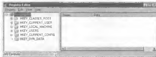
Рисунок 12.5. Редактор реестра.
