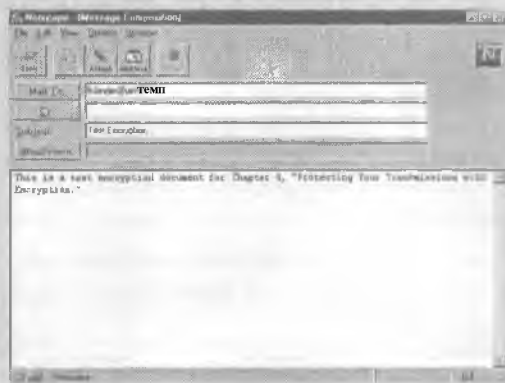
Рисунок 4.6. Незашифрованный документ.
