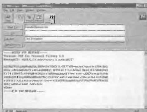
Рисунок 4.8. Зашифрованный документ.
