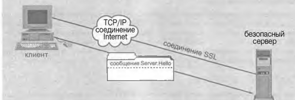
Рисунок 8.4. Ответ Server.Hello .
