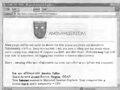
Рисунок 19.9, Web-сайт Anonymizer.
