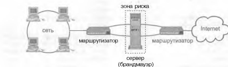
Рисунок 3.8. Зона риска сети, защищенной брандмауэром.
