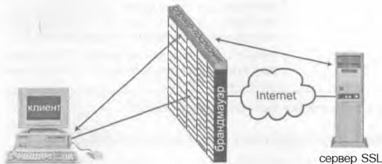
Рисунок 8.12. Клиент соединяется с сервером-посредником, а затем сервер-посредник соединяется с SSL-сервером.
