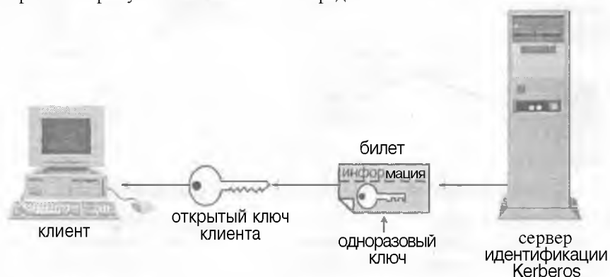
Рисунок 10.2. Сервер зашифровывает билет, а затем пересылает его клиенту.
