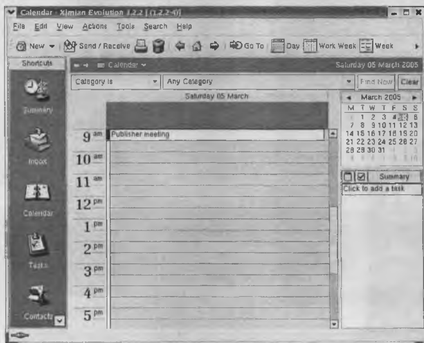
Рис. 11.6. Интерфейс ежедневника Evolution
