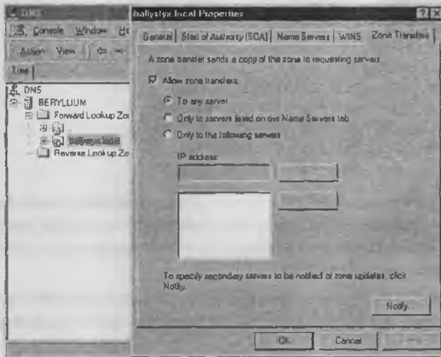
Рис. 2.12. Диалоговое окно диспетчера переноса зон DNS Windows 2000
