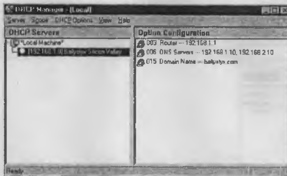
Рис. 2.8. DHCP Manager Windows NT — Ballystyx, Кремниевая Долина
