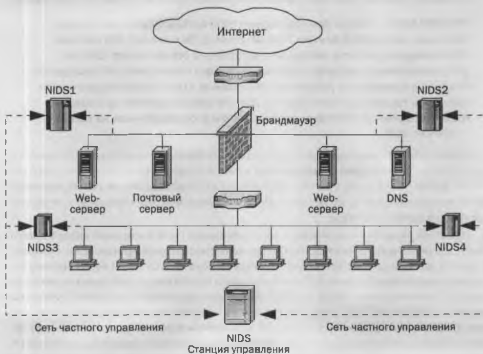
Рис. В.3. Сеть DIDS
