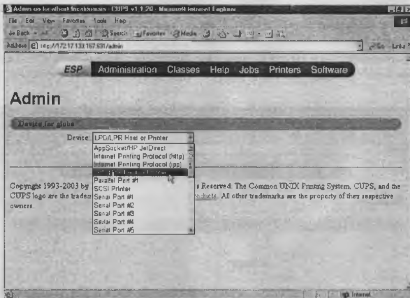
Рис. 6.3. Конфигурирование устройства принтера
