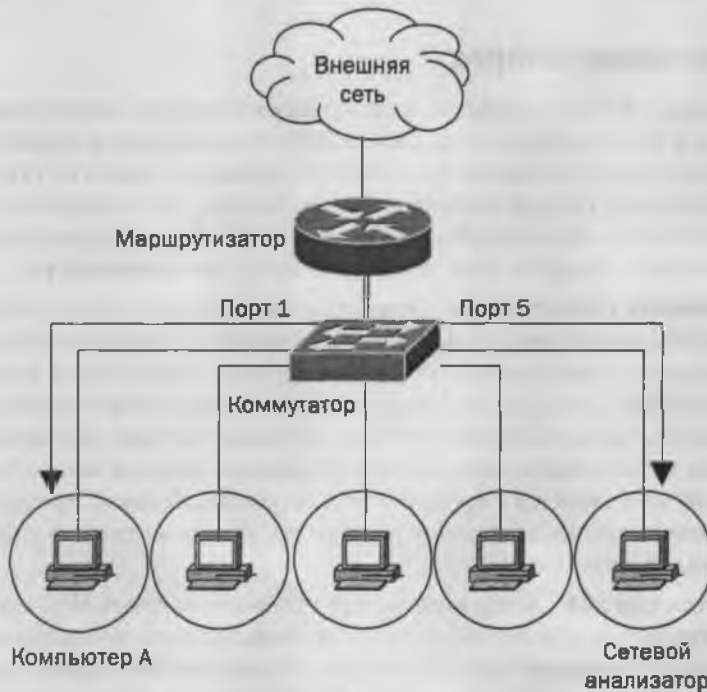
Рис. А. 6. Зеркальное отражение порта
