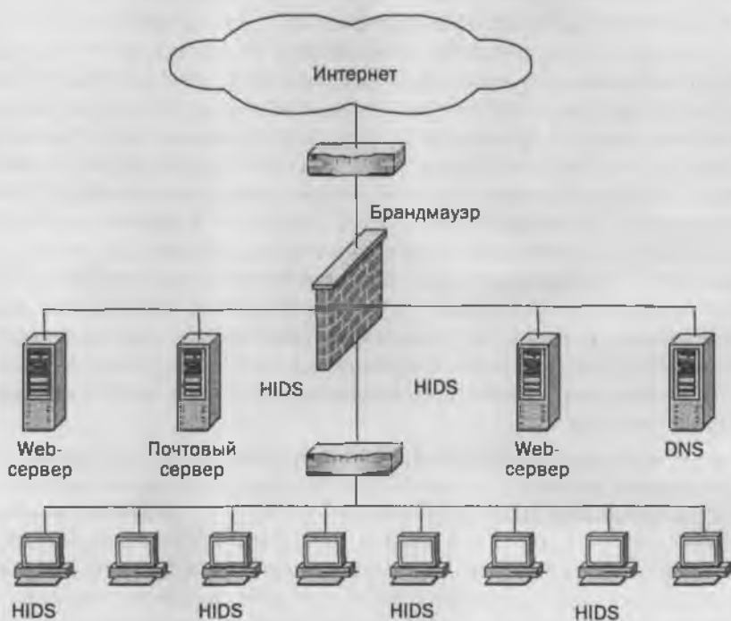
Рис. В.2. Сеть HIDS
