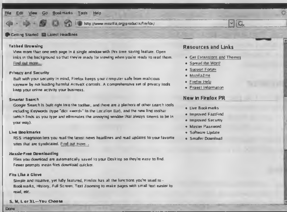
Рис. 11.16. Firefox
