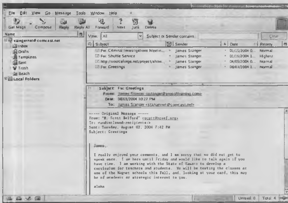
Рис. 11.8. Mozilla Mail
