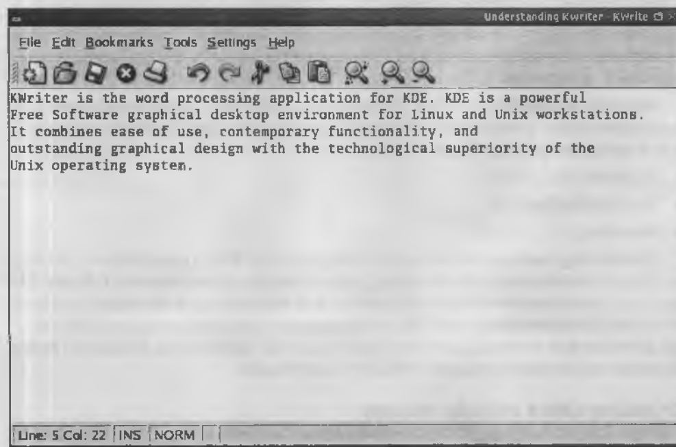
Рис. 11.23. KWriter
