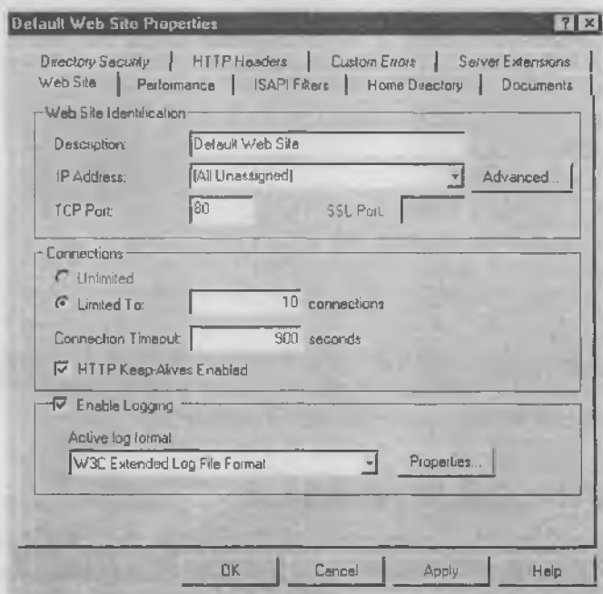
Рис. 9.3. Свойства web-сайта по умолчанию
