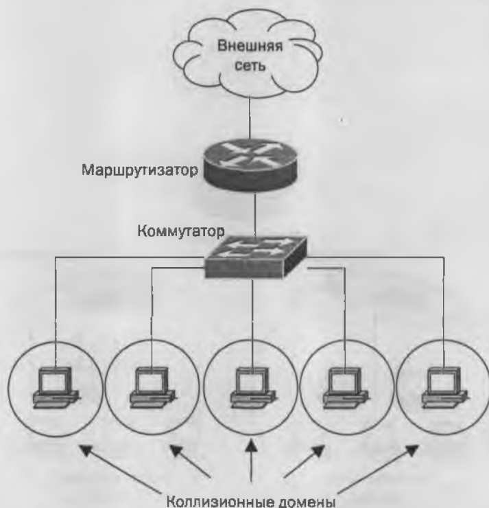
Рис. А. 5. Коллизийные домены коммутатора
