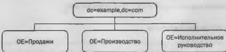
Рис. 3.2. Дерево информации каталога — Модель для рабочей группы
