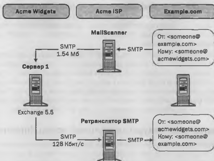
Рис. 7.7. Текущая архитектура электронной почты Интернет компании AcmeWidgets
