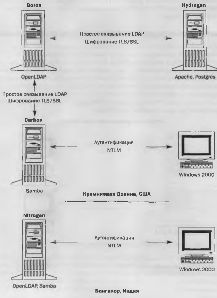
Рис. 4.7. Проект служб аутентификации компании Ballystyx Engineering
