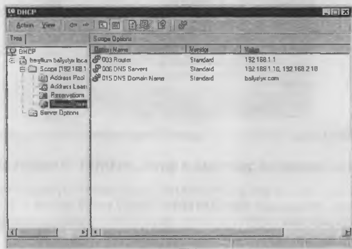
Рис. 2.11. DHCP Manager Windows 2000 — Подробная информация об области действия
