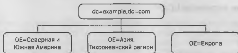
Рис. 3.3. Дерево информации каталога — Географическая модель
