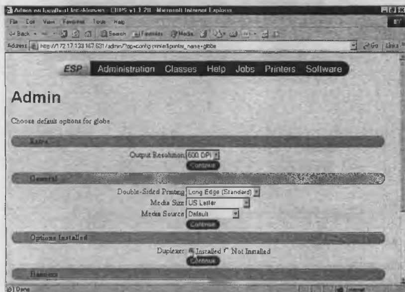
Рис. 6.8. Конфигурирование настроек принтера
