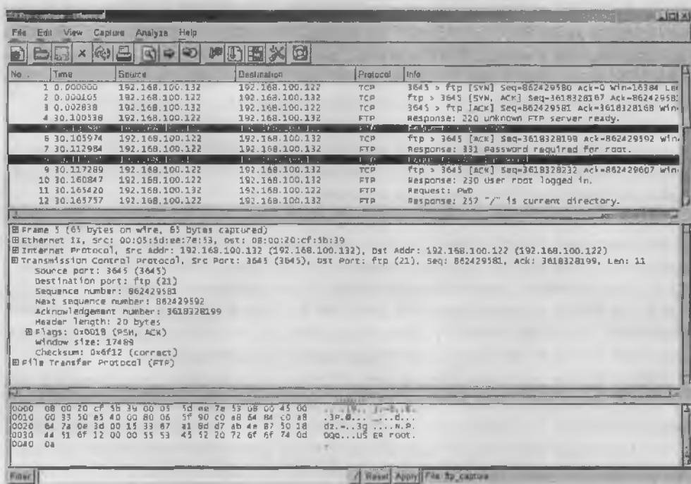
Рис. А. 2. Пример прослушивания подключения
