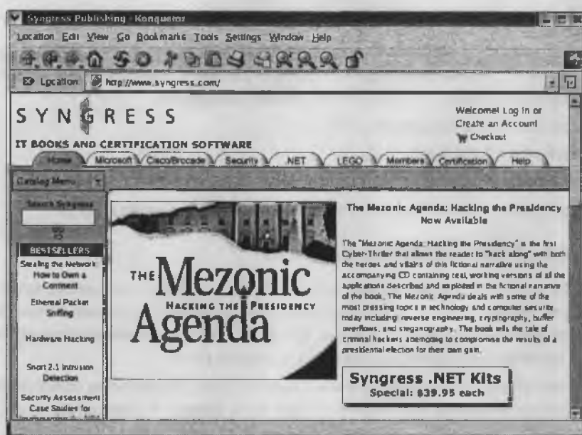
Рис. 11.17. Web-браузер Konqueror
