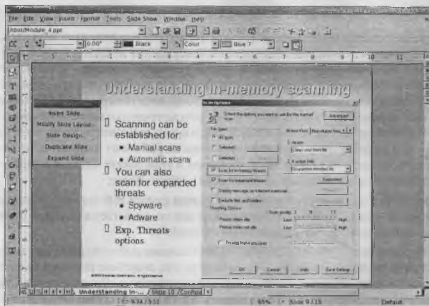
Рис. 11.21. Star Impress
