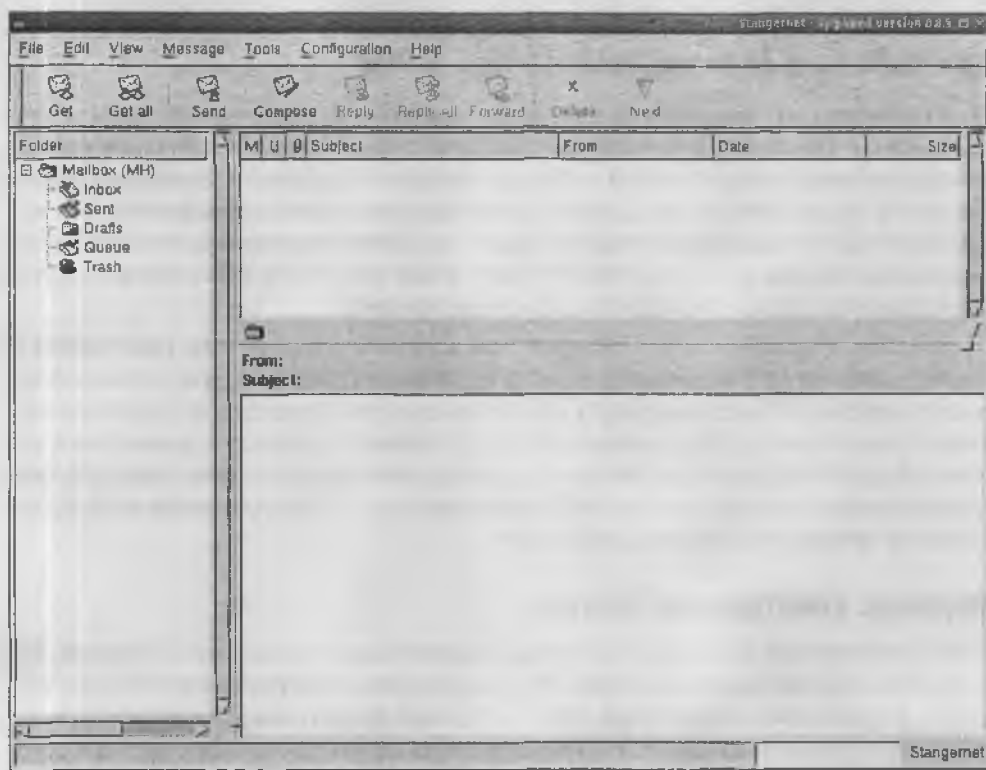
Рис. 11.10. Sylpheed
