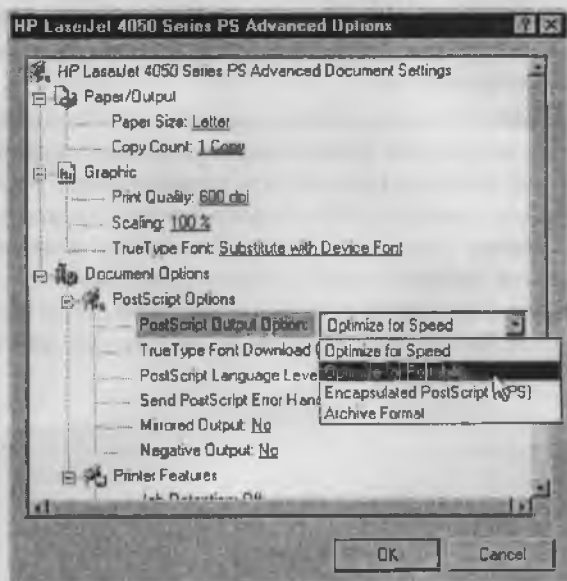
Рис. 6.14. Оптимизация портативности
