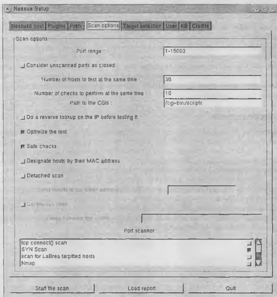
Рис. С. 2. Опции Nessus Scan
