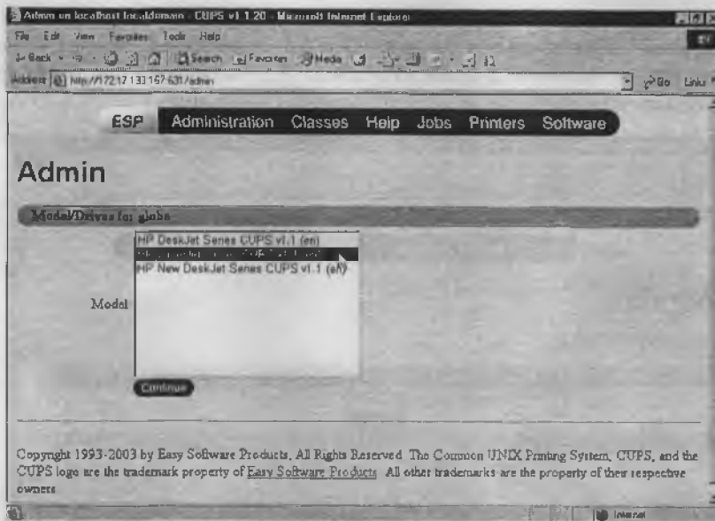
Рис. 6.6. Указание модели принтера
