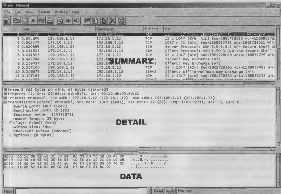
Рис. А. 1. Пример окна отображения сетевого анализатора Ethernet
