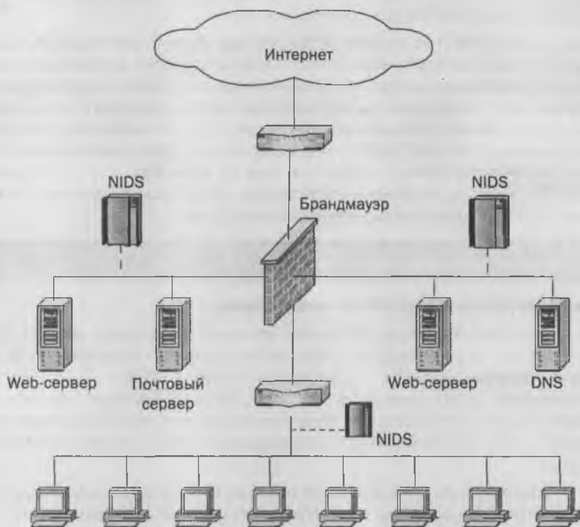
Рис. В.1. Сеть NIDS
