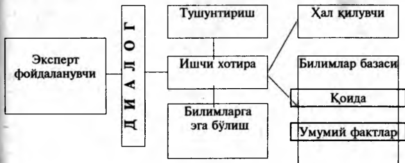
2.07-расм. Типик эксперт тизимнинг структураси
