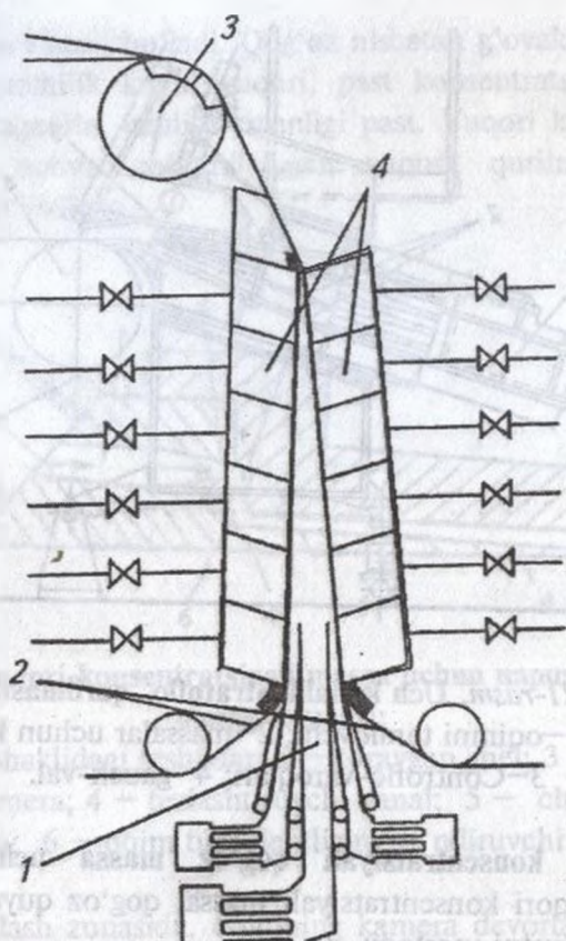
20-rasm. Controflo-Foemer shakllantiruvchi qurilmasining sxemasi: 1—uch qavatli napusk qurilma; 2—shakllantiruvchi setkalar; 3—gauch-val; 4—soʻruvchi qurilma.
