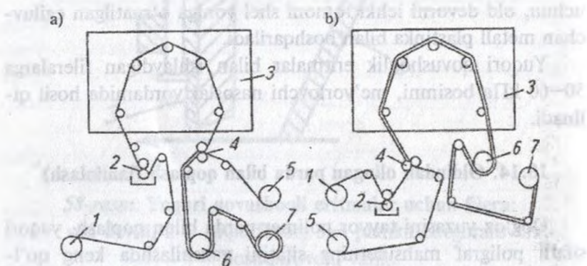
59-rasm. Laminlash sxemasi: a — quruq; b — ho'l:
