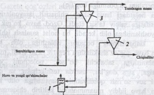
15-rasm. Vixrli tozalagichlar yordamida massadan havoni va vakuum-nasosni ishlatmasdan chiqarish qurilmasining sxemasi:
