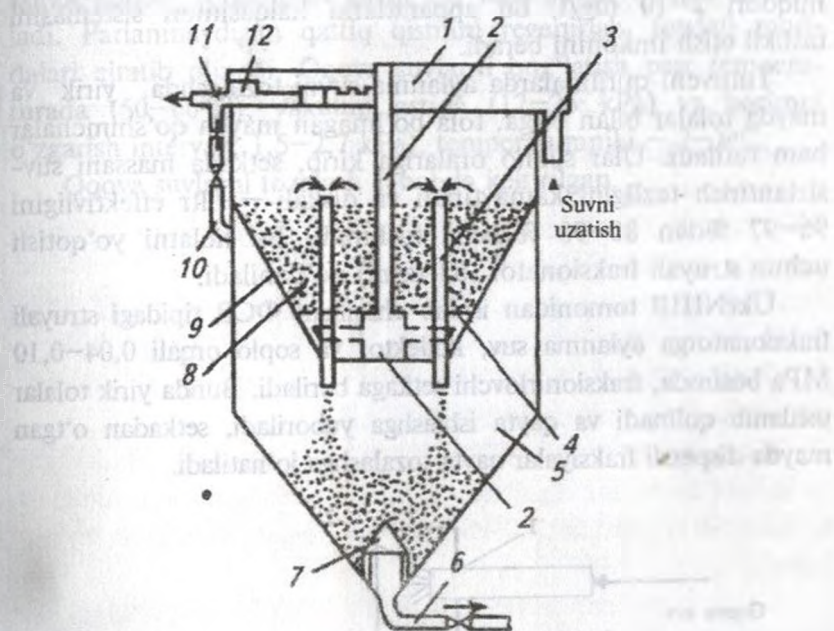
61-rasm. Aylanma suvni tindiruvchi qurilma sxemasi:
