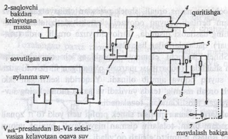
51-rasm. Massani shnek — pressdan keyin suyultirish seksiyasi:
