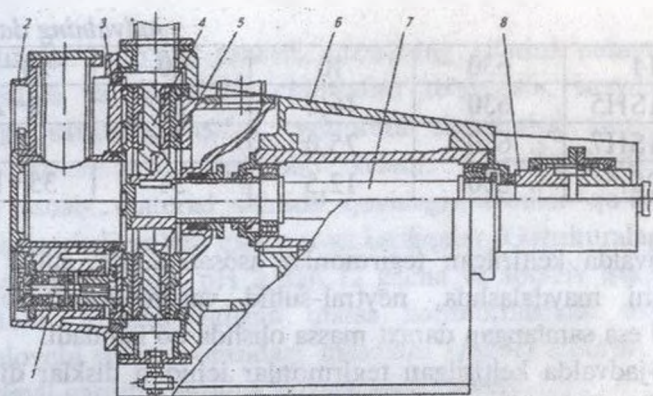
4-rasm. MD tipidagi ikkilangan diskali tegirmon:
