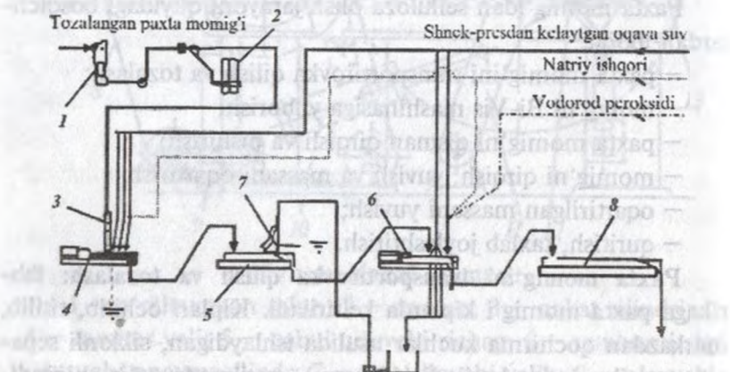
50-rasm. Bi-Vis seksiyasi:
