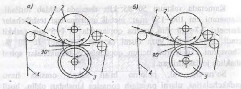
34-rasm. Jelobli pressga qog'oz polotnini uzatish sxemasi:
