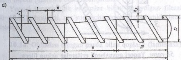
57-rasm. Ekstruzion usulida qoplama surtish: a—ekstruzion — laminlovchi qurilma; b—ekstruder sxemasi; d—shnekning asosiy o'lchamlari; 1—ekstruder; 2—ekstruder filerasi; 3—laminatorning qoplangan valigi; 4—laminatorning metalli sovituvchi val; 5—qog'oz polotno chetlarini qiruvchi qurilma; 6—tayanch podshipnik; 7—bunker; 8—silindr; 9—sovitish sistemasi; 10—qizdirish sistemasi; 11—shnek; 12—setka; 13—old tayanch; 14—dvigatel; 15—boshqaruvchi; 16—uzatkich; I—massani (polimer) kirish zonasi; II—siqish (plastifikatsiya) zonasi; III—siqib chiqarish zonasi.
