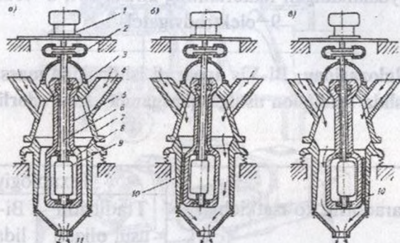
8-rasm. Vibratsion tebratuvchi tegirmon apparati rotorning har xir variantda ko'rinish sxemasi:
