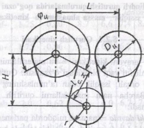
41-rasm. Qog'oz polotnini quritish silindrlari yuzasiga tegib turgan qismi va erkin yurish uzunligi.
