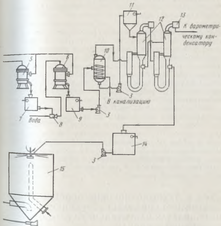
Рис. 41. Аппаратурно-технологическая схема стадий выращивания, выделения и сушки дрожжей.
