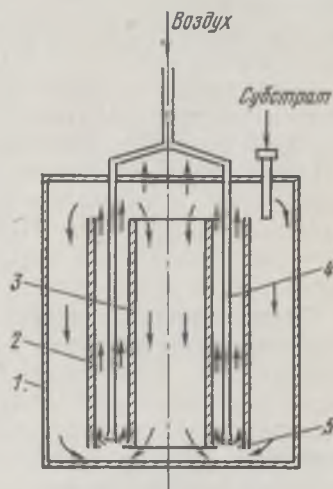
Рис. 22. Ферментатор с расщелоченным воздухоустройством:
