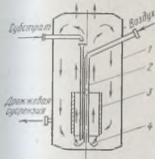
Рис. 21. Ферментатор системы Лефрансу — Марийне:
