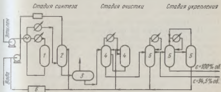
Рис. 98. Схема процесса получения этанола согласно VEBA-процессу:
