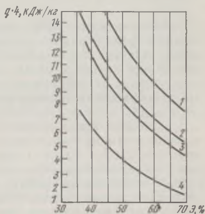
Рис. 103. Зависимость удельного тепловыделения q от эффективности потребления углерода различных субстратов:
