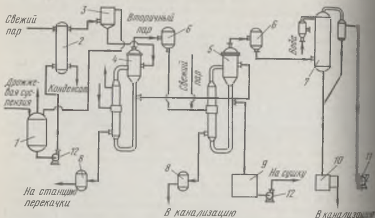
Рис. 35. Схема двухкорпусной вакуум-выпарной установки:
