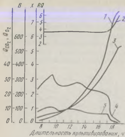
Рис. 84. Изменение концентрации биомассы x (1), коэффициента дыхания RQ (2), расхода основания B (3), удельной скорости потребления кислорода Q_{O_2} (4) и удельной скорости выделения углекислоты Q_{CO_2} (5) при периодическом культивировании C. lipolytica на гексадекане при скорости перемешивания 2000 об/мин.
