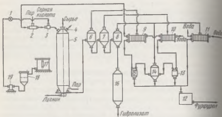
Рис. 43. Аппаратурно-технологическая схема получения гидролизата:
