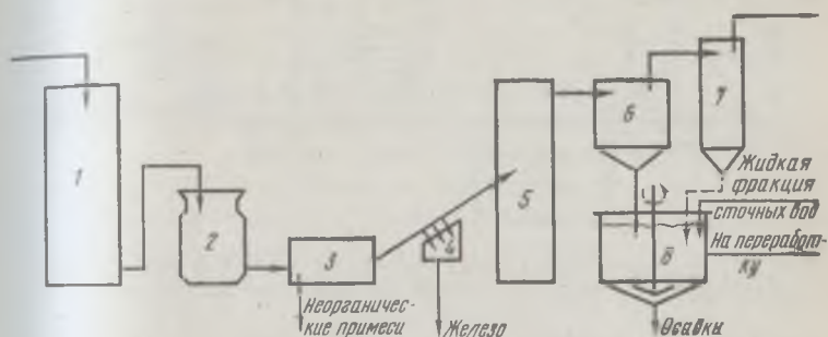
Рис. 60. Схема предварительной обработки городских отходов:
