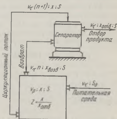
Рис. 18. Схема материальных потоков аппарата полного смешения с рециркуляцией биомассы микроорганизмов.
