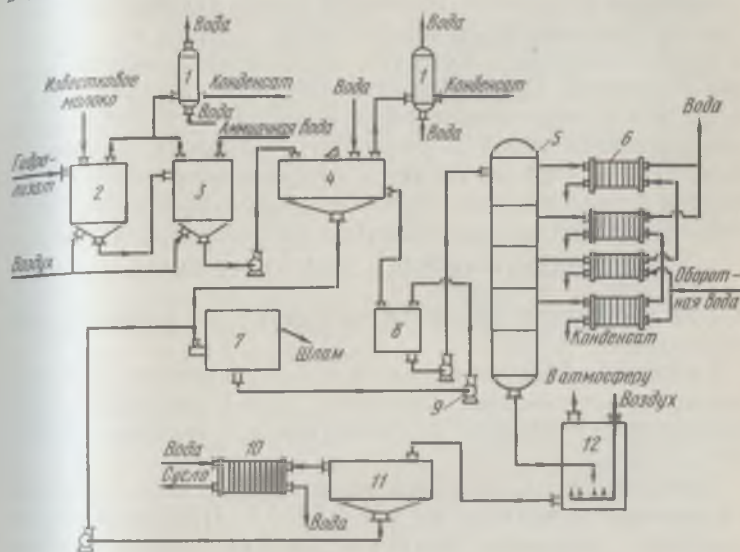
Рис. 46. Аппаратурно-технологическая схема обработки гидролизата перед подачей в дрожжерастильный аппарат:
