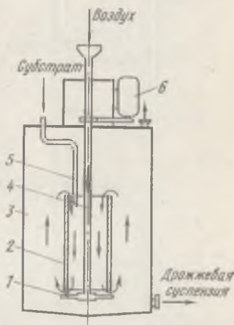
Рис. 23. Ферментатор с самовсасывающей системой аэрации:
