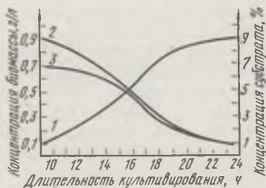
Рис. 78. Накопление биомассы и потребление субстрата в процессе периодического культивирования микроорганизмов на жидких углеводородах:
