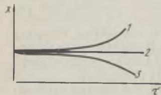
Рис. 10. Изменение концентрации микроорганизмов в непрерывно действующем аппарате полного смешения при различных соотношениях \mu и D : 1 — \mu > D ; 2 — \mu = D ; 3 — \mu < D .
