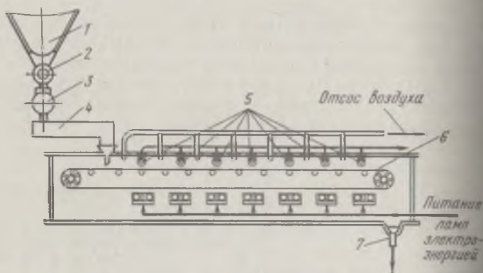
Рис. 40. Витаминизатор сухих дрожжей:
