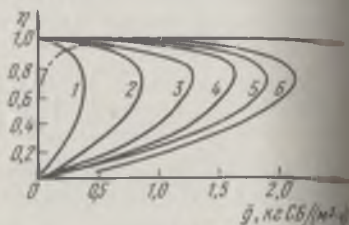
Рис. 16. Зависимость экономического коэффициента использования субстрата \eta от стационарной продуктивности аппарата g и различной исходной концентрации субстрата при выращивании дрожжевой культуры Candida tropicalis (в \text{кг}/\text{м}^3 ):
