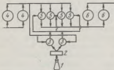
Рис. 113. Принципиальная схема получения посевного материала Brevibacterium sp. 22Л непрерывным способом:
