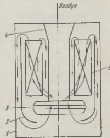
Рис. 31. Ферментатор с турбоэжекторными перемешивающими устройствами:
