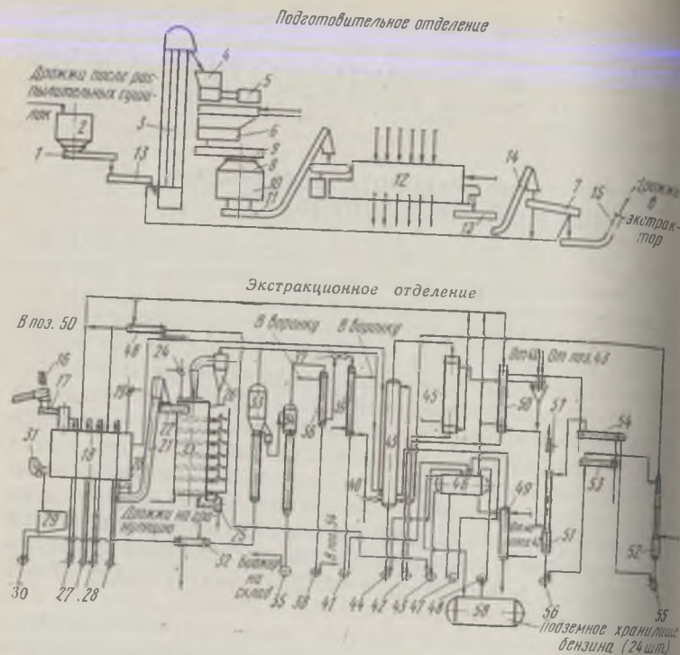
Рис. 104. Технологическая схема выделения микробных жиров:
