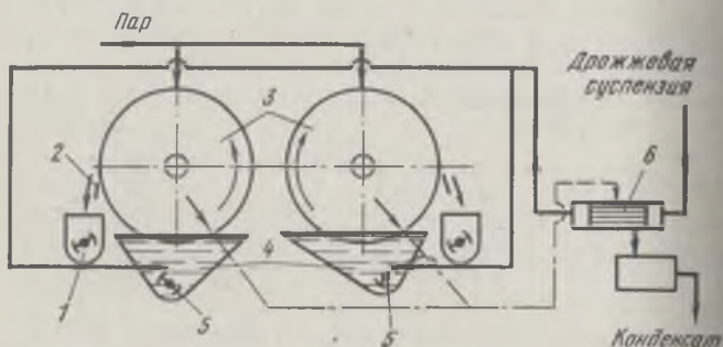
Рис. 37. Двухвальцовая паровая сушилка погружного типа:
