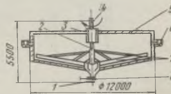
Рис. 48. Отстойник:
