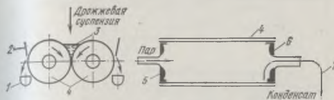
Рис. 36. Двухвальцовая паровая сушилка непогружного типа:
