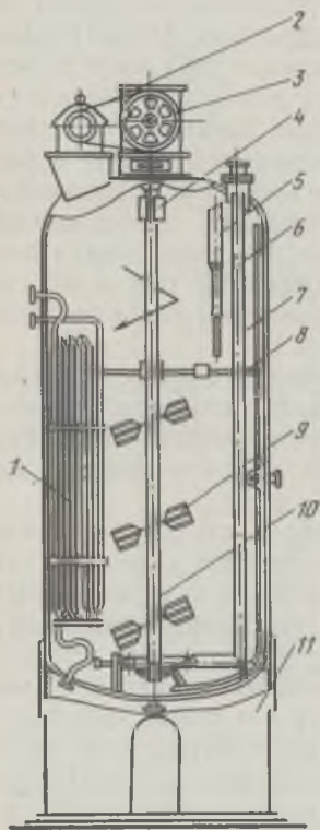
Рис. 116. Ферментатор вместимостью 50 м 3 :
