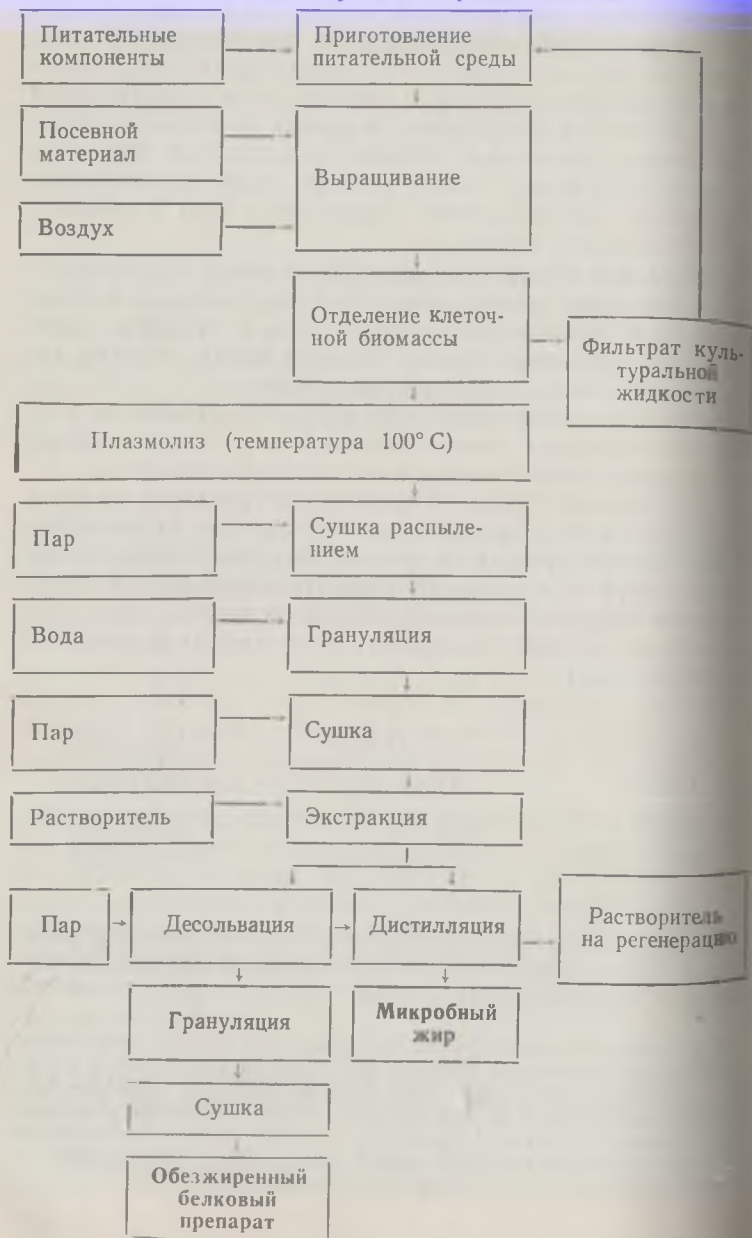
Схема 5. Основные этапы получения микробных липидов
