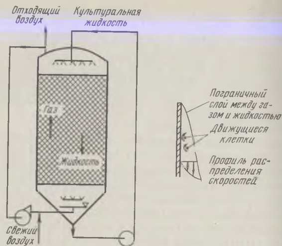
Рис. 28. Ферментатор со струящейся пленкой.
