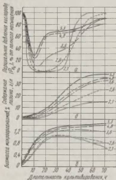
Рис. 110. Динамика изменения парциального давления кислорода (а), образования биомассы (б) и накопления лизина (в) при культивировании Corynebacterium glutamicum T-3 при различных значениях сульфитных чисел ( K_v ) в ферментаторе (на кривых цифра указывает величину сульфитного числа в ферментаторе).
