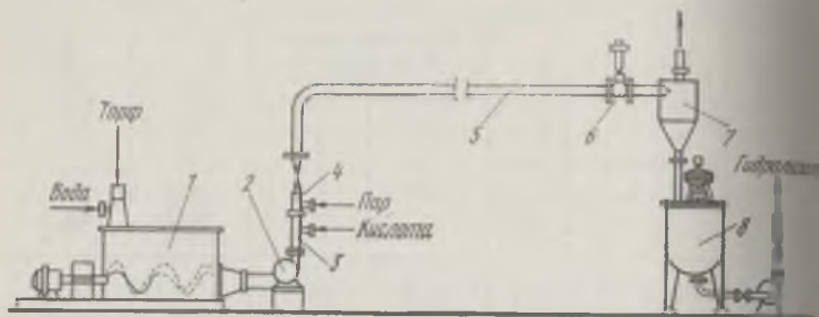
Рис. 57. Схема непрерывного гидролиза торфа с применением реактора идеального вытеснения:
