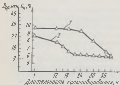
Рис. 81. Потребление фракции парафинов (1) и изменение величины среднего диаметра капель (2) в процессе периодического выращивания C. lipolytica при скорости аэрации 3,92 \text{ м}^3/\text{ч} .
