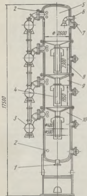
Рис. 49. Вакуум-охлади- тельная установка:
