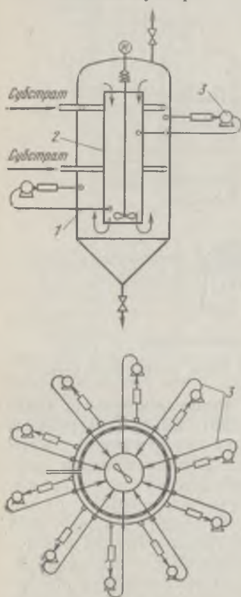
Рис. 26. Ферментатор с внешними циркуляционными потоками:
