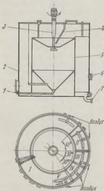
Рис. 33. Одноступенчатый флотатор:
