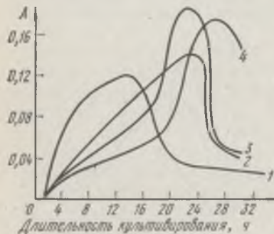
Рис. 66. Зависимость относительной скорости образования биомассы A. T. candida ФК от интенсивности аэрации среды (в г O_2 на 1 л/ч): 1 — 0,4; 2 — 2,16; 3 — 3,49; 4 — 5,23. Содержание лактозы в среде 4,56%.
