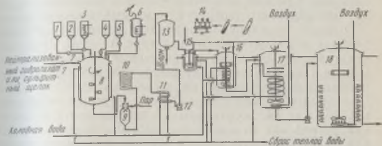
Рис. 20. Схема получения чистой культуры посевного материала:
