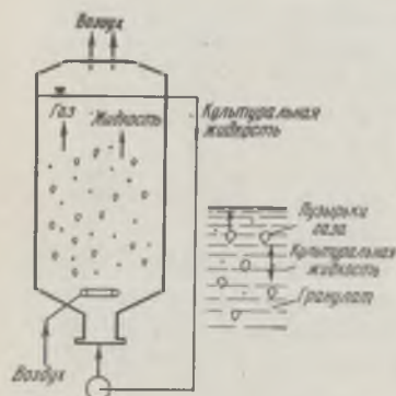
Рис. 29. Ферментатор с добавками гранулата.
