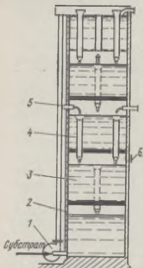
Рис. 24. Струйный ферментатор:
