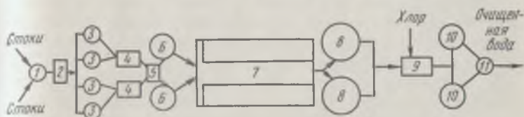
Рис. 119. Технологическая схема очистки стоков:
