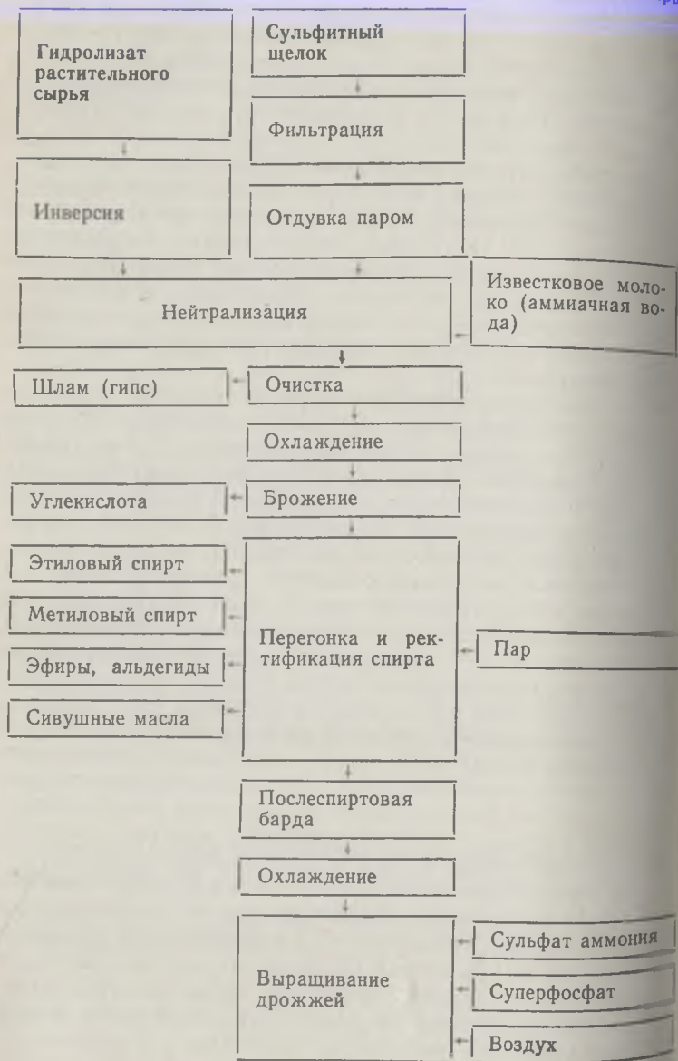
Схема 2. Основные стадии процесса производства этилового спирта и кормовых дрожжей из отходов переработки растительного сырья
