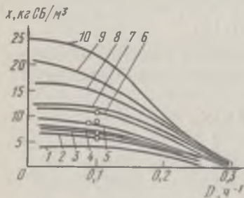
Рис. 13. Зависимость концентрации биомассы дрожжей культуры Candida tropicalis от коэффициента разбавления при различной исходной концентрации субстрата (в кг/м³):
