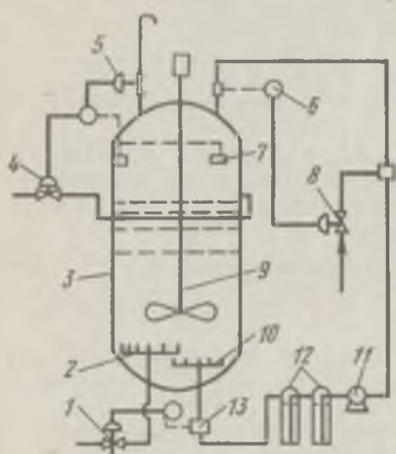
Рис. 32. Ферментатор барботажного типа с мешалкой:
