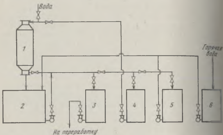
Рис. 50. Схема отбора сульфитного щелока ступенчатым способом:
