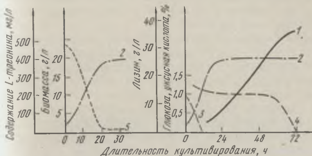
Рис. 107. Динамика накопления L -лизина (1), биомассы (2) и изменения компонентов питательной среды (3 — глюкоза; 4 — уксусная кислота; 5 — L -треонин при культивировании Brevibacterium 22Л на средах, содержащих уксусную кислоту).
