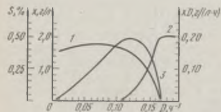
Рис. 94. Влияние скорости разбавления D на концентрацию клеточной биомассы x (1), метилового спирта S (2) и продуктивность xD (3).
