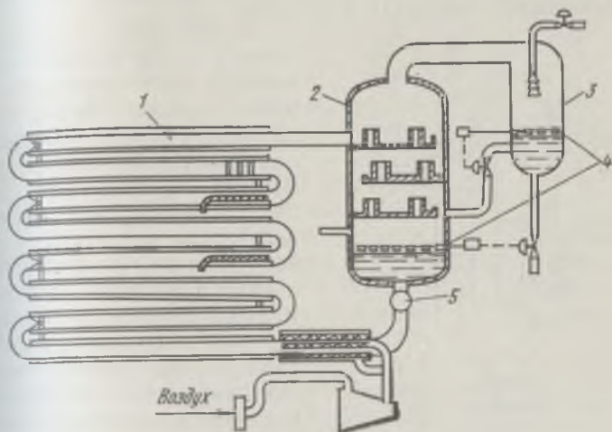
Рис. 25. Ферментатор с выносным теплообменником:
