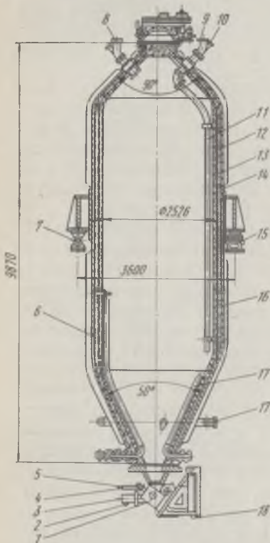
Рис. 44. Гидролиз-аппарат:
