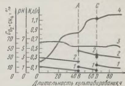
Рис. 89. Динамика роста культуры, изменения величины pH, потребления метана и кислорода при введении свежей смеси метана и воздуха (AB и CD) в фазе логарифмического роста культуры:
