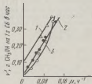
Рис. 95. Зависимость удельной скорости потребления метилового спирта от удельной скорости роста дрожжей (1) и бактерий (2, 3).
