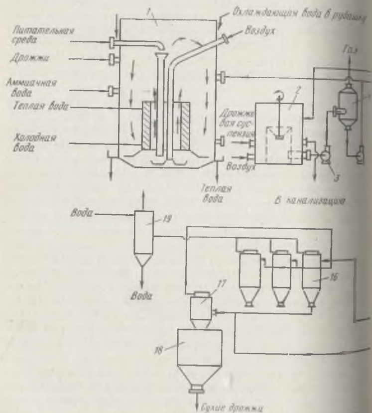
Рис. 41. Аппаратурно-технологическая схема стадий выращивания, выделения и сушки дрожжей.
