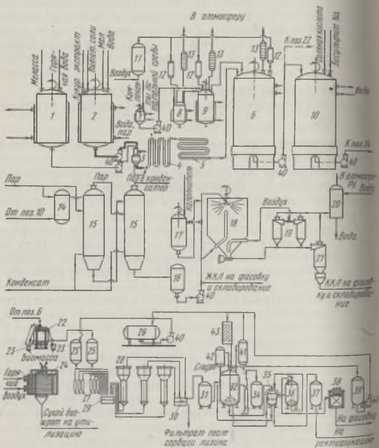
Рис. 117. Аппаратурно-технологическая схема производства лизина.
