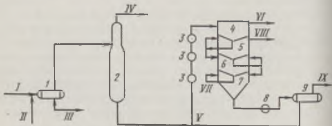
Рис. 68. Схема депарафинизации дизельного топлива водно-спиртовым раствором карбамида:
