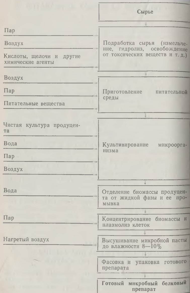
Схема 1 Основные стадии процесса производства микробных белковых препаратов
