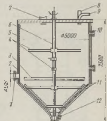
Рис. 47. Нейтрализатор с коническим дном:
