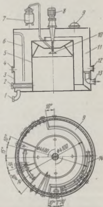
Рис. 34. Двухступенчатый флотатор:
