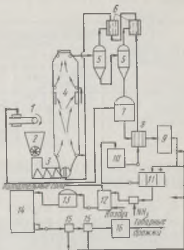
Рис. 59. Технологическая схема получения белковых препаратов при культивировании микроорганизмов на продуктах щелочного расщепления древесины:
