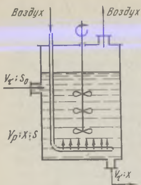
Рис. 9. Схема материальных потоков в непрерывно действующем аппарате полного смешения.
