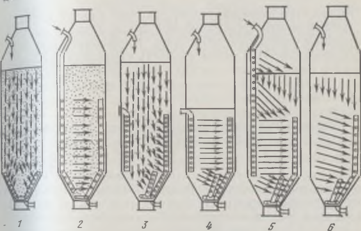
Рис. 45. Схемы расположения фильтрующих устройств в гидролиз-аппаратах:
