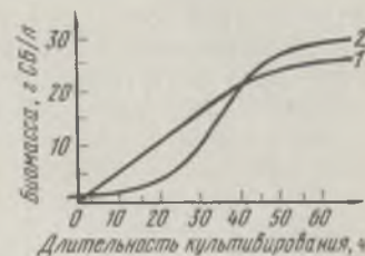
Рис. 30. Накопление биомассы в процессе культивирования микроорганизмов на n -парафинах в ферментаторах:
