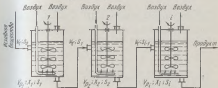
Рис. 17. Схема материальных потоков в однопоточной батарее непрерывно действующих аппаратов полного смешения для получения биомассы микроорганизмов.
