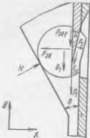
Рис. 7.42. Схема для определения усилия прижатия P_{3n} в овощерезке с вертикальным опорным диском
