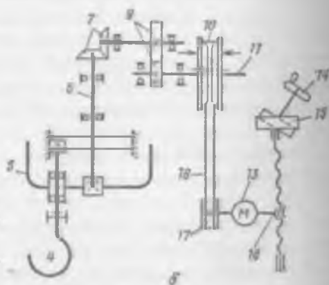
Рис. 8.10. Взбивальная машина MB-6: а — общий вид; б — кинематическая схема
