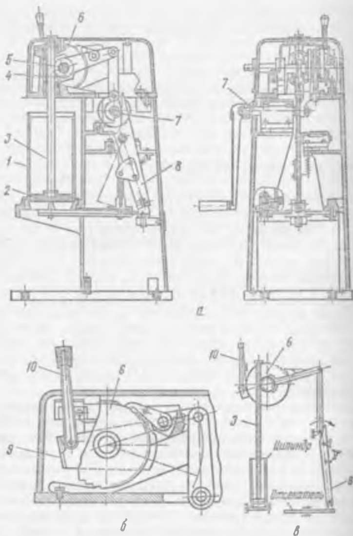
Рис. 9.5. Ручной делитель масла РДМ-5:
