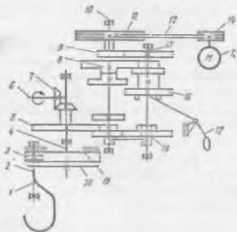
Рис. 8.13. Кинематическая схема взбивальной и перемешивающей машины ИН-40, ИН-60 («Савария» производство ВНР)
