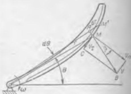
Рис. 7.31. Схема к определению коэффициента скольжения для криволинейного ножа
