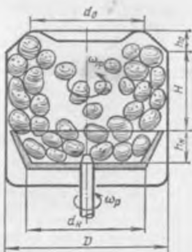
Рис. 5.8. Схема расположения продукта при работе конусной картофелеочистительной машины
