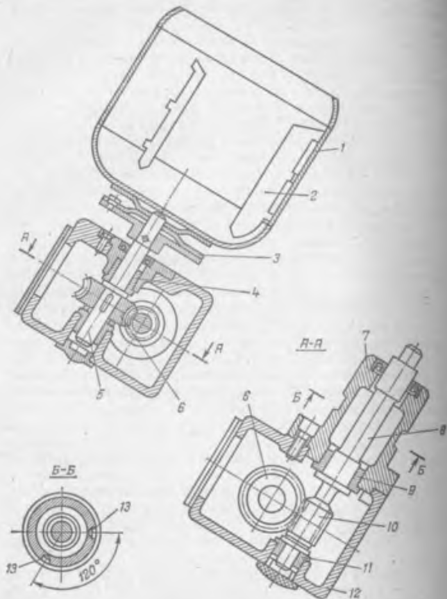
Рис. 8.3. Механизм МС25-200 для перемешивания овощей при приготовлении салатов и винегретов
