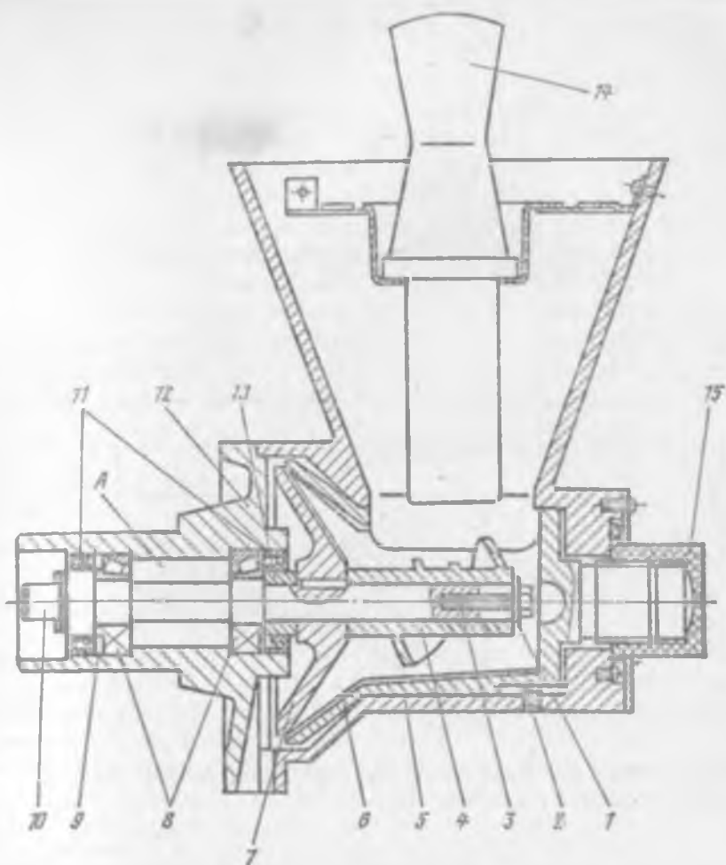
Рис. 6.2. Механизм для измельчения сухарей и специй МИП-II-1
