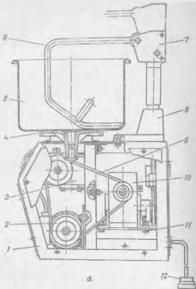
Рис. 8.5. Тестомесильная машина ТММ-60М:
