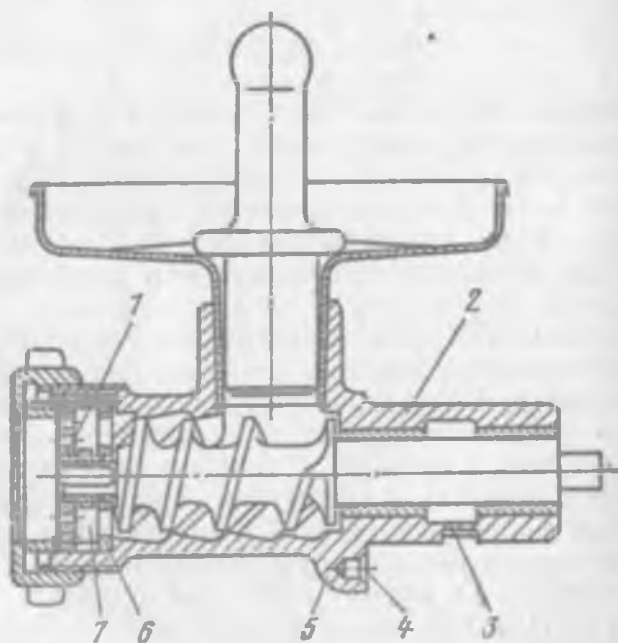
Рис. 7.54. Мясорубка УММ-2
