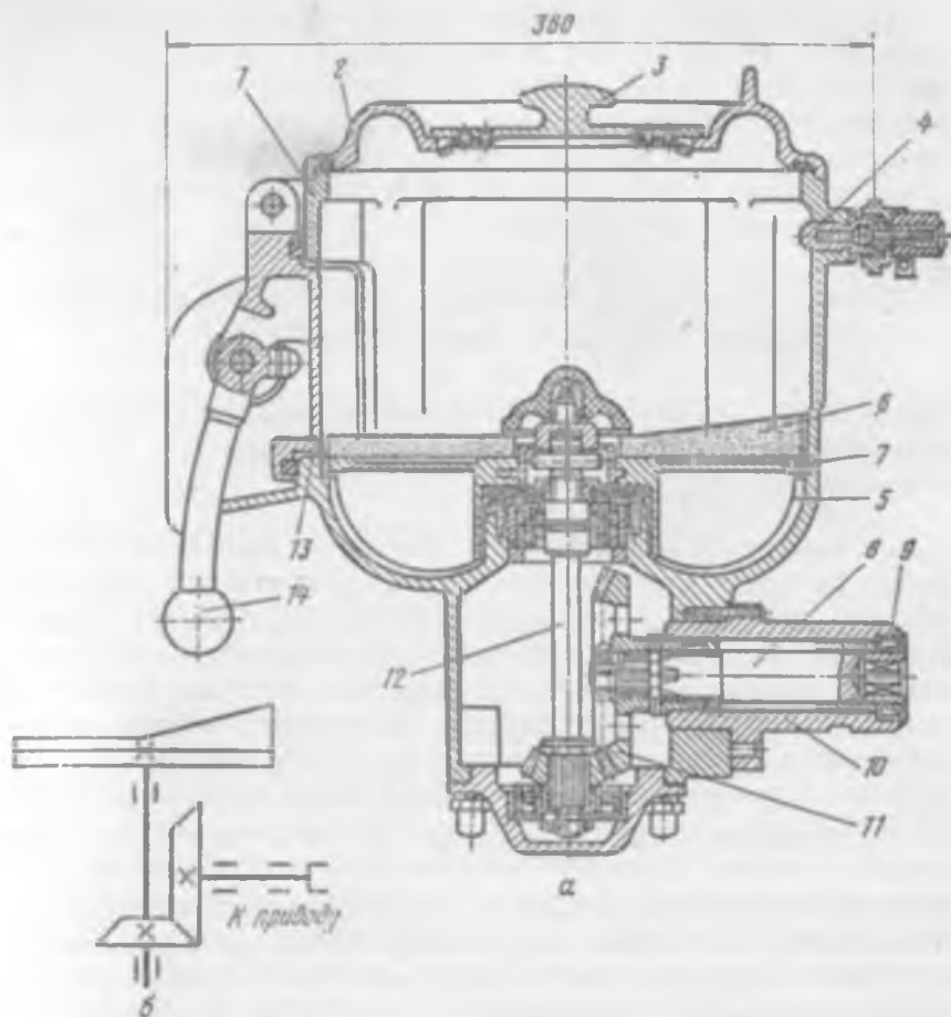
Рис. 5.6. Сменный картофелеочистительный механизм УММ-5: а — общий вид; б — кинематическая схема
