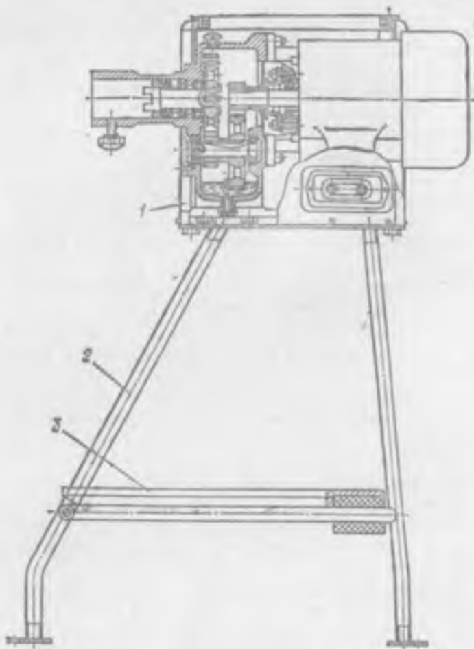
Рис. 2.2. Привод П 1 -0,6-1,1 на станине-подставке с выдвижным столом
