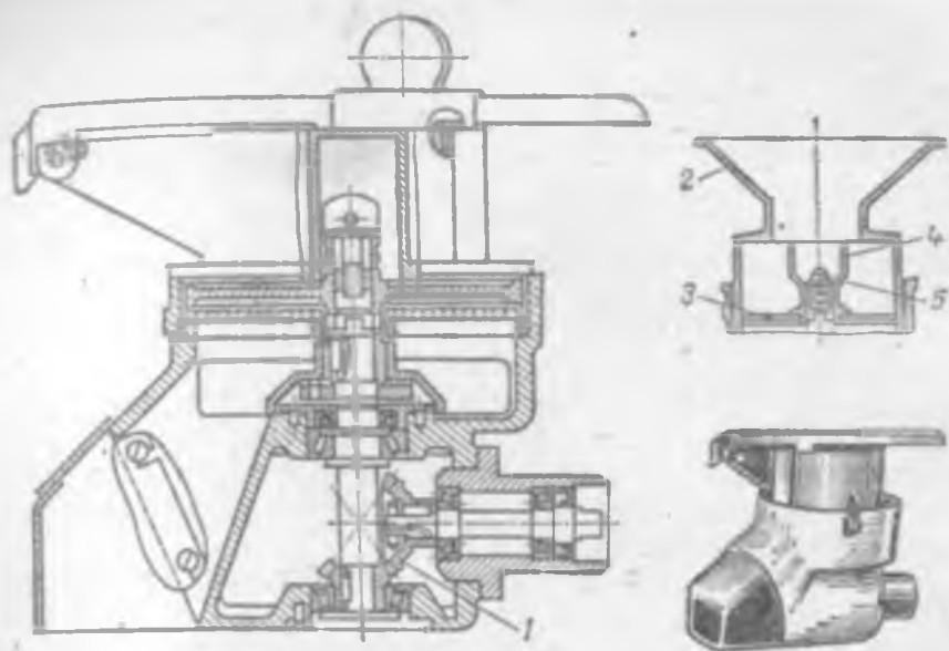
Рис. 6.11. Механизм МОП-II-1 с протирачным приспособлением
