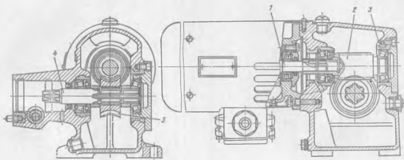
Рис. 2.4. Малогабаритный привод УММ-ПР
