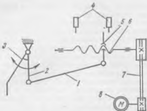
Рис. 5.5. Схема привода для открытия шибер загрузочного ковша
