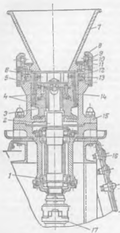
Рис. 6.8. Машина для тонкого измельчения вареных продуктов МИВР
