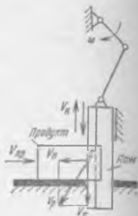
Рис. 7.12. Схема скользящего резания при поступательном движении продукта и возвратно-поступательном движении ножа
