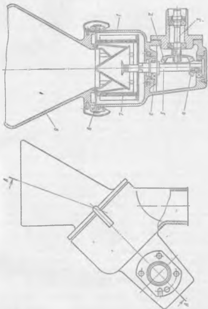
Рис. 3.2. Просеиватель МПП-11-1
