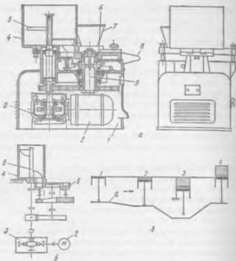
Рис. 9.1. Котлетоформовочная машина МФК-2240:
