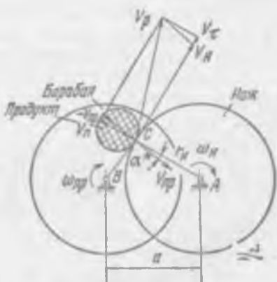
Рис. 7.17. Схема скользящего резания при вращательном движении продукта и дискового ножа
