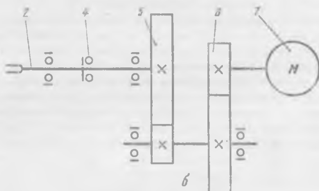
Рис. 2.1. Привод П 1 -0,6-1,1: а — общий вид; б — кинематическая схема
