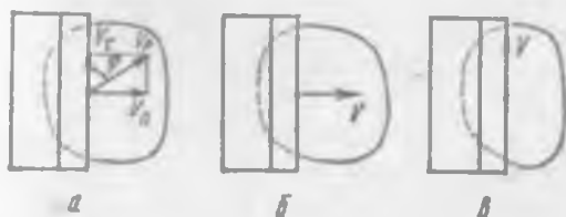
Рис. 7.3. Схема относительного перемещения ножа и продукта:
