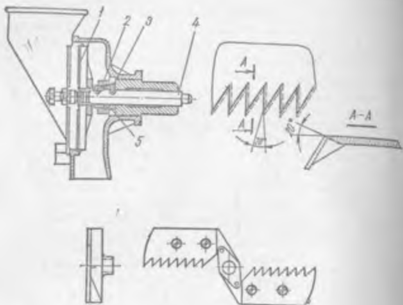
Рис. 7.38. Овощерезательный механизм 822-10
