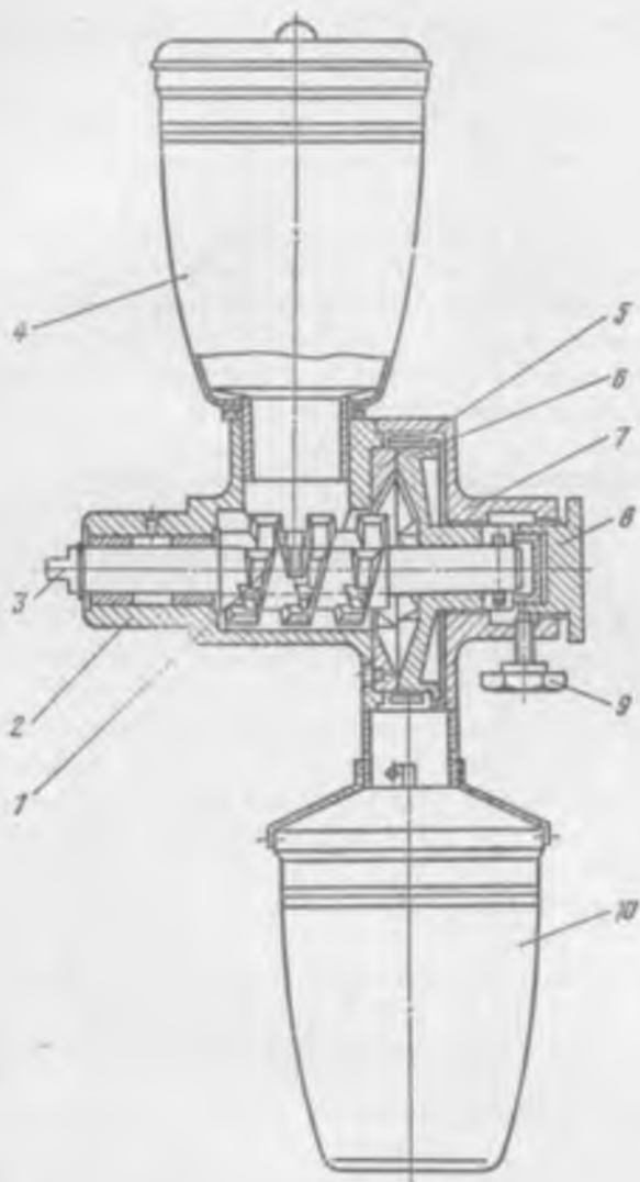
Рис. 6.5. Механизм для размола кофе МКК-120
