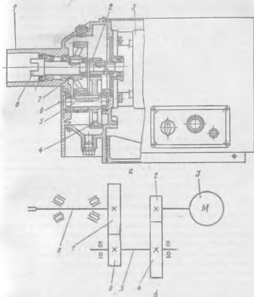
Рис. 2.3. Привод П-II:
