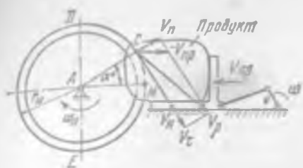
Рис. 7.15. Схема скользящего резания при возвратно-поступательном движении продукта и вращательном движении дискового ножа
