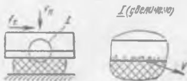
Рис. 7.5. Схема скользящего резания
