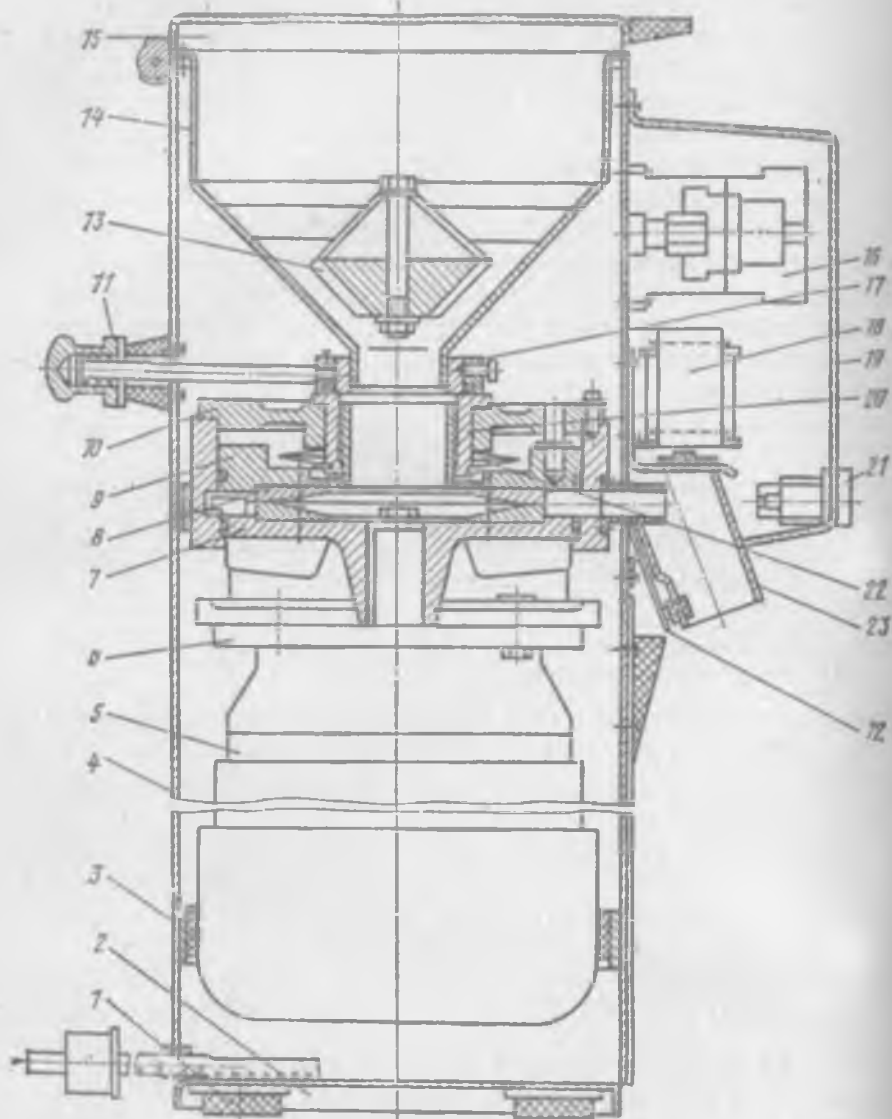
Рис. 6.4. Кофемолка МИК-60
