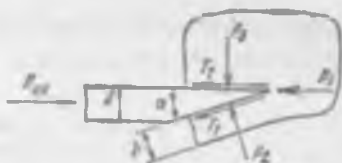
Рис. 7.20. Силы, действующие на нож при рубящем резании и свободном отгибании продукта
