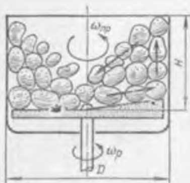
Рис. 5.10. Схема расположения продукта при работе дисковой картофелеочистительной машины
