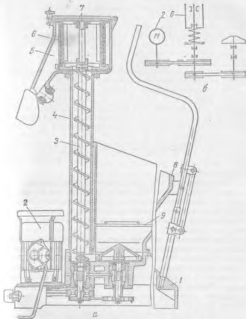
Рис. 3.3. Просенватель МПМ-800: а — общий вид; б — кинематическая схема
