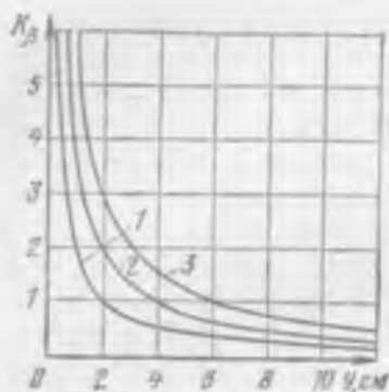
Рис. 7.30. Изменение коэффициента скольжения по длине прямолинейного лезвия:
