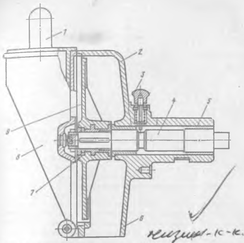
Рис. 7.37. Овощерезательный механизм УММ-10
