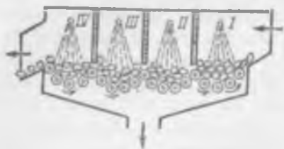
Рис. 5.14. Схема устройства картофелеочистительной машины непрерывного действия КНА-600М
