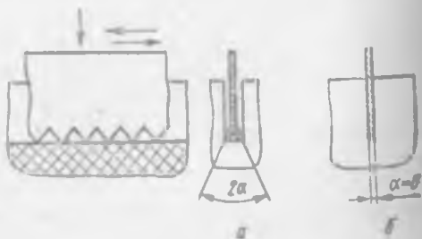
Рис. 7.2. Схема резания продукта пилой с разведенными зубьями: а — с отрицательным углом заточки; б — с углом заточки, равным 0
