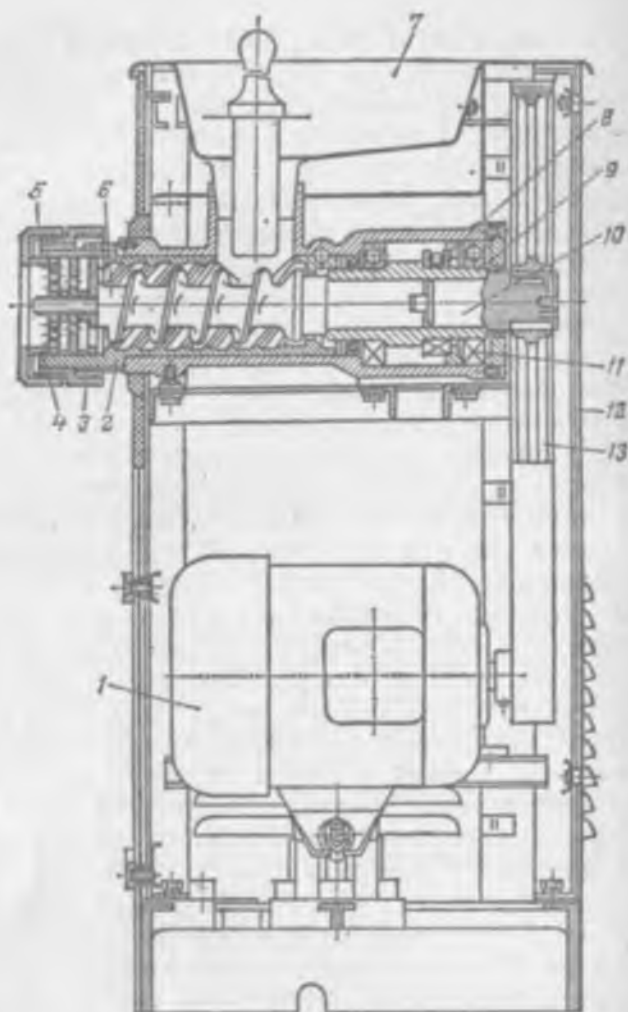
Рис. 7.50. Мясорубка МИМ-82М
