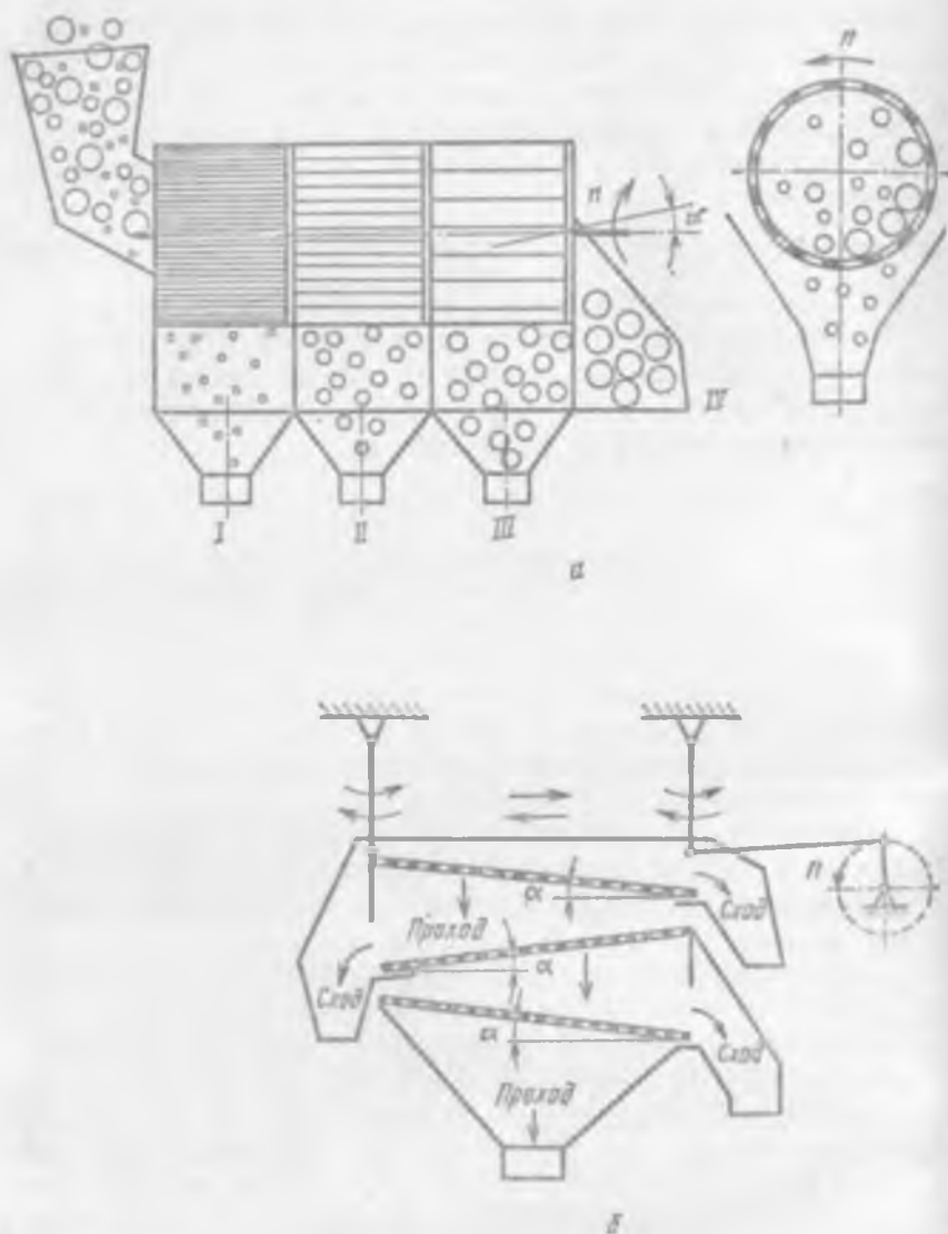
Рис. 3.1. Схемы сортировочно-калибровочных устройств: а — барабанное многосекционное сортировочное устройство; б — много- ярусное просеивающе сортировочное устройство с плоскими ситами
