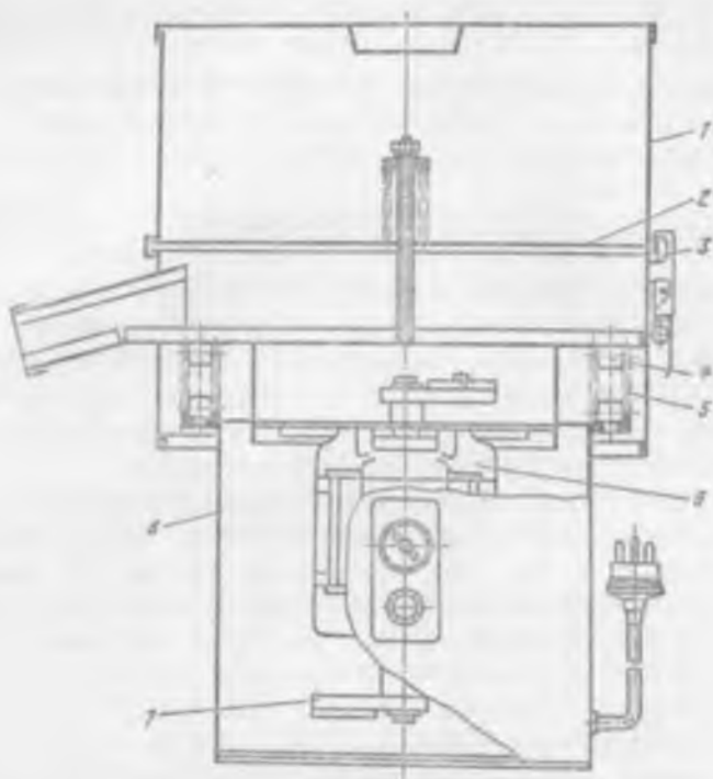
Рис. 3.4. Просеиватель МПМВ-300
