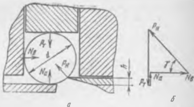
Рис. 7.41. Схема удержания продукта с помощью толкателя:
