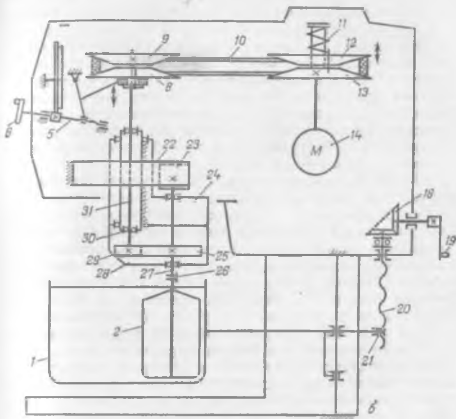
Рис. 8.12. Вибивальная машина МВ-35(2М):
