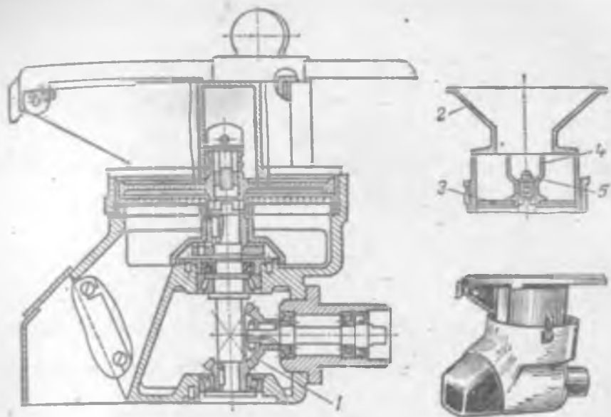
Рис. 6.11. Механизм МОП-II-1 с протирачным приспособлением
