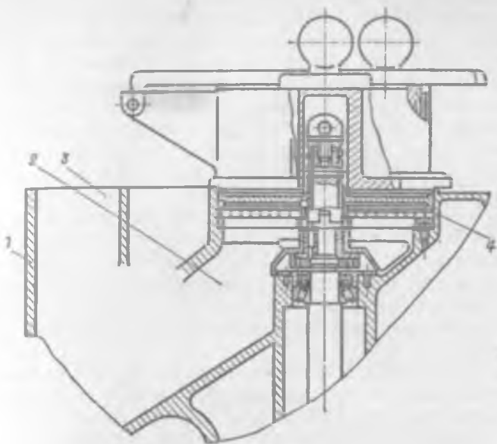
Рис. 7.35. Универсальная овощерезательная машина МРО 400-1000
