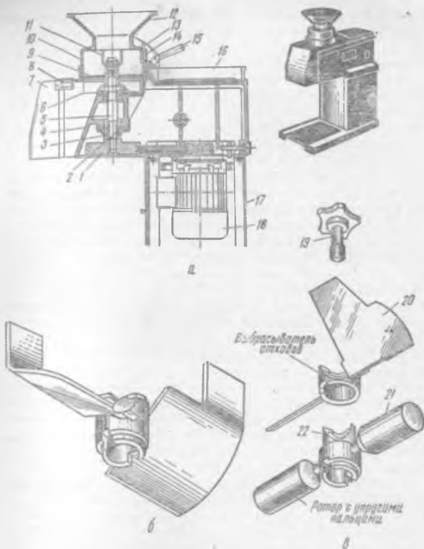
Рис. 6.9. Протирочная машина МП-800:
