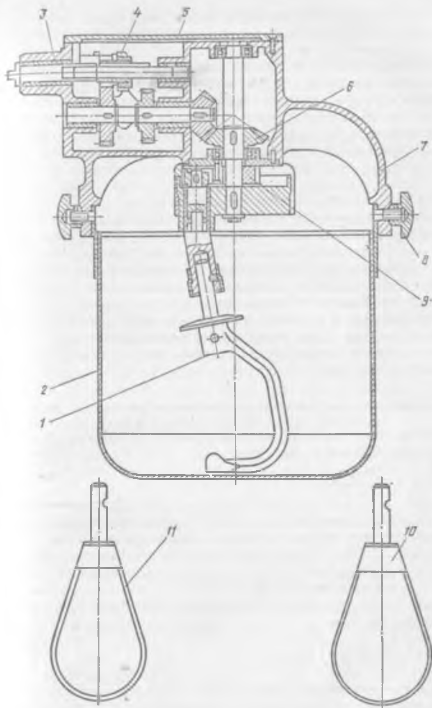
Рис. 8.15. Механизм взбивальный и перемешивающий МКР-25 (производство ПНР) к универсальному приводу
