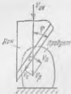
Рис. 7.9. Схема скользящего резания при поступательном движении прямолинейного ножа
