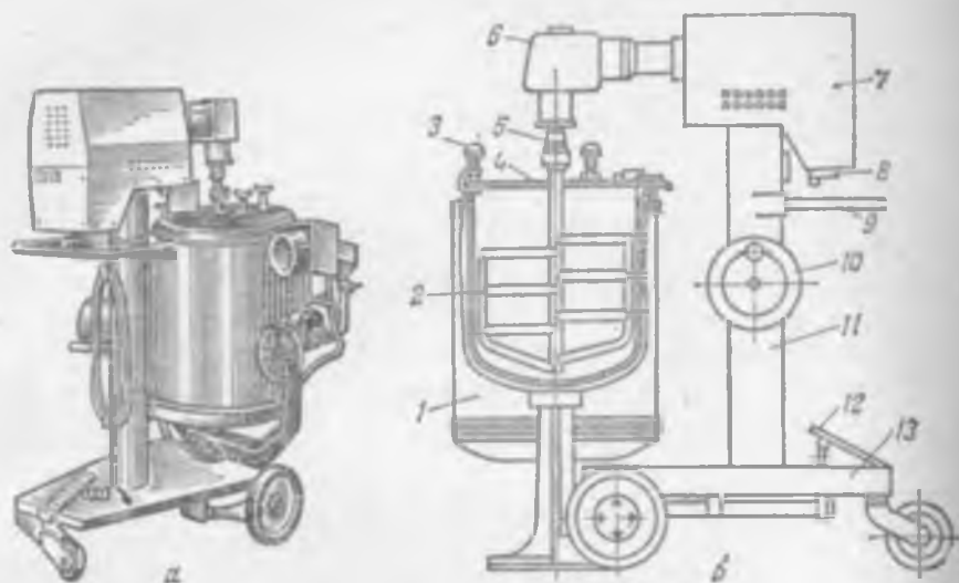
Рис. 6.14. машина для протирання картофеля в варочном котле МКП-60:
