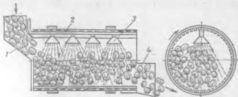
Рис. 4.2. Схема мытья овощей в барабанной овощемоечной машине
