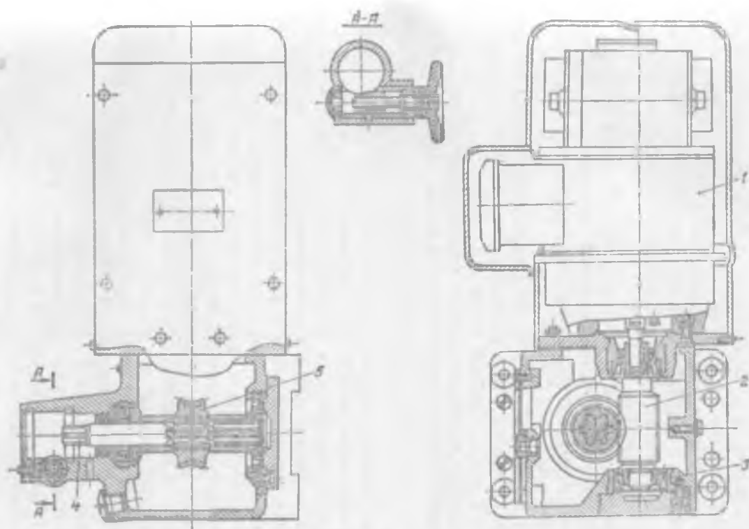
Рис. 2.5. Малогабаритный привод УММ-ПС
