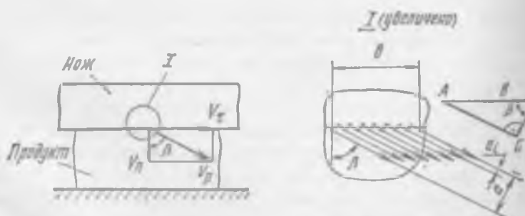
Рис. 7.23. Схема определения эффективной длины лезвия
