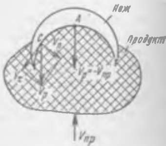
Рис. 7.14. Схема скользящего резания при поступательном движении продукта и неподвижном криволинейном ноже
