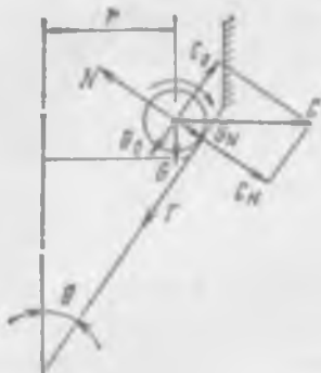
Рис. 5.12. Силы, действующие на клубень, находящийся на конической части рабочего органа
