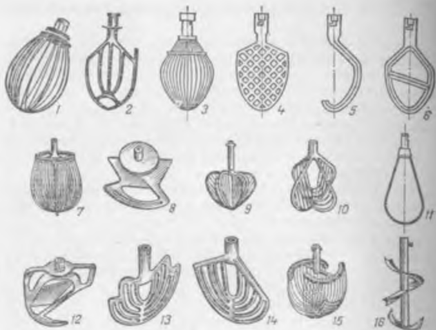
Рис. 8.9. Взбиватели для приготовления кондитерских смесей к взбивальным машинам с вертикальной осью вращения
