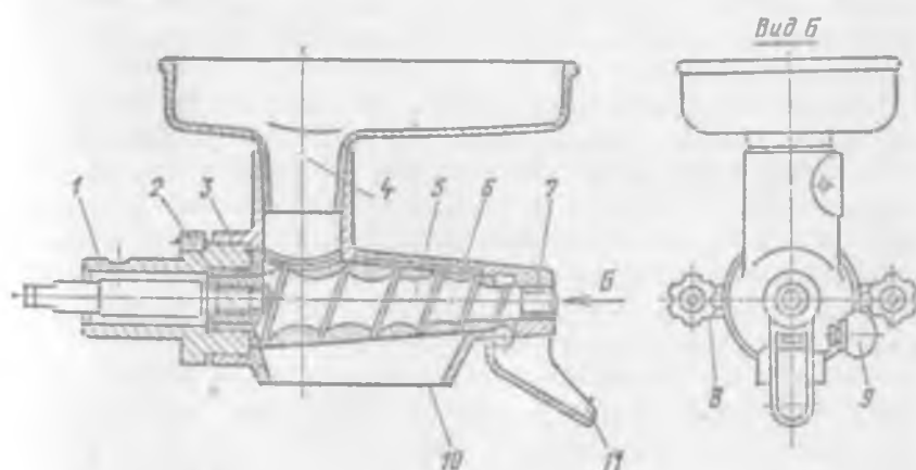
Рис. 10.1. Соковыжималка МСЗ-40
