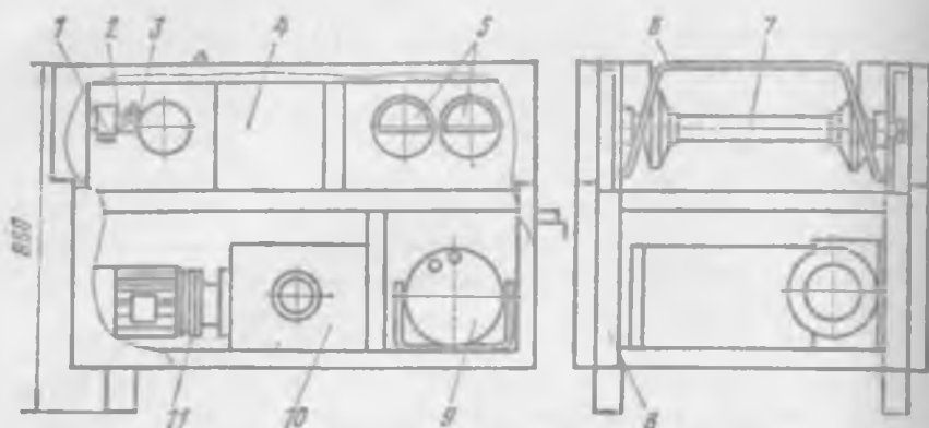
Рис. 4.12. Приводная секция машины ММУ-2000
