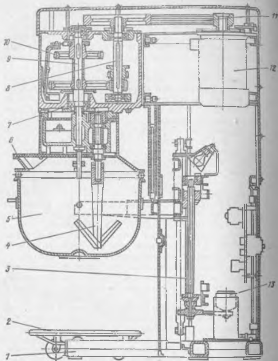
Рис. 8.8. Машина интенсивного замеса МТИ-100: а — общий вид; б — кинематическая схема
