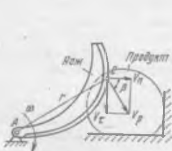
Рис. 7.13. Схема скользящего резания при вращательном движении криволинейного ножа
