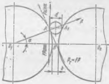
Рис. 6.7. Расчетная схема механизма МС 12-40
