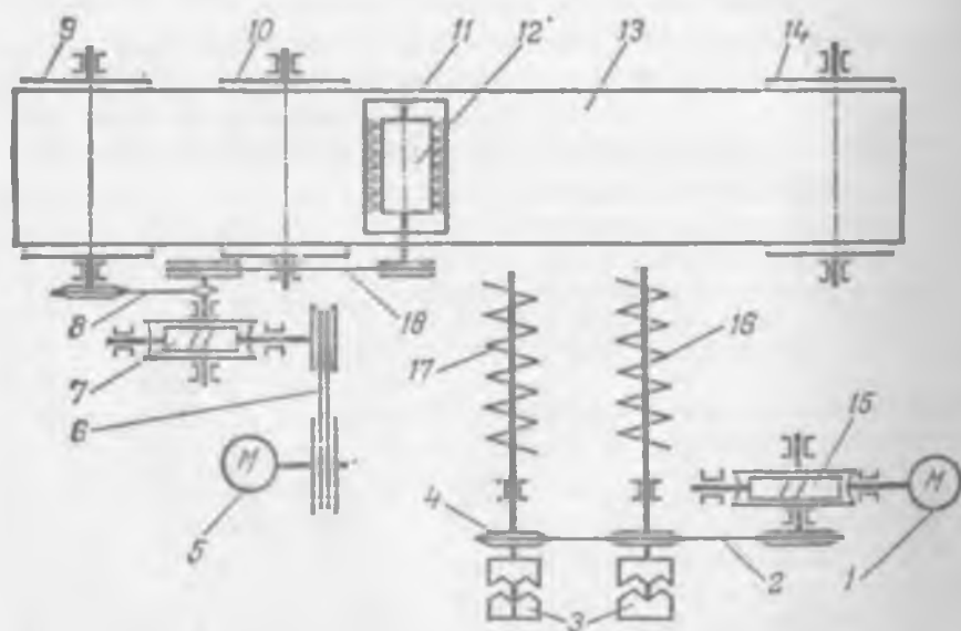
Рис. 9.2. Кинематическая схема варенично-пельменной машины
