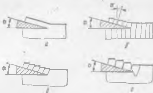
Рис. 7.4. Схема деформации различных продуктов при рубящем резании:
