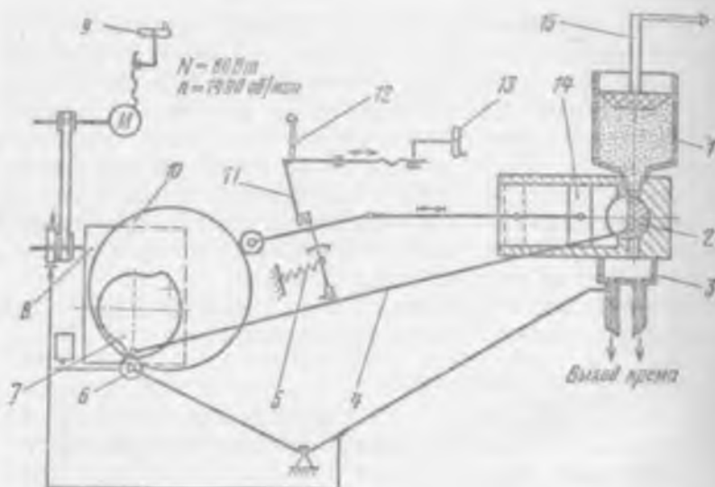
Рис. 9.6. Кинематическая схема дозатора крема ДК
