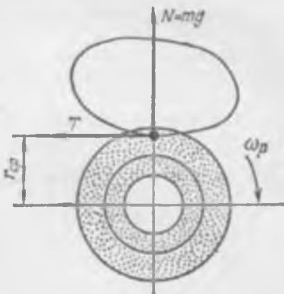
Рис. 5.17. Силы, действующие на клубень, находящийся на роликовом рабочем органе
