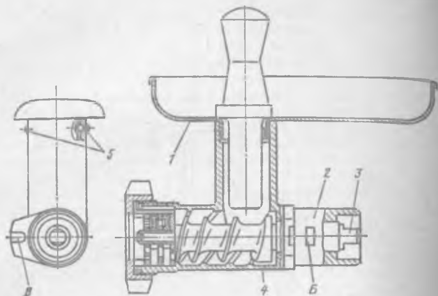
Рис. 7.53. Мясорубка ММП-II-1
