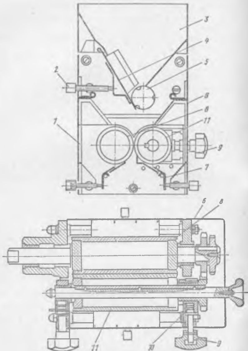
Рис. 6.6. Механизм МС 12-40 для дробления и растирания мака
