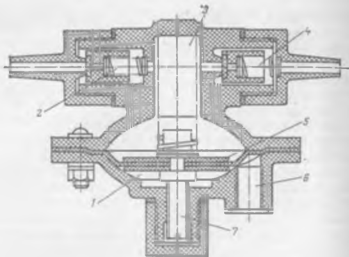
Рис. 4.7. Дозатор моющего средства
