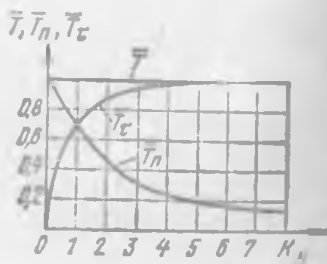
Рис. 7.27. Зависимость сопротивления трению от коэффициента скольжения
