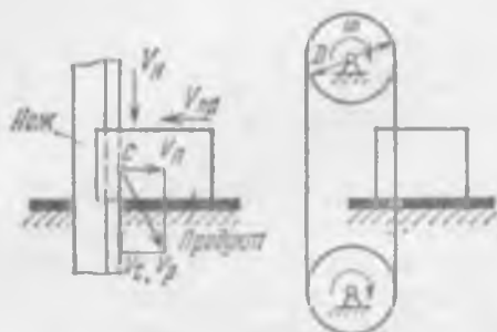
Рис. 7.11. Схема скользящего резания при поступательном движении продукта и ножа
