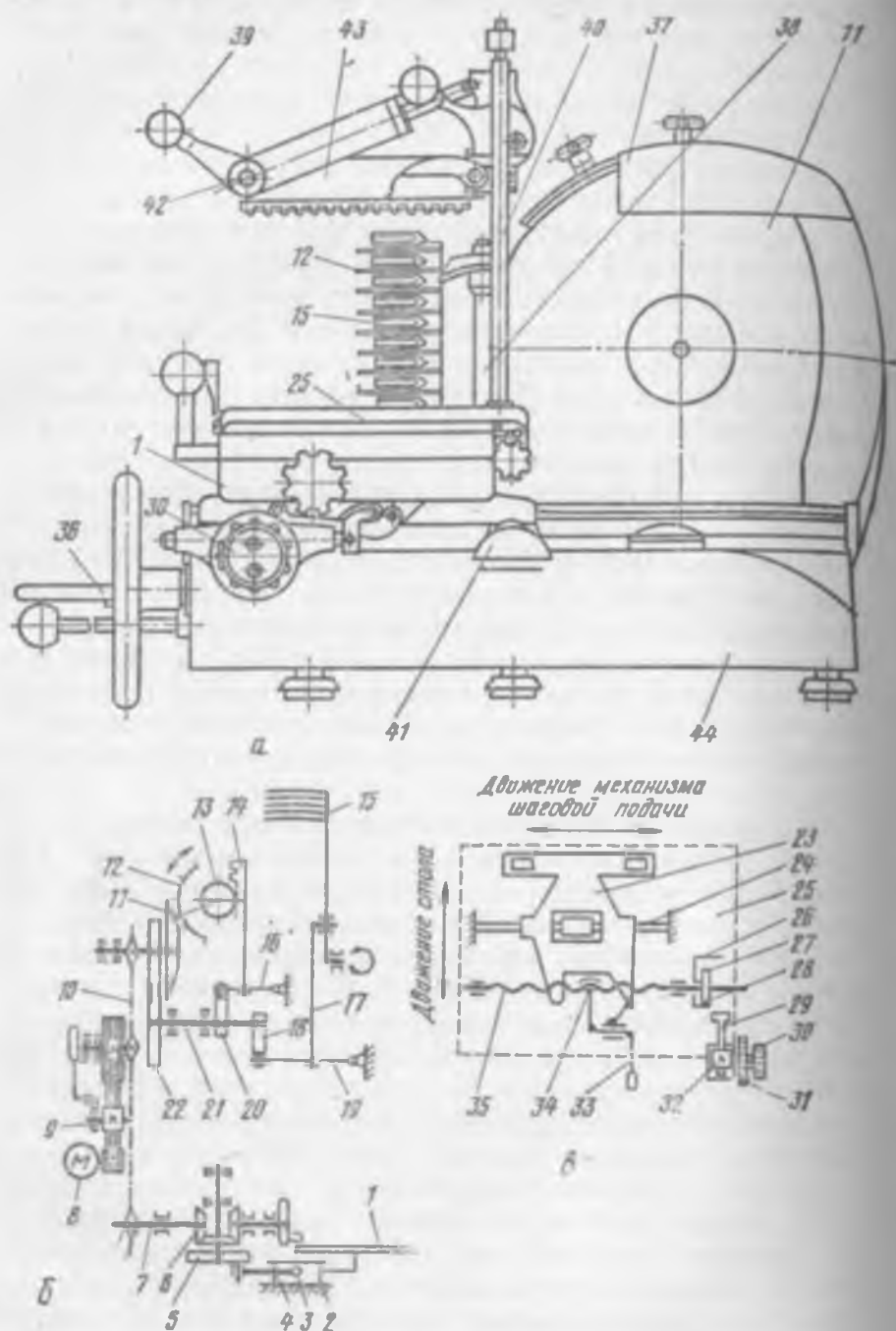
Рис. 7.63. Машина МРГУ-370 для нарезки гастрономических товаров:
