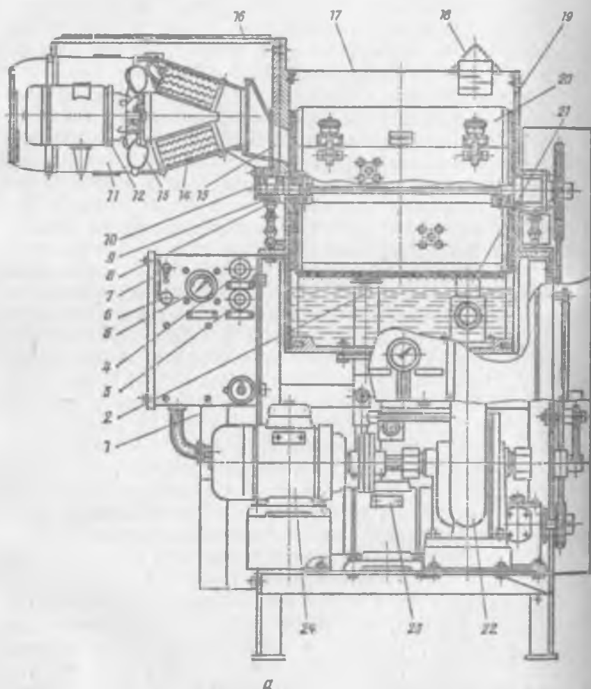
Рис. 4.10. Машина для мытья столовых приборов ММП-4000:
