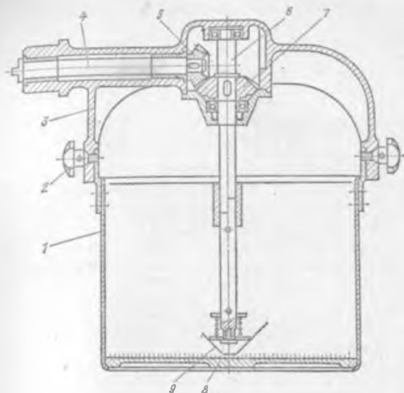
Рис. 6.12. Механизм для протирания сусов МКЗ-20 (производство ИИР) к универсальному приводу
