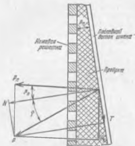
Рис. 7.55. Схема воздействия последнего витка шнека на продукт
