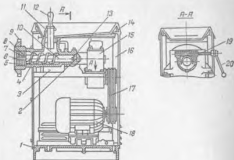
Рис. 7.49. Мясорубка МИМ-500
