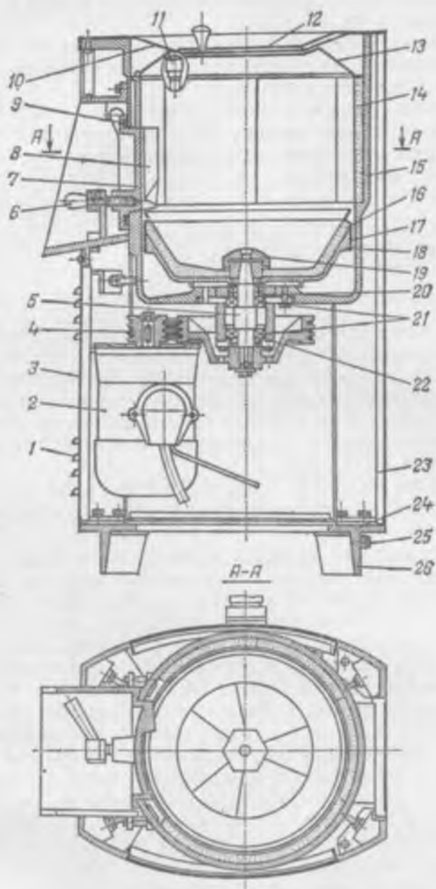
Рис. 5.2. Картофелеочистительная машина МОК-250
