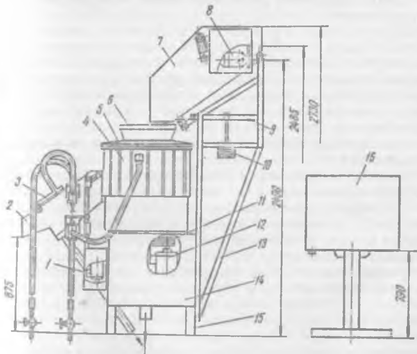
Рис. 5.4. Картофелеочистительная машина МОК-1200
