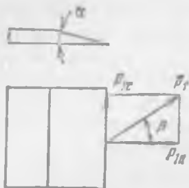
Рис. 7.24. Схема разложения сопротивления перерезанию при скользящем резании
