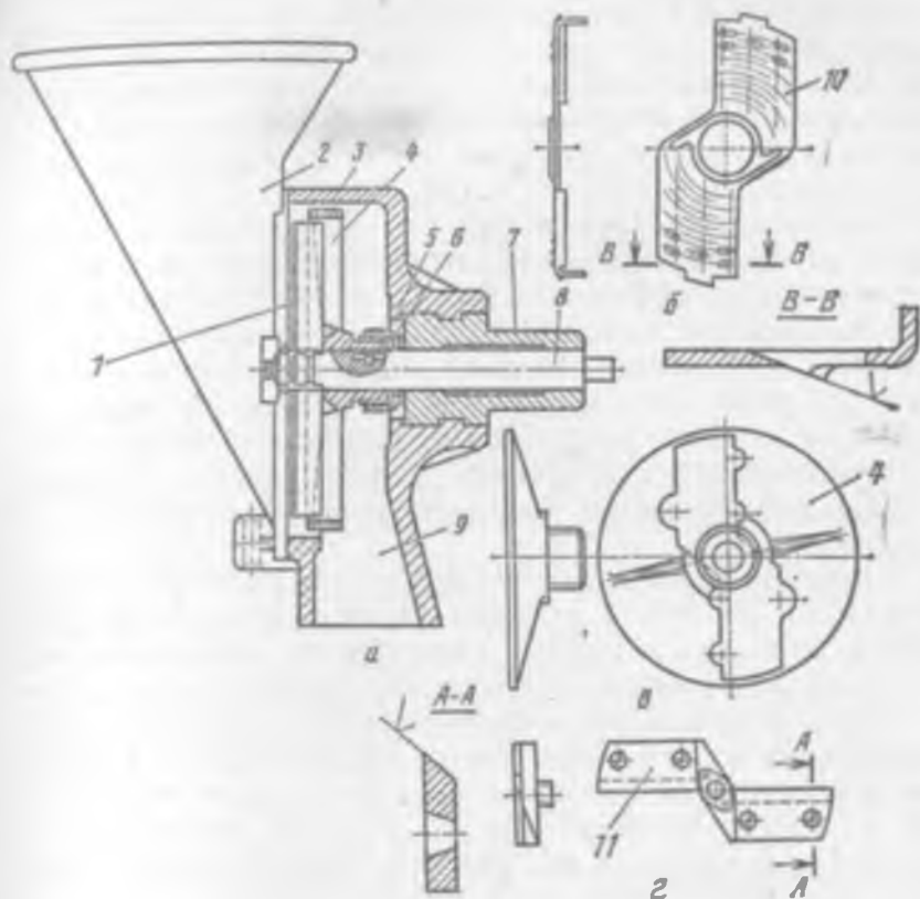
Рис. 7.36. Овощерезательный механизм МС 10-160:
