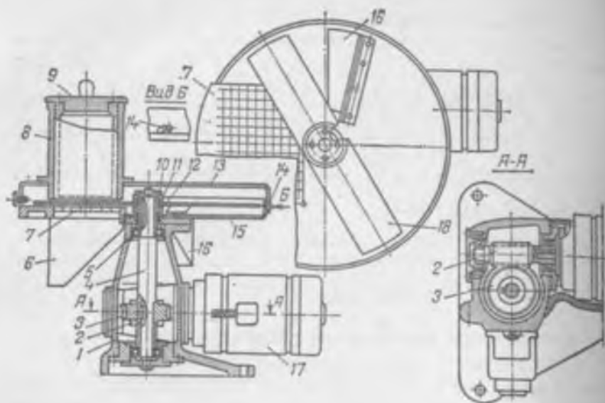
Рис. 7.45. Машина МРОВ-160 для нарезки вареных овощей
