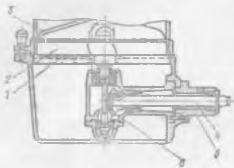
Рис. 6.10. Протирачный механизм МУ-1000 (модель 723-7М)
