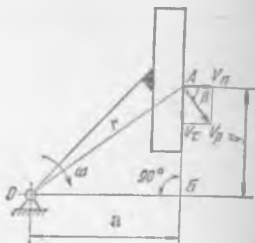
Рис. 7.29. Схема к определению коэффициента скольжения по длине прямолинейного лезвия
