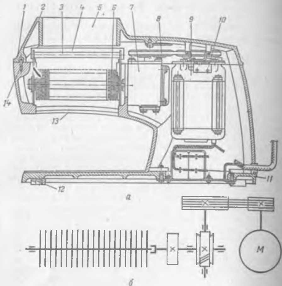
Рис. 7.56. Мясорыхлитель МРМ-15: а — общий вид; б — кинематическая схема
