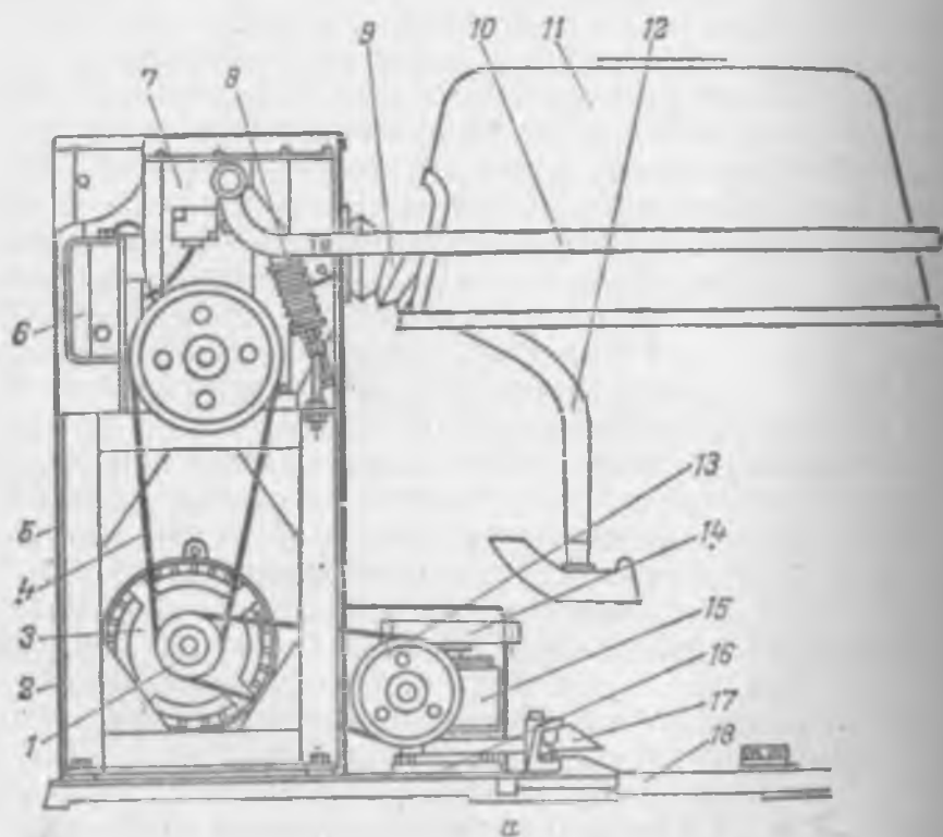
Рис. 8.6. Тестомесильная машина «Тасема»: а — общий вид; б — привод месильного рычага
