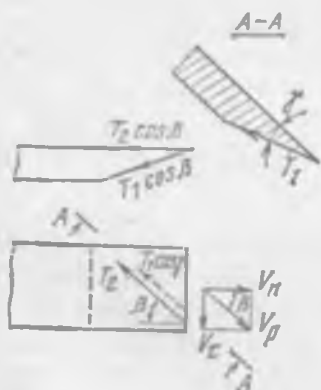
Рис. 7.26. Схема сопротивления трению при скользящем резании
