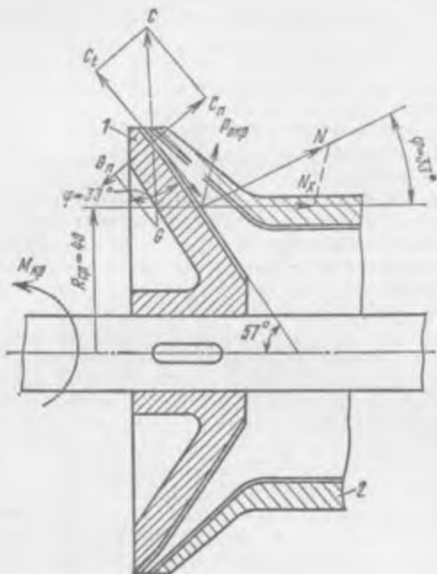
Рис. 6.3. Расчетная схема мелющих органов механизма МС 12-15
