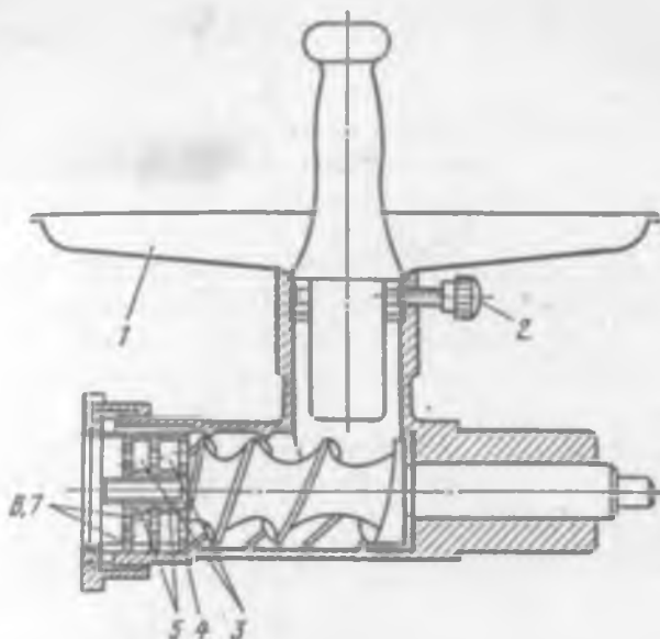
Рис. 7.52. Мясорубка МС2-70
