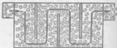
Рис. 5.15. Схема движения продукта в картофелеочистительной машине непрерывного действия (вид сверху)
