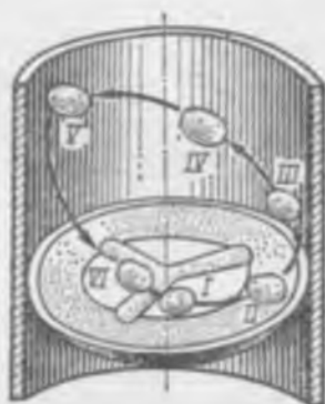
Рис. 5.9. Схема движения клубня в конусной картофелеочистительной машине
