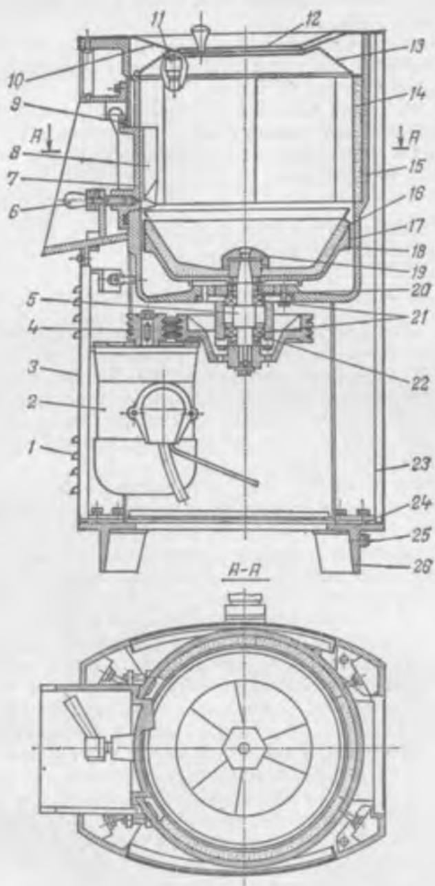
Рис. 5.2. Картофелеочистительная машина МОК-250
