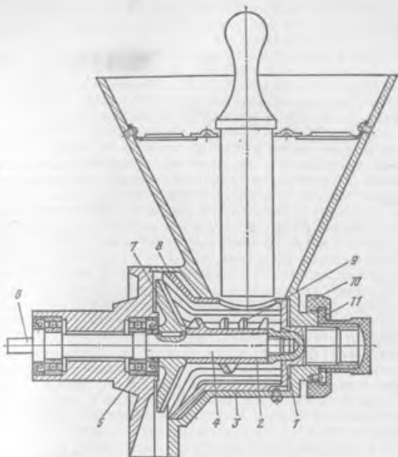
Рис. 6.1. Размолочный механизм МС 12-15
