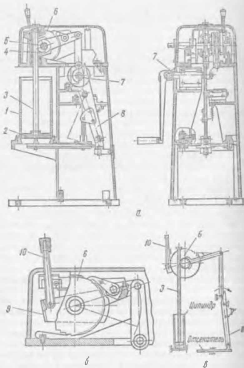
Рис. 9.5. Ручной делитель масла РДМ-5: а, б — общий вид; в — кинематическая схема
