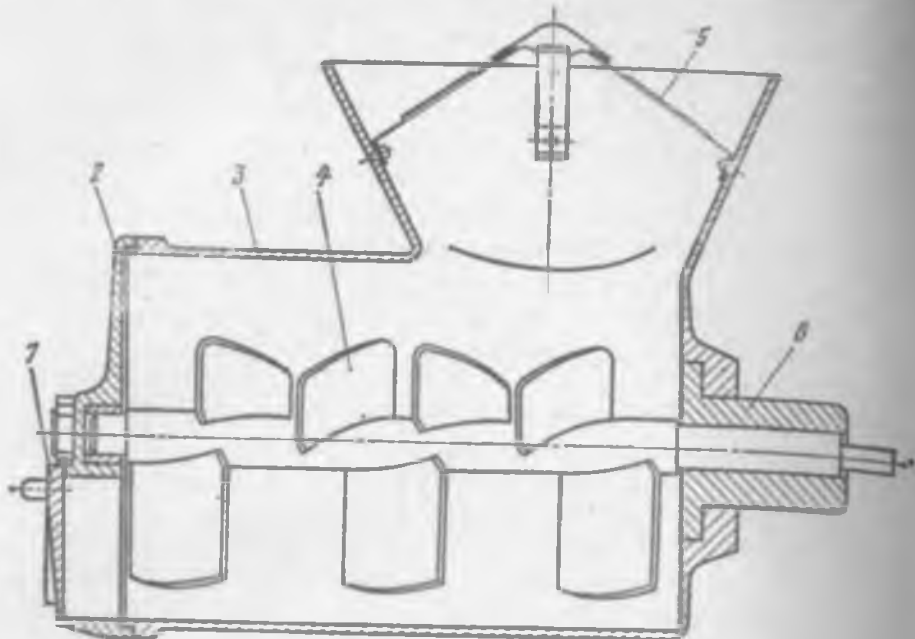
Рис. 8.1. Фаршемешалка МС8-150
