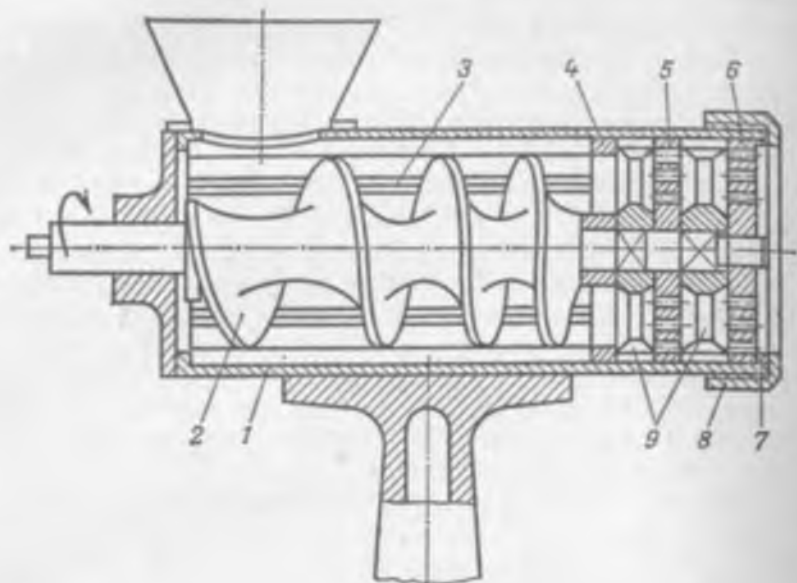
Рис. 7.47. Принципиальная схема мясорубки
