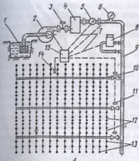
39-rasm. Tomchilatib sug'orish tizimining sxemasi: 1 – suv olish uzel; 2 – bosim hosil qiluvchi uzel; 3 – bosh surma klapan; 4 – filtr; 5 – suv o'lchash qurilmasi; 6 – manometr; 7 – aloqa liniyalari; 8 – o'g'itlarni aralastirgich-uzatgich; 9 – magistral quvur; 10 – taqsimlash quvuri; 11 – masofadan turib boshqariluvchi surma klapan; 12 – sug'orish quvurlari; 13 – suv chiqargich-tomchilatgich; 14 – sug'orish muqarrarligini aniqlovchi datchik; 15 – boshqarish pulti.
