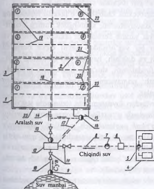
58-rasm. Oqova va zovur suvlari qayta ishlatiladigan maxsus sug'orish tizimlarining sxemasi:
