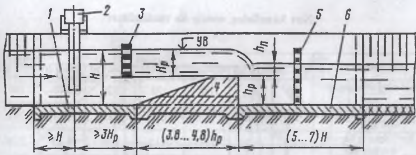
61-rasm. SANIIRI ning suv o'lchash ostona: 1, 6 – kanalning betonlashirilgan qismi; 2 – sath o'lchagich; 3, 5 – o'lchov reykalari; 4 – ostona.
