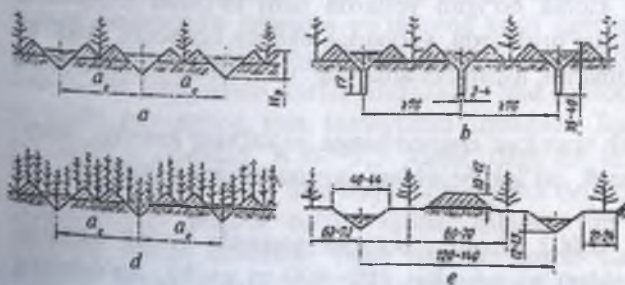
17-rasm. Sug'orish egatlari: a – qator oralari chopiq qilinadigan ekinlarni sug'orishda; b – ekin ekiladigan; d – tubi tirqishli; e – terrasali; a c – qator orasining kengligi. (O'lchovlar sm hisobida).
