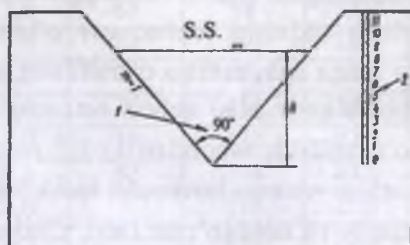
65-rasm. 90^\circ li BT–90 Tomson suv o'lchagichi: 1 – 90^\circ li burchak; 2 – suv o'lchash reykasi; h – suv qatlami qalinligi, m; s.s. – suv sathi.
