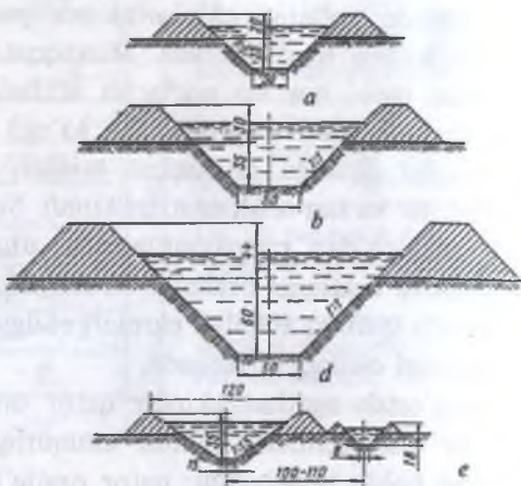
50-rasm. Turli xil ariqqazgich-tekislagichlar bilan muvaqqat tarmoqlar olinganda ariqning ko'ndalang kesimi o'lchamlari (sm hisobida): a - K3Y-0,3; b - K3Y-0,5; d - KOP-500A; e - KBH-0,35 (o'lchovlar m hisobida).
