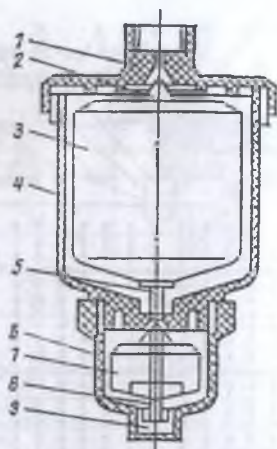
41-rasm. Uzgi provodhoz-2 suvchiqargich-tomchilatgichi: 1 — ustki qopqog; 2,5,8 — ninalar; 3 — suv bosimini pasaytiruvchi suzgich; 4 — ustki kamera korpusi; 5 — pastki kamera korpusi; 7 — suv sarfini ravonlashtiruvchi suzgich; 9 — nippel-suv chiqargich teshik.
