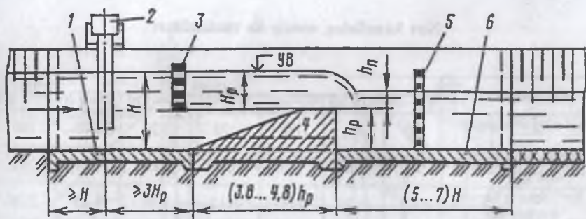
61-rasm. SANIIRI ning suv o'lchash ostonasi: 1, 6 – kanalning betonlashirilgan qismi; 2 – sath o'lchagich; 3, 5 – o'lchov reykalari; 4 – ostona.
