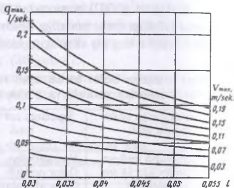
42-rasm. Egatning nishobligi ( i ) va egatdagi suv oqimining yo'l qo'yiladigan tezligi ( v_{\max} )ga bog'liq holda suv sarfini yo'l qo'yiladigan qiymati ( q_{\max} )ni hisoblash sxemasi.
