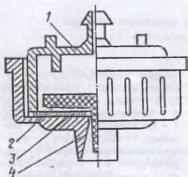
40-rasm. Moldaviya-1A mikrosuvchiqargich-tomchilatgichi: 1 — korpusi; 2 — drossel; 3 — shayba-qistirma; 4 — qopqog'i.
