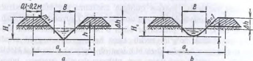
20-rasm. Egatlarning ko'ndalang kesimi: a — uchburchakli; b — trapetsiya-parabolik; B — egatning kengligi; a_e — qator orasining kengligi; H_e — egatning umumiy chuqurligi; h — egatning chuqurligi.
