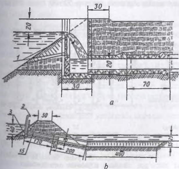
53-rasm. Sug'orish tarmog'idan cheklarga suv chiqargichlar: a — Kubanqishxo'jloyiha instituti konstruksiyasi; b — Janubsvxo'jloyiha instituti konstruksiyasi; 1 — shandorlar; 2 — qopqoq dastasi; 3 — qopqoq zatvori.
