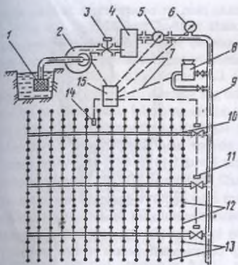
39-rasm. Tomchilatib sug'orish tizimining sxemasi: 1 – suv olish uze-li; 2 – bosim hosil qiluvchi uzel-li; 3 – bosh surma klapan; 4 – filtr; 5 – suv o'lchash qurilmasi; 6 – ma-nometr; 7 – aloqa liniyalari; 8 – o'g'it-larni aralash tirgich-uzatgich; 9 – ma-gistral quvur; 10 – taqsimlash quvu-ri; 11 – masofadan turib boshqarilu-vchi surma klapan; 12 – sug'orish quvurlari; 13 – suv chiqargich-tom-chilatgich; 14 – sug'orish muqarrar-ligini aniqlovchi datchik; 15 – bosh-qarish pulti.
