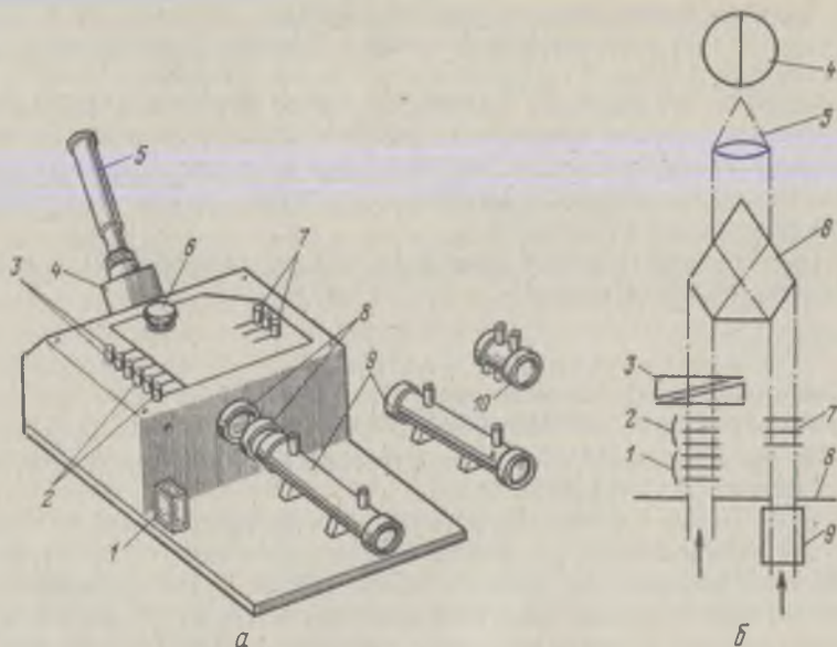
Рис. 9. Цветомер ВНИИЖ-16:
