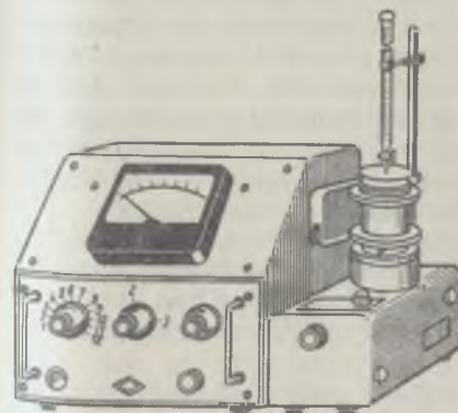
Рис. 25. Прибор для высокочастотного титрования
