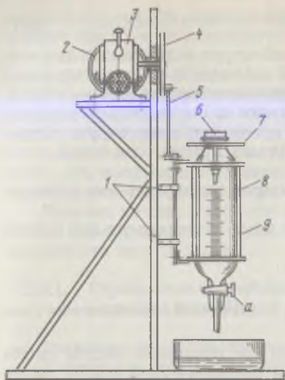
Рис. 29. Прибор ВНИИЖа для определения пенообразующей способности:
