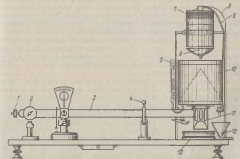
Рис. 15. Твердомер Каминского:
