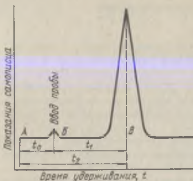
Рис. 17. Хроматограмма
