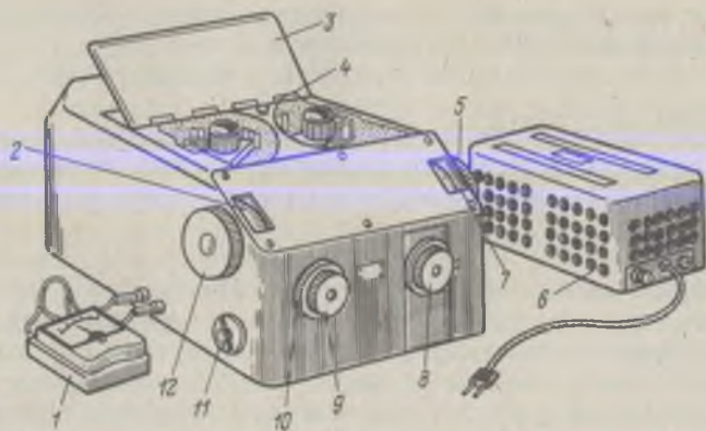
Рис. 16. Фотоэлектроколориметр ФЭК-М:
