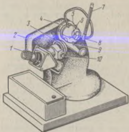
Рис. 14. Рефрактометр ИРФ-22:
