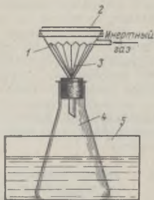
Рис. 11. Устройство для фильтрования масла:
