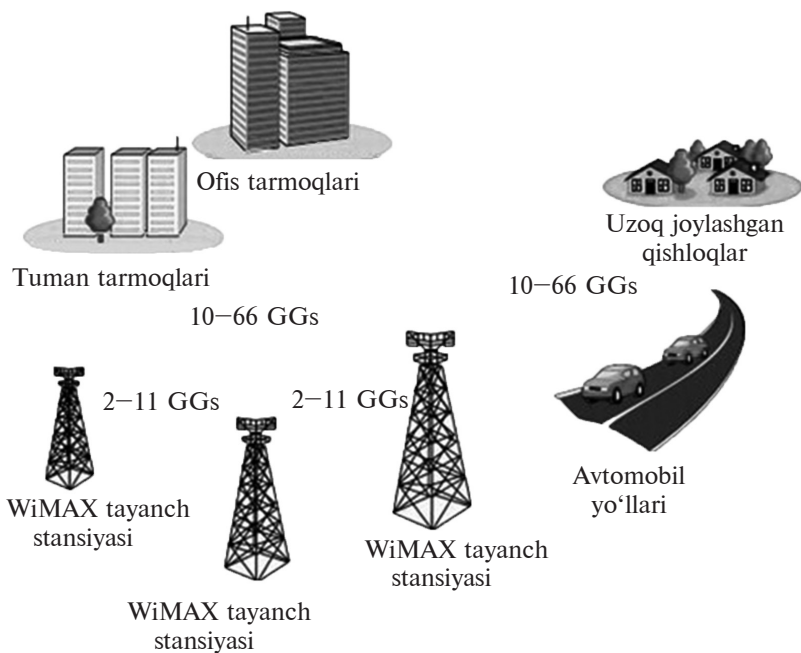
25.1-rasm. WiMAX tarmog'i topologiyasi.
