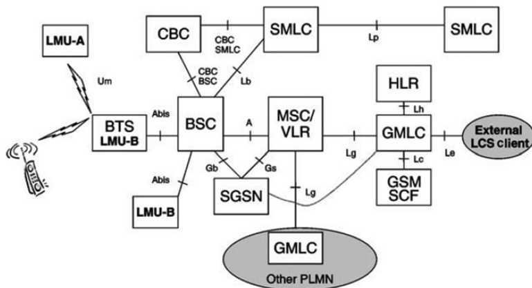
4.6-rasm. PBS arxitektura LVP.
