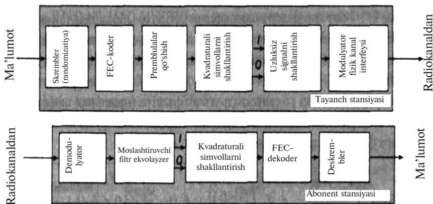
29.1-rasm. WirelessMAN-SC rejimida signalni qayta ishlash trakti.
