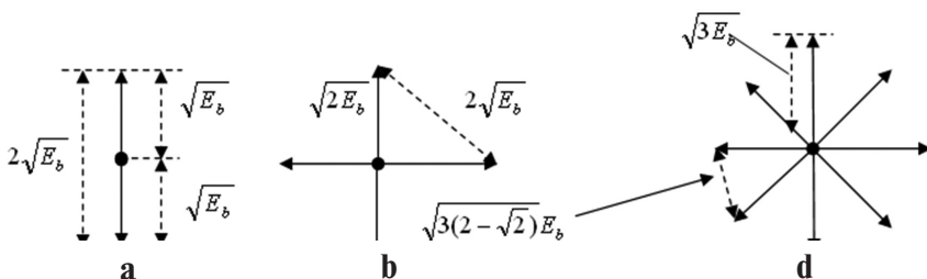
6.3-rasm. Fazali manipulyatsiyani geometrik izohlash.
