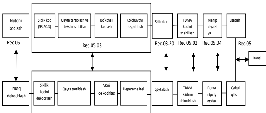
7.4-rasm. Radiotraktning tuzilish sxemasi.
