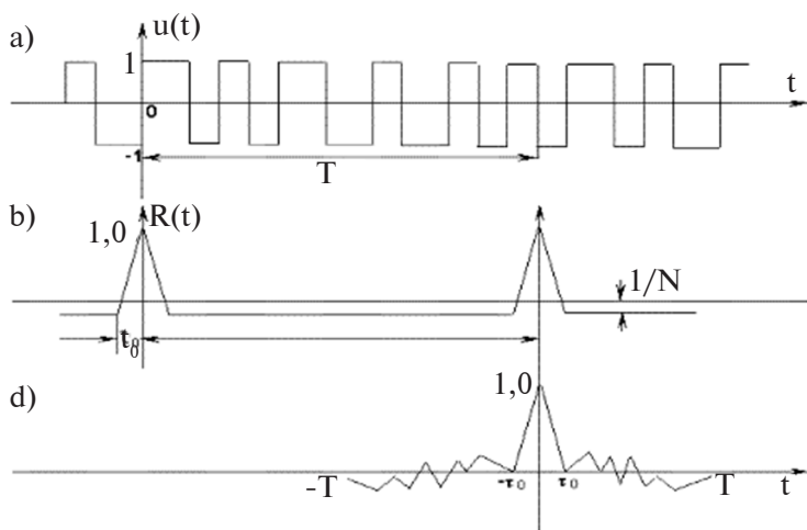
12.4-rasm. N=15 li M — ketma-ketlikning strukturasi (a), davriy AKF (b) va nodavriy AKF (d).
