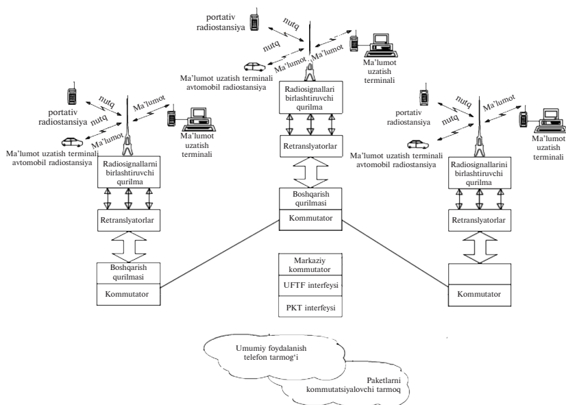
10.3-rasm. Markazlashtirilgan zonalararo kommutatsiyali trunking tizimning umumlashtirilgan strukturaviy sxemasi.
