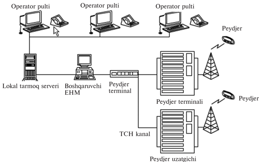
3.1-rasm. Peydjing stansiyasining tuzilish sxemasi.
