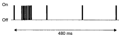
5.7-rasm. SACCH multifreymeni DTX rejimida quvvat o'zgarishi. Sinov jarayonida Samsung GT B3710 hamda Huawei E398 rusumli modemlardan foydalanildi.
