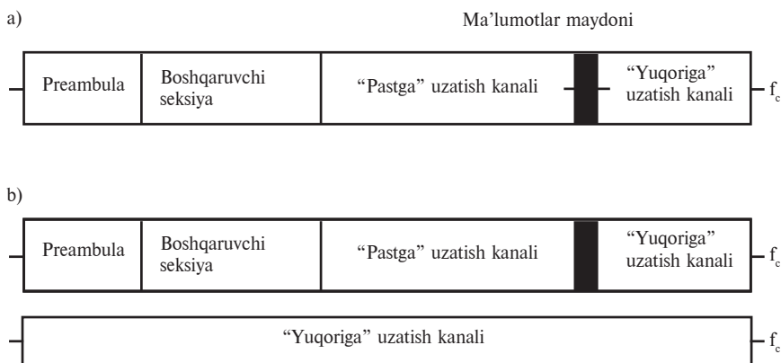
29.2-rasm. Kanallarni vaqtli (a) va chastotaviy (b) dublekslashli tizimlar uchun IEEE 802.16a standartidagi kadrlar tuzilmasi.
