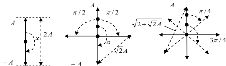
6.5-rasm. MCHM signalning kvadraturali tashkil etuvchilari.
