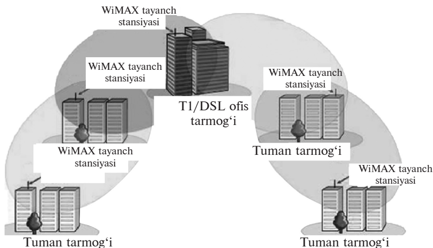
25.6-rasm. “Ko‘p nuqta-ko‘p nuqta” rejimidagi WiMAX tarmog‘ining topologiyasi.
