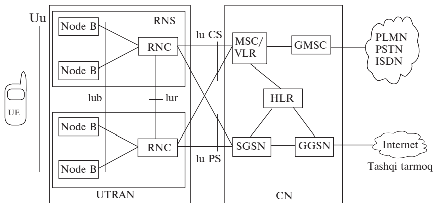
4.4-rasm. UMTS tizimlarining arxitekturası.
