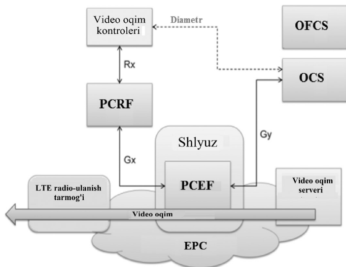
18.1-rasm. LTE tarmog‘ida RSS funksiyasini ishlash prinsipi (videokontent uzatish misolida).
