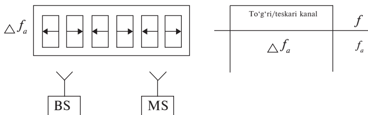
9.5-rasm. Vaqt bo'yicha dupleksli tarqoqlashni tashkillashtirish prinsipi.
