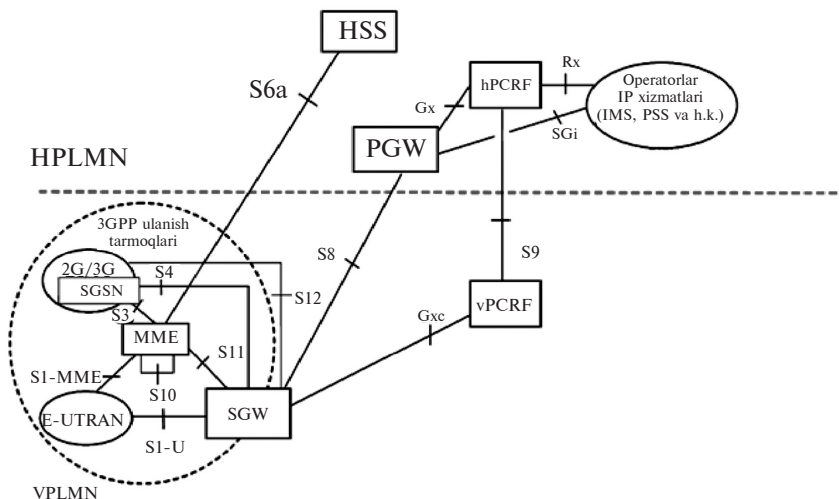
17.1-rasm. “Rouming” jarayonida LTE tarmoqlarining 3GPP tarmoqlari bilan PMIPv6 protokoli asosida o‘zaro hamkorligi.
