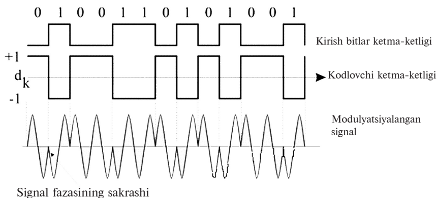
6.1-rasm. BFM (BPSK)ning ikkilik faza modulyatsiyasi.
