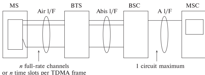
1.5-rasm. HSCSD tizimli arxetekturasi.
