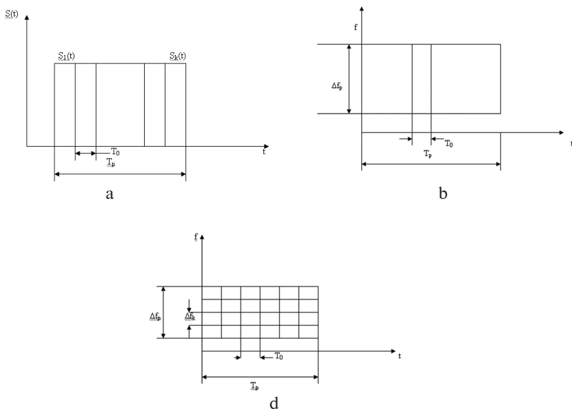
9.2-rasm. Kanal signallarining vaqt bo'yicha joylanishi (a), abonentlar orasidagi chastota va vaqt bo'yicha resursning taqsimlanishi (b), chastota va vaqt bo'yicha taqsimlanishlarning KCHAKF/KVAKF kombinatsiyasi (d).
