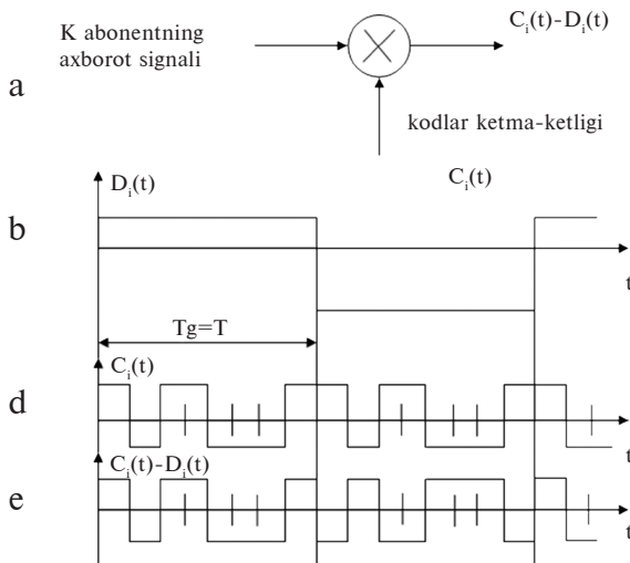
9.3-rasm. Raqamli ikkilik uzatish va binar PTK uchun to‘g‘ri-dan to‘g‘ri spektr kengaytirishning protsedurasi.
