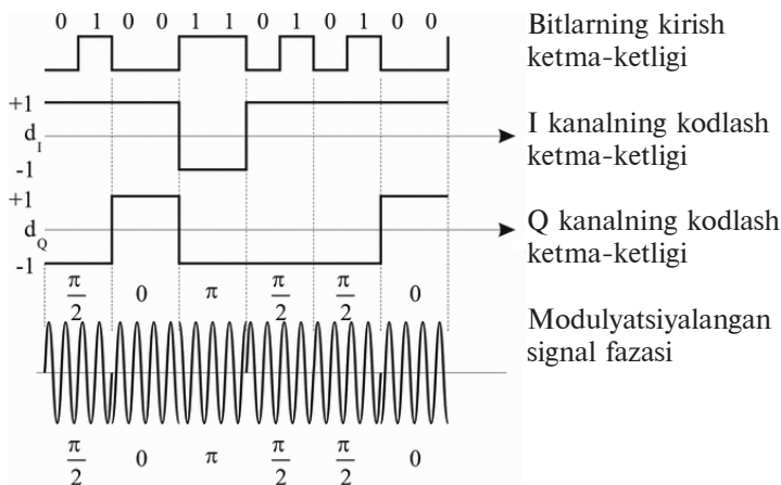
6.2-rasm. KFM (QPSK)ning kvadraturali faza modulyatsiyasi.
