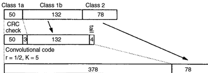
5.5-rasm. TCH/FS kodlash kanali.
