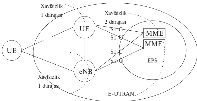
23.1-rasm. LTE tarmog'ida xavfsizlik darajalari.
