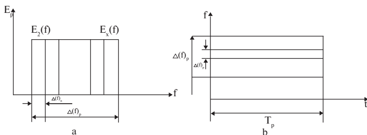
9.1-rasm. Kanal signallarining spektrlari (a) va chastotaning vaqt bo'yicha resursining abonentlar orasida taqsimlanishi (b).
