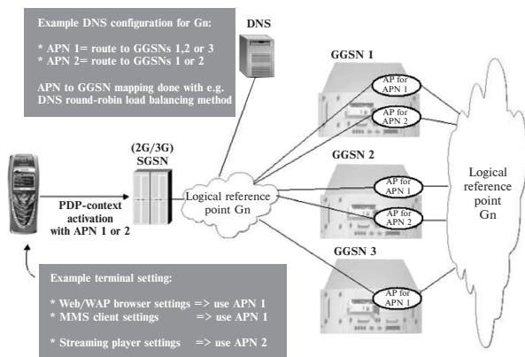
3.6- rasm. APNni DNSga bog’liqligi.
