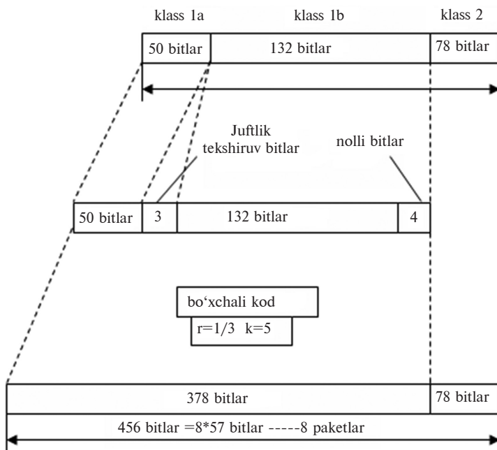
7.5-rasm. So'zlashuv kanalida kodlashtirishning umumlashtirilgan sxemasi.
