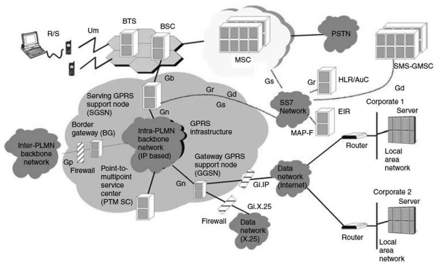
1.3-rasm. GPRSning funksiyonal ko‘rinishi.
