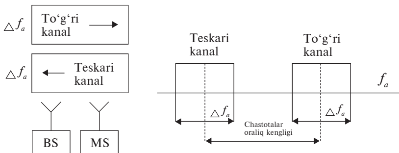
9.4-rasm. Chastotalarni dupeksli tarqoqlash prinsipida tashkillashtirish.
