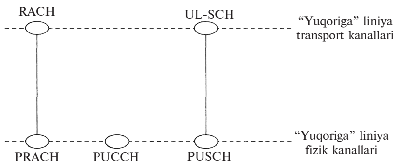
20.8-rasm. E-UTRAN tarmogʻida “yuqoriga” yoʻnalishdagi transport va fizik kanallarining oʻzaro taqsimlanishi.
