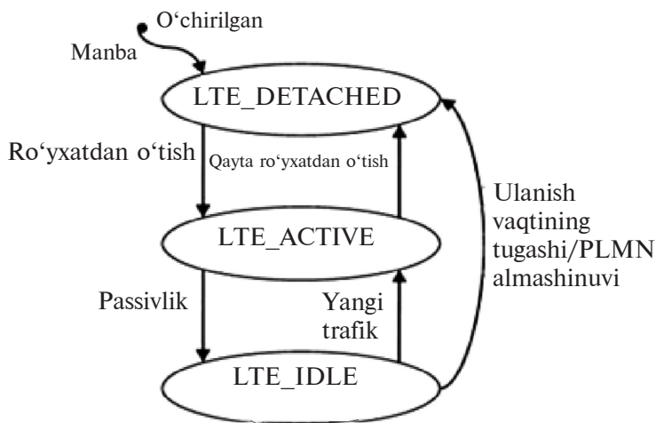
16.1-rasm. LTE tizimida A U ning mobillik holatlari.
