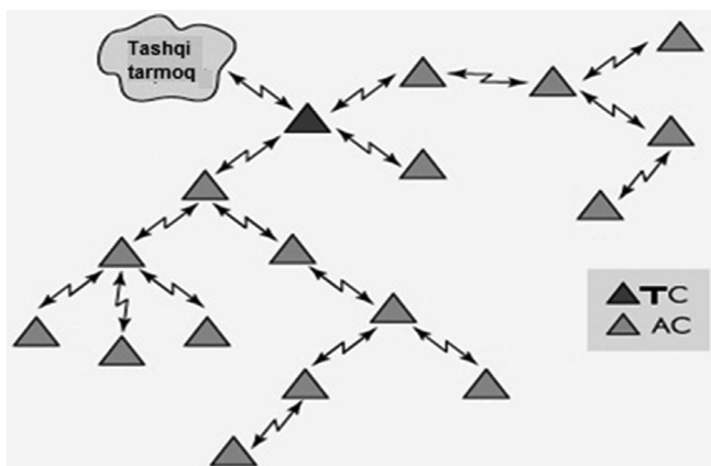
25.5-rasm. “Mesh” rejimida WiMAX tarmog‘i topologiyasi.
