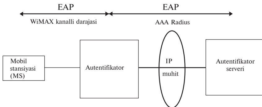
36.5-rasm. Ulanishni nazorat qilishning arxitekturasini.
