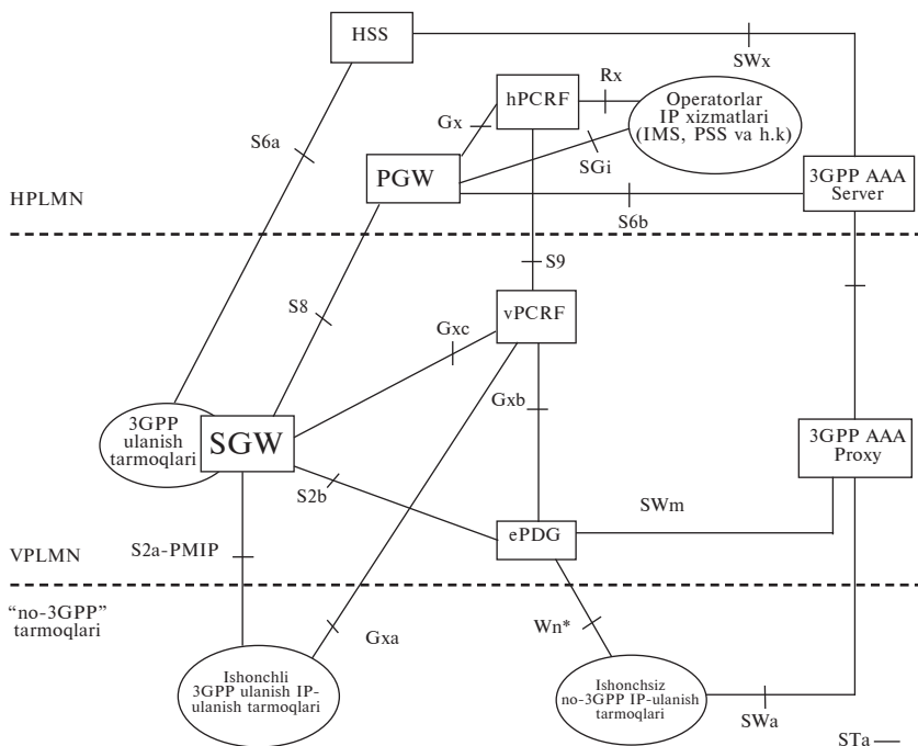
17.2-rasm. “Rouming” jarayonida LTE tarmoqlarining “no-3GPP” tarmoqlari bilan PMIPv6 protokoli asosida o‘zaro hamkorligi.
