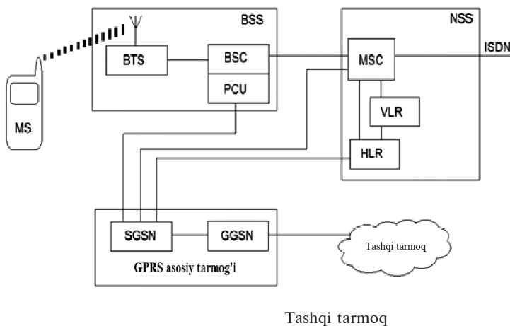
4.3-rasm. GRPS tarmog'ining tuzilish sxemasi.
