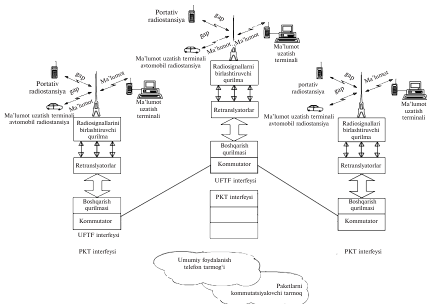
10.2-rasm. Zonalararo taqsimlangan kommutatsiyali trunking tizimning umumlashtirilgan strukturaviy sxemasi.
