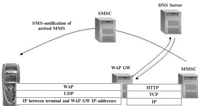
3.8-rasm. MMS bog‘lanuvchi qurilma.
