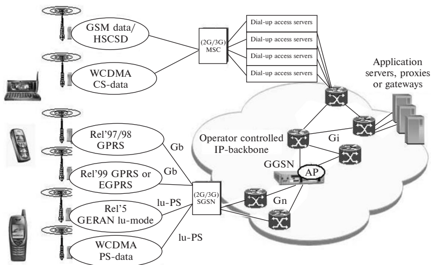
3.3-rasm. Uzatish kanali ulanishining turli variantlari.
