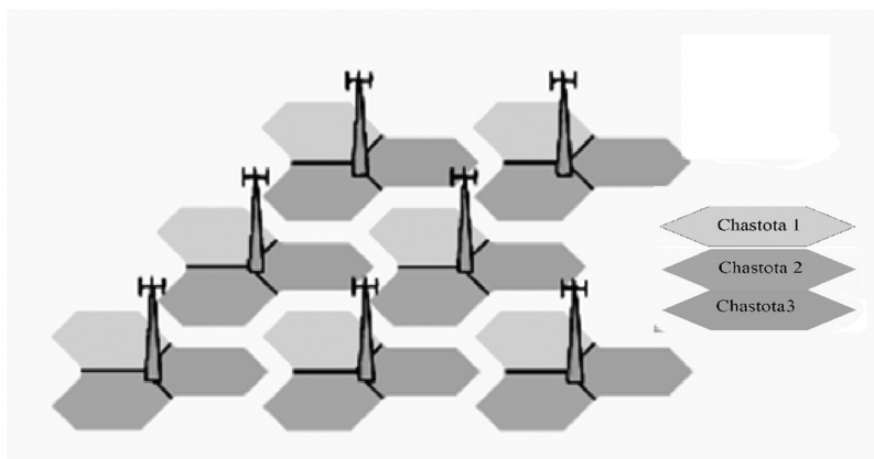
33.2-rasm. WiMAX tarmog‘ining sektorli arxitekturası.
