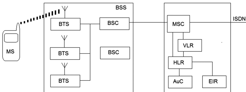
4.2-rasm. GSM tarmog‘ining tuzilish sxemasi.
