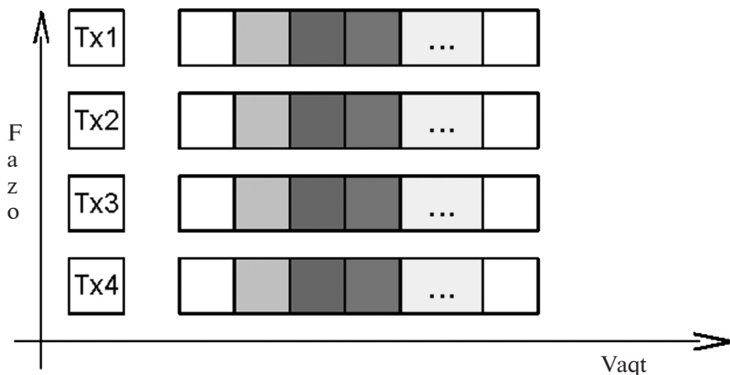
19.4-rasm. V-BLAST asosidagi fazoviy multiplekslash.
