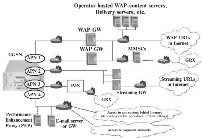
3.7-rasm. APNni proksiserverga bog’liqligi.
