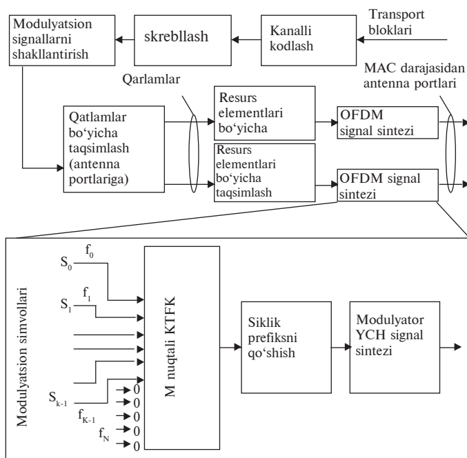
20.4-rasm. “Pastga” kanalda signalning shakllanish sxemasi.
