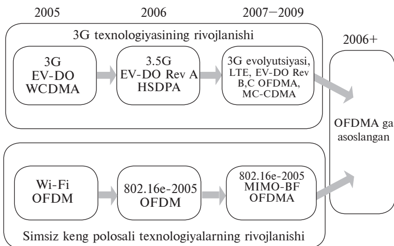
32.1-rasm. Keng polosali va mobil aloqa tizimlari evolyutsiyasi.
