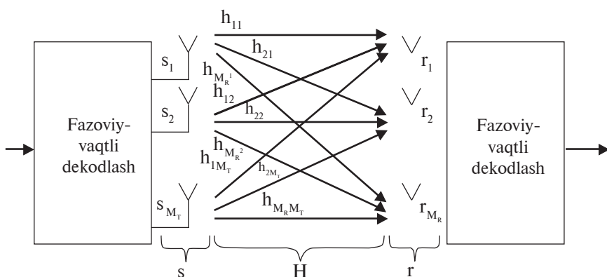
19.2-rasm. MIMO fizik kanali.
