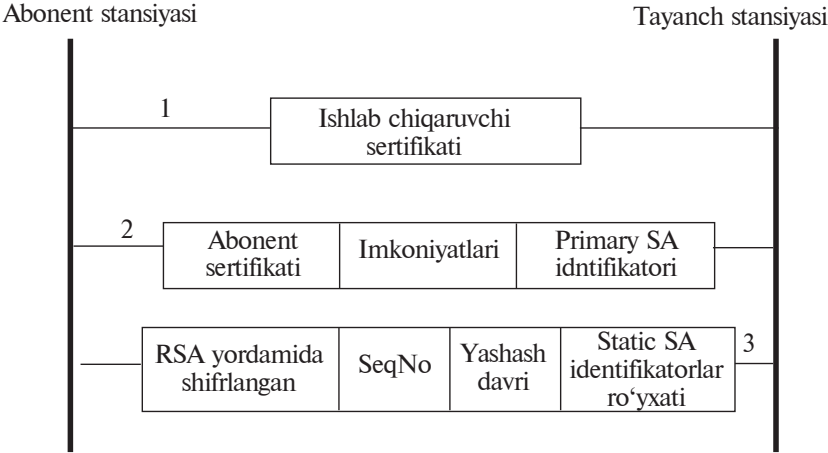
35.1-rasm. IEEE 802.16 standartidagi avtorizatsiya jarayoni.
