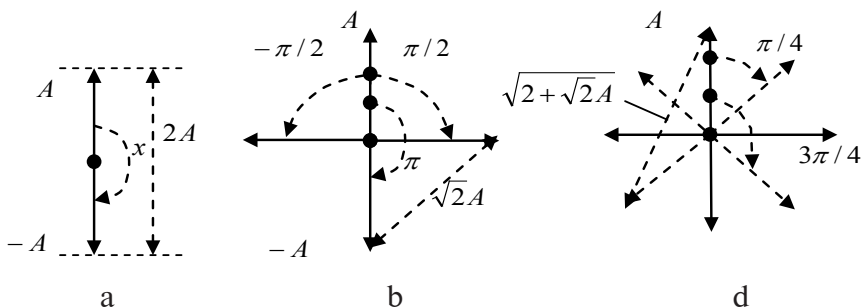
6.4-rasm. Har xil turdagi FMdagi oniy amplitudaning tafovuti.
