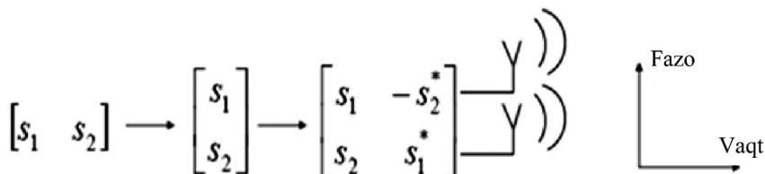
19.5-rasm. Ikki uzatuvchi antennalar uchun Alamouti fazoviy-vaqtli blokli kodlari.
