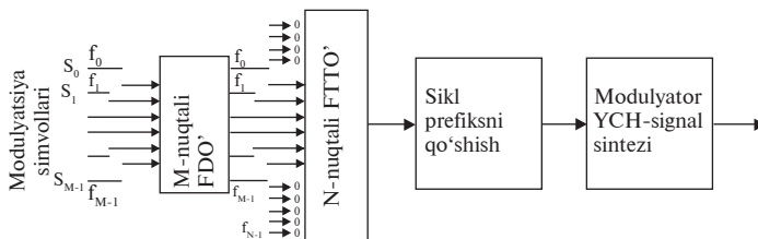
20.6-rasm. E-UTRAN tarmog‘idagi “yuqoriga” yo‘nalishda uzatishda SC-FDMA texnologiyasi yordamida signalni qayta ishlash sxemasi.
