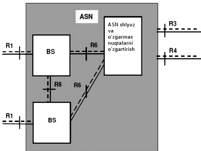
28.2-rasm. ASN tuzilmasi.
