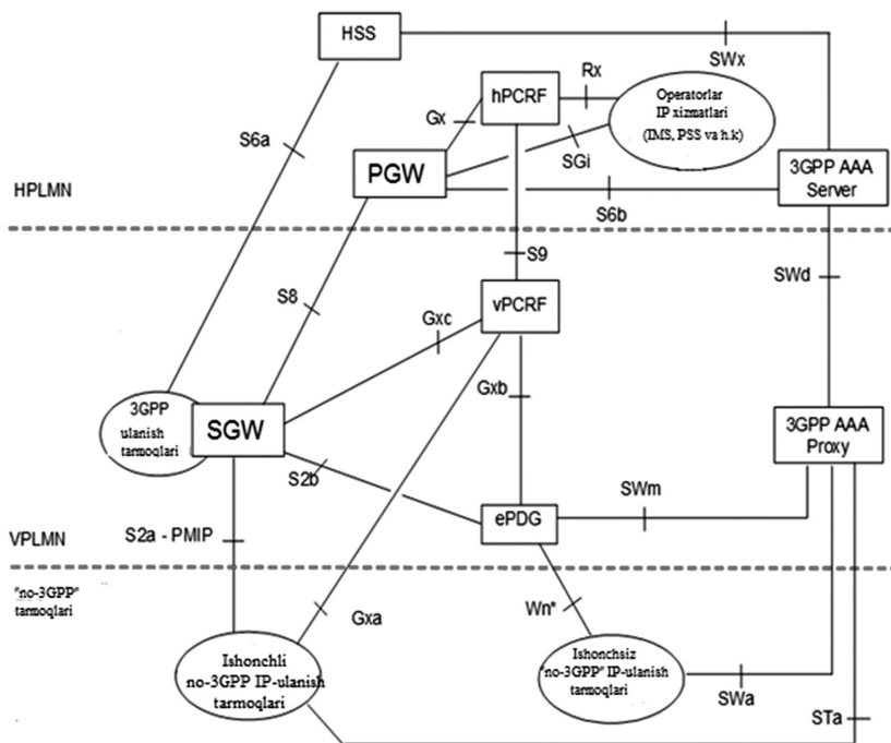
5.4-rasm. “Rouming” jarayonida LTE tarmoqlarining “no-3GPP” tarmoqlari bilan PMIPv6 protokoli asosida o‘zaro hamkorligi.
