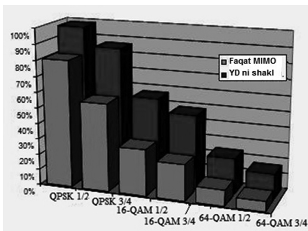
33.3-rasm. Har xil modulyatsiya va kodlash sxemalari turlarida ASS va MIMO texnologiyalari qo'llanilganda qamrab olinadigan hudud foizi.
