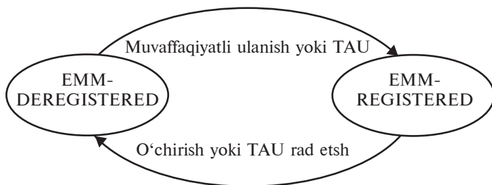
16.2-rasm. EMM darajasida A U ning mobillik holatlari.
