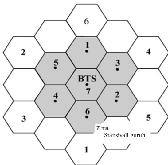
8.2-rasm. Chegaradosh qo‘shni stansiyalar guruhi.
