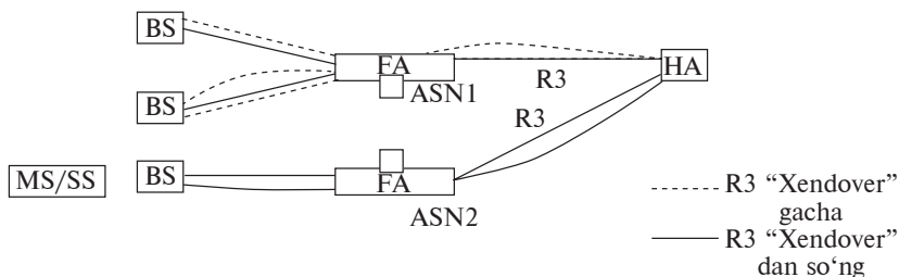
31.5-rasm. Mobillikni boshqarish turlarining aralash o'zaro ta'sirlashishi.
