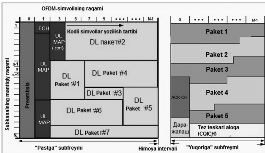
30.1-rasm. TDD usuli ishlatilgan OFDM kadrining tuzilmasi.
