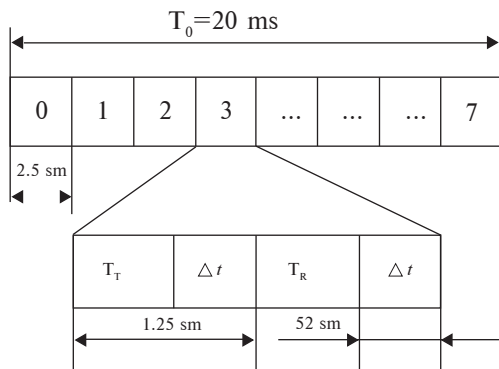
9.6-rasm. CDMA2000 tizimining TDDli aloqa kanali kadrining strukturasi.
