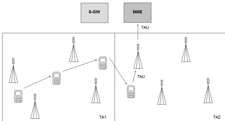
16.4-rasm. “Noaktiv LTE” holatida TAU jarayoni va “pastga” yo‘nalishda trafikni o‘tkazish jarayoni.
