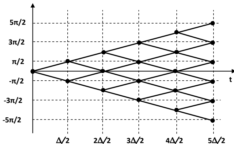
6.6-rasm. MCHM signalning oniy fazasining traektoriyalari.
