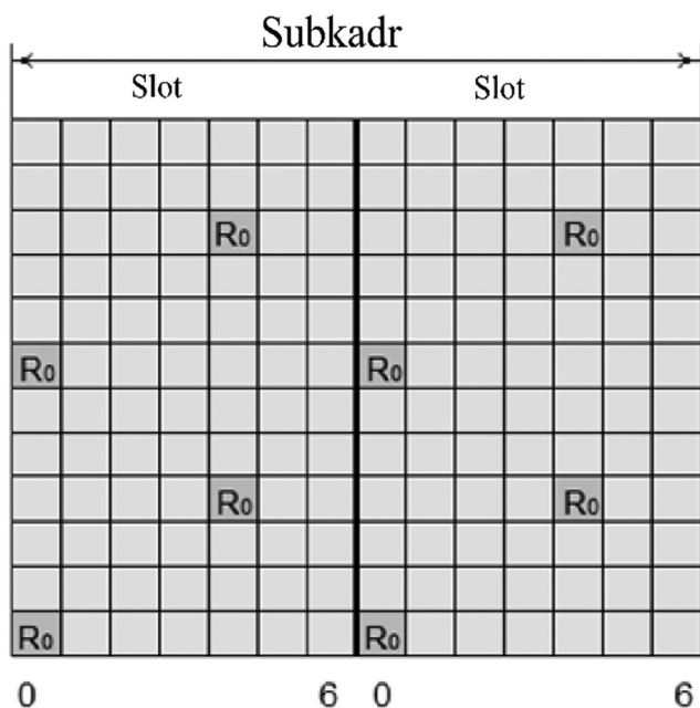
20.2-rasm. Standart SR uchun “pastga” yo‘nalishdagi signalning tuzilmasi.
