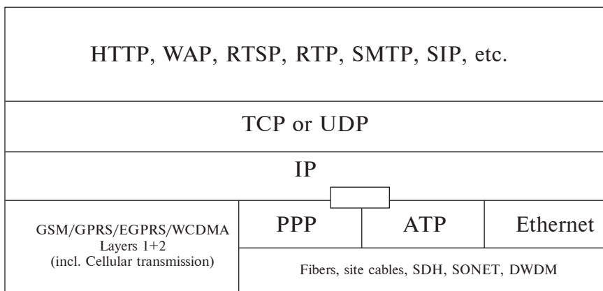
3.4-rasm. IP asosida ko'p sathli protokoli.
