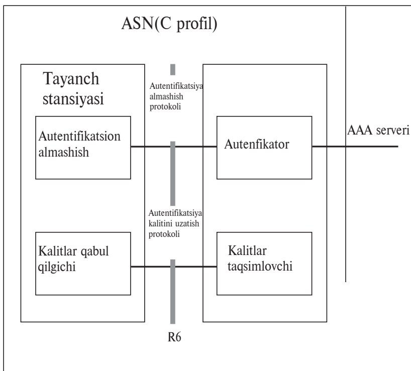
36.7-rasm. S profili uchun ASN tarmog'i xavfsizligi arxitekturası.
