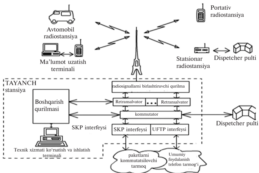
10.1-rasm. Bir zonali tranking tizimining umumlashtirilgan strukturaviy sxemasi.
