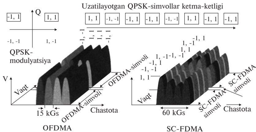
20.7-rasm. QPSK – simvollar ketma-ket uzatilishida OFDMA va SC-FDMA orasidagi farq.
