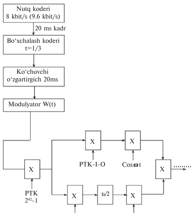
12.8-rasm. Ko'chma stansiyadagi signalning shakllanishi va qabul qiluvchi tayanch stansiyaning strukturaviy sxemasi.
