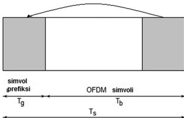
29.3-rasm. OFDM simvolning tuzilmasi.
