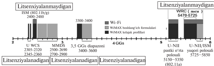
34.1-rasm. 2GGsdan 6 GGsgacha diapazonda KSU tizimlari uchun ruxsat etiladigan chastotalar polosasini.
