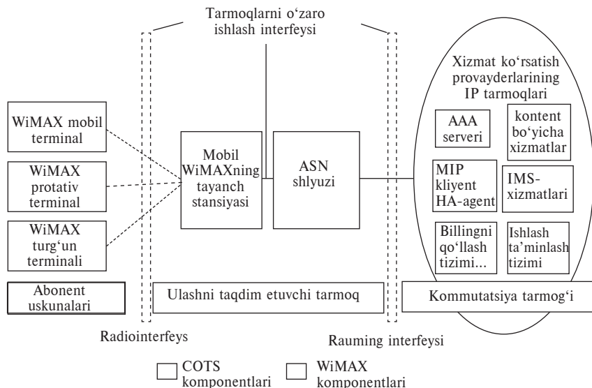
28.6-rasm. IP asosidagi WiMAX WiMAX tarmog'i arxitekturasini.
