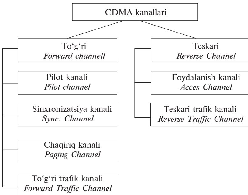
12.7-rasm. CDMA IS-95 standartidagi aloqa kanalining tuzilishi.
